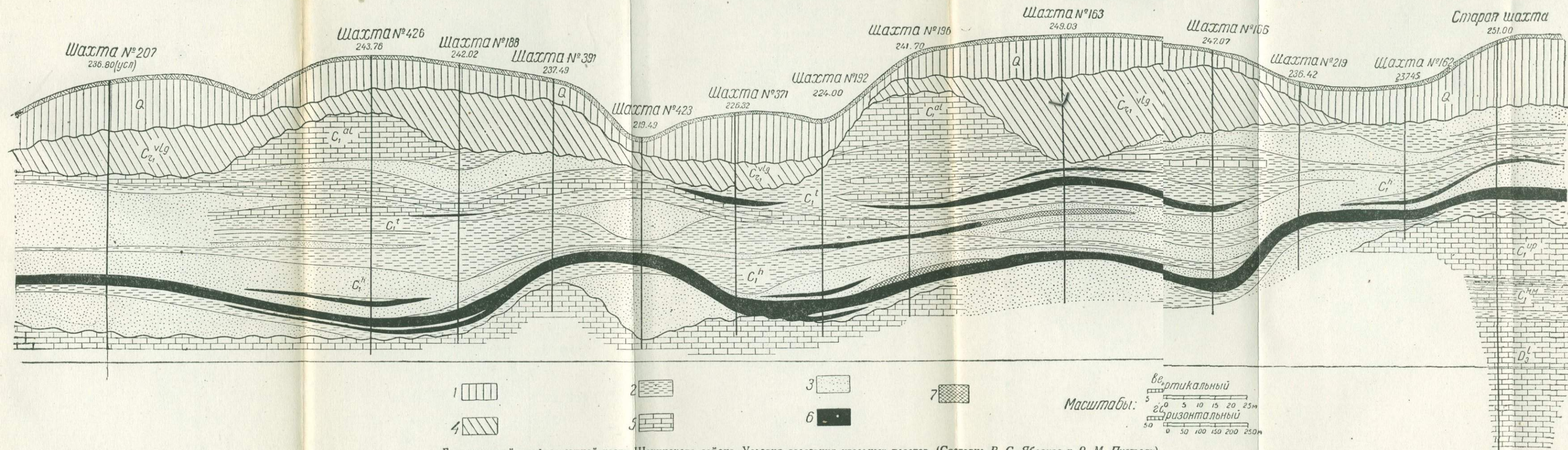
Геологический профиль южной части Шекинского района. Условия залегания угольных пластов. (Составил В. С. Яблоков и Р. М. Пистрак). 1 — жирная глина; 2 — глина; 3 — песок; 4 — глина и песок; 5 — известняк; 6 — уголь; 7 — сажистый уголь.
