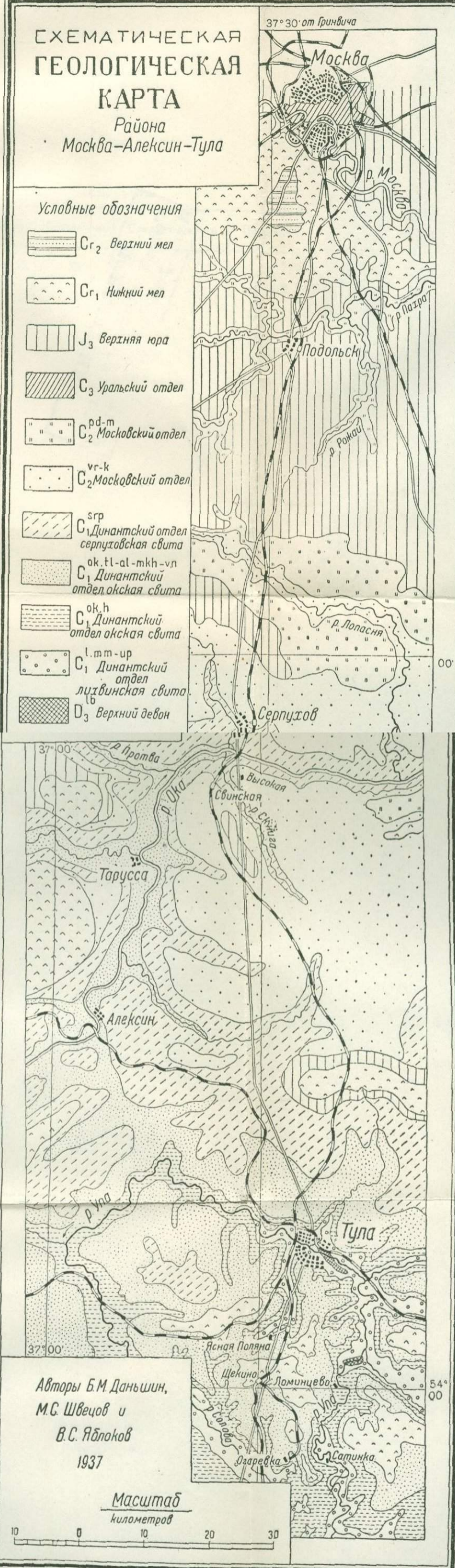
Схематическая геологическая карта полосы Москва — Алексин — Тула (по Б. М. Даньшину, М. С. Швецову, В. С. Яблокову).
