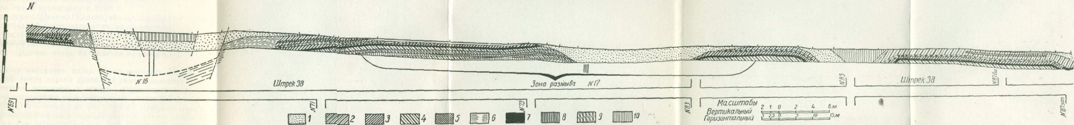
Рис. 5. Профиль — разрез угольного пласта по штрекам шахты № 6 (размыв пласта, карстовые нарушения). Составил В. С. Яблоков и Р. М. Пистрак.
