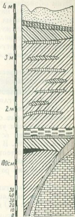
Рис. 4. Сводный разрез угольного пласта шахты № 5.
