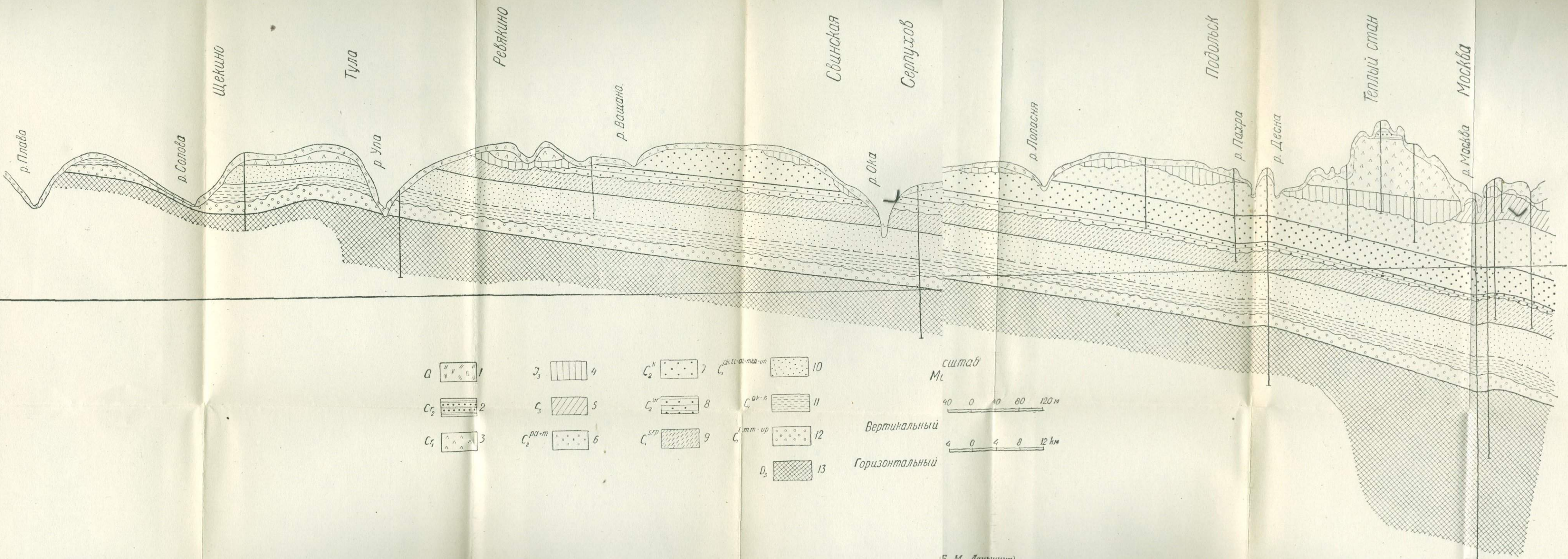
Геологический профиль (меридиональный) Щекино — Тула — Серпухов — Подольск — Москва. (По Б. М. Давышину). 1 — четвертичные отложения; 2 — верхний мел; 3 — нижний мел; 4 — верхняя юра; 5 — уральский отдел карбона; 6 — мячковская и подольская свита; 7 — каширекская свита; 8 — верейская свита; 9 — серпуховская свита; 10 — веневская, михайловская, алексинская, тульская толщи; 11 — угленосная толща; 12 — лихвинская свита; 13 — верхний девон.
