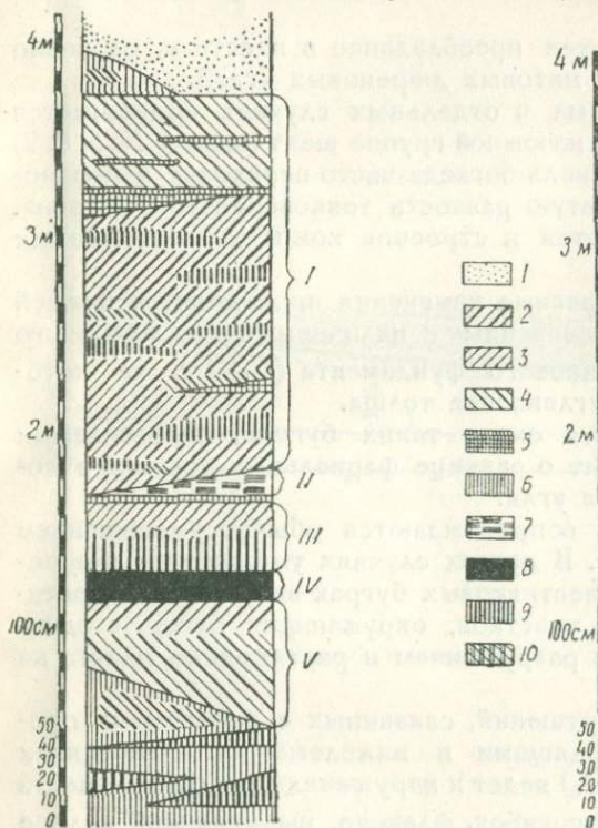
Рис. 3. Сводный схематический разрез главного угольного пласта Щекинского района Подмосковного бассейна
