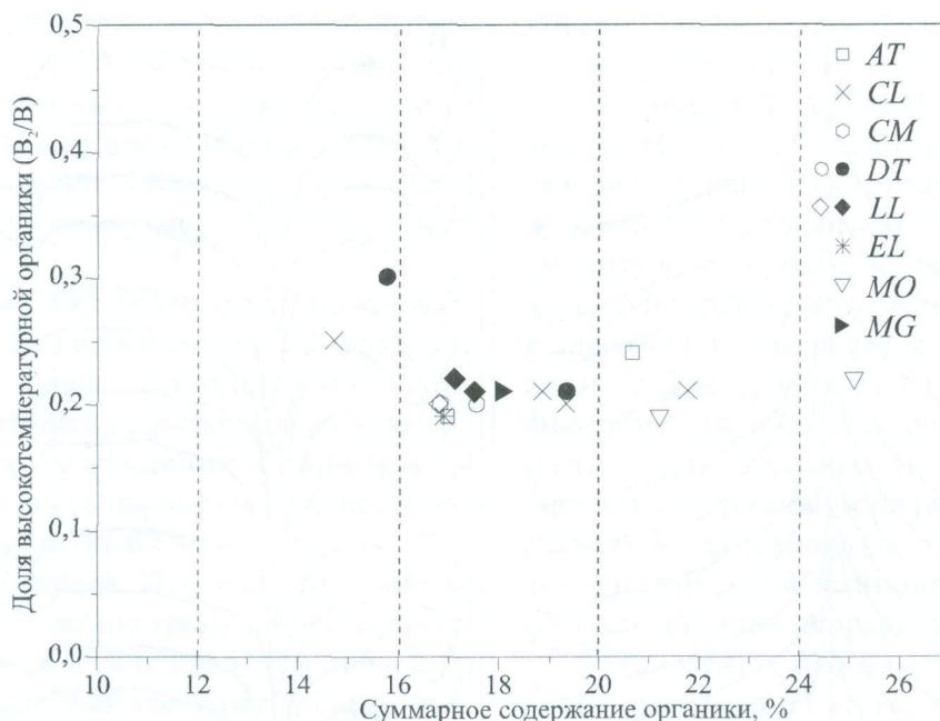
Рис. 2.14. Суммарное содержание органики и доля ее высокотемпературной формы B_2/B в костных фрагментах нижних челюстей грызунов из слоев 2 (гор. 5) и 5 (гор. 14–16) местонахождения Навес Светлый. Светлые знаки — образцы из слоя 2, черные знаки — образцы из слоя 5; AT — Arvicola terrestris , LL — Lagurus lagurus , EL — Eolagurus luteus , DT — Dicrostonyx torquatus , MG — Microtus gregalis , MO — Microtus oeconomus , CL — Clethrionomys sp. , CM — Cricetulus migratorius
