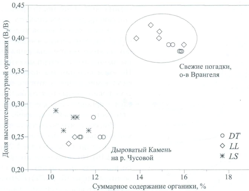
Рис. 2.17. Суммарное содержание органики и доля ее высокотемпературной формы V_2/V в щёчных зубах полевок из местонахождения Дыроватый Камень на р. Чусовой и свежих погадок полярных сов (о-в Врангеля). DT — Dicrostonyx torquatus из Дыроватого Камня на р. Чусовой, D. vinogradovi с о-ва Врангеля; LS — Lemmus sibiricus ; LL — Lagurus lagurus
