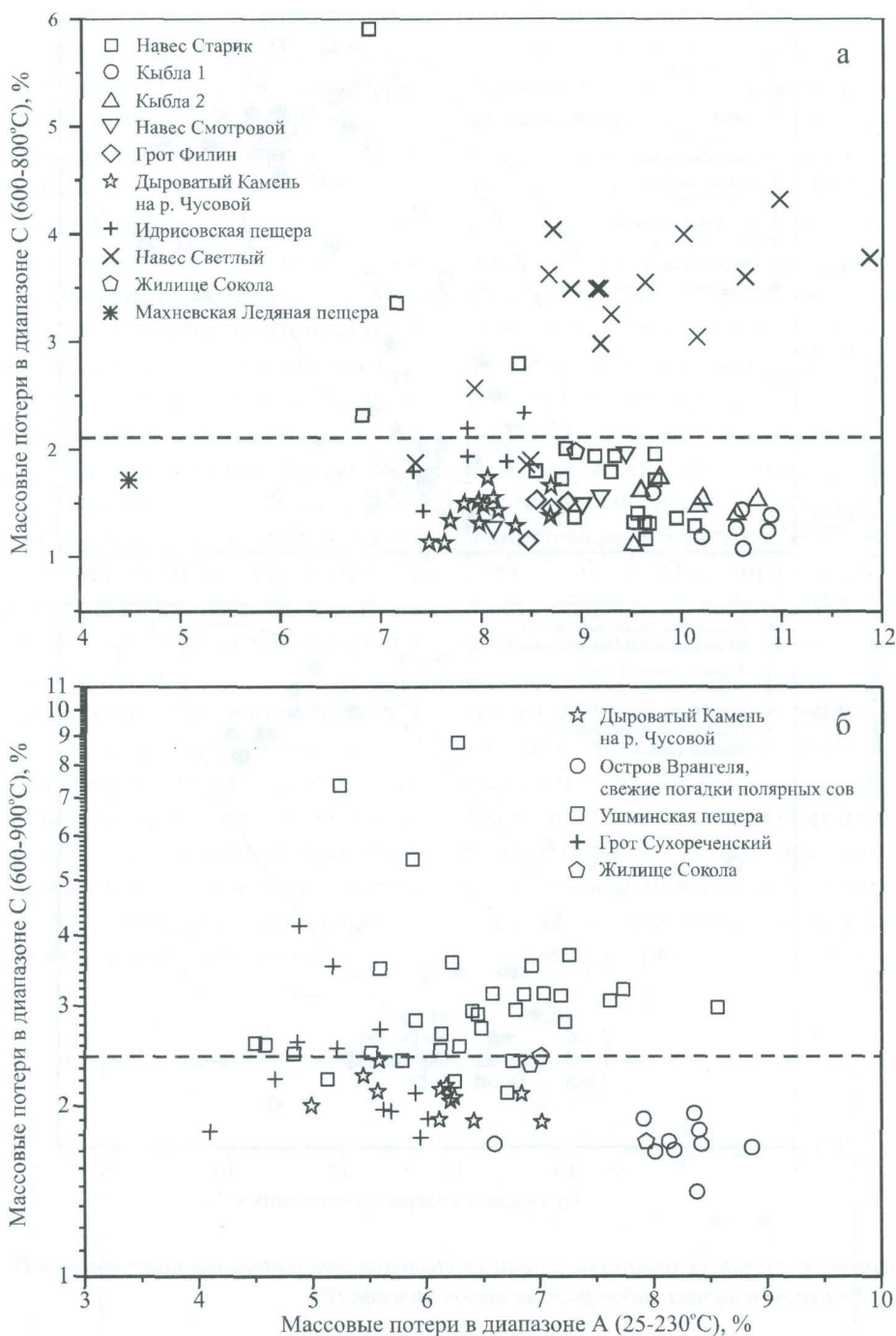
Рис. 2.4. Потери массы костных фрагментов (а) и щёчных зубов разных видов полевок (б) в температурных диапазонах А и С
