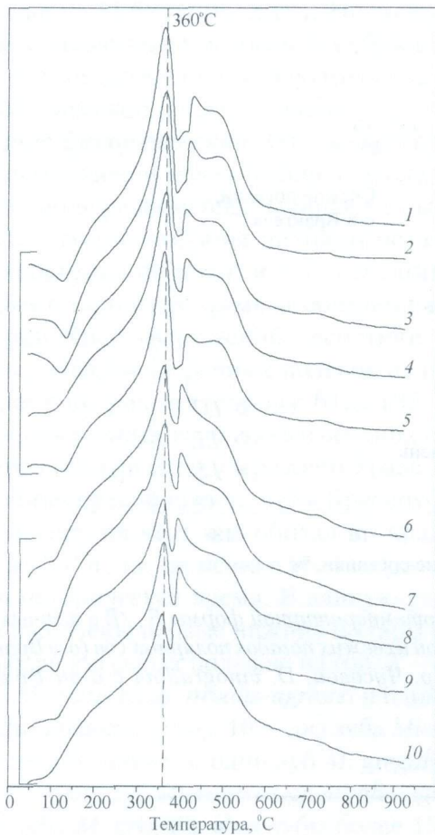
Рис. 2.16. Кривые ДТА зубов M^3 двух видов леммингов: Lemmus sibiricus (1–5) и Dicrostonyx vinogradovi (6–10), из свежих погадок полярных сов, собранных на о-ве Врангеля
