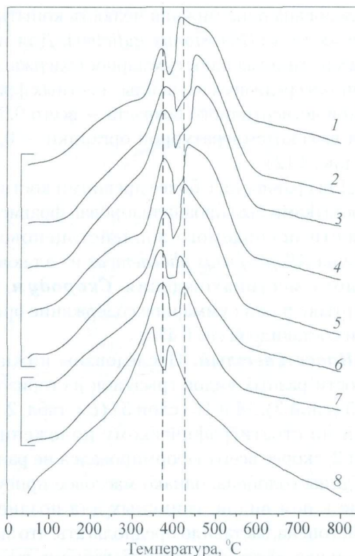
Рис. 2.10. Типичные кривые ДТА для костных фрагментов челюстей Arvicola terrestris из разных горизонтов местонахождения Навес Старик. Пунктиром обозначены средние температуры первого (370°C) и второго (420°C) экзопиков ДТА
