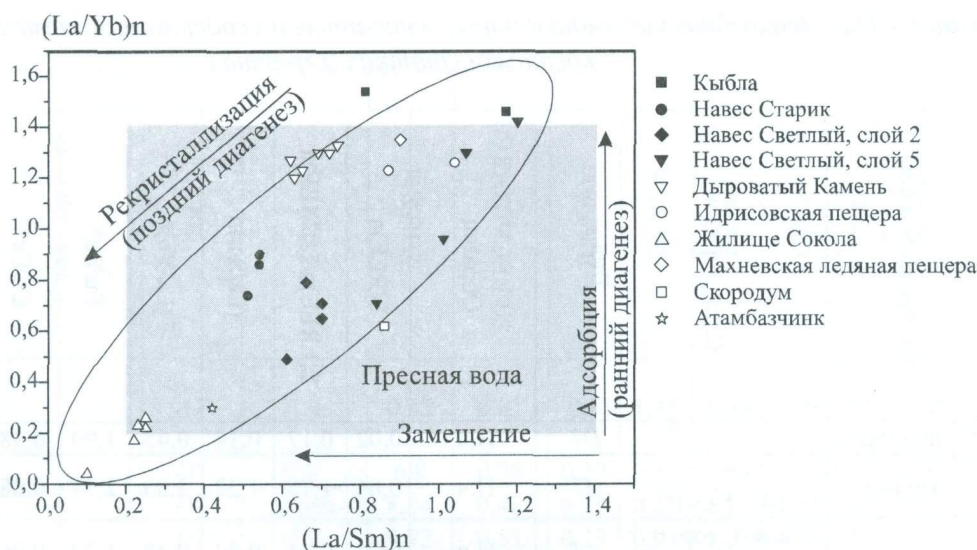
Рис. 3.9. Вариации отношений La/Sm и La/Yb в ископаемых костных остатках из различных местонахождений. Нормировка на пост-архейские австралийские сланцы PAAS, согласно McLennan (1989). Представлены данные для образцов, у которых суммарное содержание ВЗЭ составляет более 0,1 мкг/г.
