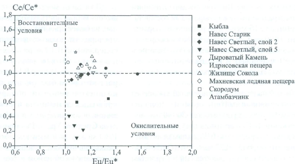
Рис. 3.12. Вариации европиевой Eu/Eu^* и цериевой Ce/Ce^* аномалий в ископаемых костных остатках из различных местонахождений. Представлены данные для образцов, у которых суммарное содержание ВЗЭ составляет более 0,1 мкг/г
