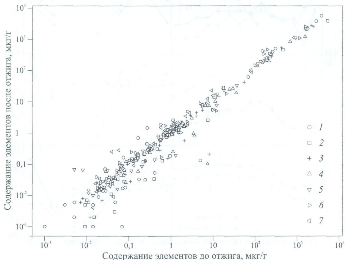
Рис. 3.6. Содержание элементов в костных остатках из различных местонахождений до и после их лабораторного отжига при 800°C
