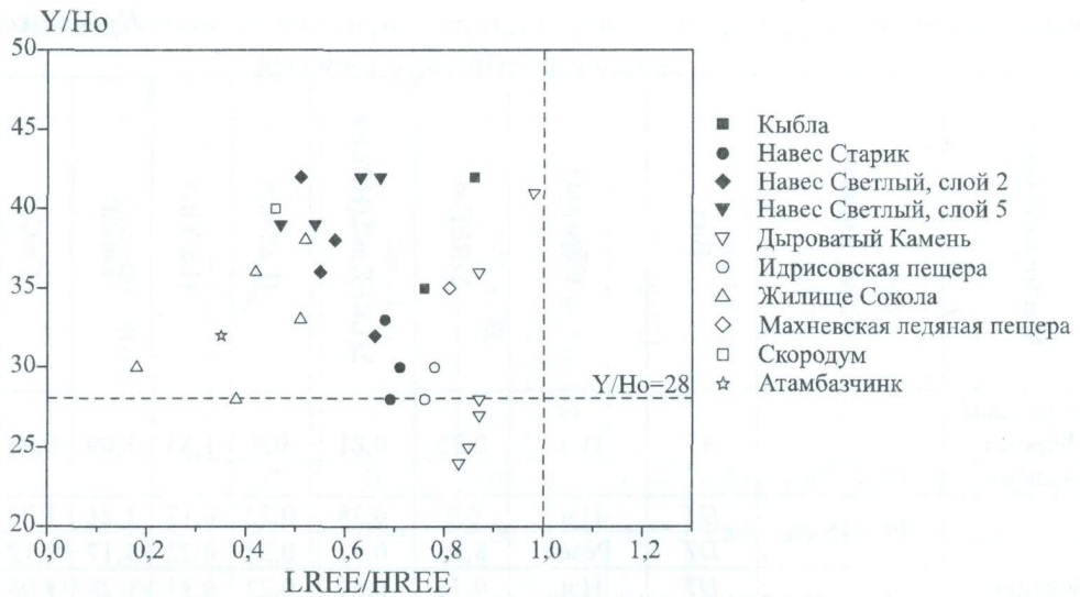
Рис. 3.11. Вариации соотношения легких-тяжелых РЗЭ и отношения Y/No в ископаемых костных остатках из различных местонахождений. Представлены данные для образцов, у которых суммарное содержание ВЗЭ составляет более 0,1 мкг/г
