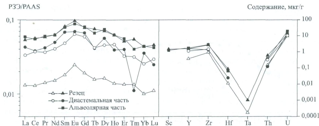
Рис. 3.3. Содержание РЗЭ (слева) и других ВЗЭ (справа) в разных фрагментах двух нижних челюстей Dicrostonyx torquatus из местонахождения Дыроватый Камень на р. Чусовой.
