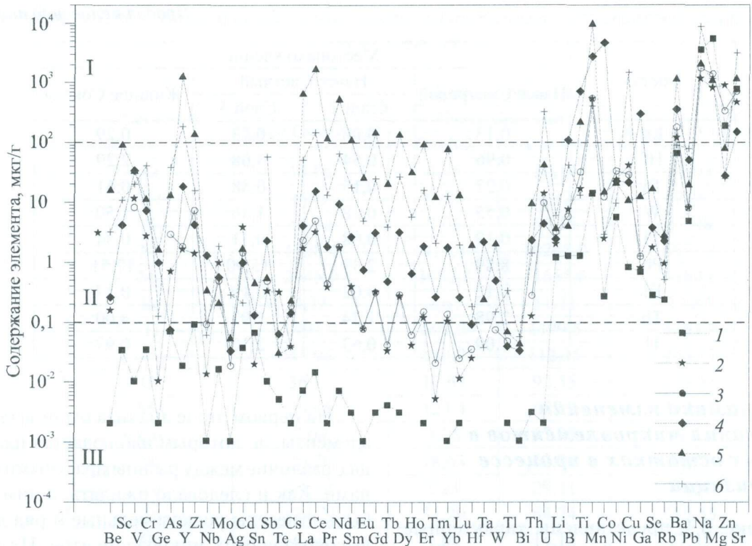
Рис. 3.1. Примеры распределения содержания макро- (I), микро- (II) и ультрамикроэлементов (III) в современных (1) и ископаемых (2–6) костных остатках разного возраста:
