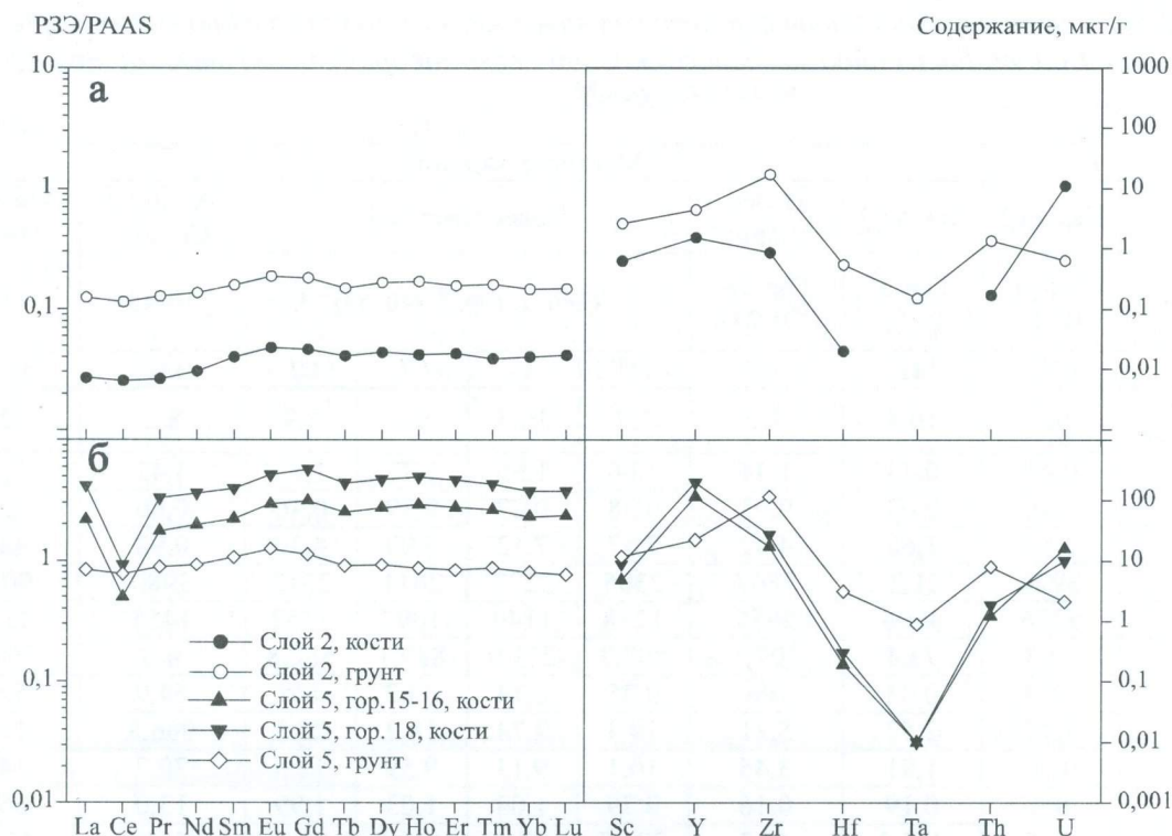
Рис. 3.5. Содержание РЗЭ (слева) и других ВЗЭ (справа) в костях (среднее) и грунтах из слоя 2 (а) и слоя 5 (б) местонахождения Навес Светлый. Нормировка РЗЭ на PAAS — постархейские австралийские сланцы
