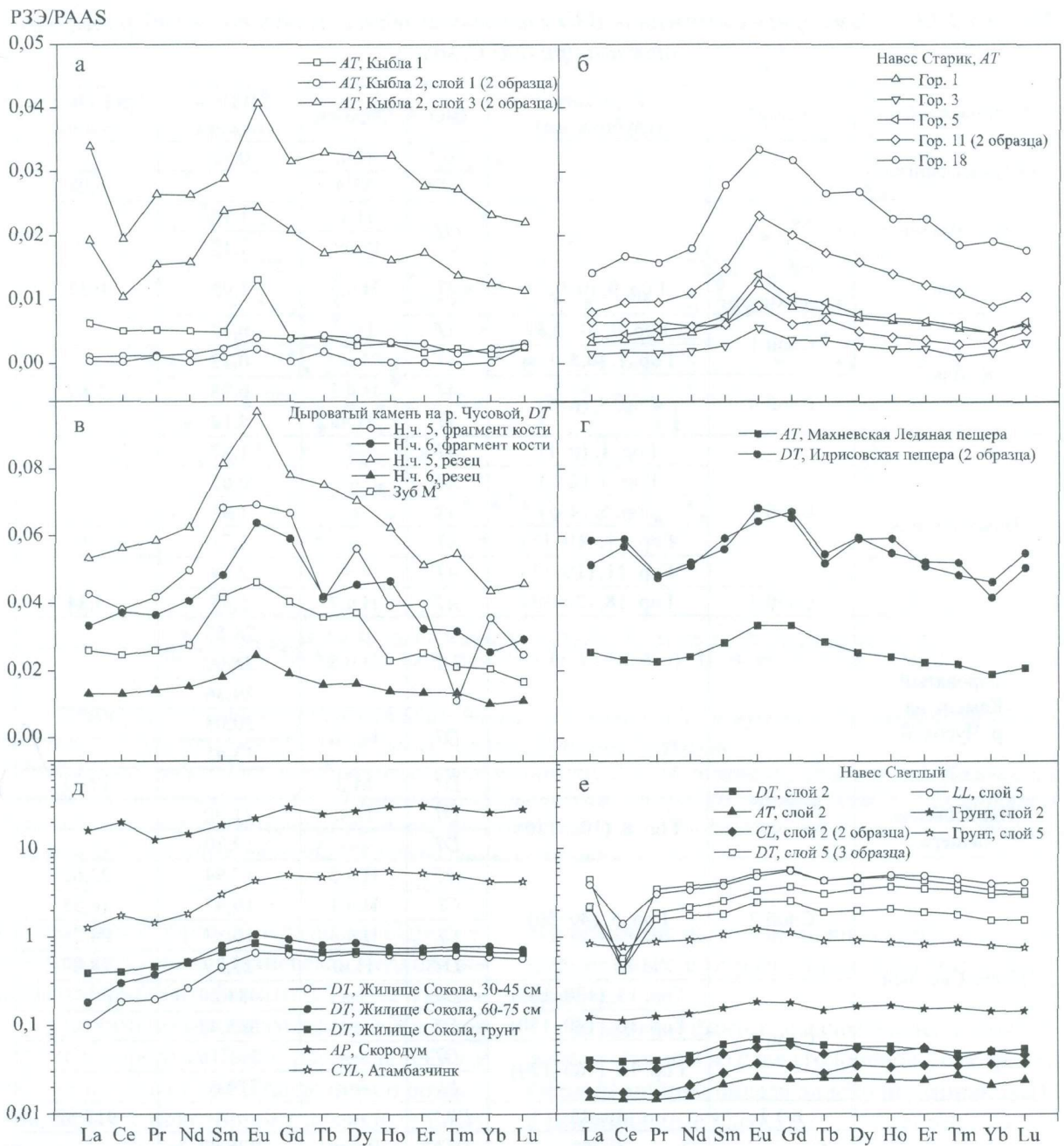
Рис. 3.2. Примеры распределений ПЗЭ в ископаемых фрагментах челюстей (а–е), зубах (в) разных видов грызунов и грунтах (д, е) из различных местонахождений. Нормировка на пост-архейские австралийские сланцы – PAAS.
