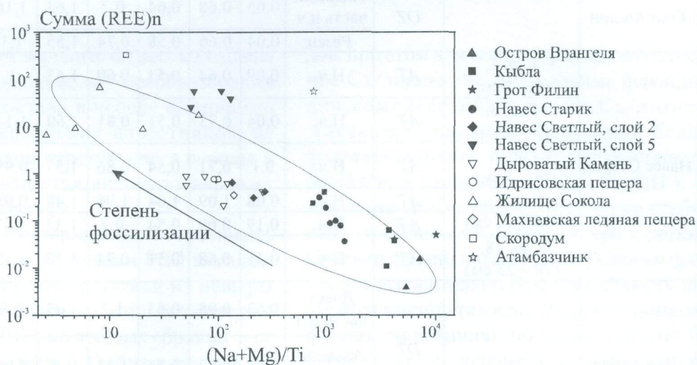
Рис. 3.10. Суммарное содержание РЗЭ и отношение (Na+Mg)/Ti в ископаемых костных остатках из различных местонахождений
