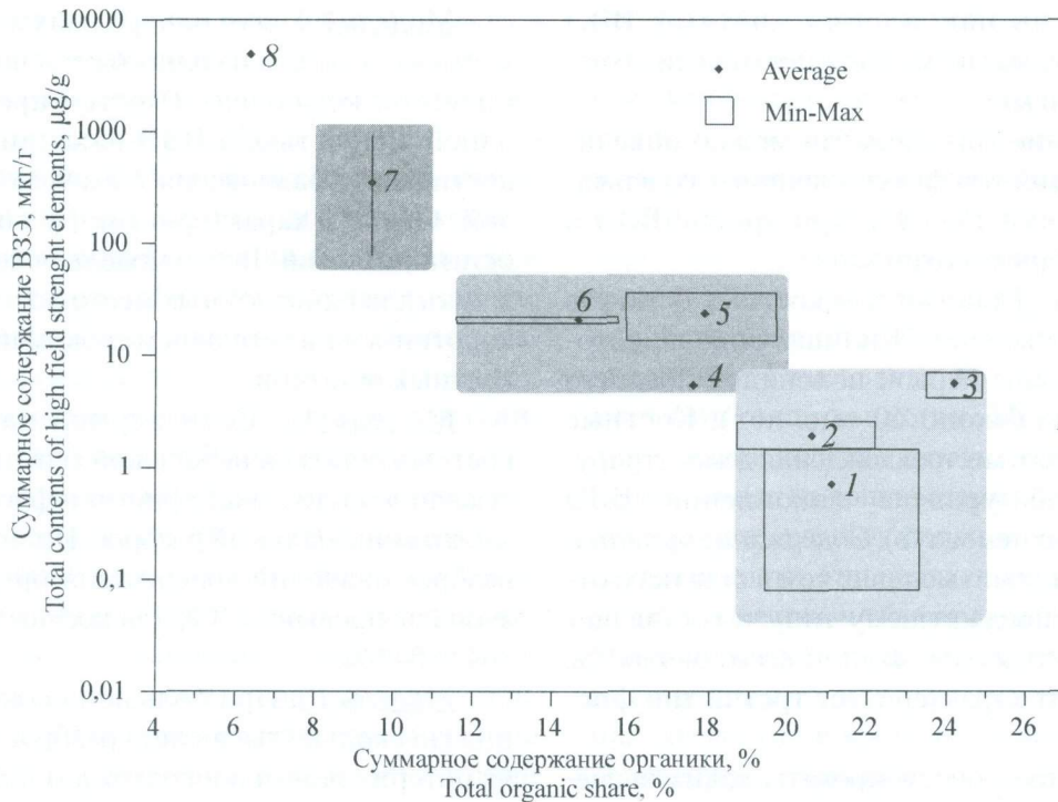
Рисунок. Тенденции изменения содержания органической компоненты и накопления ВЗЭ для остатков, относимых к разным типам фоссилизации.
