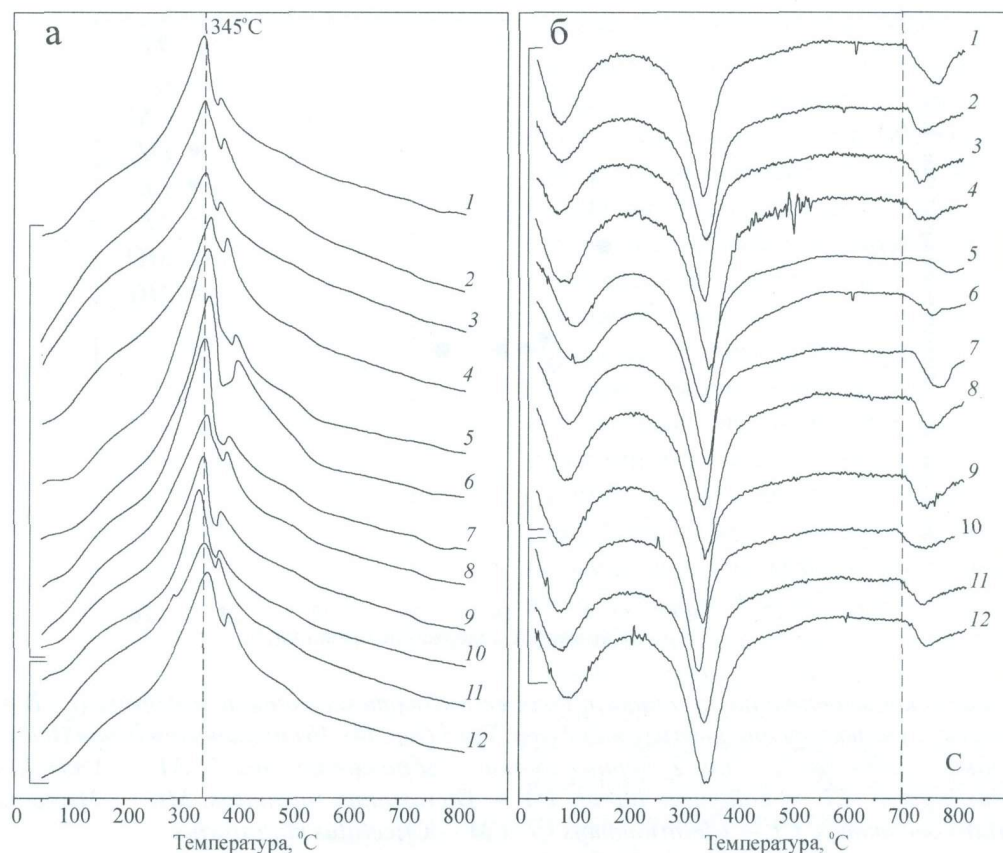
Рис. 2.13. Типичные кривые ДТА (а) и ДТГ (б) костных фрагментов челюстей разных видов полевок из слоя 2 (кривые 1–9) и слоя 5 (кривые 10–12) местонахождения Навес Светлый.
