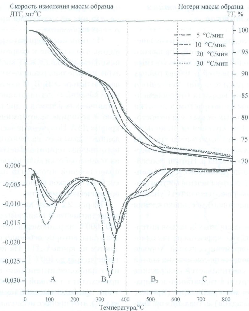
Рис. 2.1. Кривые ТГ (вверху) и ДТГ (внизу), полученные при разных скоростях нагревания для четырех сходных фрагментов челюстей водяных полевок ( Arvicola terrestris ) из горизонта 3 местонахождения Навес Старик
