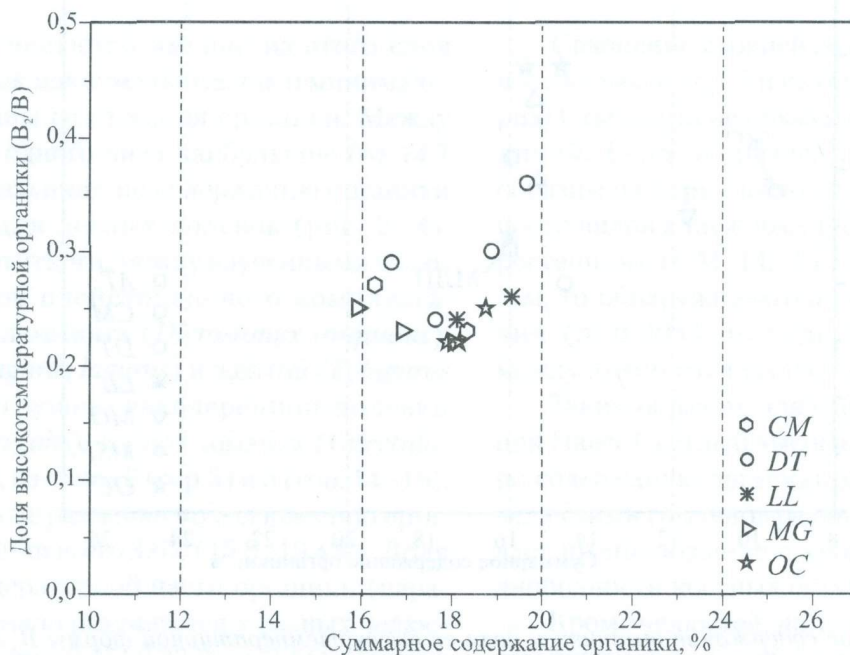
Рис. 2.11. Суммарное содержание органики и доля ее высокотемпературной фракции V_2/V в костных фрагментах нижних челюстей грызунов из местонахождения Дыроватый Камень на реке Чусовой. CM — Cricetulus migratorius , DT — Dicrostonyx torquatus , LL — Lagurus lagurus , MG — Microtus gregalis , OC — Ochotona sp.
