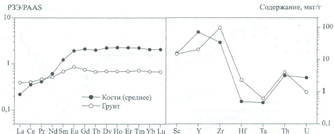
Рис. 3.4. Содержание PЗЭ (слева) и других ВЗЭ (справа) в костях и грунте из местонахождения Жилище Сокола. Нормировка PЗЭ на PAAS — постархейские австралийские сланцы
