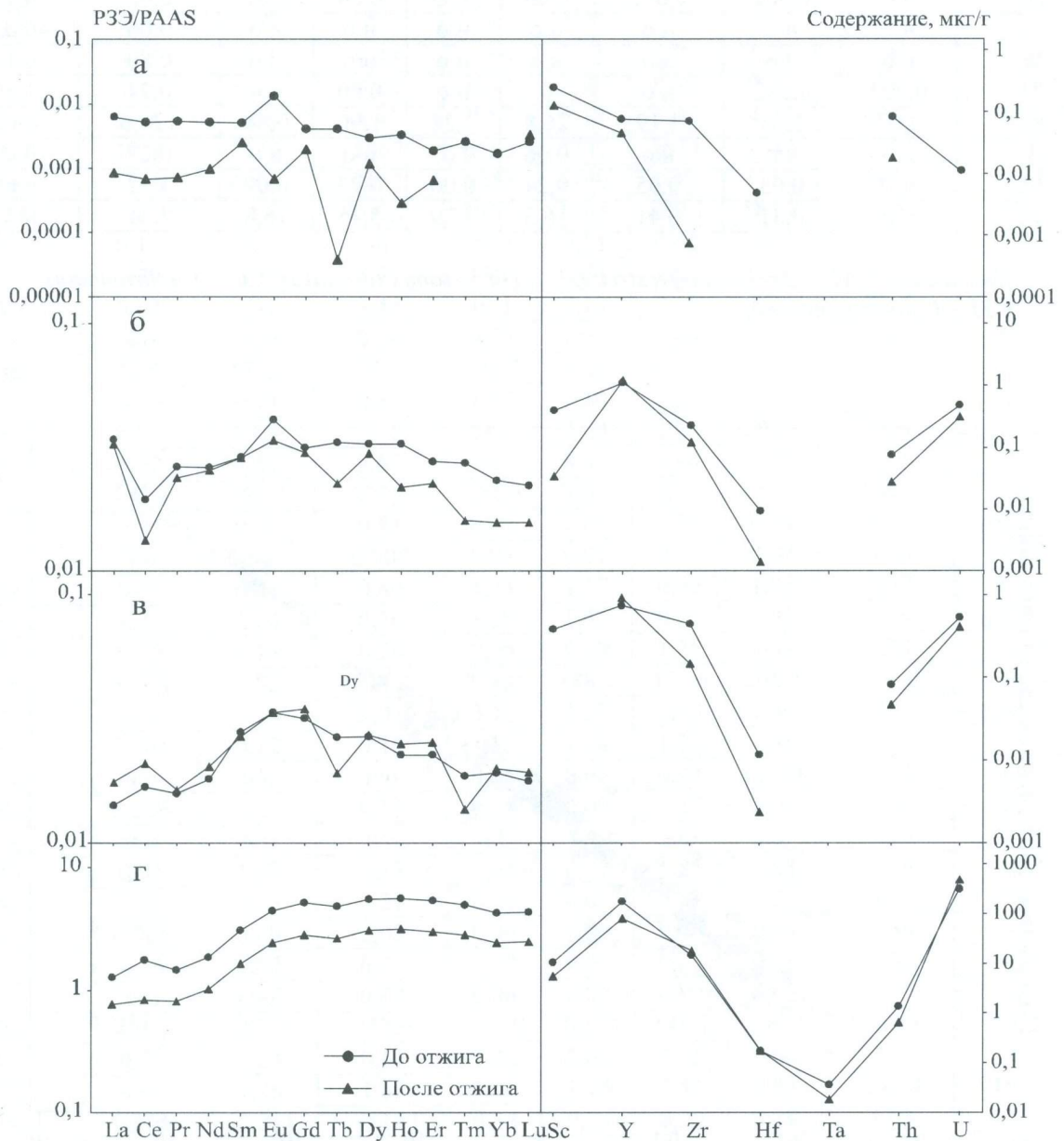
Рис. 3.7. Содержание РЗЭ (слева) и других ВЗЭ (справа) в образцах до и после лабораторного отжига при 800^\circ\text{C} . Нормировка РЗЭ на PAAS — постархейские австралийские сланцы.
