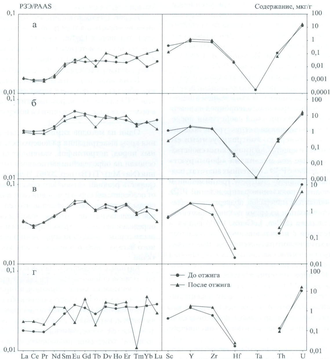
Рис. 3.8. Содержание РЗЭ (слева) и других ВЗЭ (справа) в нижних челюстях разных видов полевок из слоя 2 (гор. 5) местонахождения Навес Светлый до и после лабораторного отжига при 800°С. Нормировка РЗЭ на PAAS — постархейские австралийские сланцы.
