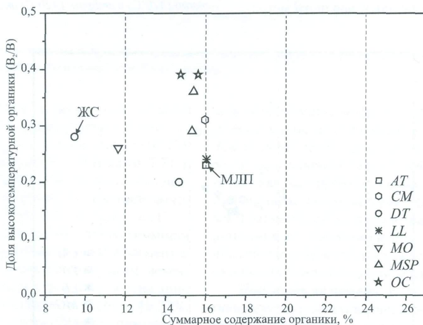
Рис. 2.12. Суммарное содержание органики и доля ее высокотемпературной формы V_2/V в костных фрагментах нижних челюстей грызунов из местонахождений Идрисовская пещера, Жилище Сокола (ЖС) и Махневская Ледяная пещера (МЛП).
