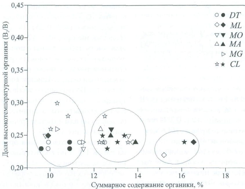
Рис. 2.18. Суммарное содержание органики и доля ее высокотемпературной формы V_2/V в щёчных зубах полевок из слоев 1 и 3 Ушиминской пещеры.
