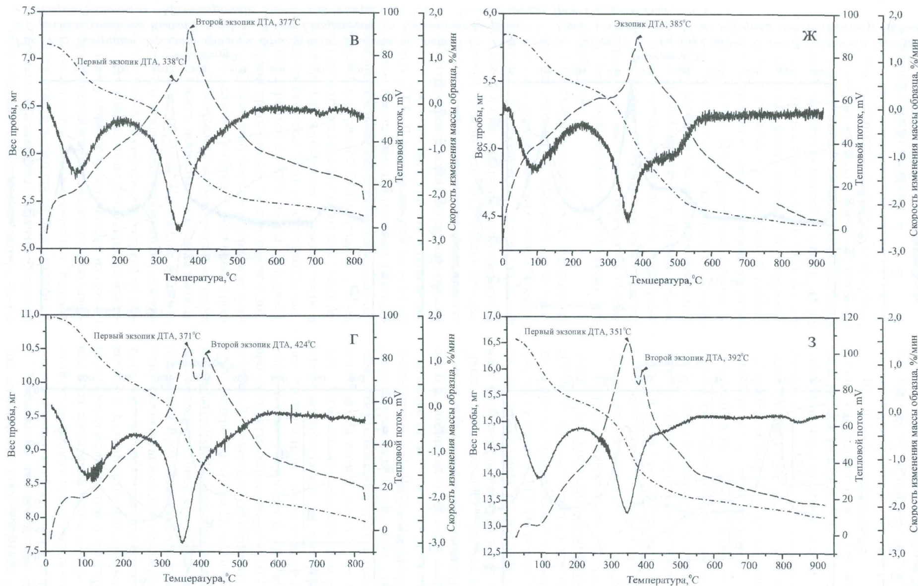
Продолжение рис. 2.2. Типичные дериватограммы фрагментов нижних челюстей (а-г) и щёчных зубов (д-з) разных видов полевок: Arvicola terrestris : а – местонахождение Кыбла 2, гор. 1, г – Навес Старик, гор. 18; Dicrostonyx torquatus : б – Навес Светлый, гор. 14; в, з - Дыроватый Камень на р. Чусовой, е - Остров Врангеля; д – Microtus gregalis , Ушминская пещера, слой 3; ж д – Microtus arvalis , Грот Сухореченский, гор. 3
