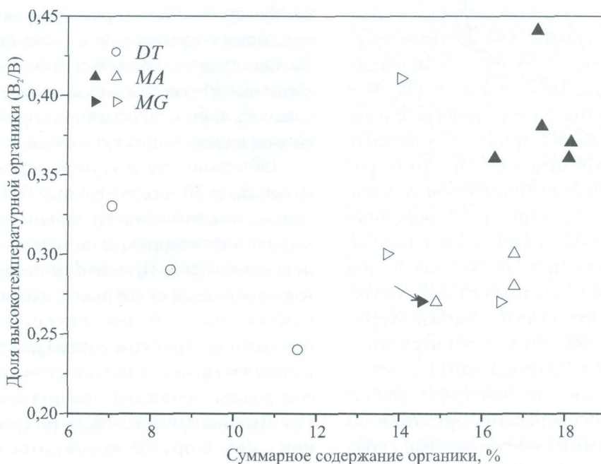
Рис. 2.19. Суммарное содержание органики и доля ее высокотемпературной формы V_2/V в щёчных зубах серых полевок из разных слоев Грота Сухореченского и копытных леммингов из пещеры Жилище Сокола. Черные знаки — образцы из гор. 3 Грота Сухореченского, белые — образцы из гор. 10, 11 Грота Сухореченского и из пещеры Жилище Сокола; DT — Dicrostonyx guillemi , MA — Microtus ex gr. arvalis-agrestis , MG — Microtus gregalis
