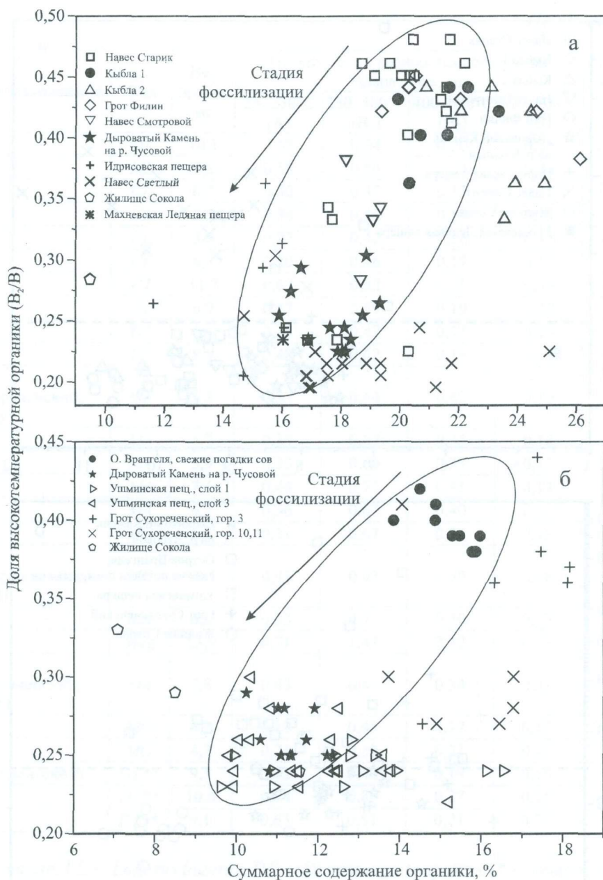
Рис. 2.5. Суммарное содержание органики и доли ее высокотемпературной компоненты V_2/V в костных фрагментах (а) грызунов и щёчных зубов разных видов полевок (б)
