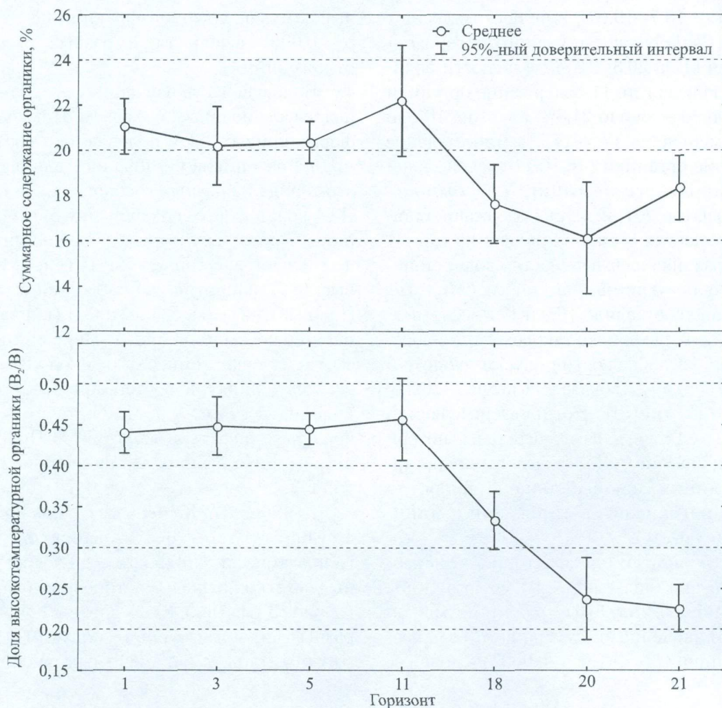
Рис. 2.9. Изменение суммарного содержания органики и доли ее высокотемпературной компоненты с ростом горизонта отложений местонахождения Навес Старик.
