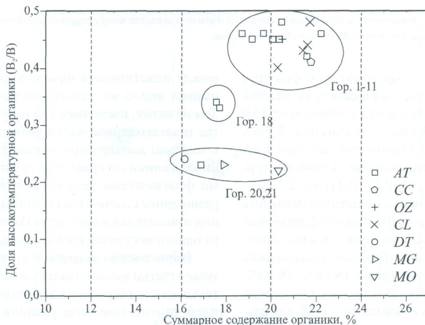
Рис. 2.8. Суммарное содержание органики и доля ее высокотемпературной формы B_2/B в костных фрагментах нижних челюстей грызунов из местонахождения Навес Старик.
