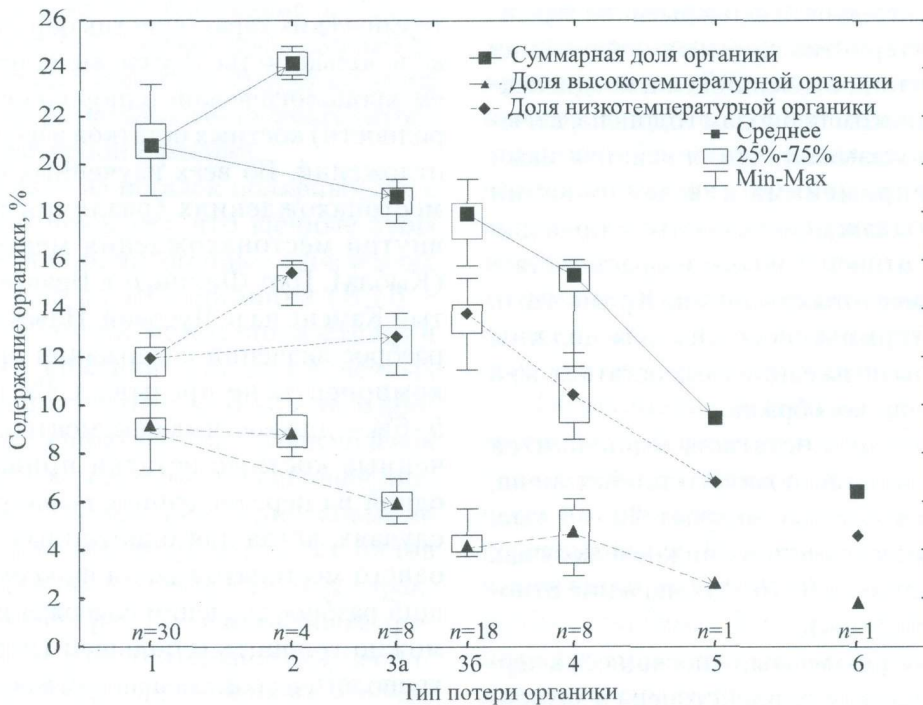
Рис. 2.20. Усредненные тенденции изменения содержания органики в нижнечелюстных костях грызунов плейстоценового и голоценового возраста, находящиеся на разных стадиях фоссилизации.
