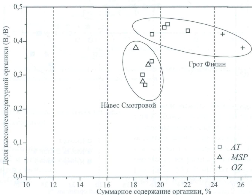
Рис. 2.7. Суммарное содержание органики и доля ее высокотемпературной формы V_2/V в костных фрагментах диастем нижних челюстей грызунов из местонахождений Грот Филин и Навес Смотровой. OZ — Ondatra zibethicus , AT — Arvicola terrestris , MSP — Microtus sp.
