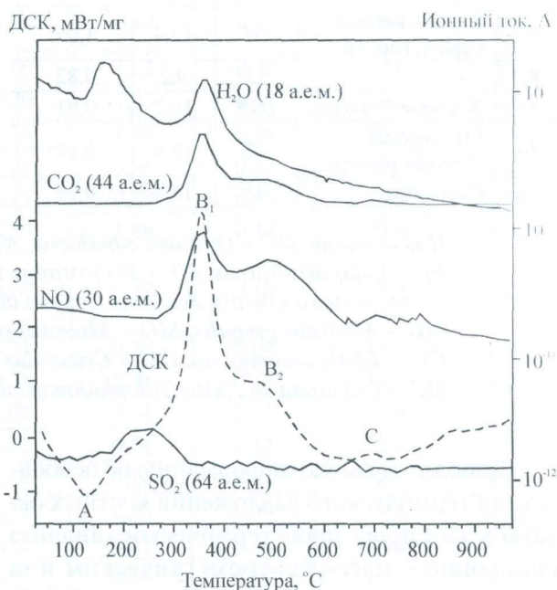
Рис. 2.3. ДТА (ДСК)-кривая зуба M 1 копытного лемминга ( Dicrostonyx vinogradovi ) из современных погадок с о-ва Врангеля с наложением спектров синхронного масс-спектрометрического анализа выделившихся газов
