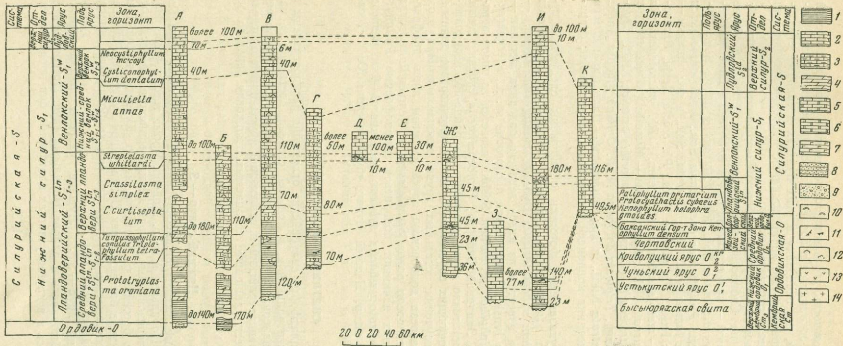
Рис. 35. Схема сопоставления главнейших разрезов ордовика и силура Сибирской платформы по ругозам
