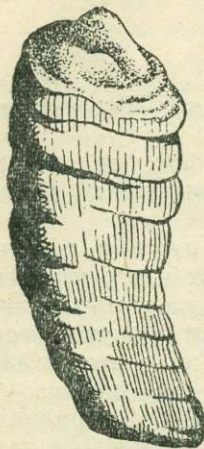
Рис. 16. Cyathactis tyurus Soshk. Нат. вел. Общий вид полипняка. Руч. Потерянный (43)
