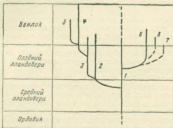
Рис. 31. Схема развития семейств Arachnophyllidae и Endophyllidae
