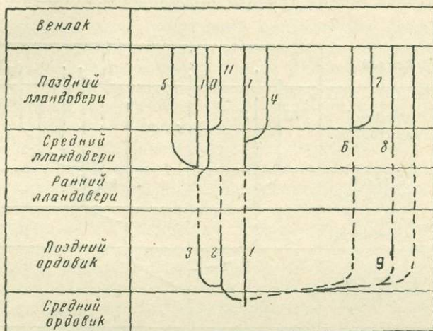
Рис. 28. Схема развития семейств Streptelasmatidae и Dinophyllidae (по материалам с Сибирской платформы, как и в последующих случаях)
