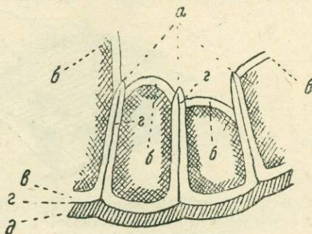
Рис. 22. Схема соотношения септ, днищ, периферического ободка и эпитеки Tabularia septata sp. n. на поперечном разрезе.
