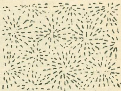
Рис. 5. Схематическое изображение массивной астреовидной колонии Palaeareaea lopatini (Lindstr.), Нат. вел.
