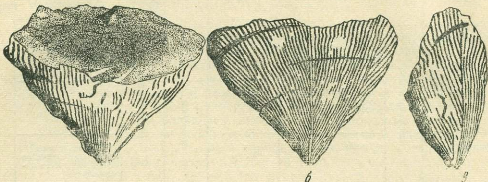
Рис. 15. Holophragma calceoloides (Lindstr.). \times 2 .
