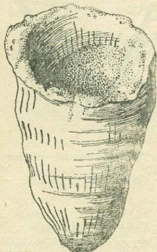
Рис. 26. Cysticonophyllum dentatum sp. n. \times 3 . Общий вид полипняка. Р. Мойеро (55)
