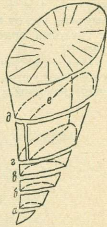
Рис. 9. Примерная ориентировка пластинок шлифов (a—e)
