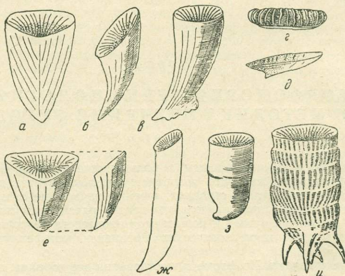
Рис. 2. Внешняя форма одиночных ругоз.
