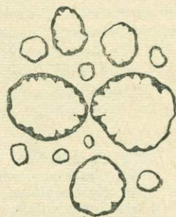
Рис. 24. Aphyllum sociale Soshk., \times 4 . Поперечное сечение колонии Р. Мойеро (66)
