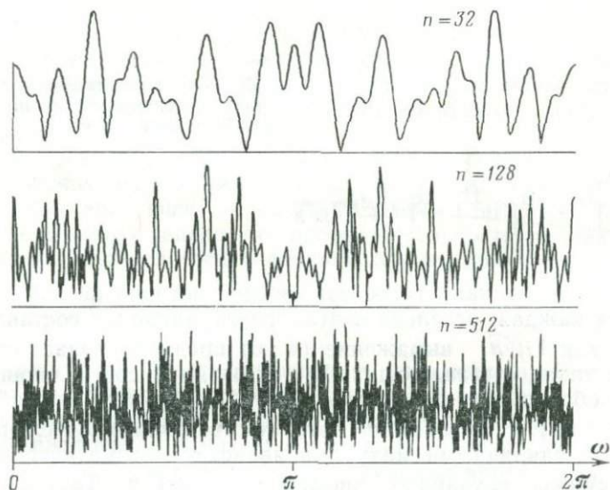
РИС. 4.2. Амплитудные спектры [\widehat{R}(Z)]^{1/2} выборки из n случайных чисел. Функции осциллируют с одинаковой амплитудой как при n=512 , так и при n=32 . При n \rightarrow \infty следует ожидать неограниченного увеличения частоты колебаний
