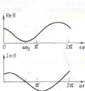
Рис. 2.4. Действительная и мнимая части Z -преобразования функции 1 - Z/(1,25e^{i2\pi/3})
