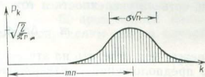
РИС. 4.9. Коэффициенты многочлена [Z^n (Z^z + Z^{-z})/2]^n
