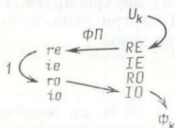
РИС. 3.4. Определение фазовой функции.
