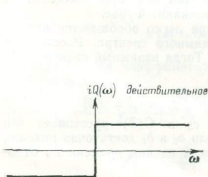
РИС. 1.13. Частотная характеристика фильтра, смещающего фазу на 90^\circ .
