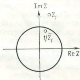
РИС. 3.1. Корни функции B(1/Z)B(Z)
