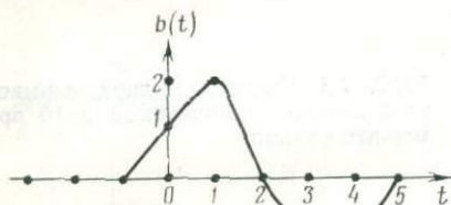
РИС. 1.1. Дискретное представление непрерывной функции времени через одинаковые временные интервалы
