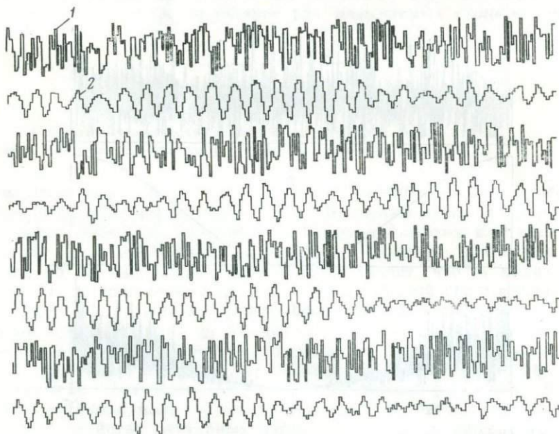
РИС. 4.7. Выборка из 1024 случайных чисел до (1) и после (2) узкополосной фильтрации. Фильтр описывается выражением
