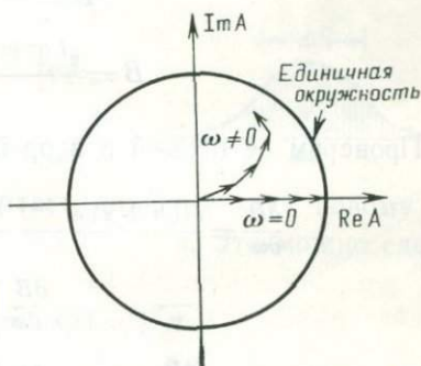
РИС. 4.8. Сложение комплексных чисел a_k e^{i\omega k}
