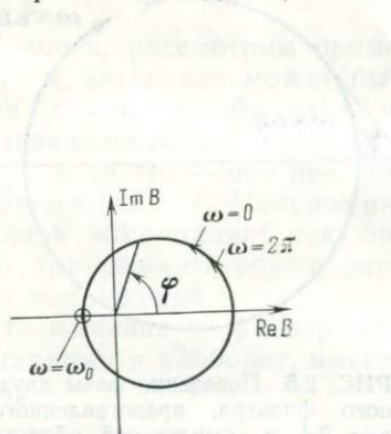
РИС. 2.8. Поведение фазы в комплексной плоскости
