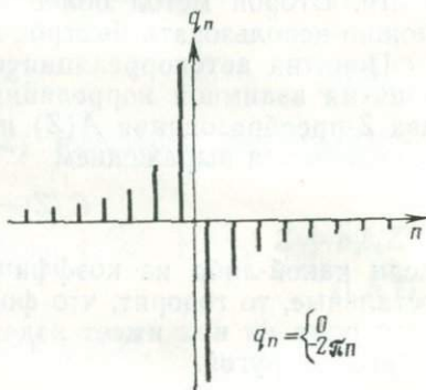
РИС. 1.14. Коэффициенты квадратурного фильтра
