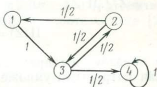
РИС. 5.3. Диаграмма состояний-переходов
