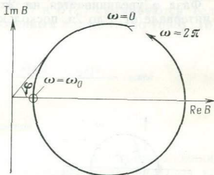
Рис. 2.5. Поведение фазы двухчленного фильтра, представленного на рис. 2.4, в комплексной области
