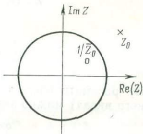
РИС. 2.17. Пример характеристики широкополосного фильтра, полюс (X) которого лежит вне единичного круга, а нуль (O) — внутри него. Полюс и нуль лежат на одном радиусе
