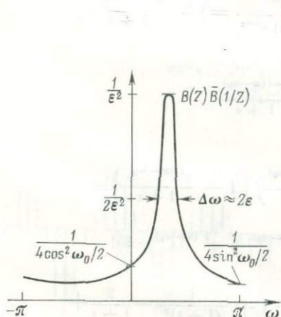
РИС. 2.15. Спектр, соответствующий функции с простым полюсом в точке Z_0^* = (1 + \varepsilon) e^{i\omega_0}
