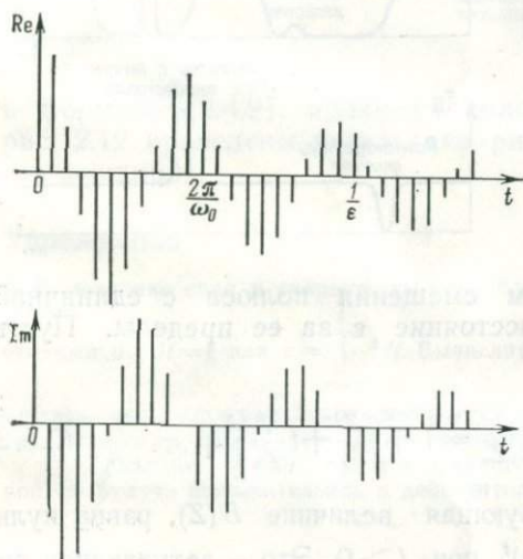
РИС. 2.14. Коэффициенты временной функции, имеющей простой полюс, лежащий вблизи единичной окружности за ее пределами в точке
