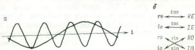
РИС. 1.7. Пример недостаточно частого квантования синусоиды по времени (а) и мнемоническая таблица, иллюстрирующая влияние Фурье-преобразования на свойства четности (нечетности) и действительности (мнимости) функций (б)
