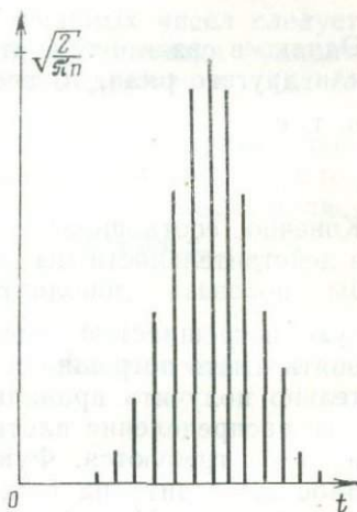
РИС. 4.1. Биномиальные коэффициенты, распределенные по закону гауссовой функции. Представлены коэффициенты при Z^t для функции (0,5+0,5Z)^{20}
