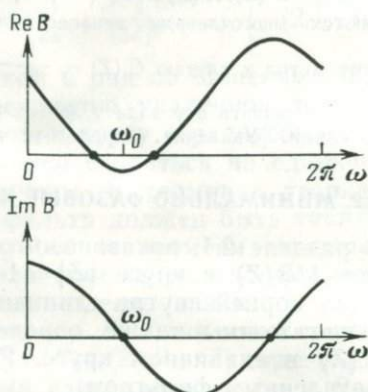
Рис. 2.7. Действительная и мнимая части частотной характеристики двухчленного неминимально фазового фильтра 1 - 1,25Ze^{-i2\pi/3}
