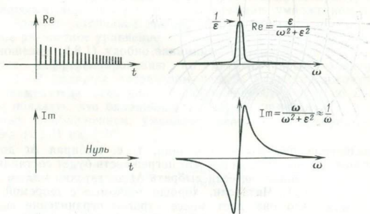
РИС. 2.23. Свойства оператора интегрирования
