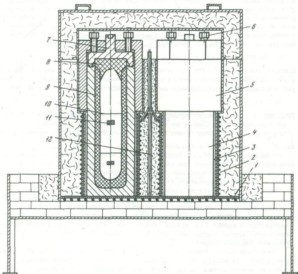
Рис. 4. Лабораторный автоклав
