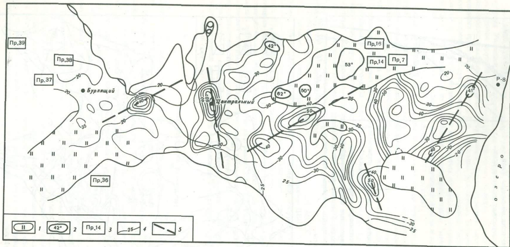
Рис. 10. Схема изотерм участка Центральной Узонской аномалии на глубине 5 см 1 - термальные болота; 2 - термальные озерки; 3 - места отбора проб воды; 4 - изотермы на глубине 5 см; 5 - предполагаемые термовыводящие трещины
