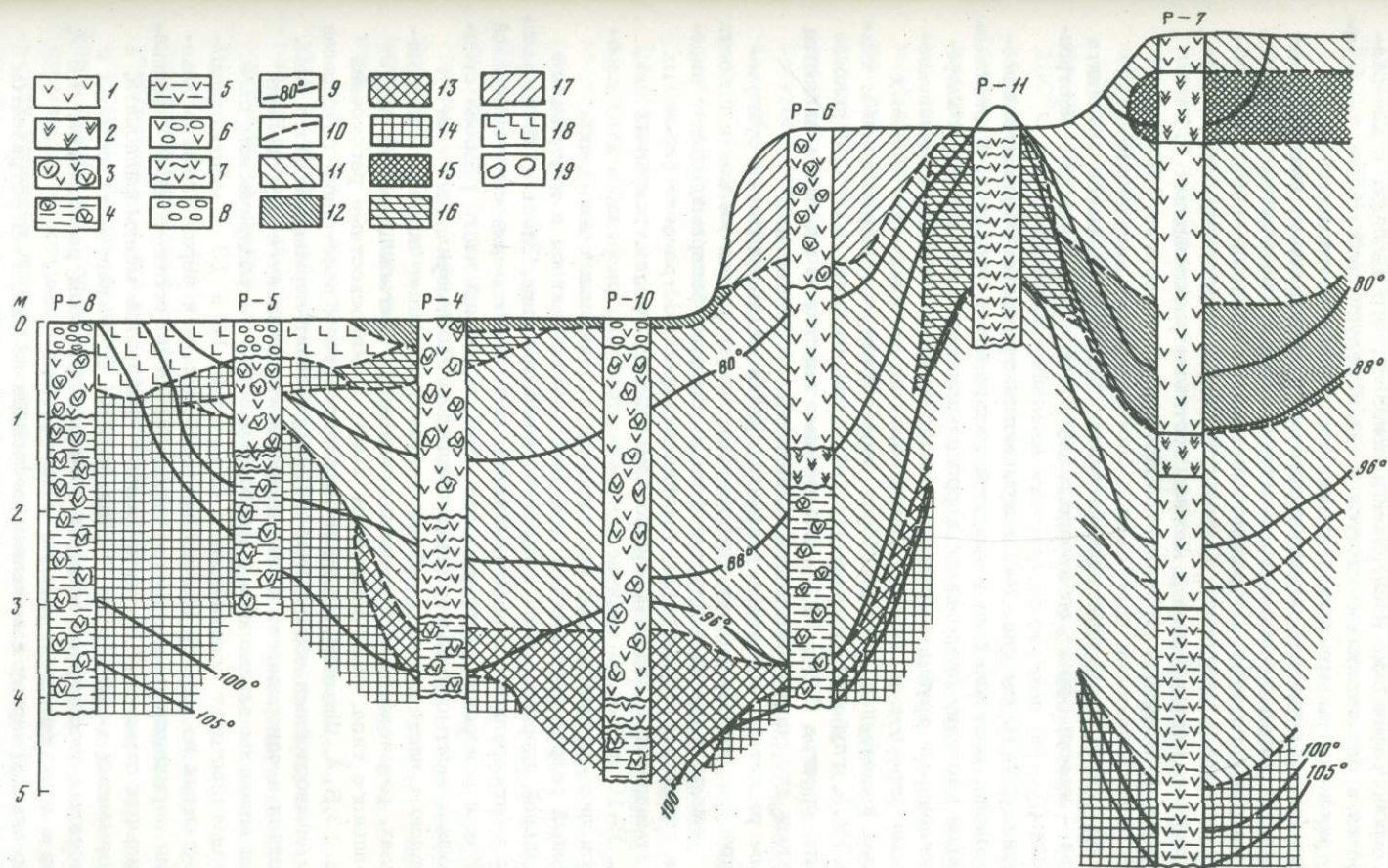
Рис. 12. Зональность гидротермально измененных пород Центральной Узонской термоаномалии (по В.А. Ерошеву-Шаку и др., 1974)
