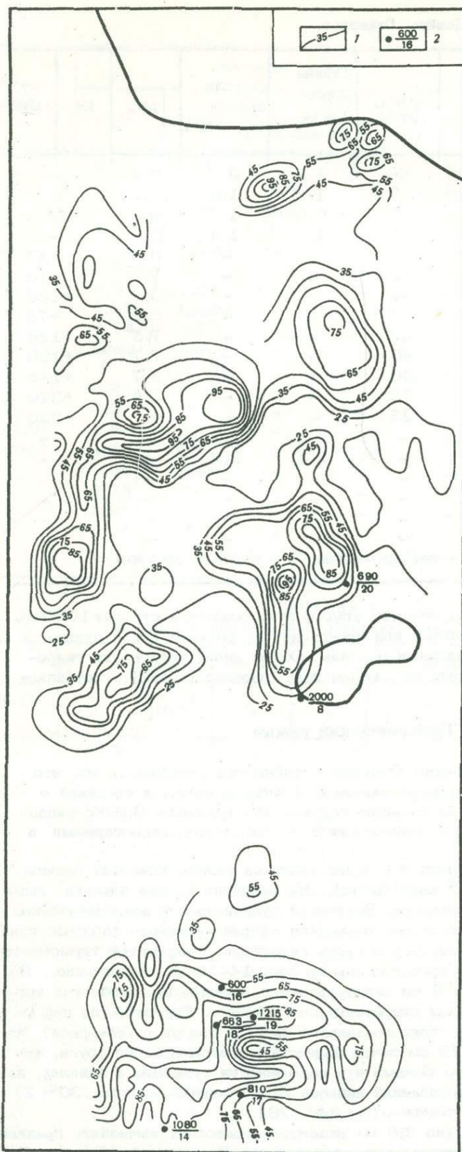
Рис. 15. Схема изотерм района Главных Гейзеров на глубине 50 см
