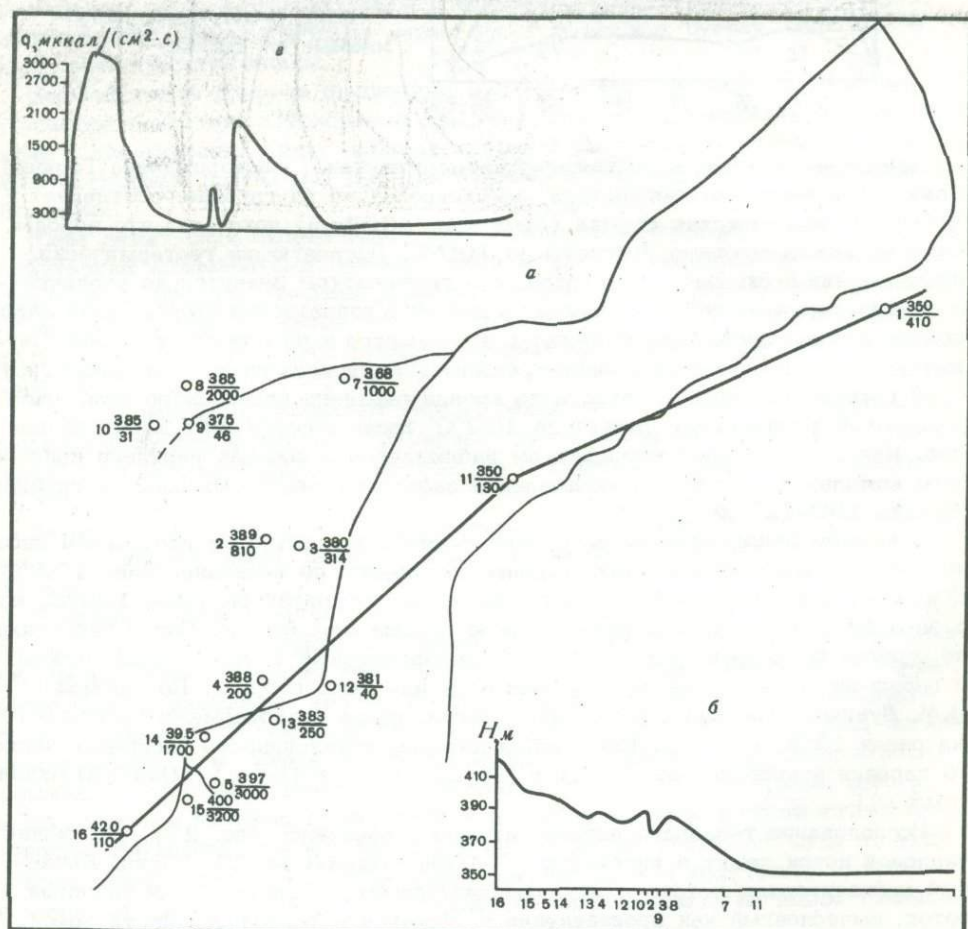
Рис. 22. Схема расположения точек (а) наблюдения за вариациями теплового потока [мккал/(см 2 ·с)] на Северо-Восточном сольфатарном поле вулкана Менделеева; гипсометрический (б) и геотермический (в) профили
