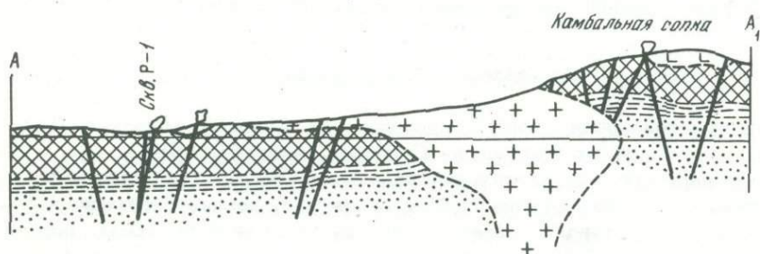
Рис. 24. Схематическая геологическая карта северо-западной части Камбарского хребта (по В.И. Белоусову, В.М. Сугророву, 1971)
