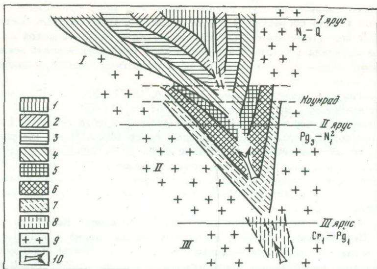
Рис. 28. Обобщенная схема зональности гидротермально измененных пород Срединного хребта Камчатки (по Г.М. Власову, М.М. Василевскому, 1964)
