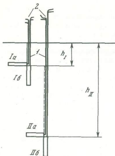
Рис. 2. Схема установки тепломеров 1 - тепломеры; 2 - выводы контактов тепломеров; Iа, Iб, IIа, IIб - варианты установки тепломеров; h_I и h_{II} - глубины установки датчиков (~30 и ~100 см соответственно); пунктиром изображена стенка шурфа
