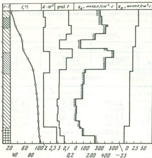
Рис. 26. Соотношение кондуктивной ( q_\lambda ) и "хемогенной" ( q_x ) составляющих теплового потока Центральной Узонской термоаномалии
