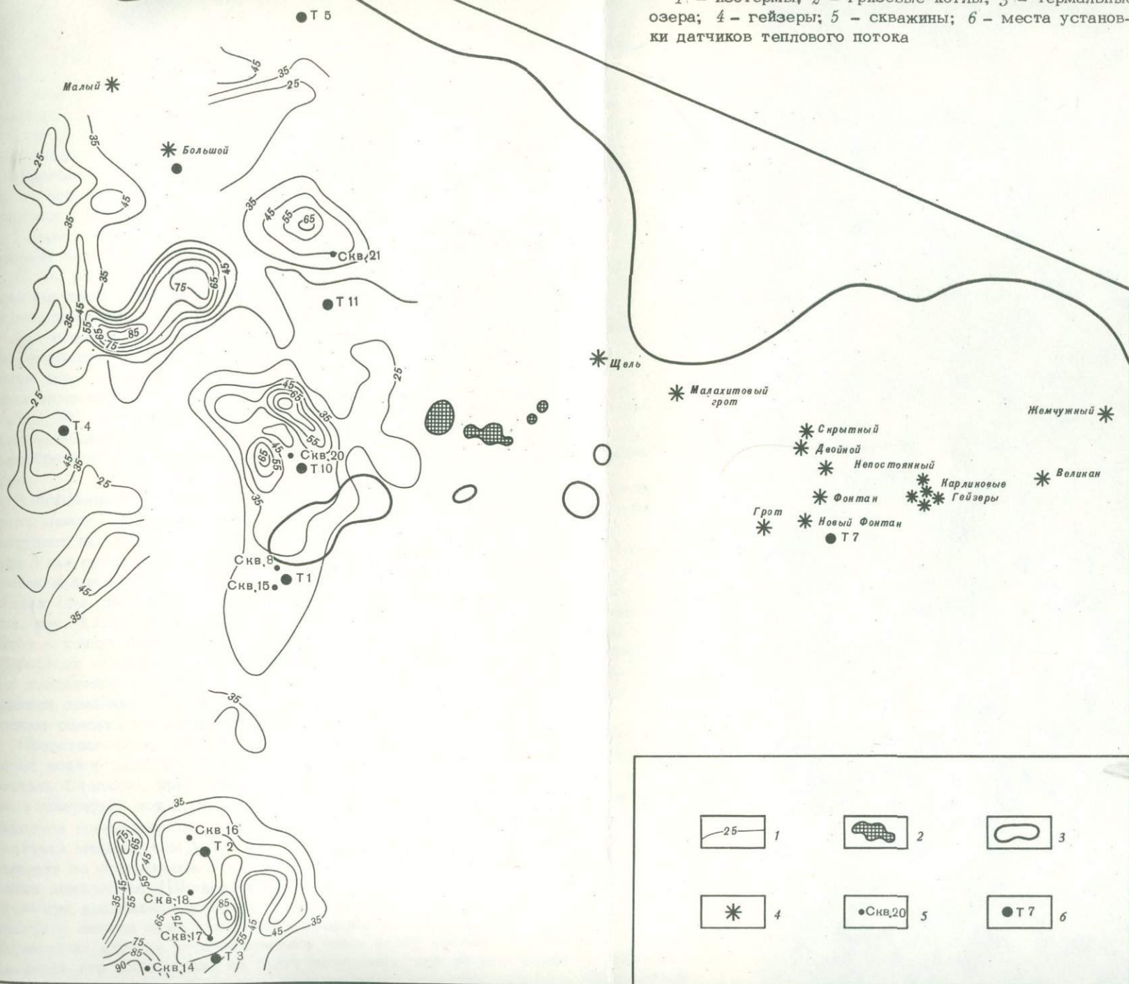
Рис. 14. Схема изотерм района Главных Гейзеров на глубине 5 см
