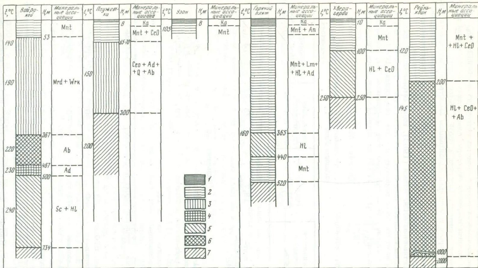
Рис. 27. Зональность гидротермально измененных пород современных геотермальных систем
