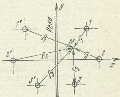
Рис. 17. Система взаимодействующих скважин у совершенной реки: 1, 2, 3 — скважины; 1', 2', 3' — зеркальные отображения скважин
