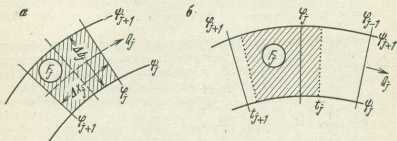
Рис. 50. Фрагмент гидродинамической сетки:
