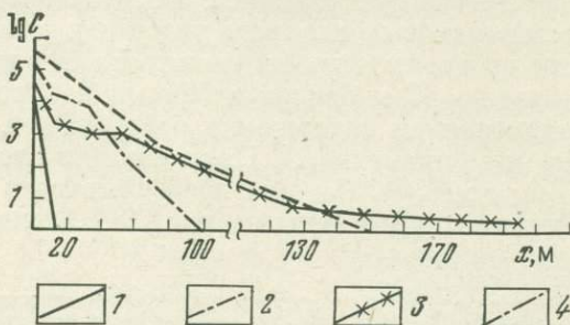
Рис. 14. Дальность распространения микроорганизмов в среднезернистых песках на участке искусственного пополнения подземных вод при скорости движения воды 2—3 м/сут: C — количество бактерий в подземных водах; x — расстояние от наблюдательных скважин до инфильтрационного бассейна; 1 — Esh. Coli ; 2 — бактерии группы кишечной палочки ( Citrobacter , Enterobacter ); 3 — энтерококк; 4 — бактерии семейства Pseudomonadaceae
