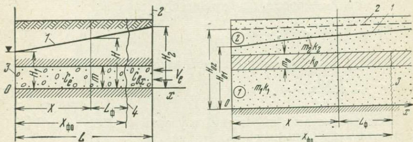
Рис. 44. Схема к расчету фронта загрязнений в одномерном потоке подземных вод (пласт, изолированный водоупорными кровлей и подошвой): 1 — пьезометрическая поверхность; 2 — контур питания; 3 — контур стока; 4 — начальное положение фронта фильтрации
