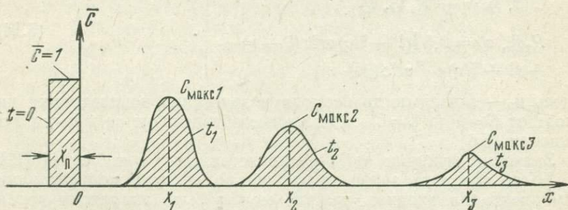
Рис. 33. Изменение концентрации вещества при «пакетном» запуске: x_n — длина пакета; x_1, x_2, x_3 — координаты точки с максимальной концентрацией в пакете в моменты времени t_1, t_2, t_3
