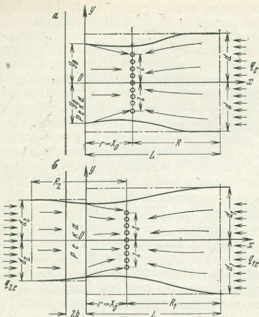
Рис. 61. Схемы фильтрации к линейному водозабору:
