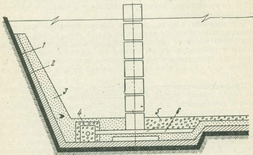
Рис. 51. Пластовый дренаж под полом здания для защиты подземных вод от инфилирующих технологических и сточных вод:
