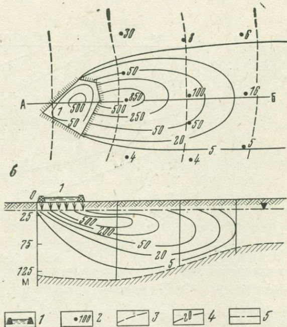
Рис. 37. Схема распространения загрязнения в подземных водах (по В. А. Грабовникову) а — план; б — разрез по линии А-Б: 1 — хвостохранилище; 2 — скважина и содержание микрокомпонента в мкг/л; 3 — гидроизогипсы; 4 — изолинии содержания микрокомпонента в мкг/л; 5 — уровень подземных вод
