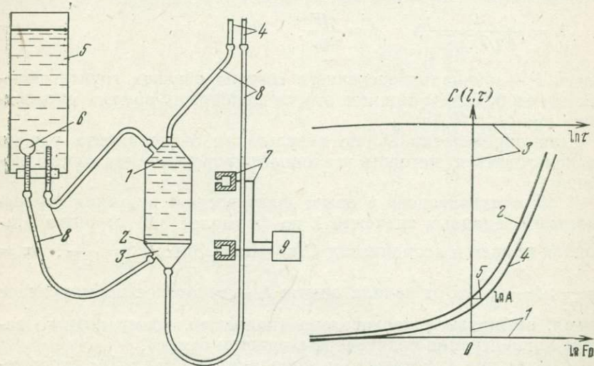
Рис. 62. Схема установки для изучения молекулярной диффузии:
