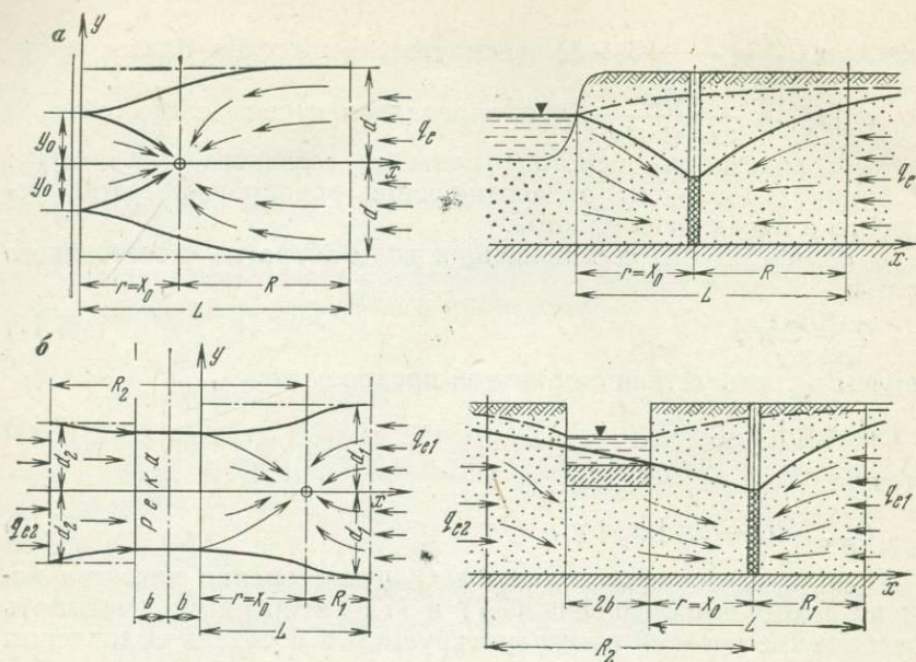
Рис. 59. Схемы фильтрации к береговому водозабору: а — вблизи гидравлически совершенной реки при большом расходе водозабора; б — вблизи гидравлически несовершенной реки
