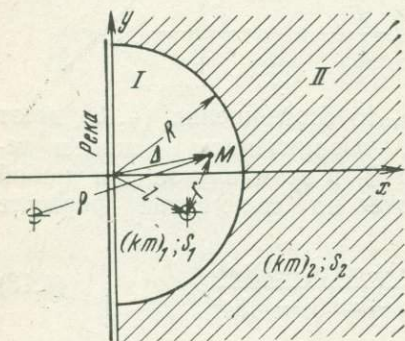
Рис. 21. Схема к расчету скважины в неоднородном пласте с круговой границей раздела зон: I, II — зоны с различной водопродвижимостью
