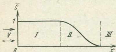
Рис. 32. Конвективная дисперсия в одномерном потоке:
