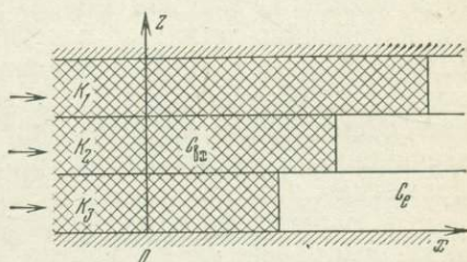
Рис. 6. Концентрационные языки загрязненных вод в слоистом пласте:
