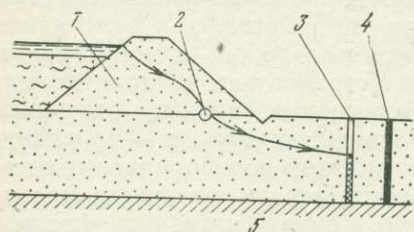
Рис. 54. Перехватывающий дренаж в нижнем бьефе шламохранилища:
