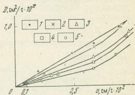
Рис. 5. Значение D в зависимости от скорости фильтрации при различных \eta'_0 = \eta_2/\eta_1 по [12]: \eta_0 : 1 — 1,00; 2 — 0,976; 3 — 0,954; 4 — 0,927; 5 — 0,903
