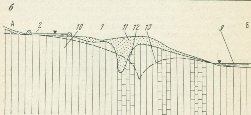
Рис. 75. Загрязнение поверхностных и подземных вод фтором в районе химического завода: a — план; б — разрез.
