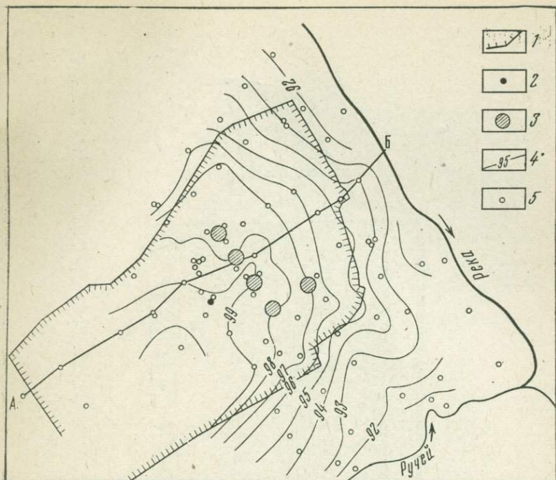
Рис. 71. Схематическая карта гидроизогипс в районе сажевого завода:
