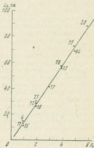
Рис. 10. График L_{я}(n_1) при b=l=4 см. В опытах 4, 15—20: d_1=4 см; n_2=0 ; в опытах 11—14: d'_1=d_2=4 см; n_2=3 ; в опыте 21: d_1=52 см; n_2=0 . Цифры при точках на графике — номера опытов
