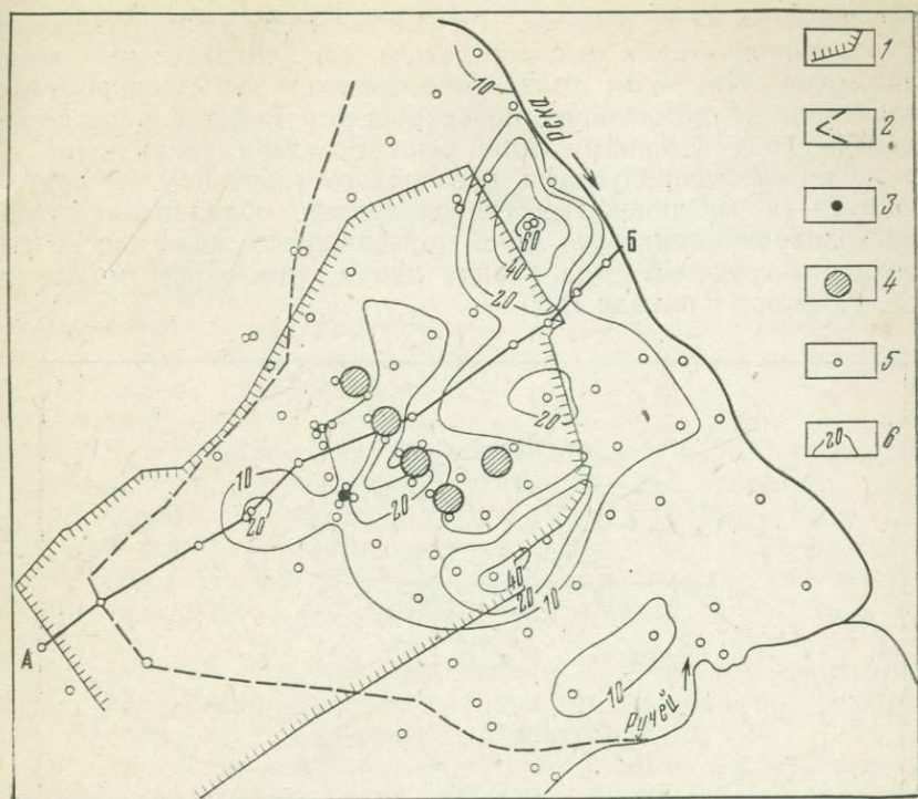
Рис. 73. Содержание нефтепродуктов в грунтах (г/кг массы сухого грунта): 1 — контур территории; 2 — контур загрязнения подземных вод и грунтов нефтепродуктами; 3 — подземная емкость для хранения сырья; 4 — баки — нефтехранилища; 5 — разведочные скважины; 6 — изолинии содержания нефтепродуктов в грунтах
