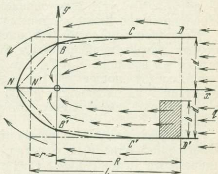
Рис. 56. Схема области захвата водозабора
