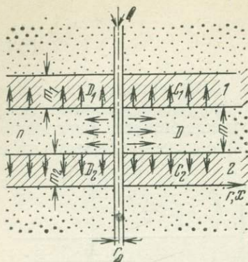
Рис. 39. Схема к расчету миграции загрязненных стоков в слоистую толщу: 1, 2 — номера слабопроницаемых слоев
