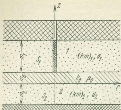
Рис. 28. Схема трехслойного пласта: 1, 2 — номера слоев
