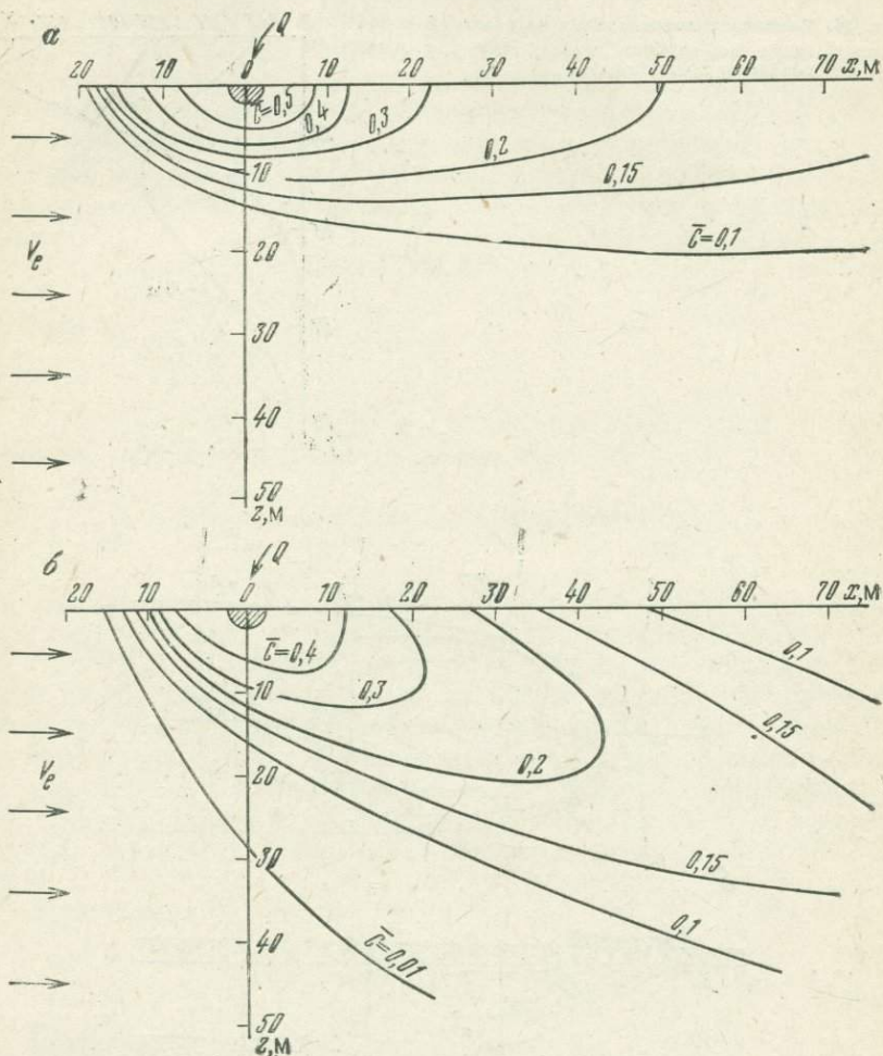
Рис. 35. Ареал распространения загрязнений в подземных водах в районе хранилища при \frac{Q}{2l} = 5 м 2 /сут, KI_e = 0.05 м/сут, D_x^* = D_y^* = 0.1 м 2 /сут.
