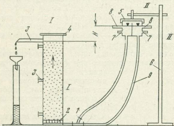
Рис. 64. Схема лабораторной установки для изучения фильтрационной дисперсии:
