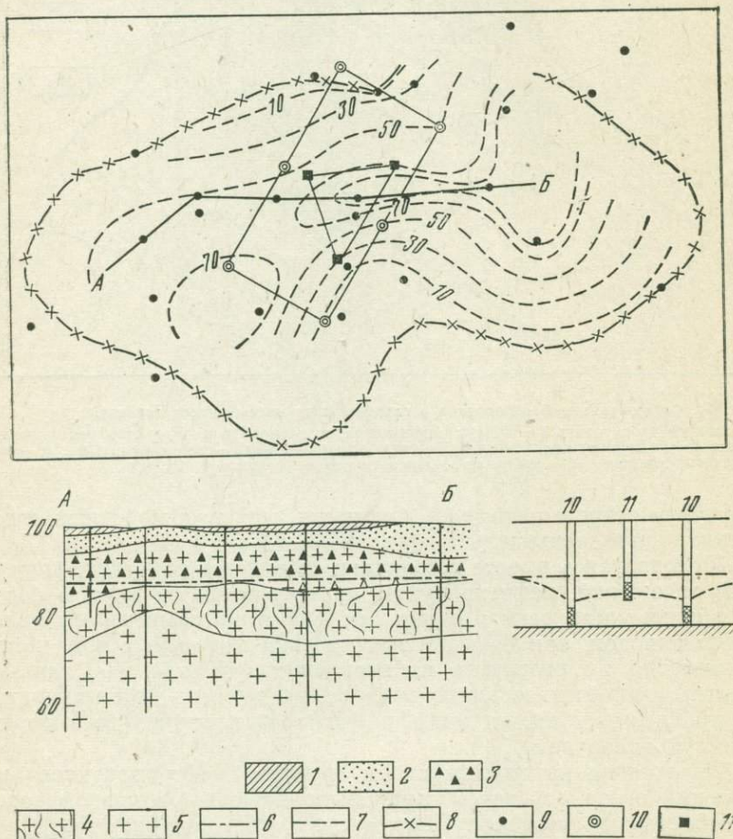
Рис. 74. Загрязнение трещинно-пластовых вод нефтепродуктами: 1 — супеси; 2 — песок; 3 — гранодиорит, выветренный до состояния рыхляка; 4 — гранодиорит с интенсивной трещиноватостью; 5 — гранодиорит монолитный; 6 — уровень грунтовых вод; 7 — изолинии мощности слоя нефтепродуктов; 8 — контур площади распространения нефтепродуктов; 9 — разведочные и наблюдательные скважины; 10 — скважины для откачки воды; 11 — скважины для откачки нефтепродуктов
