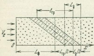
Рис. 43. Схема к определению размеров зоны загрязненных подземных вод под влиянием дисперсии и различия в плотностях
