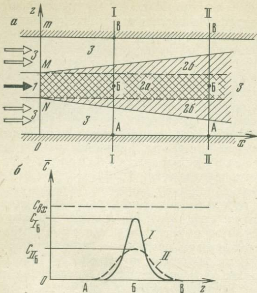
Рис. 3. Поперечная и продольная микродисперсия:
