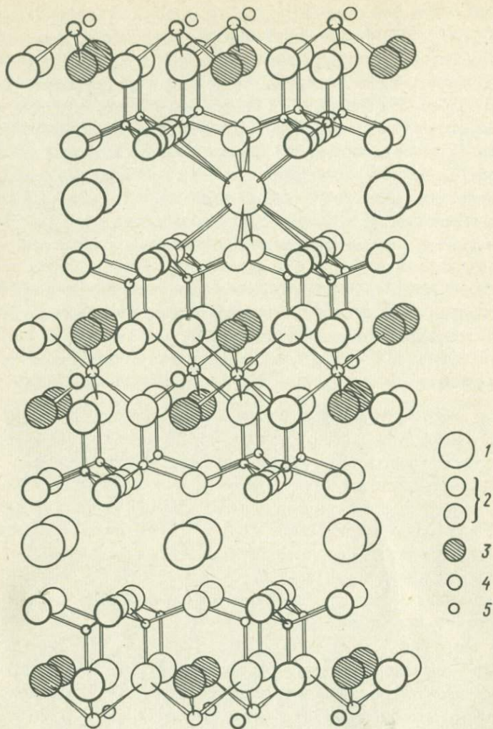
Ф и г. 21. Кристаллическая структура мусковита.
