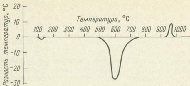
Фиг. 61. Дифференциальная кривая нагревания каолинита.
