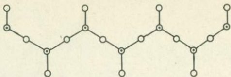
Ф и г. 15. Пироксеновая цепочка.
