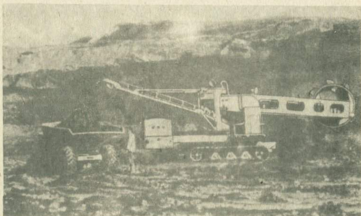
Ф и г. 32. Ковшовый роторный экскаватор на открытых разработках глин.
