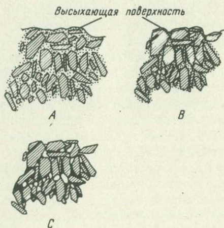
Фиг. 59. Поведение глинистых частиц при сушке.
