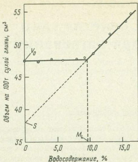
Фиг. 60. Кривая высыхания глинисто-керамической массы.
