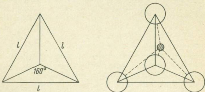
Ф и г. 8. Кремнекислородный тетраэдр.
