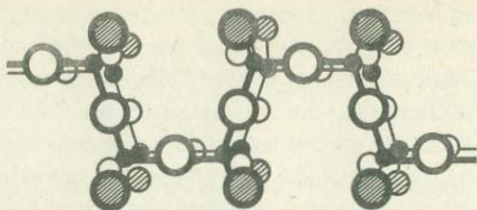
Ф и г. 22. Кристаллическая структура полевого шпата. (A.F. Wells, Structural Inorganic Chemistry.)
