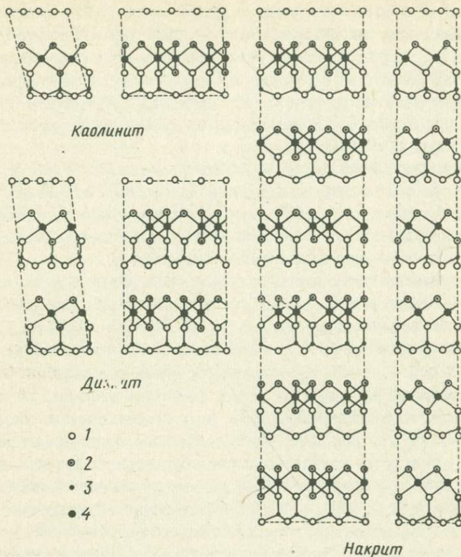
Ф и Г. 19. Сопоставление кристаллических структур каолинита, накрита и диккита. Обозначения ионов: 1 — кислород; 2 — гидроксип; 3 — кремний; 4 — алюминий.
