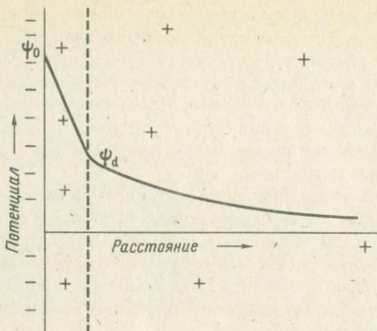
Ф и г. 37. Схема распределения ионов на заряженной частице.
