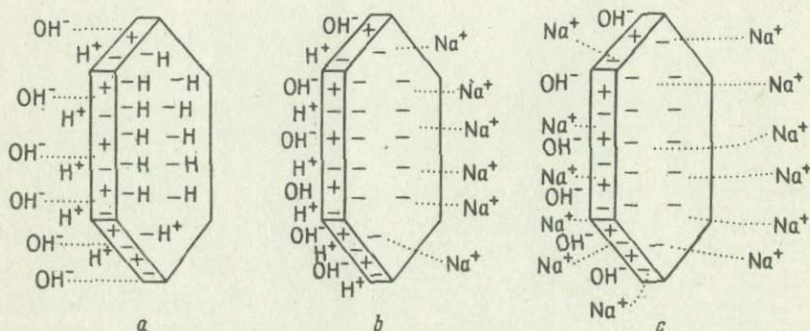
Ф и Г. 42. Распределение обменных ионов и зарядов на ребрах и плоских гранях глинистых частиц.
