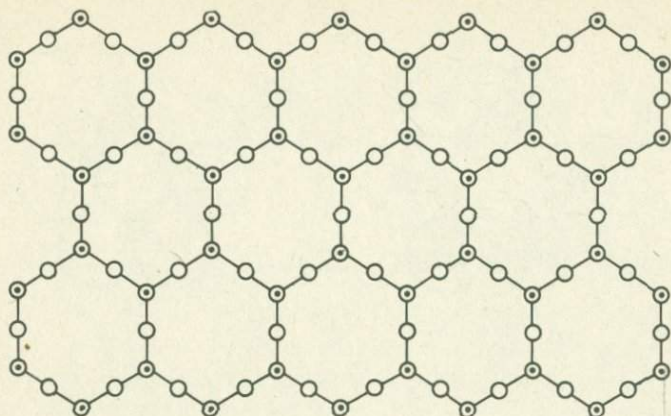
Ф и г. 17. Кремнекислородный лист
