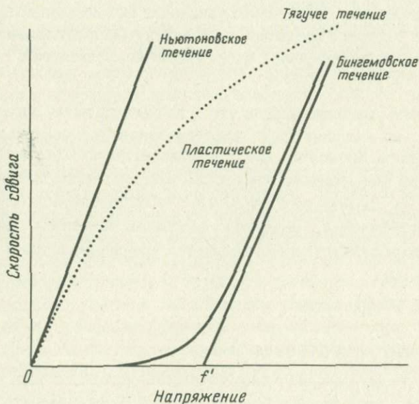
Ф и г. 47. Кривые течения различных типов.
