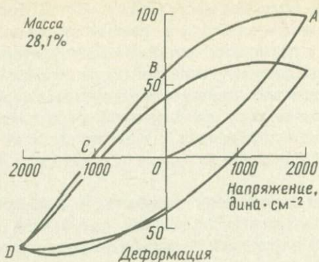
Фиг. 55. Циклическая кривая напряжение — деформация.
