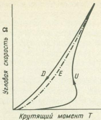
Ф и г. 48. Петля тиксотропии.
