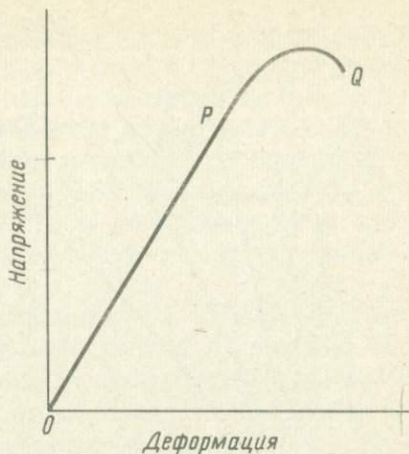
Фиг. 52. Кривая напряжение — деформация пластичной глины.
