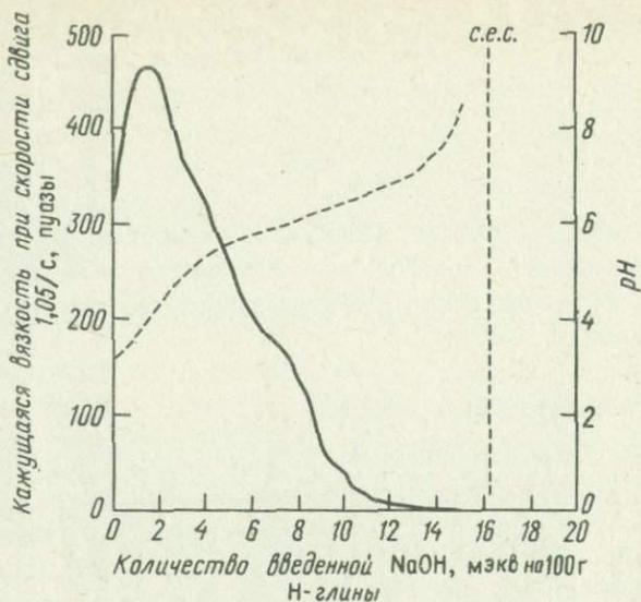
Ф и Г. 41. Изменения рН и вязкости водородных комовых глин при титровании их суспензий NaOH.
