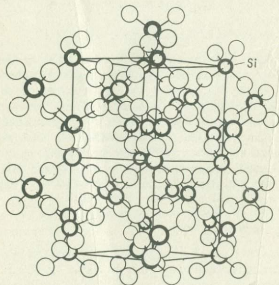
Фиг. 66. Кристаллическая структура обычной шпинели.
