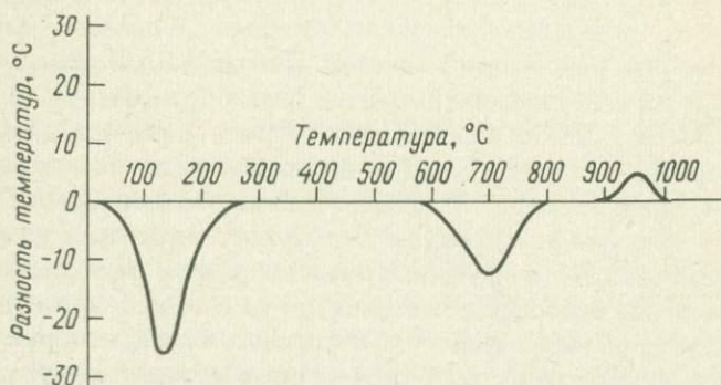
Фиг. 62. Дифференциальная кривая нагревания монтмориллонита
