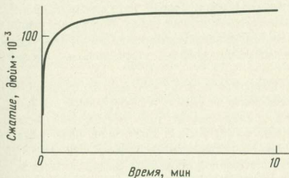
Фиг. 54. Кривая деформация — время пластичной глины.
