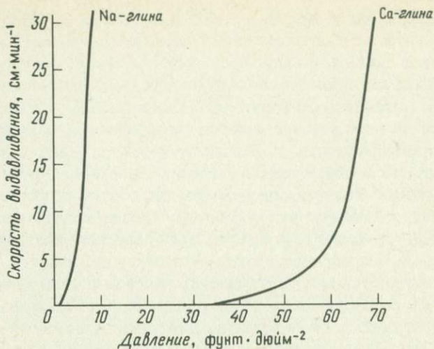
Фиг. 57. Влияние обменных ионов на кривую течения.
