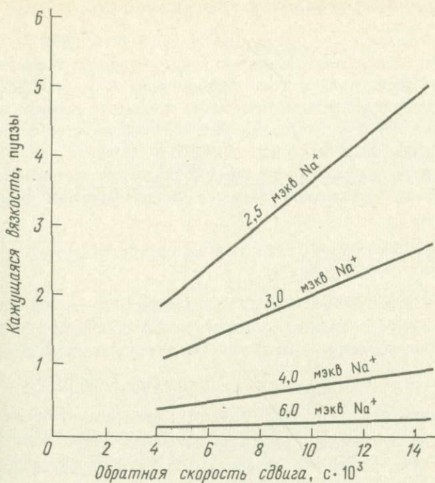
Ф и г. 49. Диспергация и бингемовские константы.
