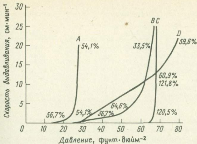
Фиг. 51. Кривые течения различных глин. А — комовая глина; В — огнеупорная глина; С — бентонит; D — китайский камень.
