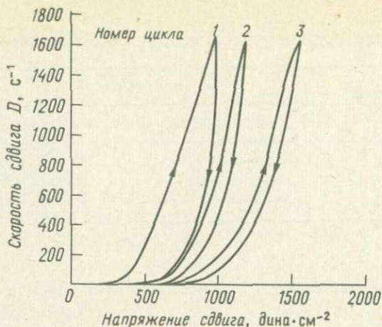
Ф и г. 50. Эффект старения.
