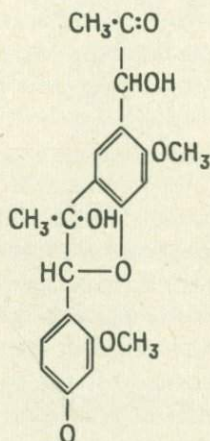
Ф и г. 24. Структура лигнина.
