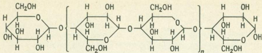
Ф и г. 23. Структура целлюлозы.
