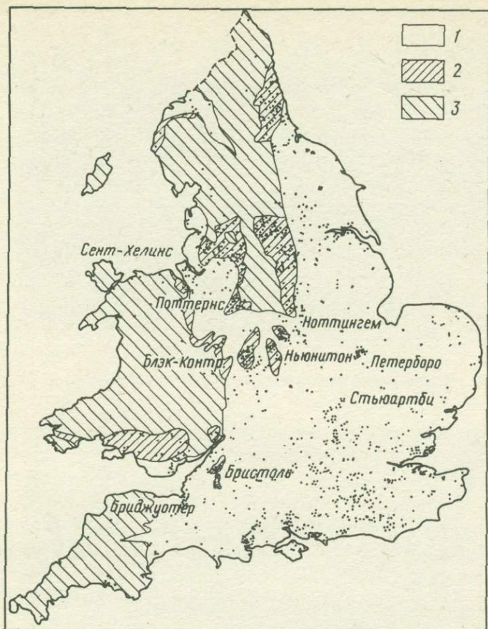
Ф и Г. 27. Схема геологического строения Англии и Уэльса.
