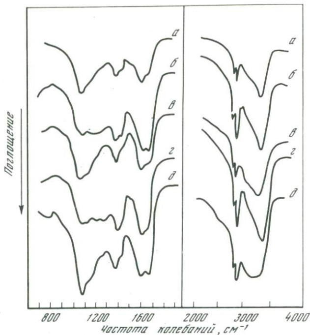
Р и с. 22. ИК-спектры препарата 2, выделенного из белемнитов [154]
