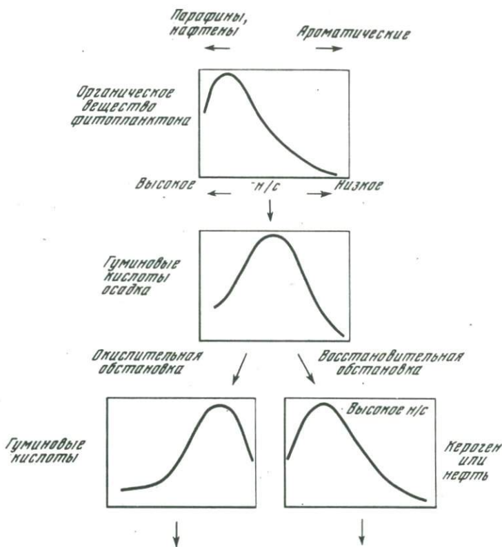
Р и с. 33. Изменение органического вещества в процессе диагенеза [413]
