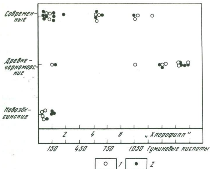
Р и с. 5. Содержание хлорофилла и гуминовых кислот в осадках Черного моря (в миллиграммах на 100 г сухого осадка) 1 – хлорофилл, 2 – гуминовые кислоты
