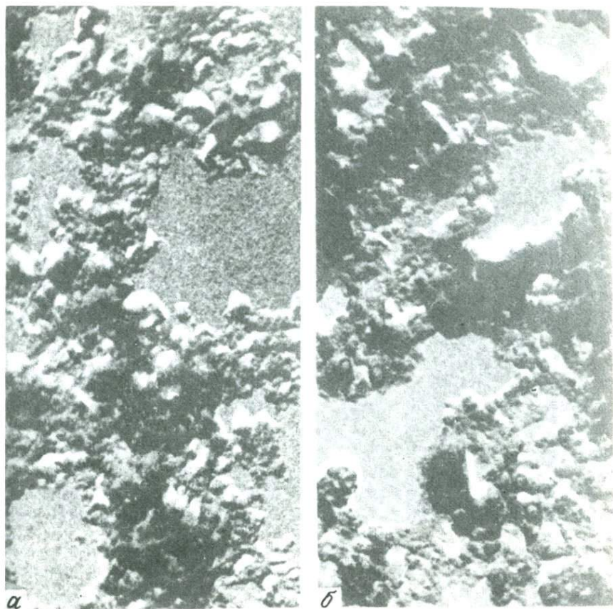
Р и с. 23. а. Конхиолин перламутрового слоя наutilusа после нагревания раковины при 600^{\circ}\text{C} на воздухе без воды. Появляются сферидальные корпускулы. Увелич. 42 000. б. Наутилоид аммоноид, меловой период. Фрагменты остатка органического вещества перламутрового слоя после декальцирования. Есть сферидальные корпускулы. Увел. 42 000 [368]
