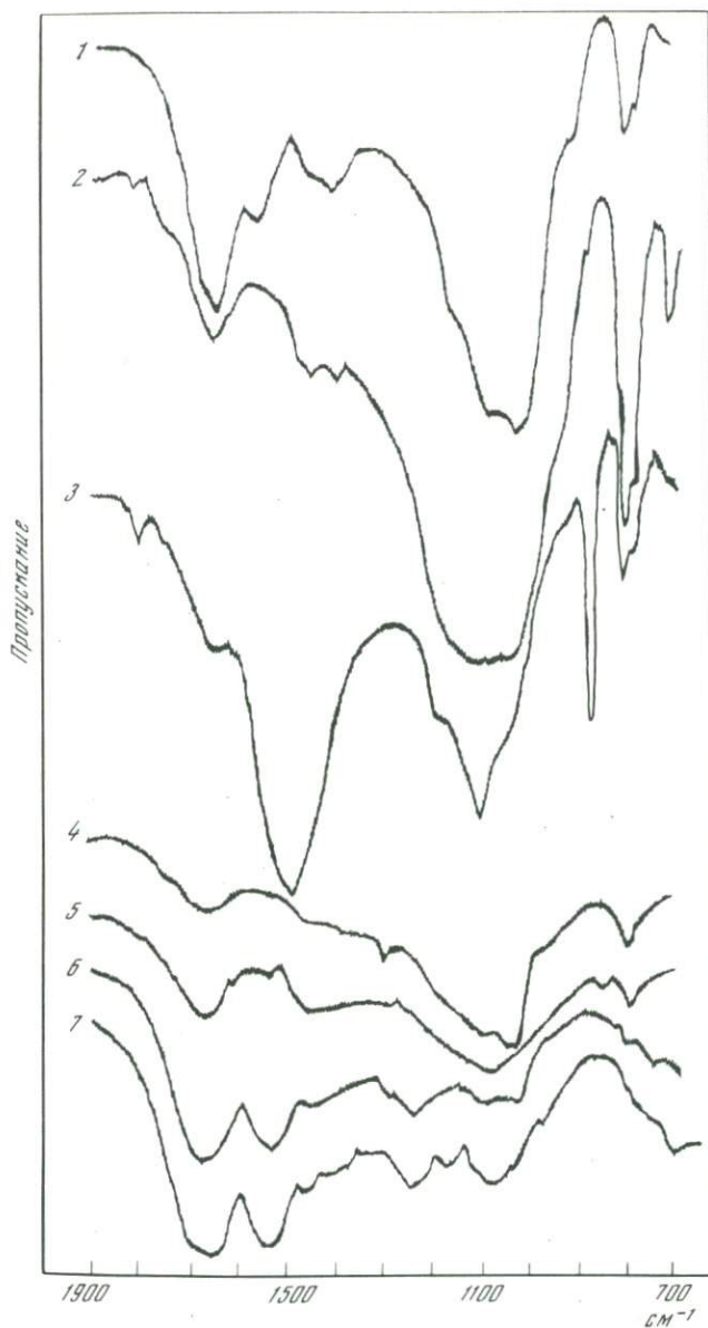
Р и с. 25. ИК-спектры органического вещества раковин двустворок
