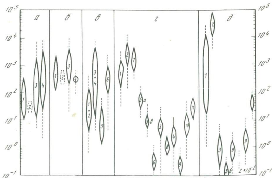
Р и с. 1. Средние данные по распределению углеводов, О–N–S соединений, пигментов, аминокислот и углеводов в различных геологических материалах [ 81 ]
