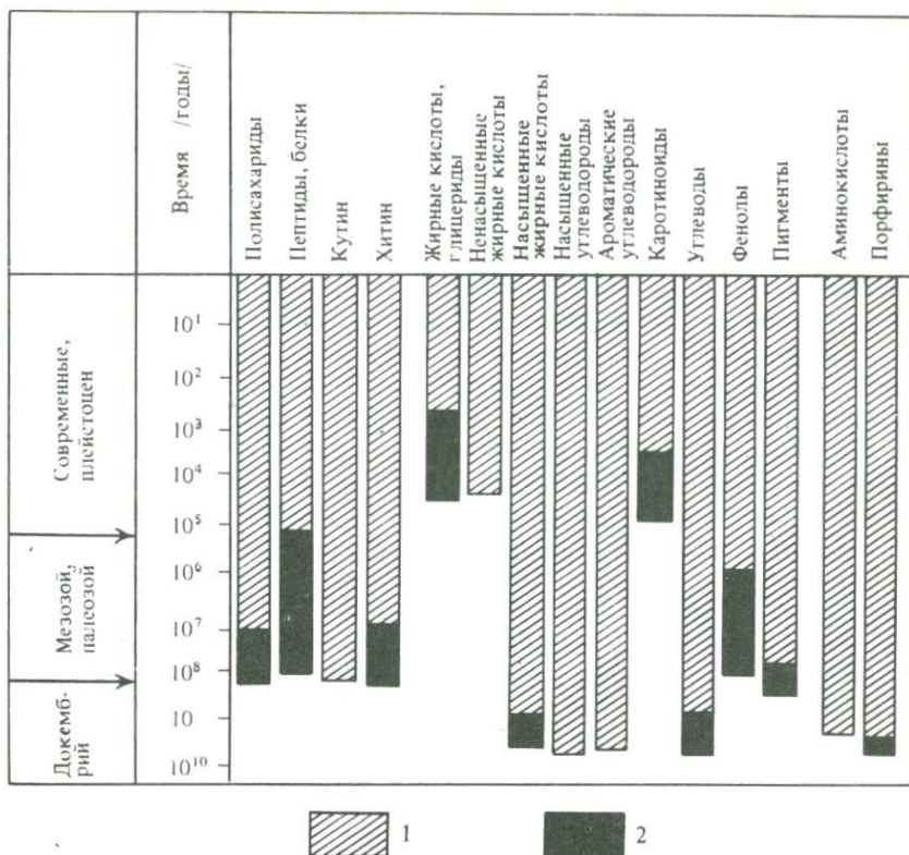
Р и с. 2. Биохимически важные органические соединения в осадочных отложениях разного геологического возраста [ 331 ]
