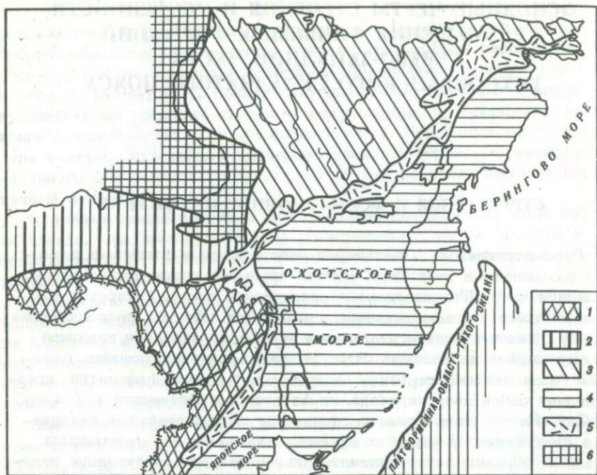
Рис. 15. Схема расположения мегаблоков в северо-западной части Тихоокеанского складчатого пояса, по Л.И. Красному (Геологическое строение..., 1966).
