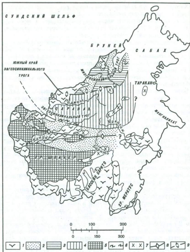
Рис. 21. Схематическое строение геосинклинали Северного Борнео, по Н. Хайлю (Haile, 1969) с упрощениями
