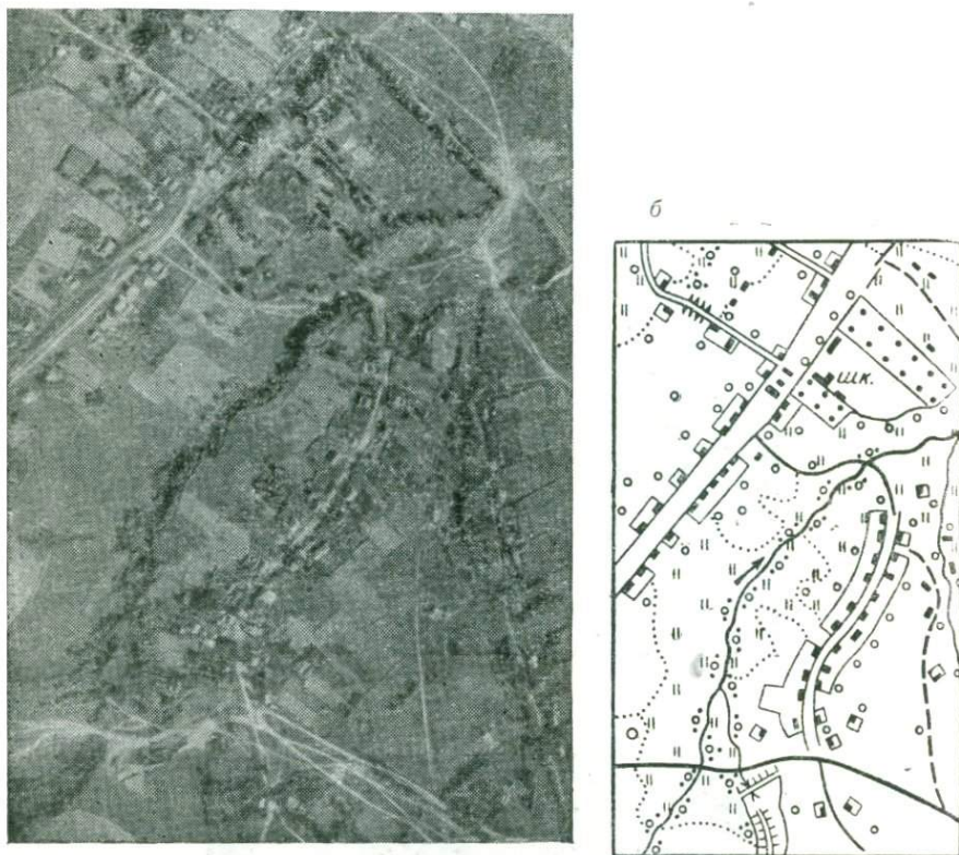
Рис. 25. Пример генерализации аэроснимка для топографической карты масштаба 1 : 25 000:
