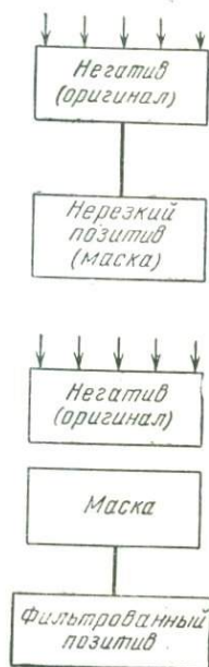
Рис. 33. Схема фотографической фильтрации
