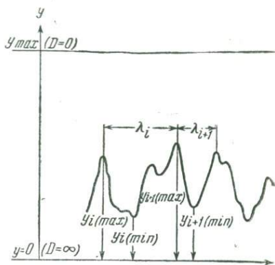
Рис. 28. Элементы регистрограммы
