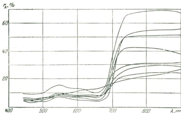
Рис. 12. Кривые СКЯ объектов 3-ей группы
