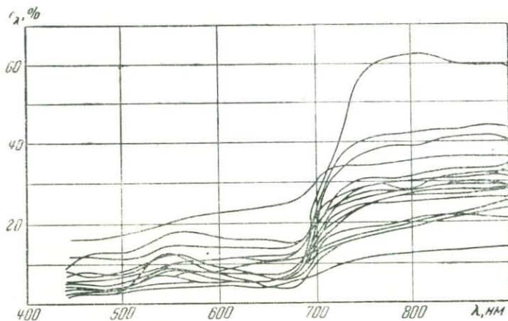
Рис. 11. Кривые СКЯ объектов 2-ой группы
