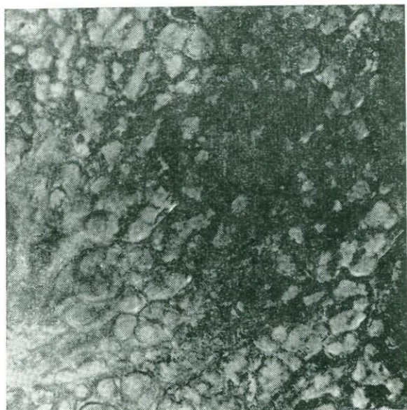
Рис. 4. Каравеобразная структура изображения бугристой тундры
