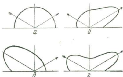
Рис. 7. Основные типы индикатриссы отражения:
