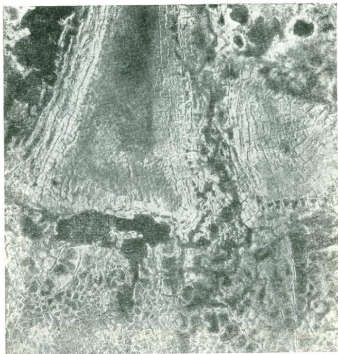
Рис. 3. Сетчатая структура изображения полигональной тундры
