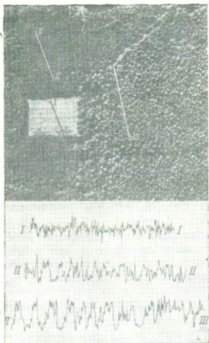
Рис. 29. Аэроснимок и регистрограммы, полученные с него по избранным профилям:
