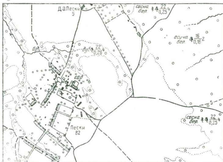
Рис. 21. Образец топографического дешифрирования обжитого лесостепного ландшафта
