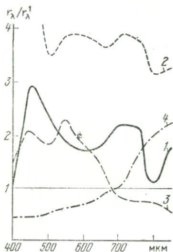
Рис. 5. Кривые отношений спектральных коэффициентов яркостей некоторых сочетаний растительности:
