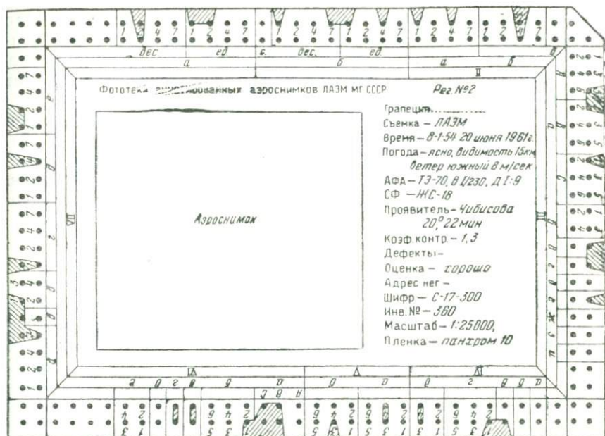
Рис. 17. Образец эталона дешифрирования на перфокарте
