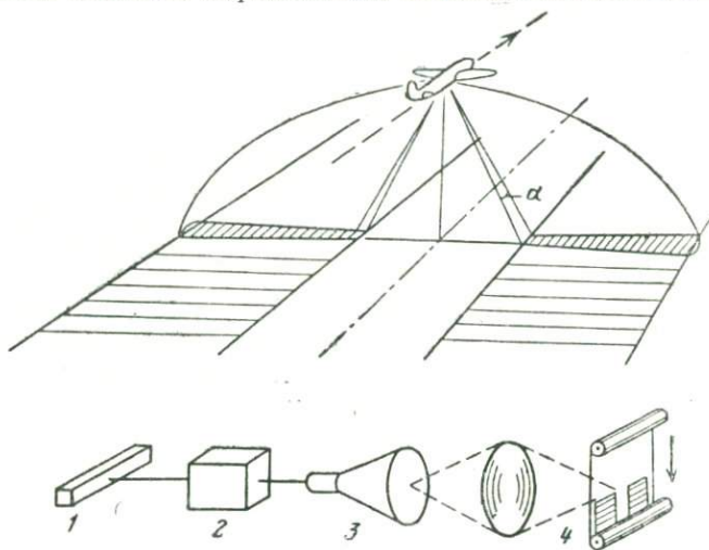
Рис. 36. Принцип действия радиолокационной станции бокового обзора:
