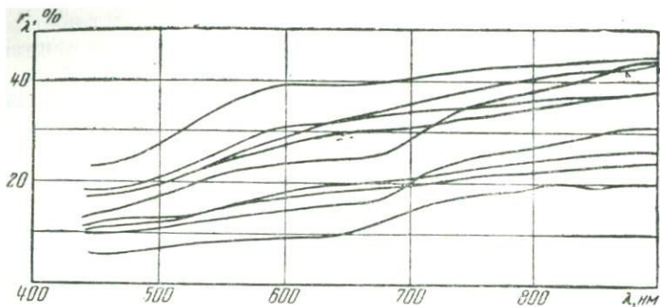
Рис. 10. Кривые СКЯ объектов 1-ой группы
