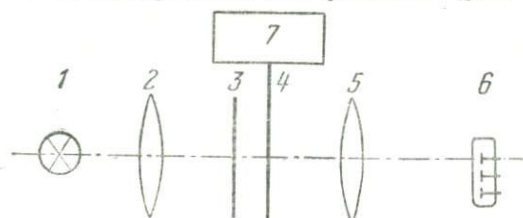
Рис. 35. Схема оптического коррелятора
