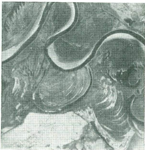
Рис. 16. Индикационное значение реки для почвы и растительности
