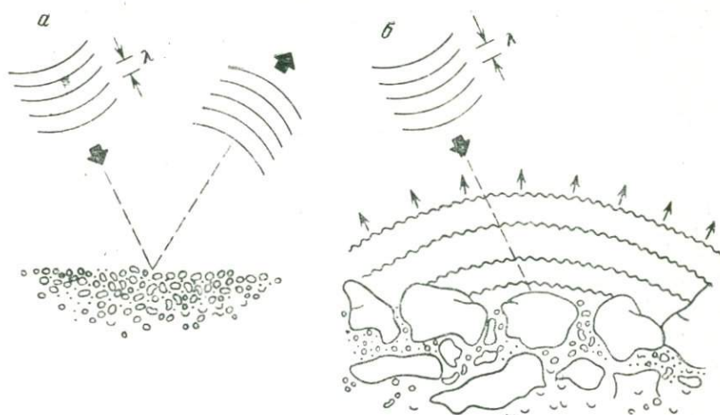
Рис. 37. Отражение радиолокационных сигналов различными поверхностями
