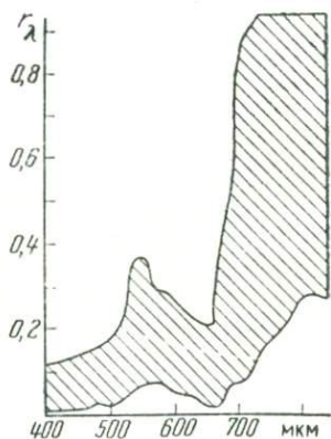
Рис. 6. Площадь распространения кривых СКЯ травянистой растительности, полученных в разных условиях
