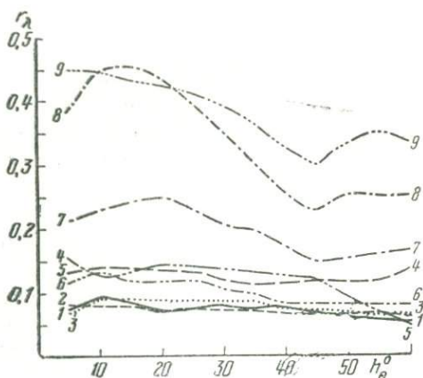
Рис. 9. Изменение СКЯ разнотравно-злакового луга в зависимости от высоты стояния Солнца. Значения:
