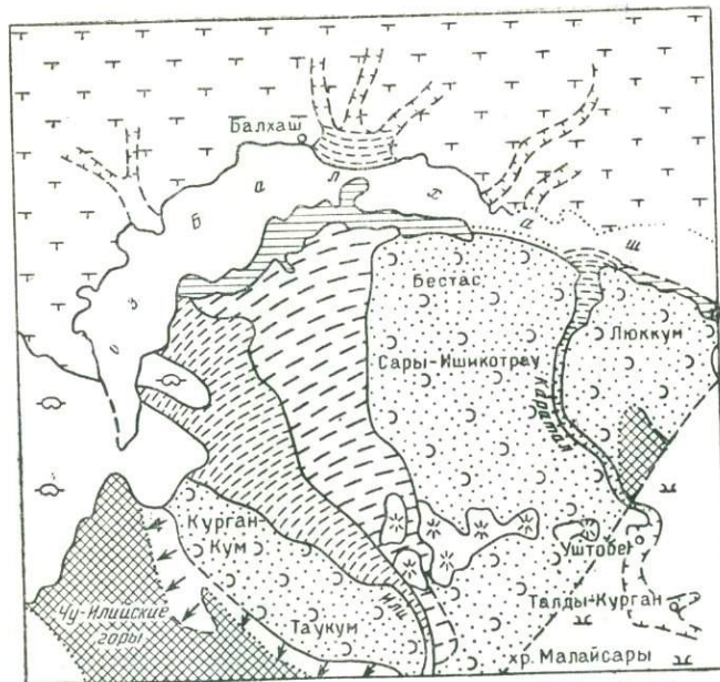
Рис. 40. Геоморфологическая интерпретация телевизионного изображения Прибалхашья:
