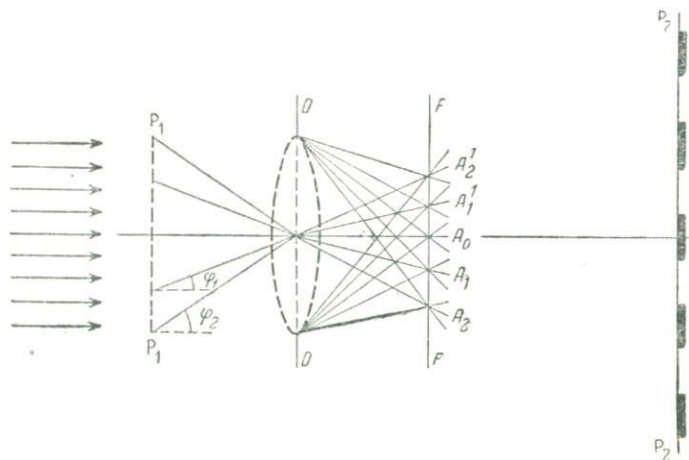
Рис. 32. К дифракционной теории фильтрации
