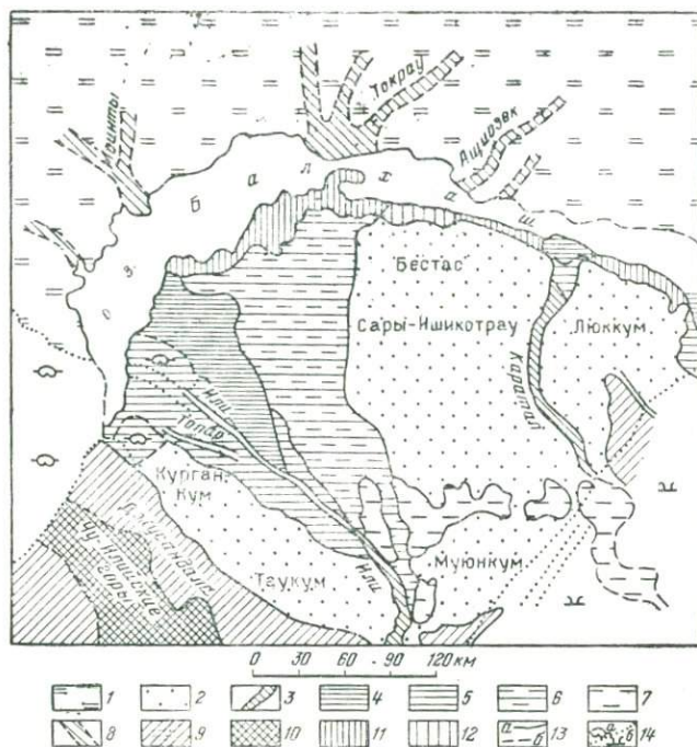
Рис. 41. Почвенно-геоботаническая интерпретация теле- визионного изображения Прибалхашья:
