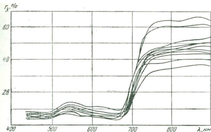
Рис. 13. Кривые СКЯ объектов 4-ой группы
