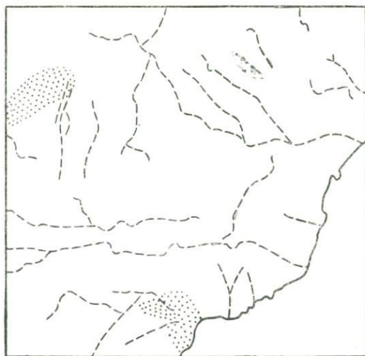
Рис. 38. Сравнение космической фотографии ( a ) с фрагментом Международной карты мира масштаба 1 : 2 500 000 ( б )
