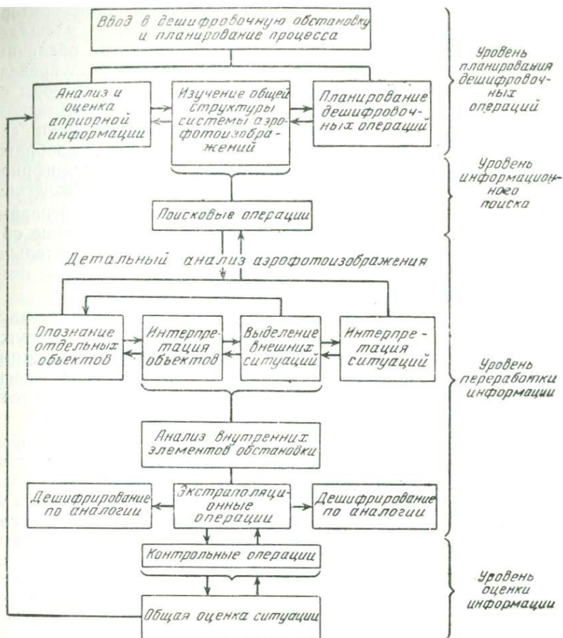
Рис. 1. Структурная схема дешифровочного процесса
