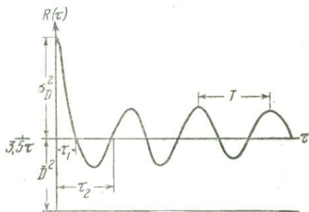
Рис. 30. АКФ изображения со сложной структурой
