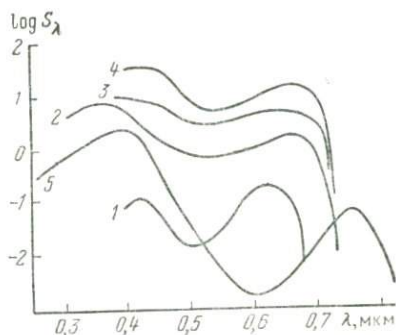
Рис. 14. Кривые спектральной чувствительности основных сортов аэропленок:
