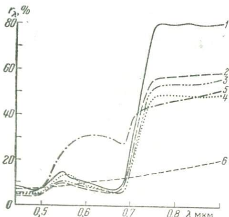
Рис. 8. Кривые СКЯ листьев осины в разных фазах вегетации:
