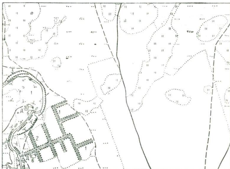
Рис. 22. Образец топографического дешифрирования степного ландшафта
