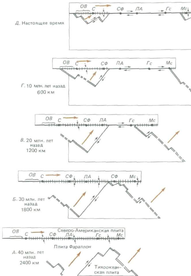
Рис. 6-4. Схематическая модель взаимодействия плит Северо-Американской, Тихоокеанской и Фараллон за последние 40 млн лет. Допускается, что Северо-Американская и Тихоокеанская плиты двигались с постоянной относительной скоростью 6 см/год параллельно разлому Сан-Андреас. Западный берег Северной Америки почти параллелен разлому Сан-Андреас. Слева показаны расстояния, на которые должна была перемещаться Северо-Американская плита в каждый интервал времени, чтобы достичь своего современного положения относительно Тихоокеанской плиты. ОВ — остров Ванкувер; С — Ситл; СФ — Сан-Франциско; ЛА — Лос-Анджелес; Гс — Гуаймас; Мс — Масатлан [21].
