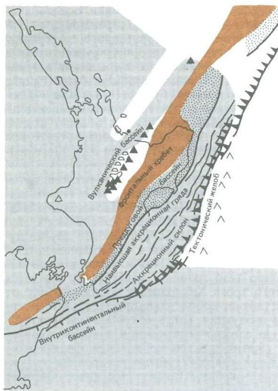
Рис. 12-15. Главные структурные элементы окраины Хикуранги острова Северный Новая Зеландии. Видно продолжение на сушу некоторых элементов системы Кермадек в северной части и окончание зоны косяк субдукции на трансформной границе – в южной части структурного комплекса [200, 648].
