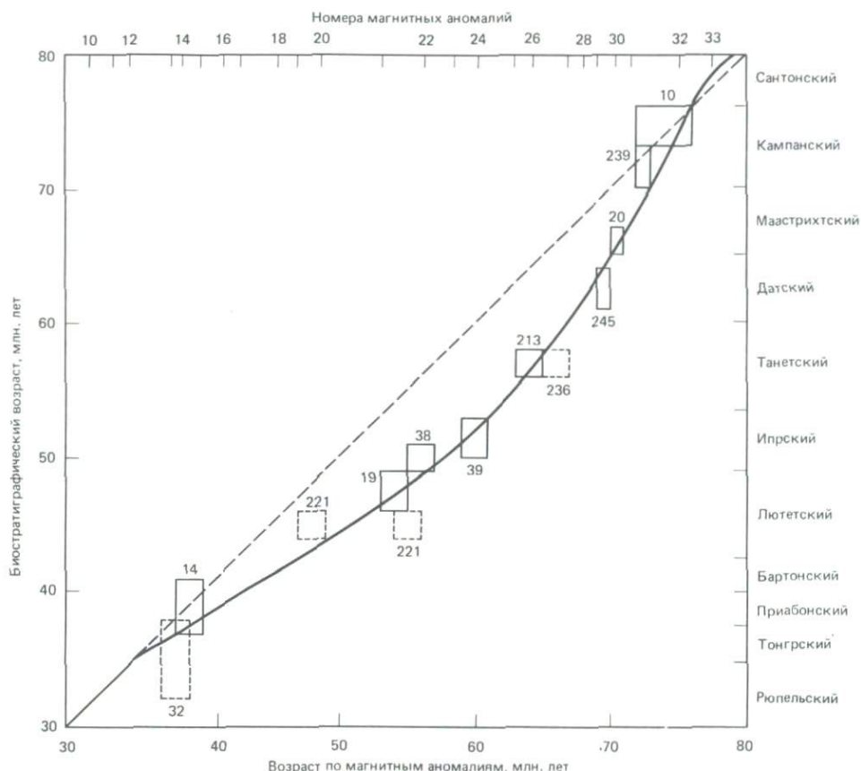
Рис. 4-10. Сравнение возрастов фундамента, определенных по магнитным аномалиям океанского дна, с возрастными по микрофоссилиям в осадках, залегающих непосредственно на базальтах фундамента (в скважинах DSDP, номера которых даны на рисунке) [917]. (Публикуется с разрешения Геологического общества Франции.)
