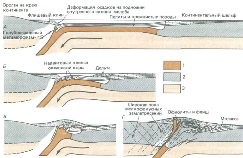
Рис. 12-23. Разрезы, иллюстрирующие последовательность событий при столкновении двух континентов [252, с. 2642]. Условные обозначения слоев литосферных плит см. на рис. 12-22.
