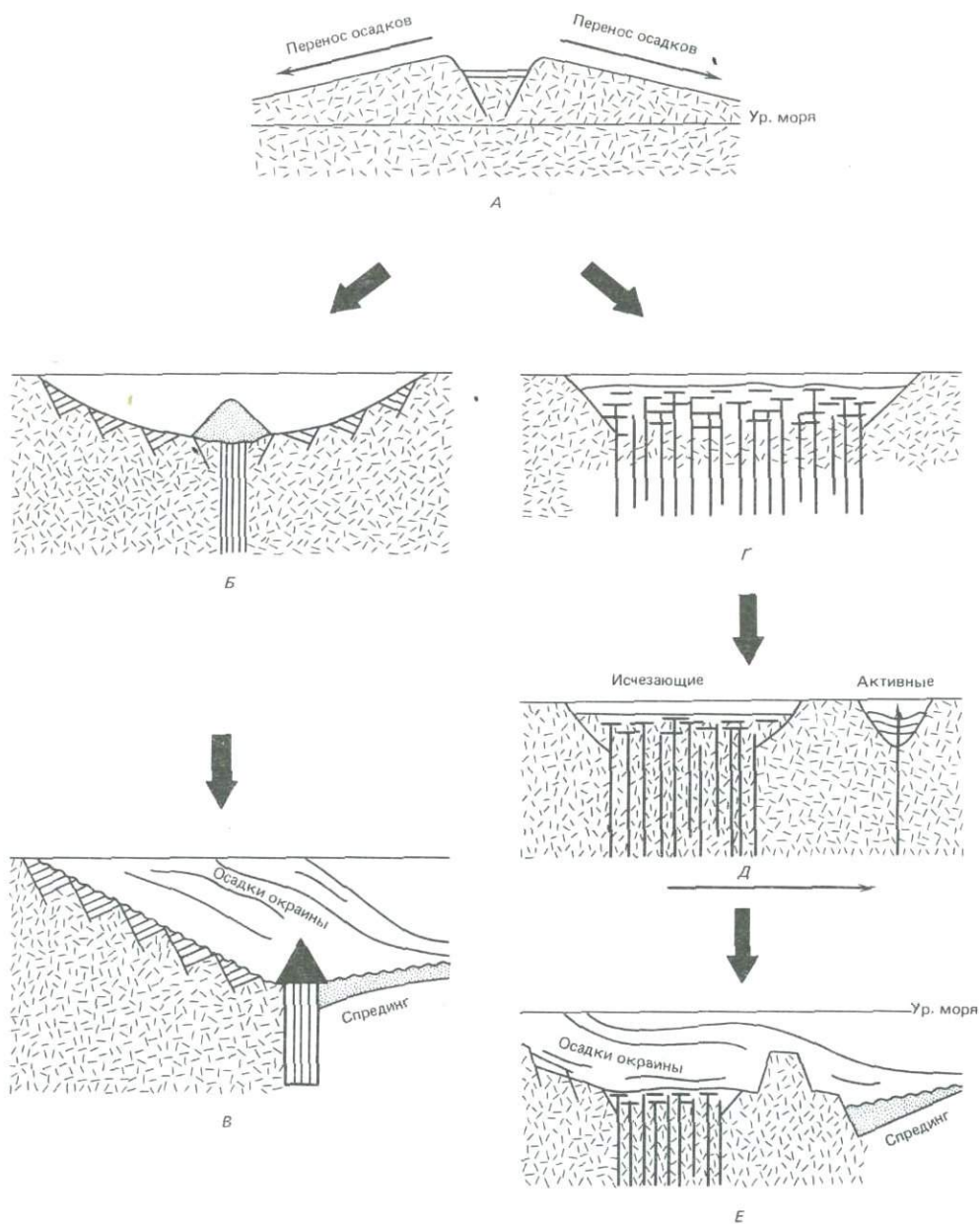
Рис. 11-5. Эволюция пассивных окраин. Слева (А–В): за вулканической активностью в относительно узкой зоне последовало сооружение хребта, а затем послерифтовое погружение и спрединг. Справа (Г–Е): после рассредоточенного внедрения первичных вулканических пород произошел перескок центра вулканизма, а затем начался спрединг. А – подъем кристаллического фундамента континента, рифтогенез, эрозия; Б – вулканизм в узкой зоне, возникновение вулканического хребта; В – погружение после раскола континента с мощной толщей осадков, под которой погребен вулканический хребет – возможный источник склоновой магнитной аномалии (?); Г – дайки и силлы в рифтовых отложениях; земная кора переходного, «рифтового», типа; зона спокойного магнитного поля; Д – перескок центра вулканизма; Е – краевое плато, внешний гребень с континентальной корой.
