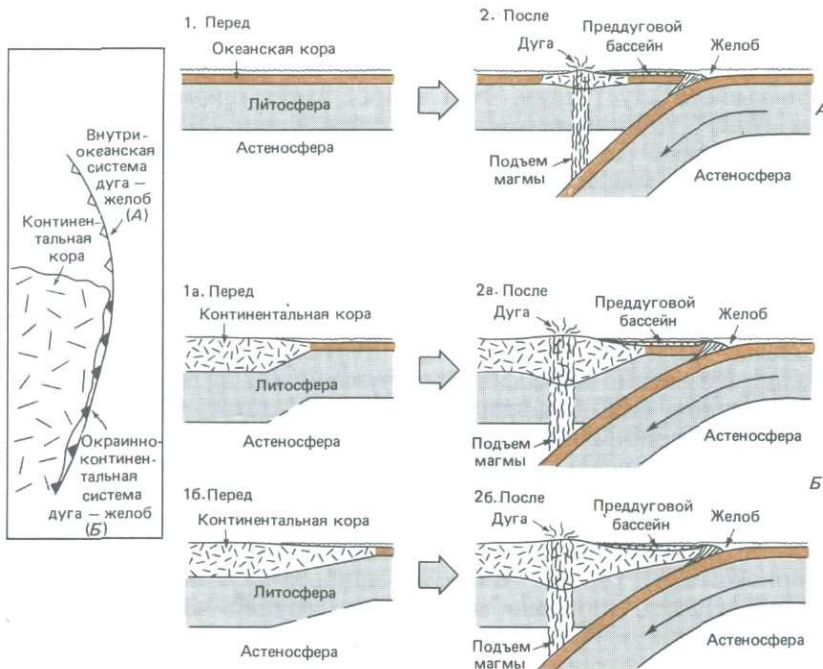
Рис. 12-18. Две модели зарождения конвергентной окраины [258]. А — раскол океанской плиты (внутриокеанская дуга); Б — активация континентальной окраины (дуга континентальной окраины). Слева на врезке показано возможное соотношение вариантов А и Б в плане.
