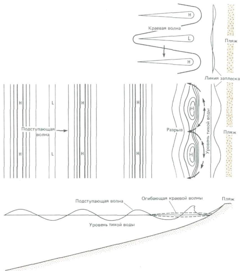
Рис. 10-8. Схема формирования разрывного течения (наверху – в плане, внизу – в разрезе). Взаимодействие между наступающими (падающими) и краевыми волнами, перемещающимися вдоль берега, создаст чередующиеся зоны высокого (H) и низкого (L) прибоя. Вдольбереговые течения расходятся от зон высокого прибоя, где нагон максимален, и сходятся в точках низкого прибоя, где возникают направленные в сторону моря разрывные течения [513].
