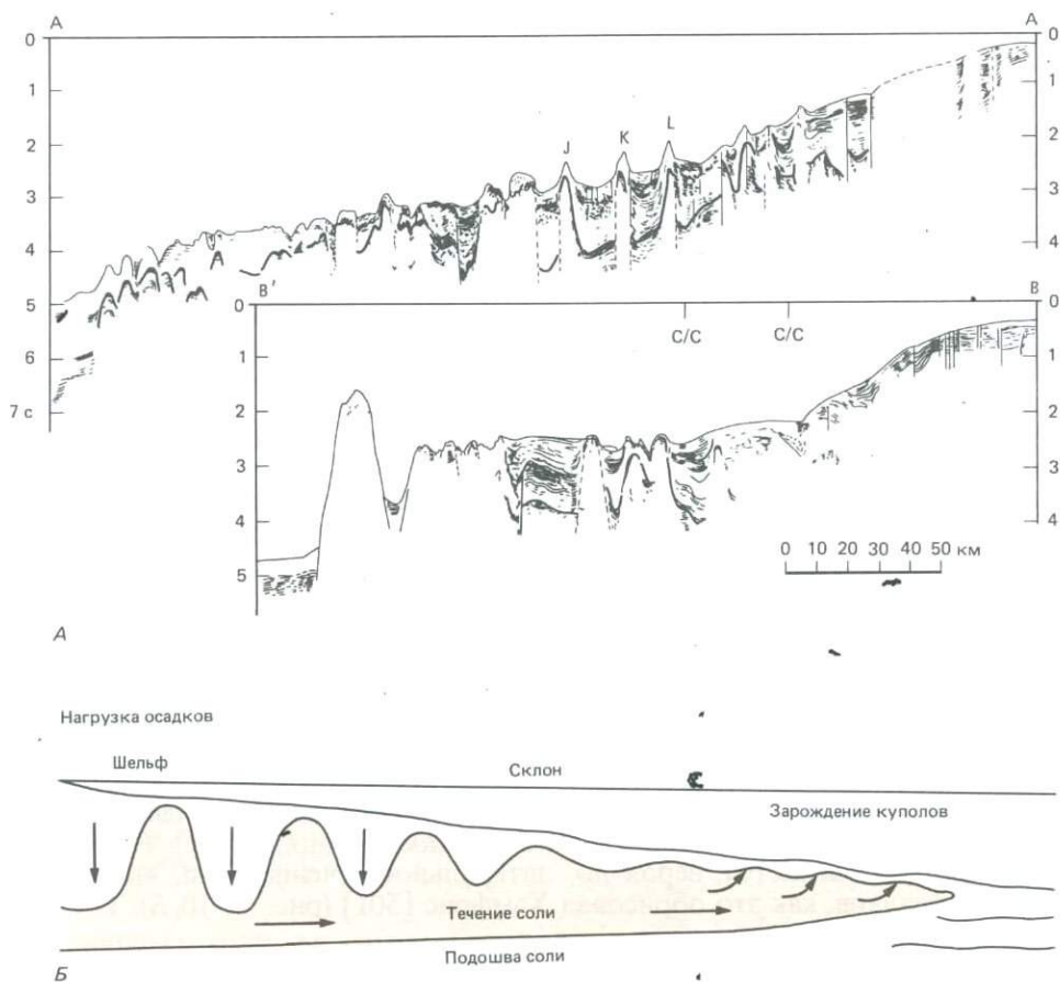
Рис. 11-10. Рост соляных куполов. А – интерпретация сейсмических профилей отраженных волн континентальной окраины Западной Африки у побережья Анголы, демонстрирующая ярко выраженные диапиры. Прямыми вертикальными линиями показаны предполагаемые сбросы. Вертикальный масштаб увеличен примерно в 20 раз [47]. Б – схема зарождения и роста соляного купола на континентальном склоне в результате нагрузки масс осадков шельфа и верхней части склона [501].
