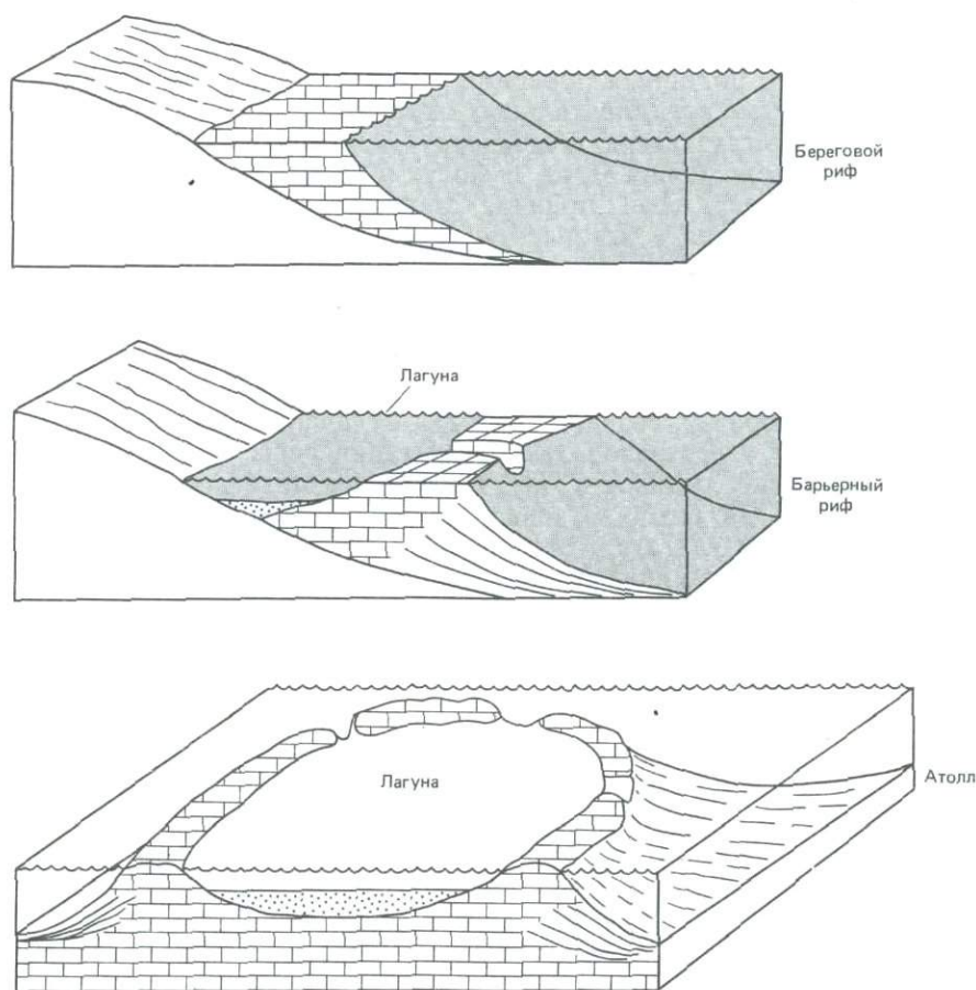
Рис. 10-17. Блок-диаграммы трех главных типов современных рифов [944].
