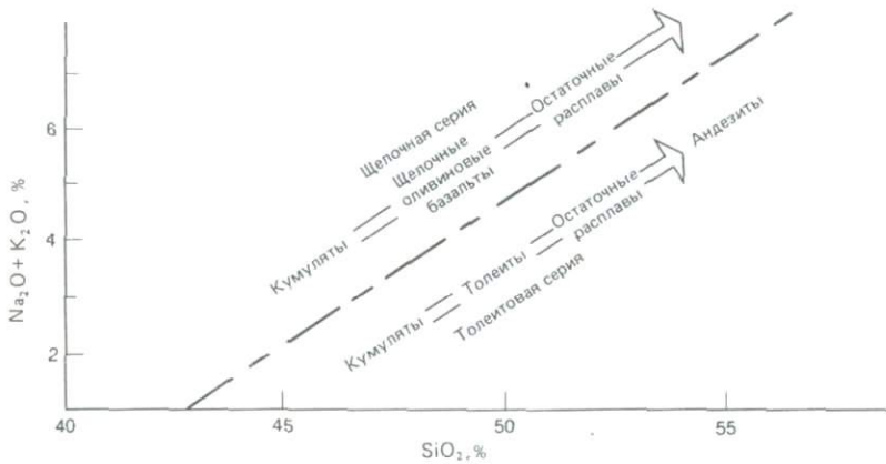
Рис. 7-5. Соотношения двух главных вулканических серий Японии, Кореи и Северо-Восточного Китая от миоцена до современности. Пунктиром обозначена граница между полями толеитовой и щелочной серий пород [618].
