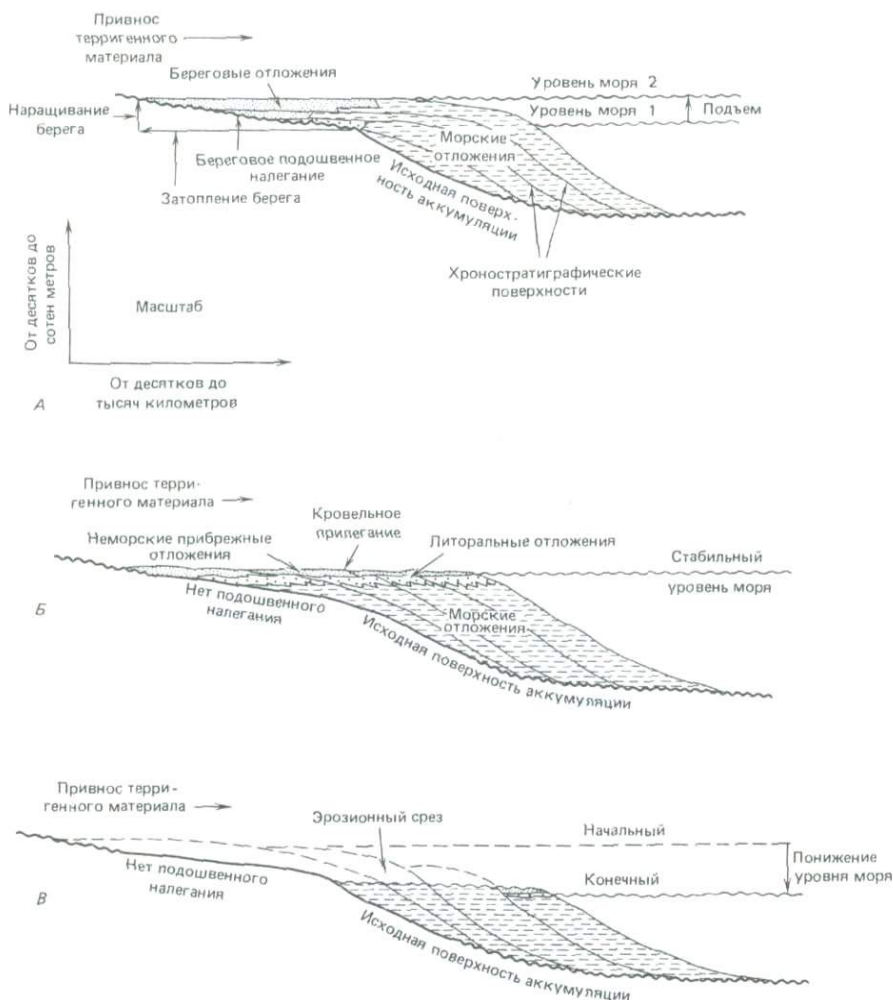
Рис. 9-7. Характер залегания отложений береговой зоны: А – при относительном повышении уровня моря; Б – при стабильном уровне; В – при понижении уровня. На разрезе А – береговое подошвенное налегание указывает на повышение уровня моря. Подъем базиса аккумуляции (base level) создает условия для наращивания береговых отложений и перекрытия ими прежней поверхности аккумуляции. На разрезе Б береговое кровельное прилегание указывает на относительную стабильность уровня моря. Без относительного подъема базиса аккумуляции неморские прибрежные и литоральные отложения не будут наращиваться, и подошвенного налегания не получится, а вместо этого проходящий транзитом осадочный материал создает кровельное прилегание. На разрезе В смещение вниз прибрежного подошвенного налегающего аккумулятивного тела указывает на опускание уровня моря. Относительное понижение базиса эрозии создает условия размыва. Осадконакопление возобновляется в виде берегового подошвенного налегания во время последующего подъема уровня [1068].
