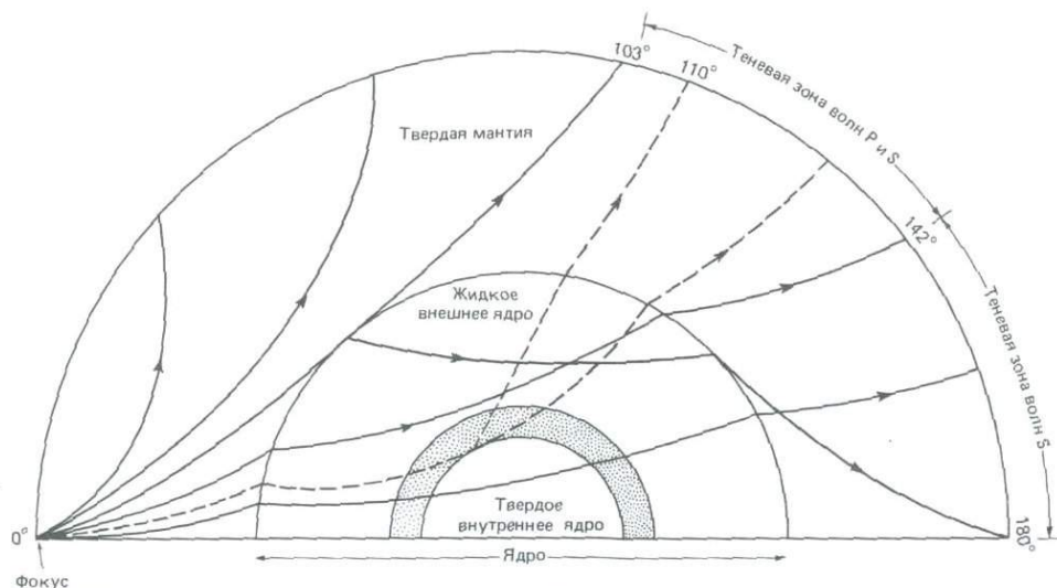
Рис. 2-1. Прохождение через земной шар лучей продольных волн (Р), служащих главным источником информации о внутреннем строении Земли [103]. Справа показаны теньевые зоны для волн Р и S. Пунктирными линиями обозначены лучи слабых Р-волн в теньевой зоне, свидетельствующие о наличии внутри ядра зоны высокой скорости продольных волн.
