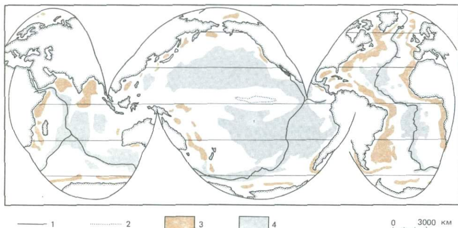
Рис. 2-19. Мощность осадочного чехла над фундаментом в Мировом океане [70]. 1—ось спрединга; 2—экваториальная линза осадков (мощность более 0,5 км); 3—осадки мощностью более 1 км; 4—осадки мощностью менее 0,1 км.
