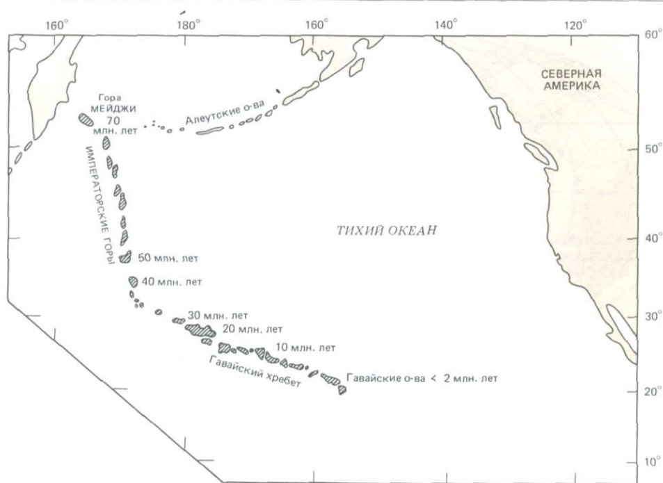
Рис. 5-19. Возраст островов и подводных гор (в млн. лет) в Гавайско-Императорской вулканической цепи [193].
