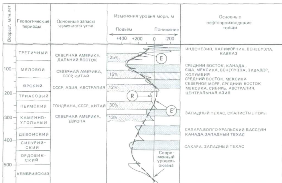
Рис. 9-12. Основные периоды накопления нефтематеринских и угленосных отложений в сравнении со всемирными трансгрессиями и регрессиями, установленными Вейлом с соавторами [1068] – Р и Питманом [840] – Е. В показанные на графике периоды накопления нефтематеринских пород образовалось более 10^8 т нефти за 1 млн. лет в первый цикл (570–200 млн. лет назад) и более 10^9 т нефти за 1 млн. лет во второй цикл (200–0 млн. лет назад) [1044].
