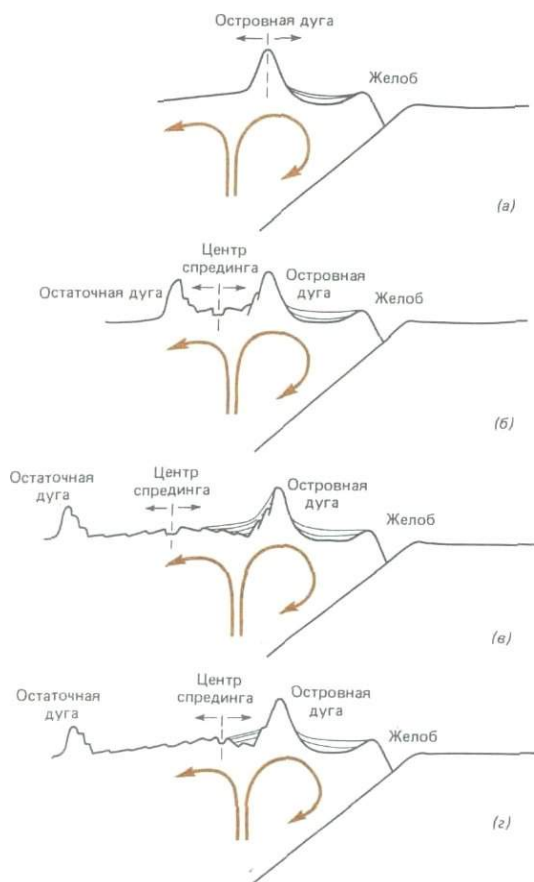
Рис. 12-13. Развитие задугового бассейна с перескоком оси спрединга. Возможная модель, объясняющая сдвиг оси спрединга в сторону активной островной дуги внутри задугового бассейна: а —движущий механизм создает поле напряжений растяжения, которое вызывает раскол активной дуги, представляющей собой ослабленную зону; б —образование бассейна с центром спрединга, расположенным посередине между двумя расходящимися дугами; в —симметричное нарастание литосферы приводит к перемещению центра спрединга в сторону от желоба и поля растяжения; г —изменение поля напряжений около центра спрединга вызывает его перескок обратно в сторону активной дуги, в результате чего ось спрединга займет асимметричное положение внутри бассейна [96, с. 95].
