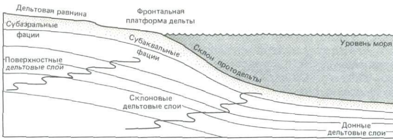
Рис. 10-3. Основные черты морфологии дельты на поперечном разрезе. Вертикальный масштаб сильно увеличен [697].
