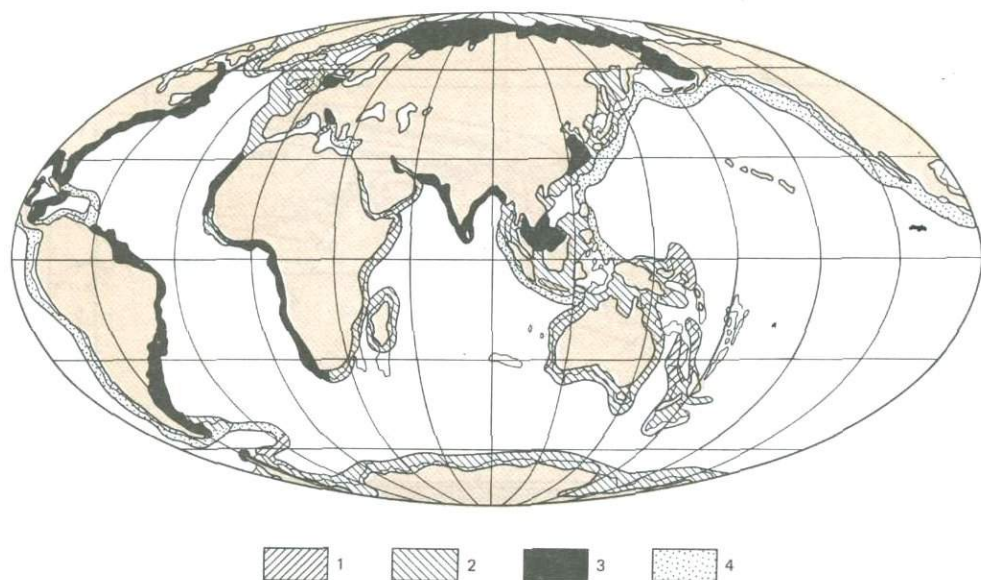
Рис. 11-12. Распространение четырех типов континентальных окраин по классификации К. О. Эмери [298]. 1—зачаточные; 2—юные или с дефицитом осадочного материала; 3—зрелые или с высокими скоростями осадконакопления; 4—конвергентные.
