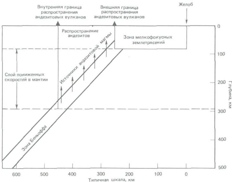
Рис. 12-9. Модель образования андезитовой магмы Хатертонга и Диккинсона [428].
