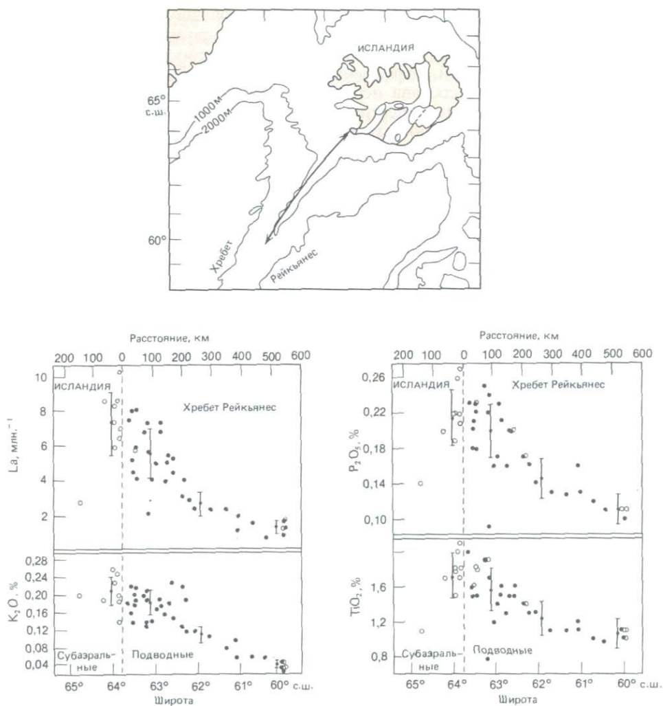
Рис. 7-8. Вариации концентраций La, K_2O , P_2O_5 и TiO_2 в толеитовых базальтах вдоль простираания хребта Рейкьянес к юго-западу от Исландии. Наблюдаются закономерные изменения. Пределы ошибок показаны вертикальными отрезками [908].
