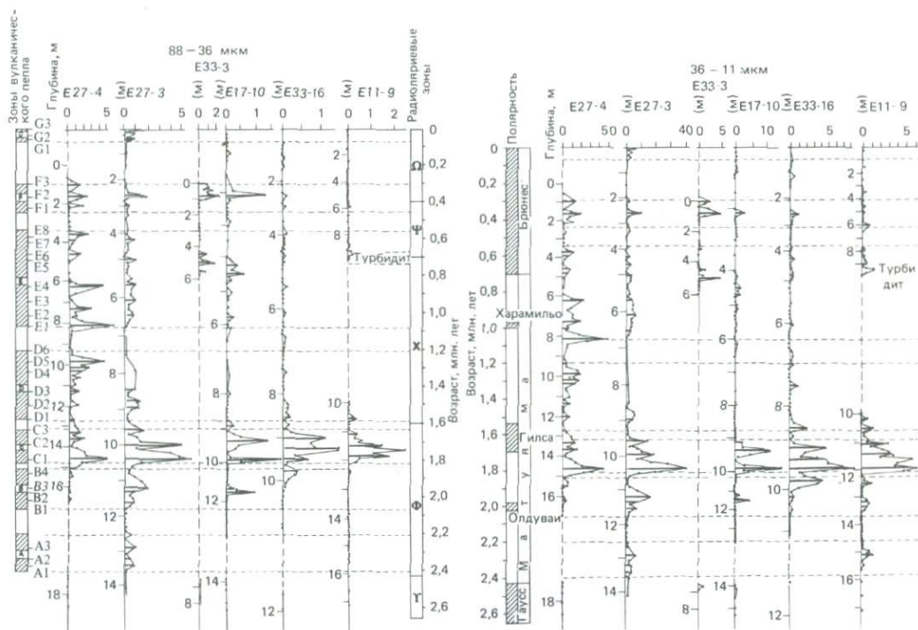
Рис. 3-3. Тефрохронология серии колонок Южного океана, взятых в секторе между морем Росса и юго-восточной частью Тихого океана. Периоды максимальных скоростей накопления вулканического стекла (в двух фракциях различной размерности слева и справа) отмечены буквами от А до G. Цифрами (от 1 до 8), помещенными возле букв, отмечены возможные единичные вулканические извержения или серии близко расположенных извержений. Скорости аккумуляции даны в абсолютных массах ( \text{мг}/(1000 \text{ лет} \cdot \text{см}^2) ). Возрасты колонок определены палеомагнитным методом. Заимствовано у Хуанга и др. [499, с. 1307]; публикуется с разрешения Геологического общества США.
