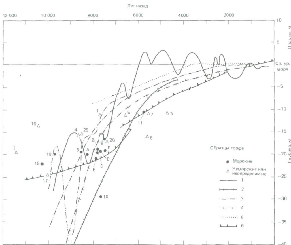
Рис. 9-3. Связь между возрастом и глубиной залегания голоценовых торфяников на восточном побережье США и ряд кривых колебаний уровня океана для последних 10 тыс. лет (по [224], с изменениями, Field et al., 1979, Geol. Soc. Amer. Bull., Part I, v. 90, p. 626). Кривые колебаний уровня: 1 — Фейрбридж, 1961 [329]; 2 — Миллиман, Эмери, 1968 [746]; 3 — Карри, 1960, 1965 [222]; 4 — Йелгерсма, 1966 (рис. 6, кривая 3); 5 — Колеман, Смит, 1964; 6 — Крафт, 1976.
