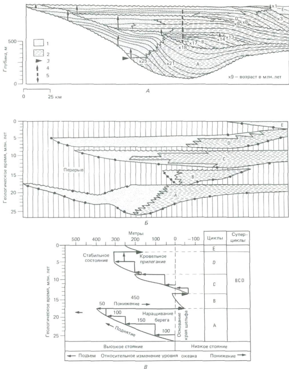
Рис. 9-6. Три этапа составления графика относительных колебаний уровня океана: А — стратиграфический разрез; Б — разрез, приведенный к шкале геологического времени; В — перевод данных на разрезе Б в региональный график циклов относительных изменений уровня океана [1068]. 1 — отложения береговой зоны; 2 — морские отложения; 3 — первоначальный край шельфа; 4 — наращивание берега; 5 — смещение вниз.
