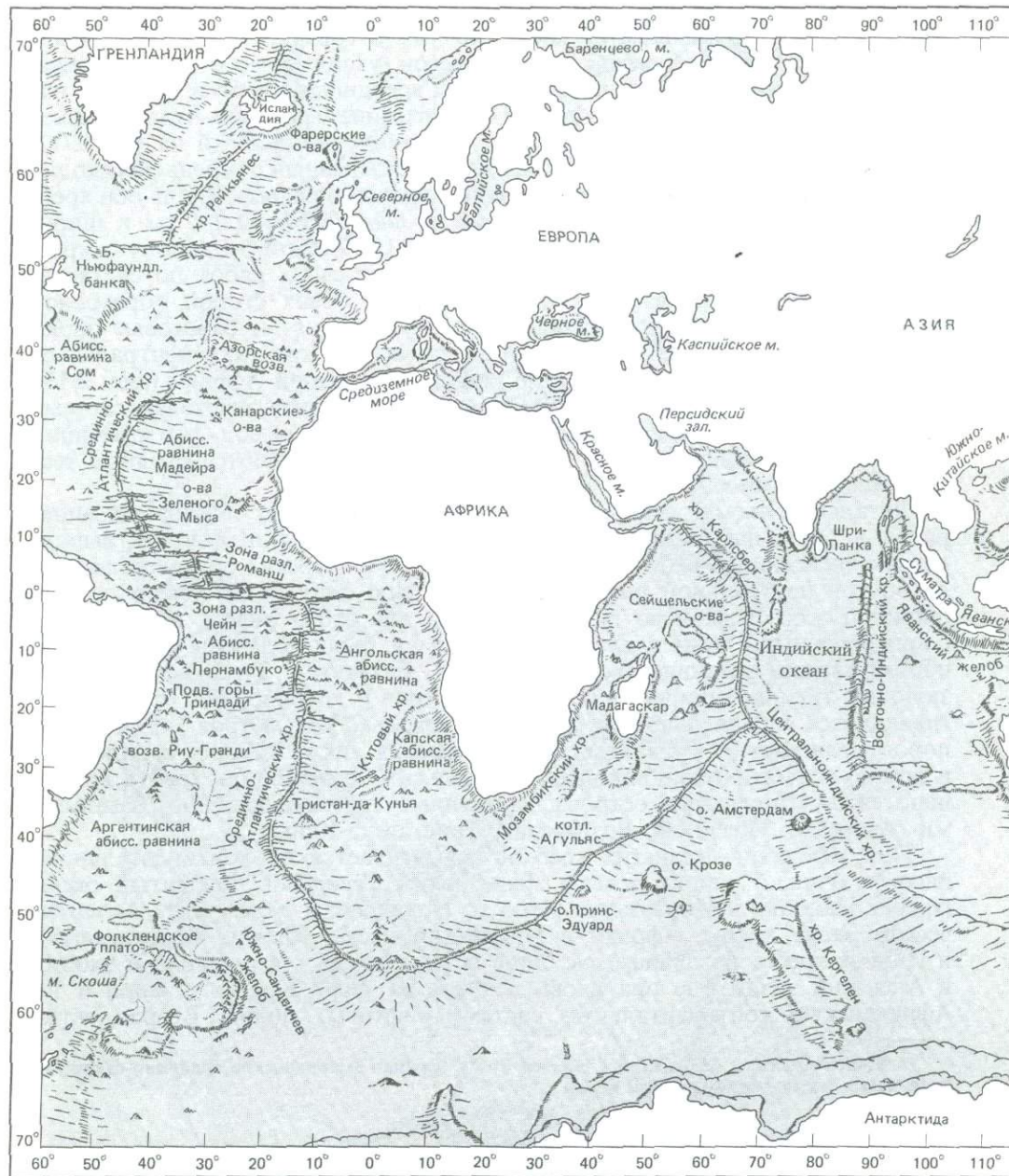
Рис. 2-11. Физиографическая карта Мирового океана; Меркаторская проекция; масштаб 1:101 000 000. (Публикуется с разрешения Hubbard Scientific Company.)
