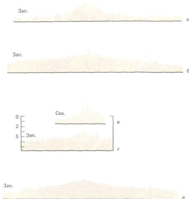
Рис. 2-12. Поперечные профили через срединно-океанские хребты [451]. На профилях Срединно-Атлантического хребта и срединных хребтов Индийского океана отчетливо видна рифтовая долина, взрезанная в сильно расчлененный рельеф гребня. На профиле Восточно-Тихоокеанского поднятия рифтовая долина отсутствует. а – Срединно-Атлантический хребет (северная часть); б – Срединно-Атлантический хребет (южная часть); в – Западно-Индийский хребет; г – Центральноиндийский хребет; д – Восточно-Тихоокеанское поднятие.
