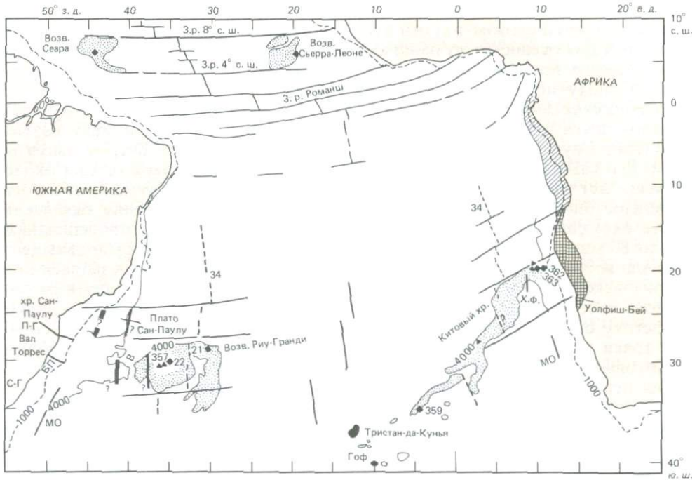
Рис. 5-22. Крупнейшие морфологические и тектонические элементы экваториальной и южной частей Атлантического океана [617]. Обратите внимание на парные асейсмичные хребты: возвышенность Риу-Гранди–Китовый хребет, возвышенности Сеара–Сьерра-Леоне. Каждая пара ограничена с севера и юга зонами разломов. Диагональной штриховкой показаны зоны соляных диапиров, сеткой–площади перекрытия на реконструкции предрифтового положения континентов. Показаны магнитные аномалии 34 (80 млн. лет) и МО и скважины глубоководного бурения (точки с цифрами) З.р.–зоны разломов; ПГ–вал Понта-Гросса; С-Г–вал Сан-Габриель; В–проход Вима; БП–бассейн Петола; Х.Ф.–хребет Фрио.
