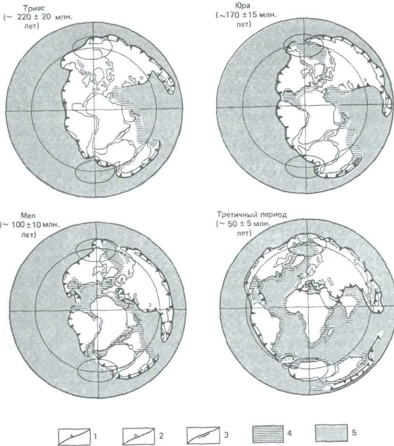
Рис. 11-2. Стадии раскола Пангеи. Реконструкция по Брайдену и др. [132] с упрощениями Балли [31]. Равноплощадная проекция Ламберта. 1—зона субдукции (на мезозойских реконструкциях); 2—зона субдукции (на третичной реконструкции); 3—трансформный разлом (на третичной реконструкции); 4—пассивная окраина; 5—океанская кора.
