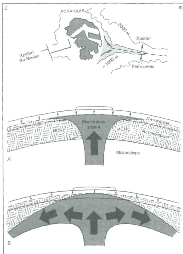
Рис. 7-10. Две модели мантйнной струи (плюмажа), предложенные Шиллингом [908] для объяснения наблюдаемых геохимических градиентов вдоль хребта Рейкьянес, к юго-западу от Исландии. Заштрихована зона глубин, где может начаться восходящее внедрение магмы. На модели А первичная мантйнная струя около Исландии поднимается быстро вдоль оси спрединга. На модели Б восходящая мантйнная струя с боков постепенно погружается, приобретая форму грозовой тучи; скорость разгрузки больше, чем на модели А. ИСНС – источник низких скоростей сейсмических волн [908].
