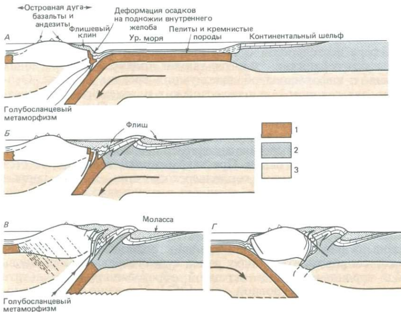
Рис. 12-22. Разрезы, иллюстрирующие последовательность событий при столкновении континентальной окраины атлантического типа с островной дугой, за которым последовало изменение направления подвига плит [252, с. 2611]. Слои литосферных плит: 1 – океанская кора; 2 – континентальная кора; 3 – мантия.
