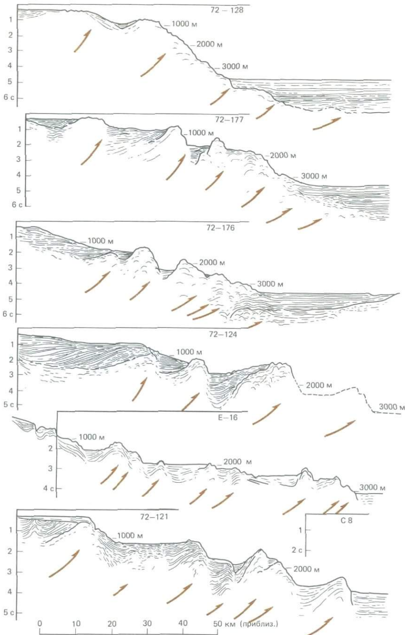
Рис. 12-17. Сейсмические профили через восточную континентальную окраину острова Северный Новая Зеландии. Профили пересекают аккреционный бордерленд (см. рис. 12-16), и на них ясно видны последовательные ступени внутри аккреционной призмы. Верхний, самый северный профиль относится к северной части залива Хокс-Бей, нижний, самый южный проходит на юго-восток от Веллингтона. С правой стороны на всех профилях видны осадки трога Хижуранги, имеющие плиоцен-плейстоценовый возраст и представленные (почти наверняка) турбидитами. Осадками показано вероятное положение взбросов с большой сдвиговой составляющей смещения. Вертикальная шкала слева — время двойного прохождения акустического сигнала (в секундах). Цифры над склоном — глубина от уровня океана. Горизонтальный масштаб приблизительный. Линия с наклоном 45^\circ на профиле соответствует уклону около 6^\circ по отношению к линии профиля [200].
