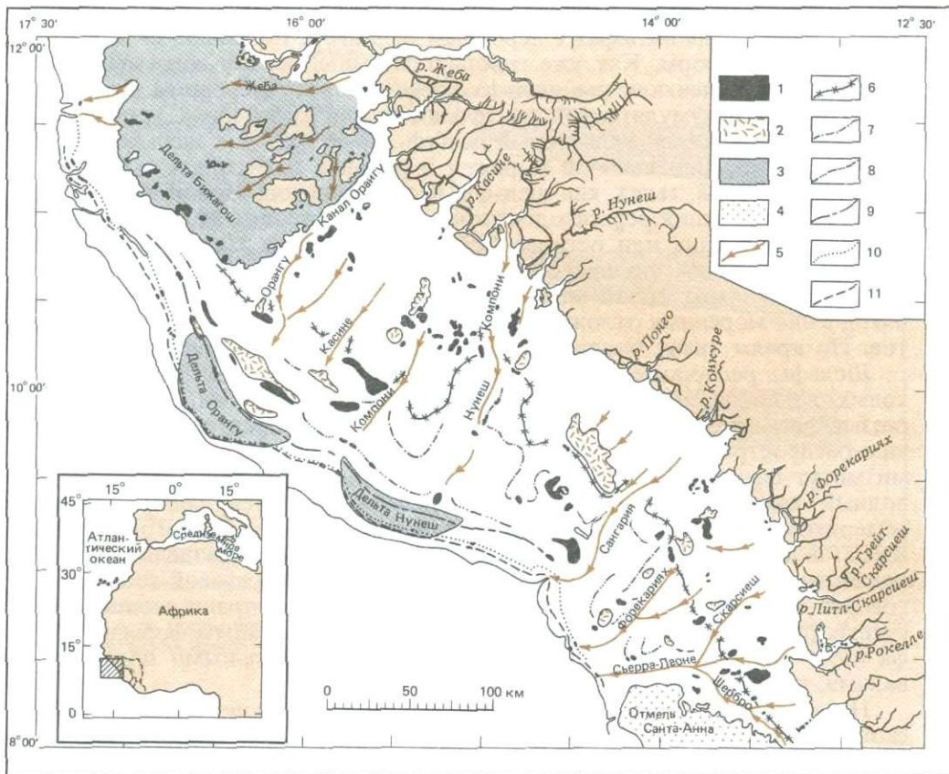
Рис. 10-13. Геоморфологические элементы континентального шельфа Западной Африки у побережья Гвинеи-Бисау и Сьерра-Леоне [727]. 1 – прибрежные гряды; 2 – прибрежные депрессии; 3 – дельты; 4 – отмели; 5 – протоки; 6–11 – древние затопленные береговые линии (в метрах ниже уровня моря); 6–25 м, 7–35 м, 8–45 м, 9–55 м, 10–80 м, 11–90 м.
