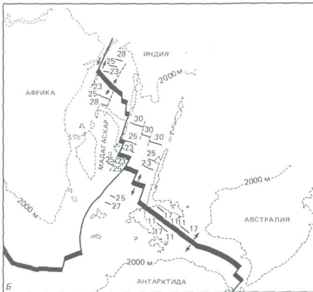
Рис. 6-11. Палеорекострукции плит и их границ в Индийском океане: 75 млн. лет назад (поздний мел) и 36 млн. лет назад (ранний олигоцен). Цифрами на схеме Б обозначены номера магнитных аномалий [725].
