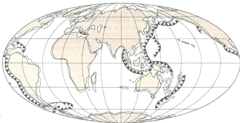
▲▲▲▲▲▲▲▲ Зоны субдукции
