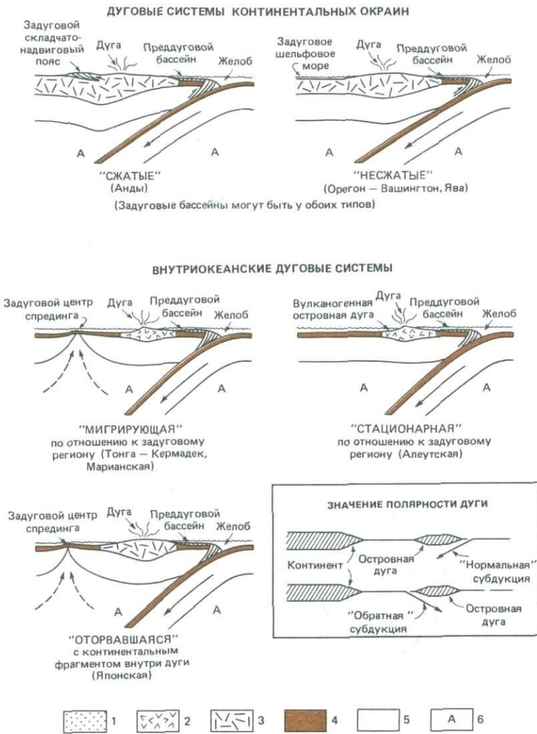
Рис. 12-5. Тектонические обстановки в системе желоб–дуга, восстановленные по задуговым структурам [258]. 1–преддуговые осадки; 2–вулканогенная земная кора островной дуги; 3–континентальная кора; 4–океанская кора; 5–мантийная часть литосферы; 6–астеносфера.
