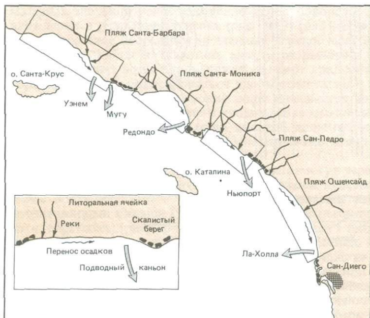
Рис. 10-9. Побережье южной Калифорнии с ячейчистым расчленением пляжевой зоны. В каждую из ячеек («карманных пляжей») песок вносится реками. Далее он переносится вдоль берега в южном направлении и перехватывается верховьями подводных каньонов, подходящими близко к берегу. По каньонам мелководные осадки выносятся в океан на большие глубины [515].
