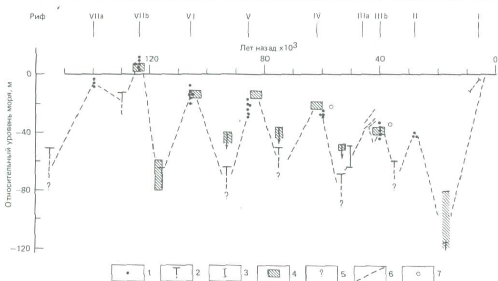
Рис. 9-4. Флуктуации уровня океана за последние 140 тыс. лет, определенные по возрастам и высоте террас коралловых рифов на тектонически активных побережьях при допущении постоянной скорости тектонического воздымания [109]. 1 — датированные вершины коралловых рифов Новой Гвинеи; 2 — недатированные рифовые комплексы Новой Гвинеи, максимально низкий уровень моря; 3 — датированные рифовые комплексы Новой Гвинеи; 4 — данные по острову Барбадос; 5 — минимальный уровень моря неизвестен; 6 — диаграмма изменений уровня моря; 7 — рассчитанный уровень моря.
