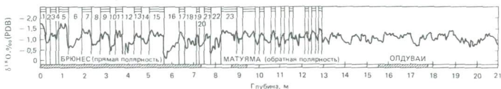
Рис. 3-12. Колебания соотношения изотопов кислорода в кальците раковин планктонных фораминифер за последние 2 млн. лет, выраженные в виде отклонений от использованного Эмилиани стандарта В-1 и сопоставленные с палеомагнитными данными по колонке поршневой трубки V28-239. Номера изотопных стадий (от 1 до 23) приведены по Эмилиани [Emiliani, 1955, 1966], Шеклону и Опдайку [952]. Последние 0,7 млн. лет (Брюнес) содержат ледниковые стадии с амплитудами, превышающими 1‰, и периодом около 100 тыс. лет. Изотопные минимумы различных стадий близки. Вторая половина Матуямы (~1,4–0,7 млн. лет) характеризуется изотопными флуктуациями с периодом около 40 тыс. лет и амплитудами ниже (0,7‰), чем в Брюнесе [953].
