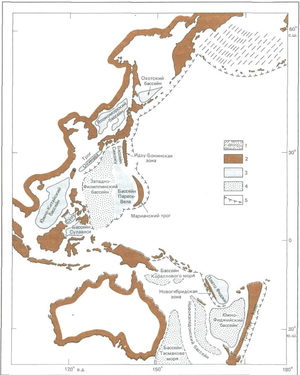
Рис. 12-11. Распространение окраинных (задуговых) бассейнов в западной части Тихого океана, классифицированных по стадиям развития [544]. 1 – неразвитая стадия; 2 – стадия активного спрединга; 3 – зрелая стадия; 4 – неактивная стадия; 5 – желоб.
