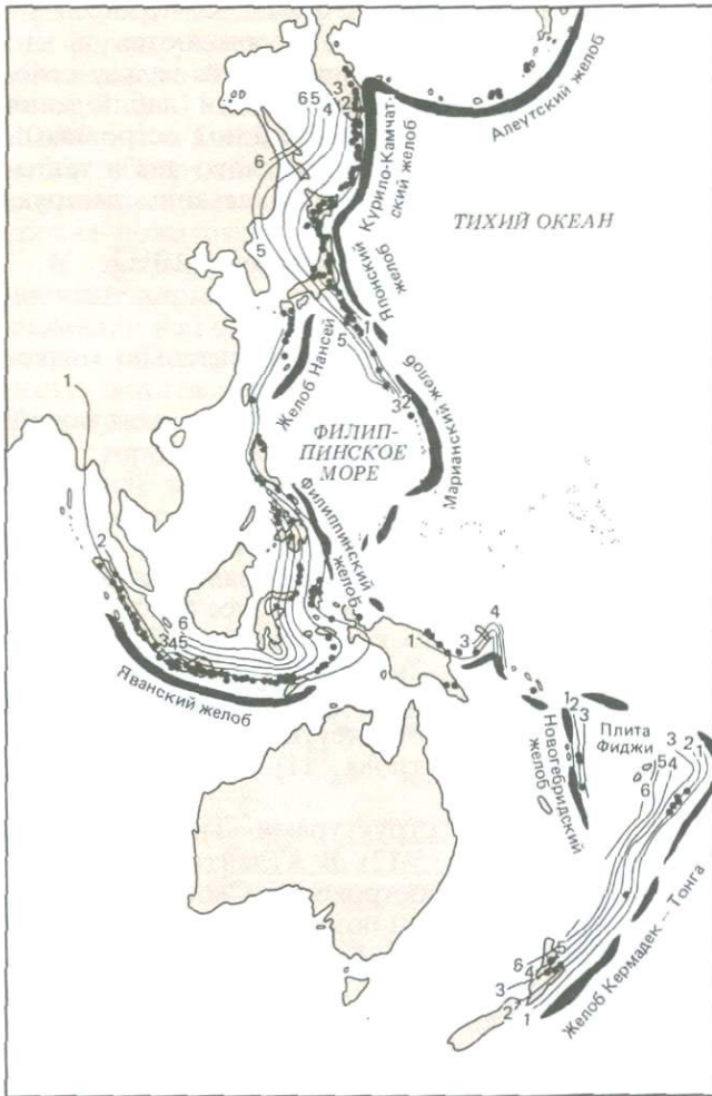
Рис. 5-12. Распределение глубоководных желобов, вулканов и изолинии глубины погружения зон Бенъофа (в 10^2 км от уровня океана) в западной части Тихого океана [804, 805].
