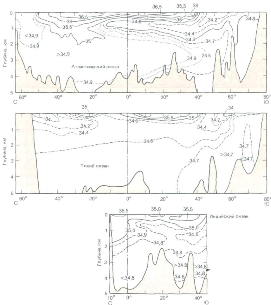
Рис. 8-12. Изменение солёности (‰) по вертикали в трех океанских бассейнах [259].
