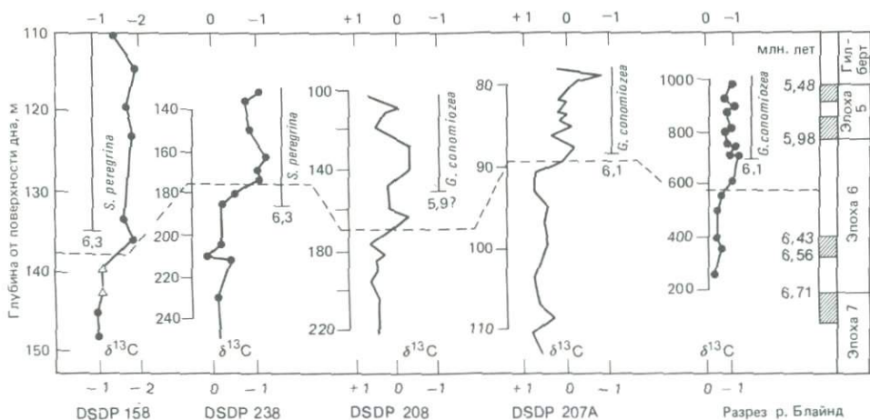
Рис. 3-13. Колебания соотношения изотопов углерода ( \delta^{13}\text{C} ) с глубиной в ряде позднемiocеновых морских разрезов. Пунктирной линией показана предполагаемая изохронная поверхность изотопно-углеродного сдвига в каждом разрезе. Возраст этого сдвига, установленный палеомагнитным методом в разрезе реки Блайнд (справа), равен 6,1 млн. лет.
