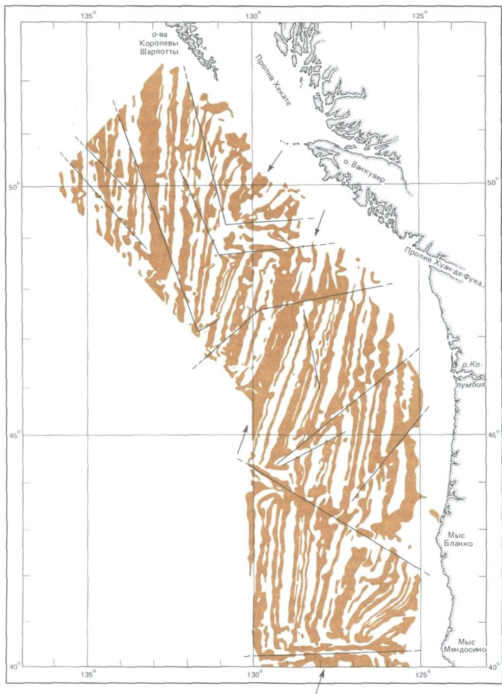
Рис. 4-5. Аномалии магнитного поля на ложе океана у западного побережья Северной Америки (штаты Орегон, Вашингтон и провинция Британская Колумбия) [696]. Коричневым показаны положительные аномалии, белым — отрицательные. Стрелки указывают на оси трех коротких хребтов (с севера на юг): Эксплорер, Хуан-де-Фука и Гордон. Линейные аномалии смещаются многочисленными разломами [696].
