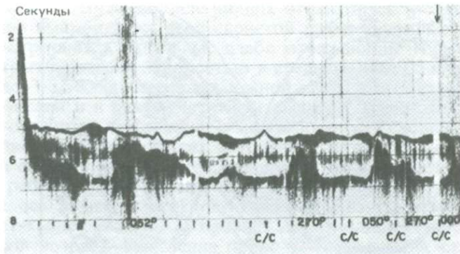
Рис. 2-18. Сейсмопрофиль через Северо-Американскую котловину северо-восточнее Бермудских островов. В средней части осадочной толщи виден отражающий горизонт А. Резкий пик на левом конце профиля – подводная гора, расположенная примерно в 300 км от Бермудских островов [318].
