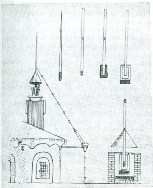
Молниеотвод конструкции Д. А. Голицына на замке Росендал в Голландии. Чертеж с рисунка Д. А. Голицына Из книги «Дмитрий Алексеевич Голицын»
