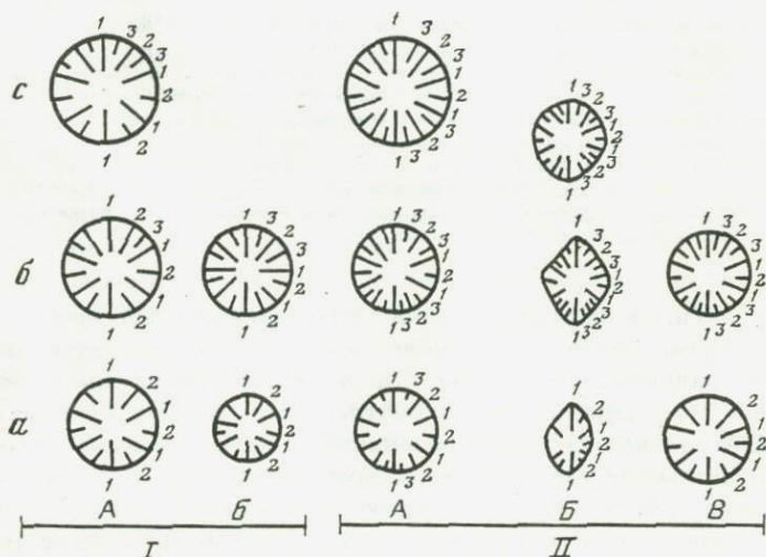
Рис. 3. Схема развития септ в blastогенезе
