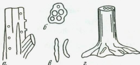
Рис. 33. Схема строения скелетных образований склераксоний Kaluginella turkmenensis Kustm. экз. N 223/183
