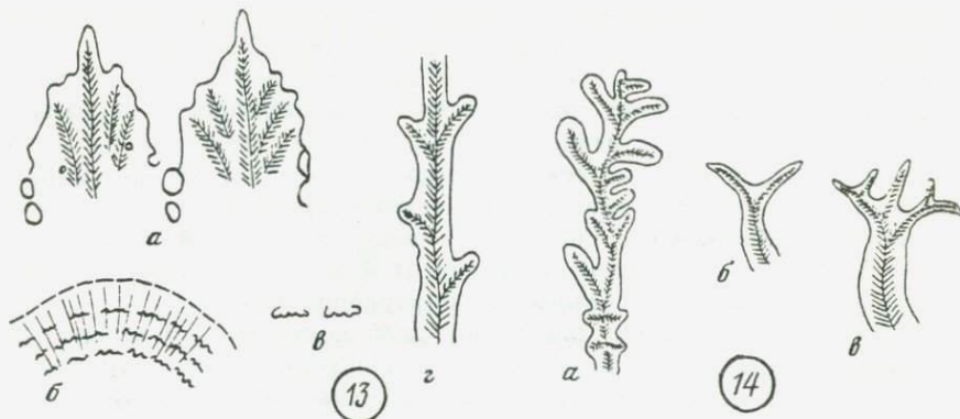
Рис. 13. Строение скелетных элементов Lithophyllon prior (Opp.); экз. N 185/330 а — дистальные края септокост ( \times 50 ); б — боковая поверхность септокосты ( \times 6 ); в — две пеннулы сбоку ( \times 15 ); г — септокоста в поперечном сечении (35)
