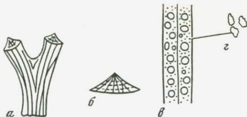
Рис. 34. Схема строения склераксонии Parisis melitensis Morr.; экз. N 223/97
