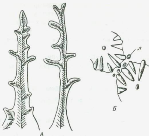
Рис. 8. Строение скелетных элементов
