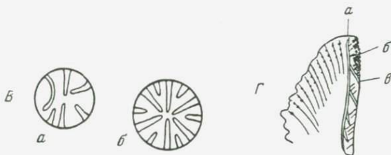
Рис. 24. Расположение септ на ранних стадиях онтогенеза
