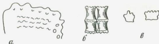
Рис. 30. Строение скелетных элементов Thecopsammia cylindrica Kusm., sp. nov.; экз. N 185/872
