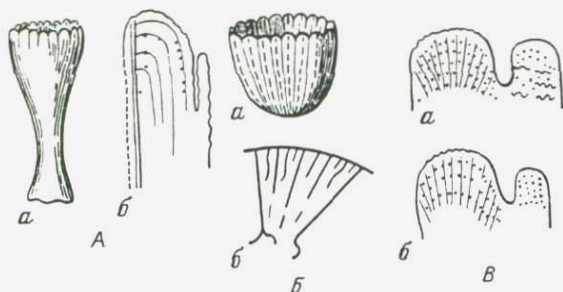
Рис. 23. Строение скелетных элементов
