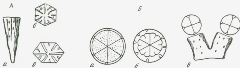
Рис. 25. Строение скелетных элементов
