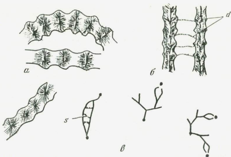
Рис. 4. Строение скелетных элементов Mesomorpha ryanovskae Kuzm.: экз. N 103/29 а — септокости в поперечном сечении ( \times 70 ); б — продольное сечение двух септокоств ( \times 40 ). б — различные типы дихотомического ветвления септокоств: s — притрабекулярные бруски, d — диссепименты, с — столбики в осевых частях кораллитов (Кузьмичева, 1970)
