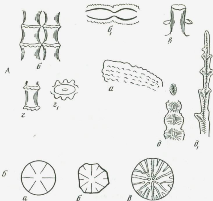
Рис. 12. Строение скелетных элементов Trochoseris helianthoides Römer; экз. N 185/325
