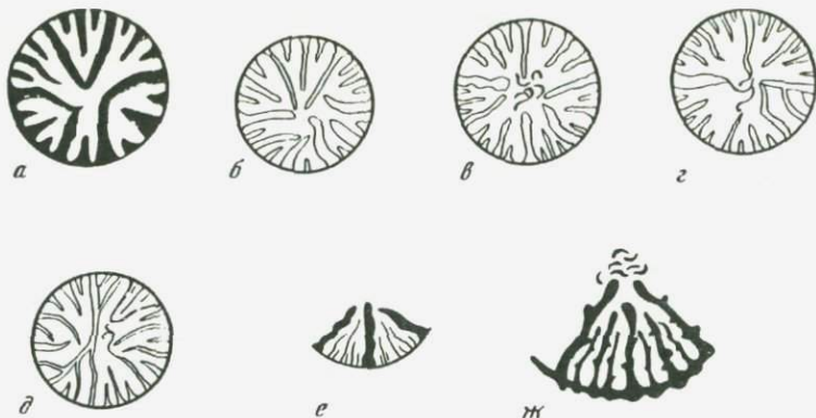
Рис. 27. Заложение септ в онтогенезе Palaeopsammia multiformis Wann.; экз. N 185/124 а — при d = 2.5 мм ( \times 12 ); б — при d = 2.8 мм ( \times 10 ); в — при d = 2.9 мм ( \times 10 ); г — при d = 3 мм ( \times 10 ); д — при d = 3.2 мм ( \times 9 ); е — при d = 3.5 мм (деталь) ( \times 9 ); ж — при d = 8 мм ( \times 5 )
