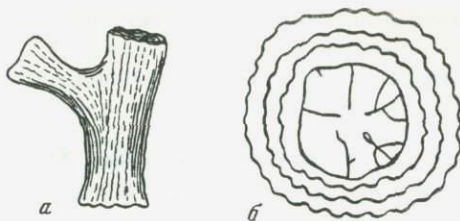
Рис. 29. Внешний облик юной колонии и строение ее протокораллита у Dendrophyllia weselovi Kusm., sp. nov.; экз. N 185/870
