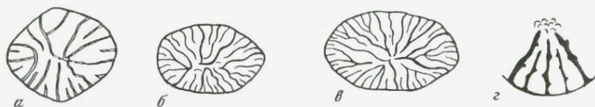
Рис. 26. Заложение септ в онтогенезе Aplopsammia collignoni All.; экз. N 185/127
