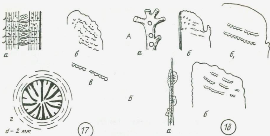
Рис. 17. Строение скелетных элементов Tarbellastraea ukrainica Kasm. sp. nov.: экз. N 185/507
