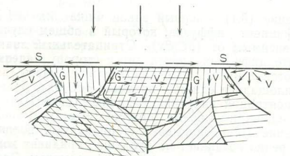
Рис. 8.1. Схематическое изображение путей поверхностной диффузии S , межзерновой диффузии G и объемной диффузии V .
