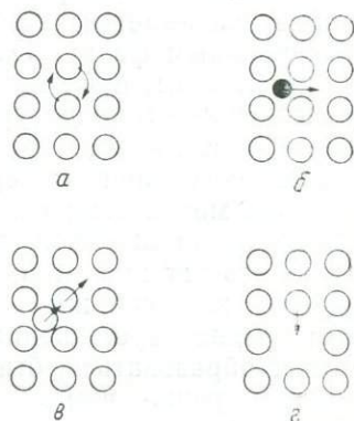
Рис. 8.7. Четыре главных типа механизма объемной диффузии: обменный механизм (а), диффузия по междоузлиям (б), диффузия по междоузлиям с вытеснением (в), перемещение вакансий (г).
