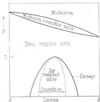
Рис. 8.15. Фазовая диаграмма бинарного твердого раствора с разрывом смешимости при низких температурах.
