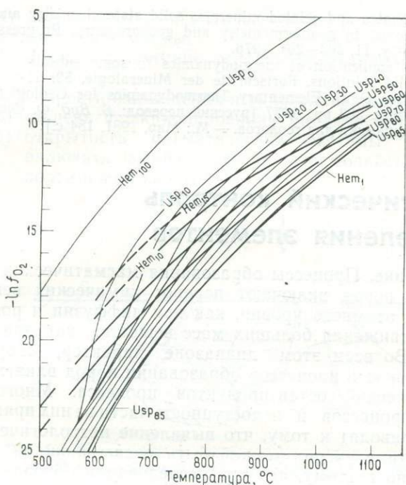
Рис. 7.11. Связь температуры, фугитивности кислорода ( \lg f_{O_2} ) и состава (мольные проценты) сосуществующих ильменит-гематитового и магнетит-ульвошпинелевого твердых растворов [41].
