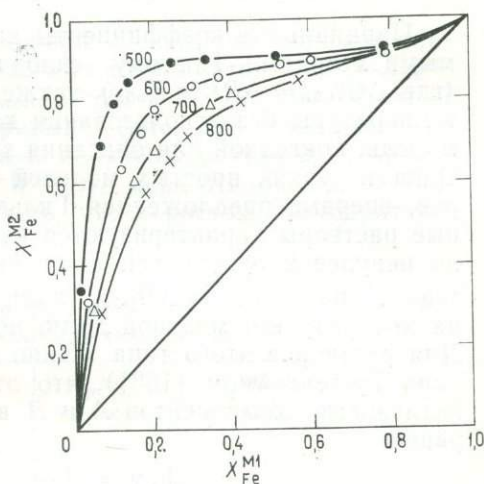
Рис. 7.3. Распределение \text{Fe}^{2+} между структурными позициями М1 и М2 (в ионных долях) в ортопироксене, нагретом до 500, 600, 700 и 800 °С [342].
