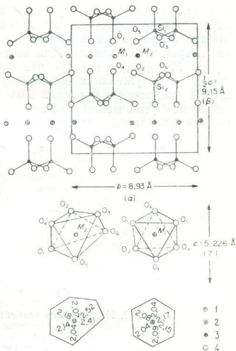
Рис. 6.1. Кристаллическая структура ортопироксена, проекция на (001). Показаны кислородные координационные полиэдры в проекциях (100) и расстояния металл — кислород (в Å) в каждой позиции. 1 — M_1 ; 2 — M_2 ; 3 — кремний; 4 — кислород. (По работе [44] (с разрешения), на основании данных работы [133]).
