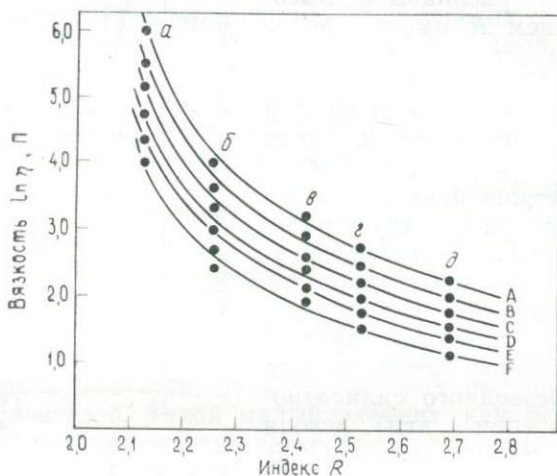
Рис. 6.5. Зависимость между вязкостью, температурой и составом расплава при давлении 1 атм. Типы расплавов те же, что и на рис. 6.4. Температуры ( ^{\circ}\text{C} ): А — 1150; В — 1200; С — 1250; D — 1300; E — 1350; F — 1400 [345].
