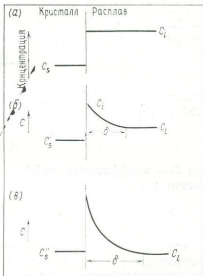
Рис. 8.12. Концентрационный профиль микроэлемента вблизи поверхности раздела кристалл—жидкость. a — равновесное распределение при бесконечно малой скорости кристалла; b — типичное распределение при конечной скорости роста кристалла; a — стационарное распределение при очень большой скорости роста кристалла. \delta — толщина диффузионного пограничного слоя [179].
