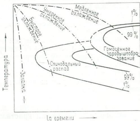
Рис. 8.17. ТТТ-диаграмма. Эффективные кривые начала (1%) и конца (99%) спинодального распада и гомогенного зародышеобразования для гипотетической системы. Четыре кривые охлаждения показывают различные скорости охлаждения на действие различных процессов кристаллизации.
