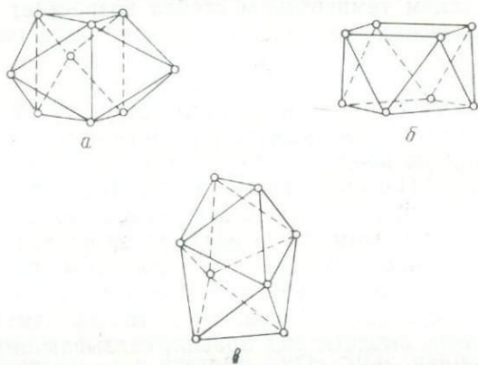
Рис. 6.8. Примеры возможных полиэдров в случайной упаковке твердых шаров. а — тригональная призма в сочетании с тремя полуоктаэдрами; б — архимедова антипризма; в — тетрагондодикаэдр [19].
