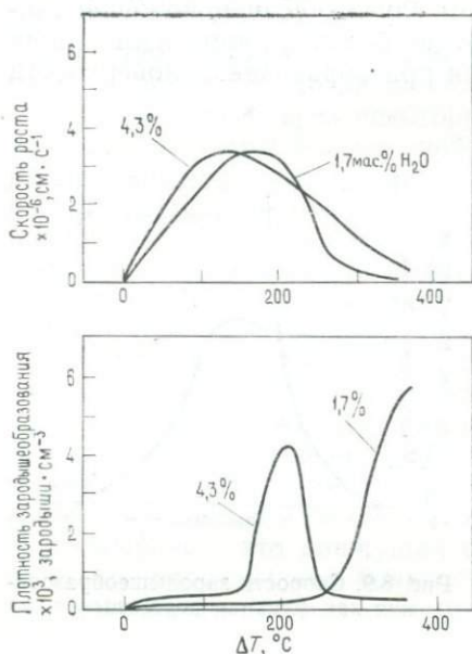
Рис. 8.10. Графики плотности зародышеобразования (числа зародышей в 1 \text{ см}^3 ) и скорости роста щелочного полевого шпата ( \text{Na}_{0,7}\text{K}_{0,3}\text{AlSi}_3\text{O}_8 ) как функций переохлаждения \Delta T в расплавах с 1,7 и 4,3 мас. % воды [107].
