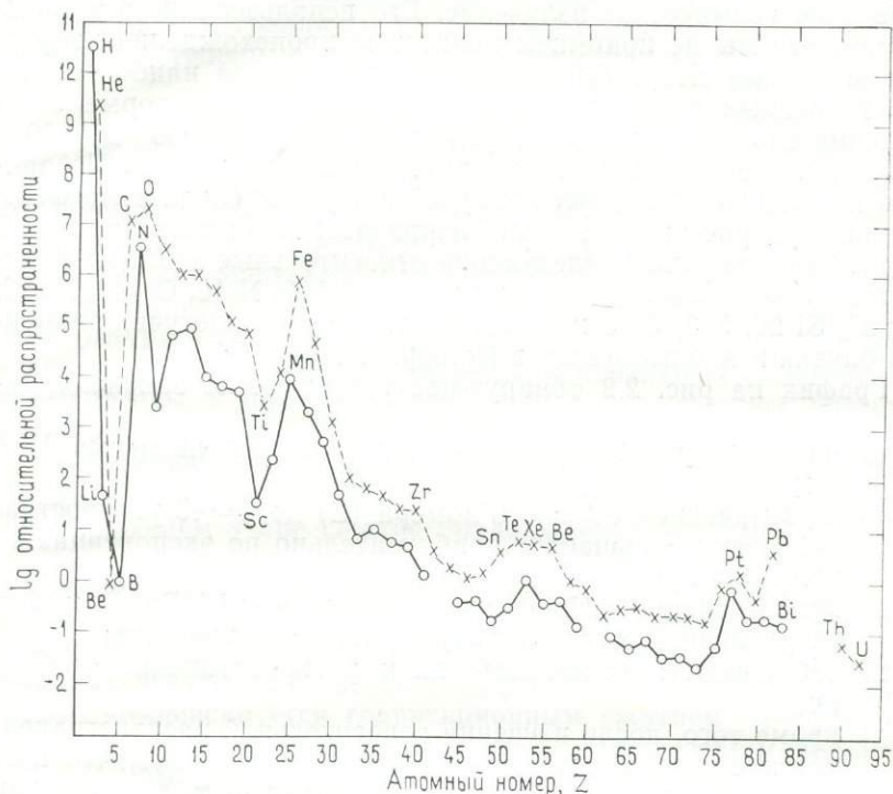
Рис. 2.2. Распространенность элементов в Солнечной системе (нормировано на 10^6 атомов Si) ([52]; значение для бора взято из работы [78]). Крестиками обозначены элементы с четными, кружками — с нечетными атомными номерами.
