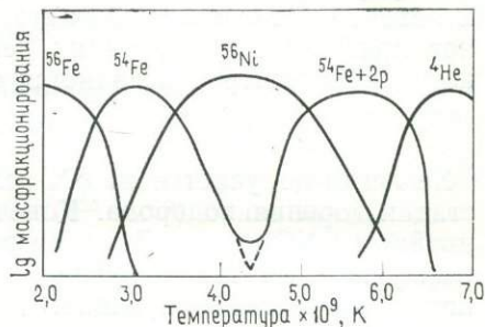
Рис. 2.4. Схематическая диаграмма, изображающая зависимость распространенности главных нуклидов, образовавшихся при горении кремния, от температуры. При относительно низкой температуре и сравнительно медленном горении стабильным нуклидом должен быть ^{56}\text{Fe} , а при более высокой температуре становится стабильным ^{56}\text{Ni} . Видна сильная зависимость состава от температуры [65].
