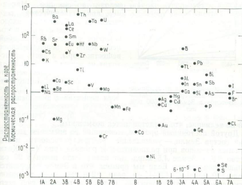
Рис. 4.5. Состав коры, нормализованный по космической распространенности и отнесенный к Si = 10 6 атомов. Диаграмма имеет тот же масштаб, что и рис. 4.3, с которым ее можно сравнить.
