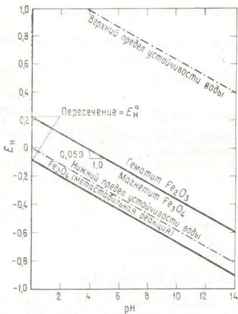
Рис. 10.2. Границы железо—магнетит и магнетит—гематит в виде функции E_H и pH ; температура 25^\circ C , общее давление 1 атм [127]. Точки пересечения оси E_H линиями равновесия дают значения E_H^0 . Граница Fe-Fe_3O_4 находится за нижним пределом устойчивости воды, поэтому соответствующая реакция (10.54) метастабильна.
