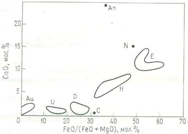
Рис. 1.4. Классификация ахондритов по содержанию CaO (мас. %) и отношению мольных долей FeO/(FeO + MgO). Контурсы примерно соответствуют составам полей различных групп: Au — обриты; U — уреилиты; D — диогениты; H — говардиты; E — эвкриты. Точки соответствуют только одному анализу из следующих групп метеоритов: C — шассиньит; N — наклит; Ap — ангрит [211].
