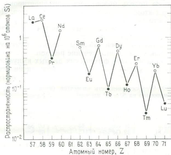
Рис. 2.1. Спектр распространенности редкоземельных элементов в осадочных породах, использованный Зюссом и Юри для оценки распространенности элементов в Солнечной системе (см. текст). Светлые кружки — элементы с четными Z , темные кружки — с нечетными Z .
