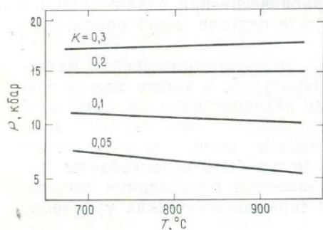
Рис. 7.7. Изолинии K для равновесия \text{CaAl}_2\text{Si}_2\text{O}_8 = \text{CaAl}_2\text{SiO}_6 + \text{SiO}_2 , плагиоклаз клинопироксен кварц (Стандартное состояние — чистые фазы при заданных P и T ) [446].
