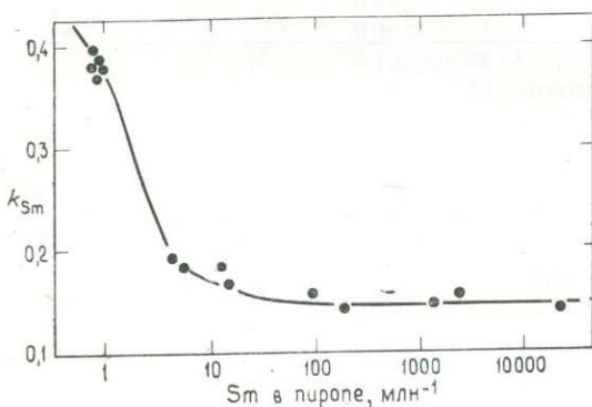
Рис. 7.6. Изменение коэффициента распределения Sm (пироп/жидкость, k_{Sm} ) как функции концентрации Sm в пиропе ( 1300^\circ C , 30 кбар) [163].
