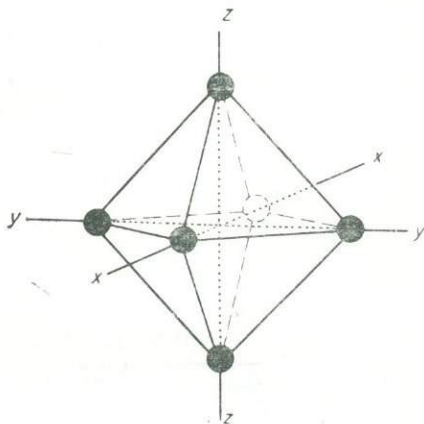
Рис. 6.14. Схематическая диаграмма расположения лигандов в октаэдрической координации.
