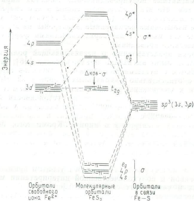
Рис. 6.20. Схема энергетических уровней \sigma -молекулярных орбиталей в пирите \text{FeS}_2 . Орбитали в связи \text{Fe-S} — орбитали атомов серы, участвующие в этой связи.
