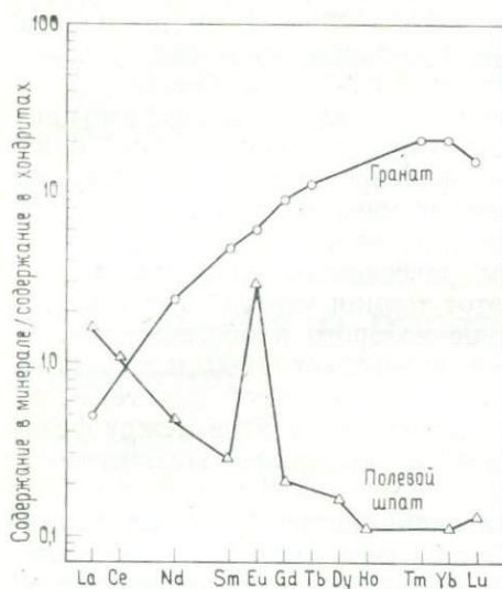
Рис. 5.1. Диаграмма Масуды — Кориэлла или нормализованный по хондритам спектр редкоземельных элементов в полево шпате и гранате из гранатосодержащего анортозита. По ординате отложены нормированные концентрации в логарифмической шкале, по абсциссе — атомные номера. Высокое содержание Eu по сравнению с другими р. з. э. в полево шпате называется «положительной европиевой аномалией». Европиевые аномалии могут быть и в других минералах и породах; см. гл. 3, разд. 3, 4, 5 и рис. 3.4 и 3.5, где обсуждаются и приводятся примеры нормированных по хондритам спектров р. з. э. для лунных пород.
