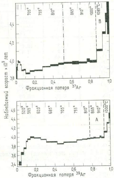
Рис. 3.2. Спектры потери аргона для брекчий «Аполлона-16». Нижняя диаграмма показывает наблюдаемый возраст, соответствующий фракционной потере ^{39}\text{Ag} ; он в основном определяется потерей Ag из богатых K и бедных Ca аксессуарных минеральных фаз. На верхнем графике изображен наблюдаемый возраст, соответствующий фракционной потере ^{37}\text{Ag} , отражающего состав Ag в кальциевом плагиоклазе. ( ^{37}\text{Ag} образуется при (n, \alpha )-реакции ^{40}\text{Ca} .) Заметно хорошо выраженное плато в средней части графика, отвечающее возрасту 3,98 млрд. лет [207].
