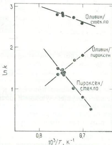
Рис. 7.9. Распределение Ni между оливином и стеклом, пироксеном и стеклом, оливином и пироксеном как функция температуры ( \text{K}^{-1} ) [157].
