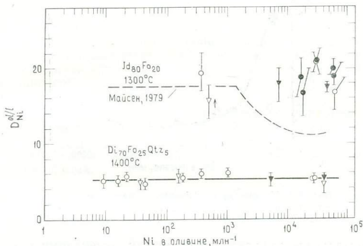
Рис. 7.5. Коэффициент распределения Ni (оливин/синтетический расплав, D_{Ni^{ol/l}} ) как функция концентрации Ni в оливине [92]. Экспериментальное определение Дрейка и Холлоуэя [92] для двух синтетических систем. В обеих системах распределение не зависит от концентрации. Пунктирная линия показывает изменение коэффициента распределения по измерениям Майсена [274]. Обсуждение см. в тексте.
