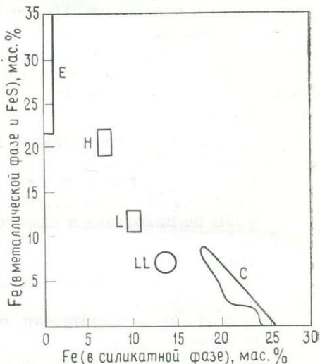
Рис. 1.1. Классификация хондритов по содержанию железа в металлической и сульфидной фазах и окисленного железа в силикатах. Контурами изображены приблизительные поля составов различных групп: E — энстатитовые хондриты; H — высокожелезистые хондриты с высоким содержанием металлической фазы; C — углистые хондриты [211].
