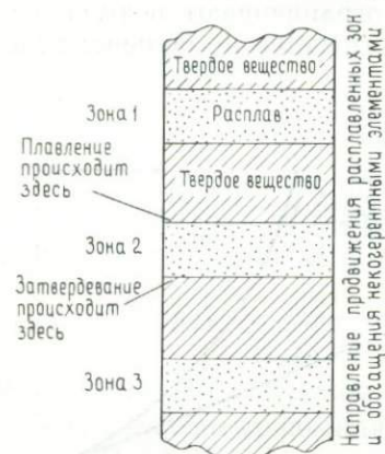
Рис. 8.25. Зонная плавка. Изображены 3 зоны жидкости, продвигающиеся через твердое вещество.
