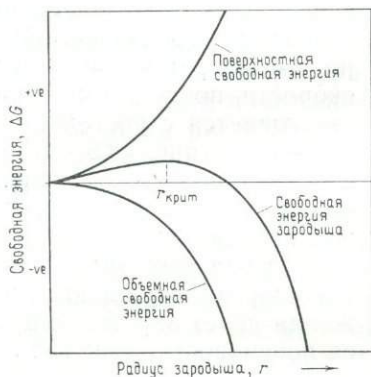
Рис. 8.8. Соотношение между свободной энергией и радиусом кристаллического зародыша. r_{\text{крит}} — критический радиус.
