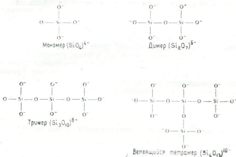
Рис. 6.7. Двумерное представление некоторых возможных полимерных блоков в силикатных расплавах.
