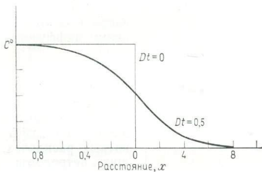
Рис. 8.3. Зависимость концентрации от расстояния для диффузионной пары при Dt=0 и Dt=0,5 .
