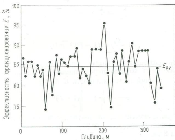
Рис. 8.22. Вариации эффективности фракционирования E с глубиной, рассчитанные по кумуласу. Данные по 350-метровой скважине, прошедшей через часть Скергаардского расслоенного интрузива. Скважина пересекла самую нижнюю обнаженную часть и примерно 200 м погребенной части этого интрузива [176].
