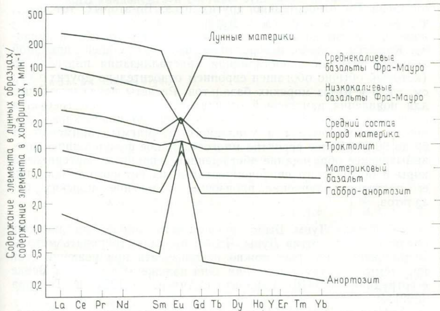
Рис. 3.5. Спектры распространенности редкоземельных элементов в типах материковых пород (нормировано на содержание в хондритах) [392].
