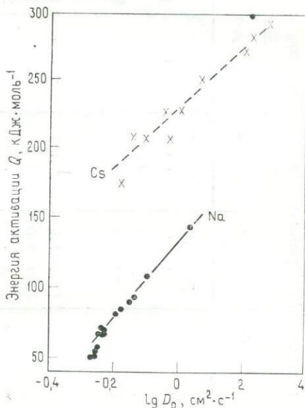
Рис. 8.6. Компенсационные зависимости для диффузии микропримесей натрия и цезия в силикатных матрицах (расплавы и стекла) различного состава [240].
