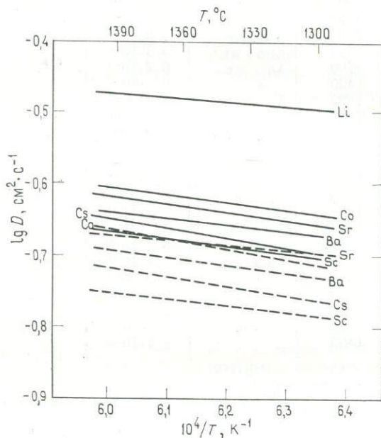
Рис. 8.5. Аррениусовская зависимость для диффузии микропримесей различных катионов в расплаве базальтового состава (сплошные линии) и андезитового состава (штриховые линии) (по данным Лоури и др. [240]).
