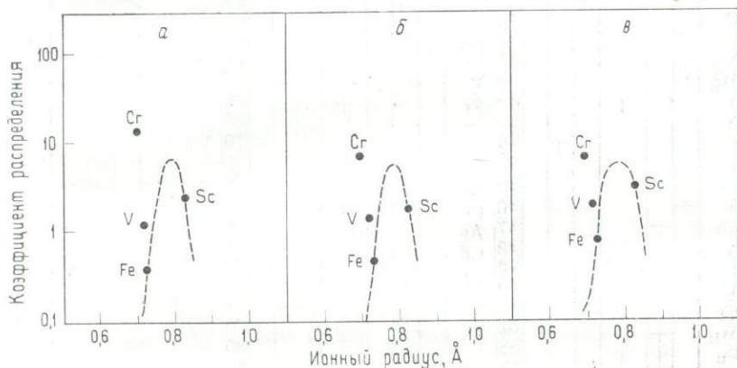
Рис. 6.11. Зависимость коэффициентов распределения ионов Sc^{3+} , V^{3+} , Cr^{3+} и Fe^{3+} между клинопироксенами и основной массой в трех образцах базальтов (а, б и в). Штриховая линия проведена по литературным данным; ее форма и положение пика базируются на кривой, построенной для пары авгит — основная масса [206]. Для облегчения сравнения с рис. 6.10а радиусы даны по данным работы [432]. (Рисунок взят из работы [177].)
