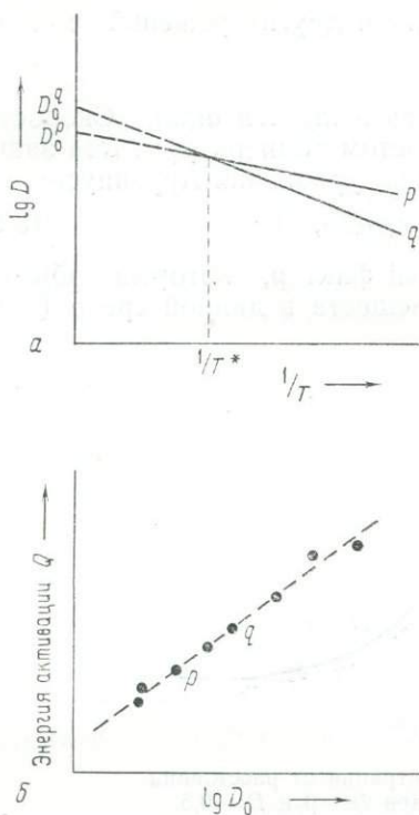
Рис. 8.4. a — схематическая диаграмма аррениусовской зависимости \lg D от обратной температуры ( K^{-1} ) для диффузии двух веществ — p и q — в одной и той же матрице. Температура T^* , при которой линии пересекаются, называется критической температурой (см. текст); b — зависимость между \lg D_0 и энергией активации Q . Экспериментальные точки, в том числе для веществ p и q , образуют «компенсационную линию» (см. также рис. 8.6).
