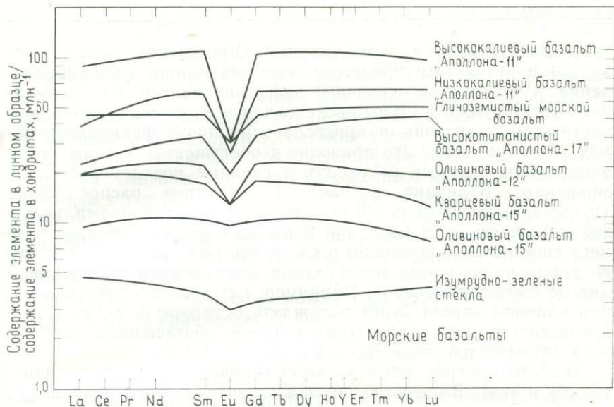
Рис. 3.4. Спектры распространенности элементов в морских базальтах (нормировано на содержание в хондритах) [392].
