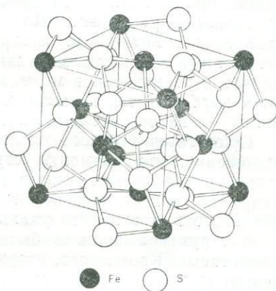
Рис. 6.3. Структура пирита [421].
