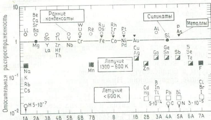
Рис. 4.3. Модельный состав Земли, отнесенный к космической распространенности. Он основан на предположении, что каждый компонент содержит свой «космический» набор микроэлементов. Положение на оси абсцисс дано по группам периодической таблицы элементов [125].
