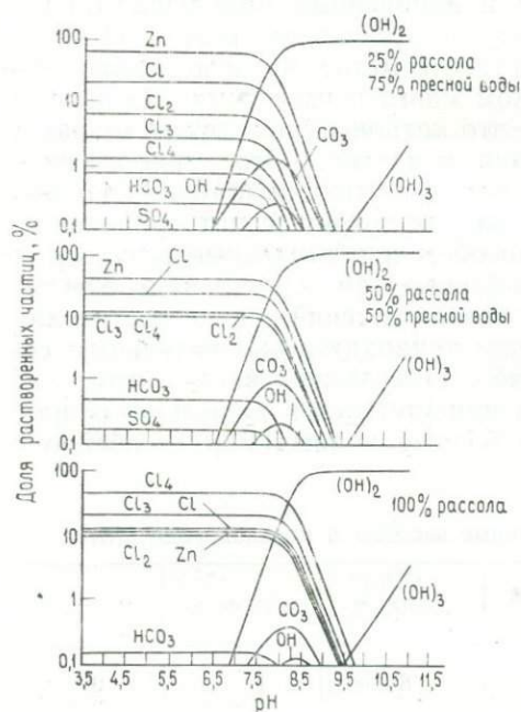
Рис. 11.2. Распределение химических форм нахождения цинка в смесях рассола и пресной воды [236].
