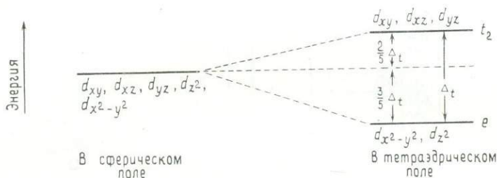
Рис. 6.17. Относительные энергетические уровни d -орбиталей ионов переходных металлов в сферическом и тетраэдрическом координационных полях.
