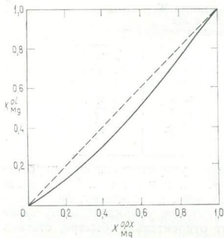
Рис. 7.4. Распределение магния между оливином и ортопироксеном. Сплошная линия — теоретическое распределение при 900 °C, точно совпадающее с экспериментально определенным распределением (непоказанным) [260].
