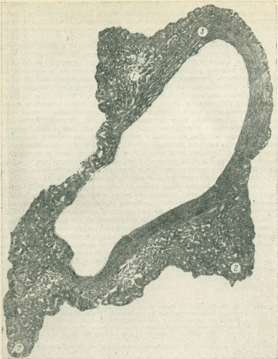
Схема ультратонкого строения ископаемой спородермы рода Archaeoperisaccus Наушова.
