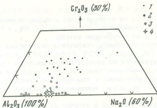
Рис. 35. Составы клинопироксенов ультраосновных включений из щелочных базальтов и базанитов карбонатитовых комплексов в системе Al_2O_3 - Cr_2O_3 - Na_2O
