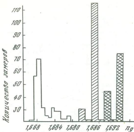
Рис. 26. Гистограмма показателей преломления ортопироксенов ультраосновных включений из кимберлитов Якутии и анальцимовых базальтов Минусинских межгорных впадин
