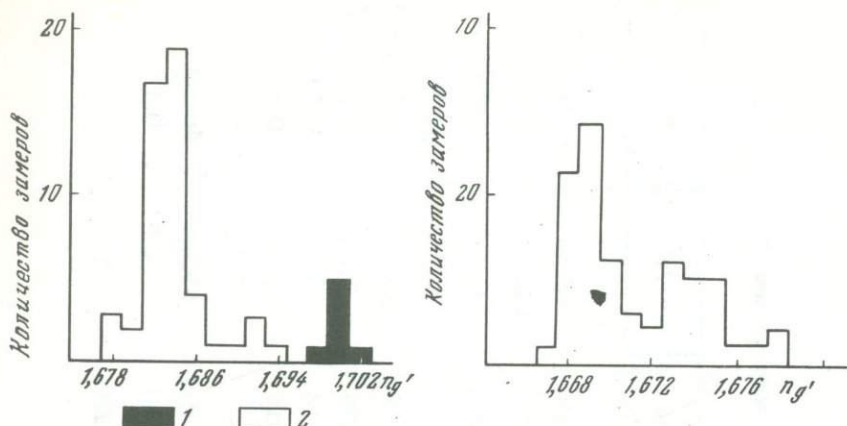
Рис. 1. Гистограмма показателей преломления оливинов из включений ультраосновных пород трубки Мир
