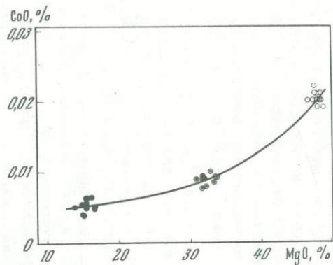
Рис. 17. Соотношение некоторых элементов группы железа и магния в силикатных минералах ультраосновных включений из базальтов Байкальской рифтовой зоны 1 - в оливине; 2 - в ортопироксене; 3 - в клинопироксене
