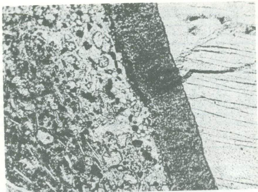
Рис. 18. Замещение ортопироксена тонкозернистым агрегатом оливины (темное) на контакте с базальтом; шлиф без анализатора, увел. 24
