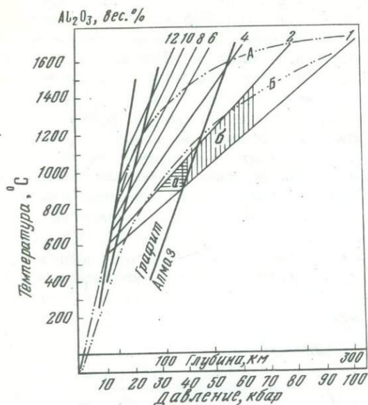
Рис. 15. Соотношение фазовых равновесий в сочетании с геотермами океанических областей (А) и докембрийских щитов (Б). По Ф.Р. Бойду и И.Д. Мак-Грегору (1968)
