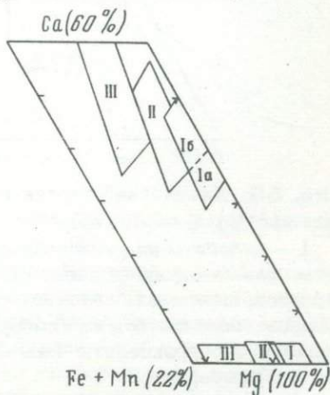
Рис. 55. Составы клино- и ортопироксенов ультраосновных включений в системе (Mg – Ca – (Fe + Mn))
