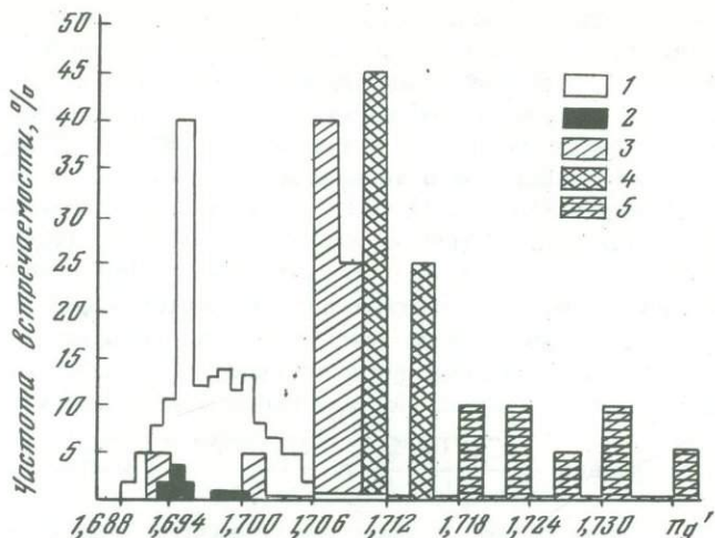
Рис. 25. Гистограмма показателей преломления клинопироксенов ультраосновных включений из кимберлитов и анальцимовых базальтов Минусинских межгорных впадин
