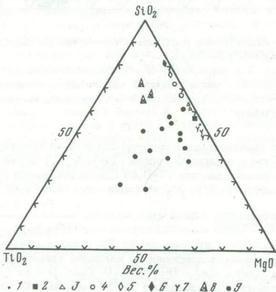
Рис. 10. Положение ильменитовых гипербазитов на диаграмме SiO_2 - MgO - TiO_2 в сравнении с магниезиальными гипербазитами, эклогитами, кимберлитами и лунными образованиями
