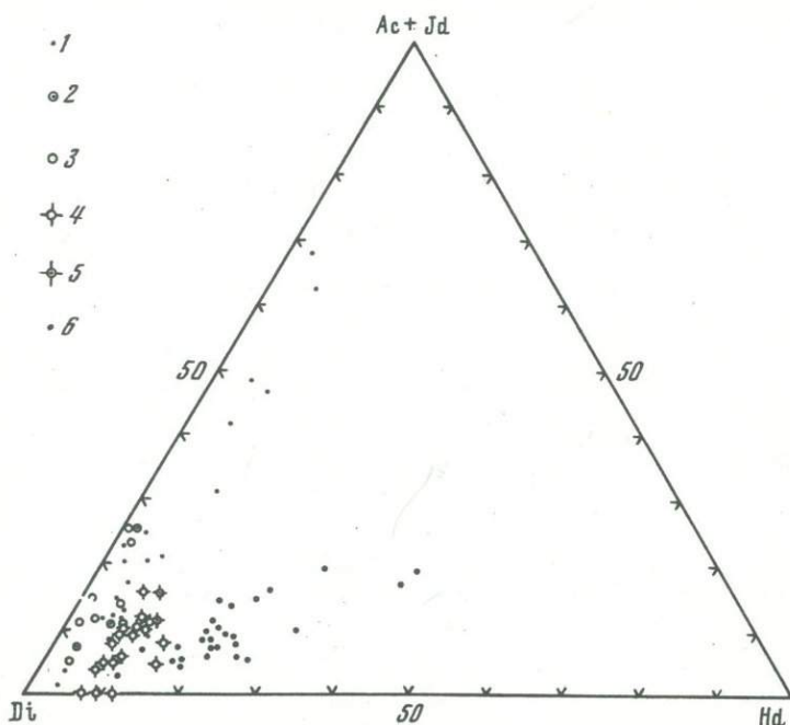
Рис. 32. Составы клинопироксенов из ультраосновных включений в системе \text{Di} - \text{Hd} - (\text{Ac} + \text{Jd})
