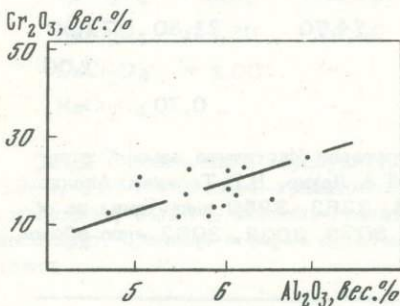
Рис. 43. График зависимости содержаний \text{Cr}_2\text{O}_3 в шпинелях и \text{Al}_2\text{O}_3 в сосуществующих клинопироксенах
