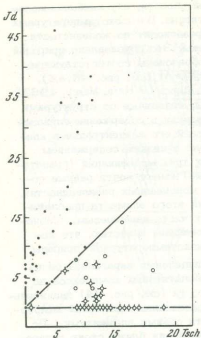
Рис. 46. Диаграмма соотношений Jd/Tsch в клинопироксенах ультраосновных включений
