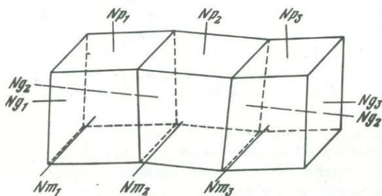
Рис. 19. Схема пластической деформации оливина с образованием блоков при скольжении вдоль (010)
