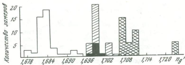
Рис. 27. Гистограмма показателей преломления оливинов ультраосновных включений из кимберлитов Якутии и анальцимовых базальтов Минусинских межгорных впадин
