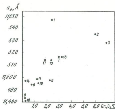
Рис. 6. Зависимость параметра элементарной ячейки ( a_0 ) гранатов из ультраосновных пород от содержания в них \text{Cr}_2\text{O}_3 . Номера точек соответствуют номерам химических анализов гранатов в табл. 16
