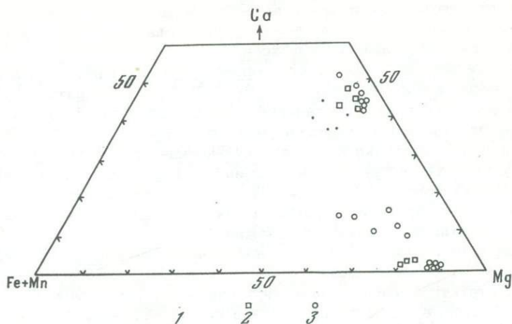
Рис. 23. Составы пироксенов и гранатов из ультраосновных включений Минусинских трубок взрыва в системе Mg - Ca - (Fe + Mn) 1 - вкрапленники; 2 - пироксены из клинопироксенит-верлитовых включений; 3 - пироксены и гранаты из шпинелевых перидотитов и пироксенитов
