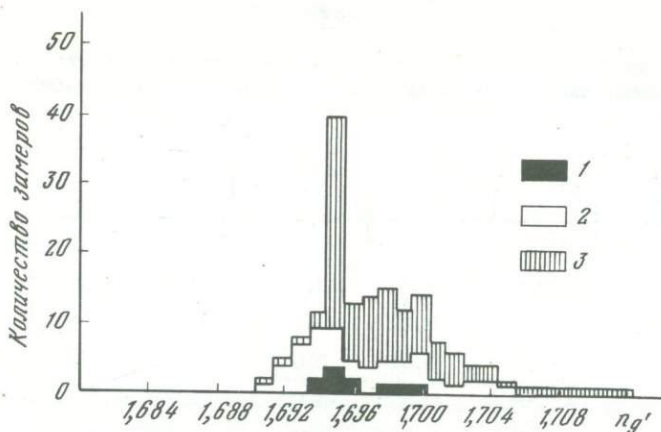
Рис. 3. Гистограмма показателей преломления моноклиновых пироксенов из включений ультраосновных пород и эклогитов в грубке Мир
