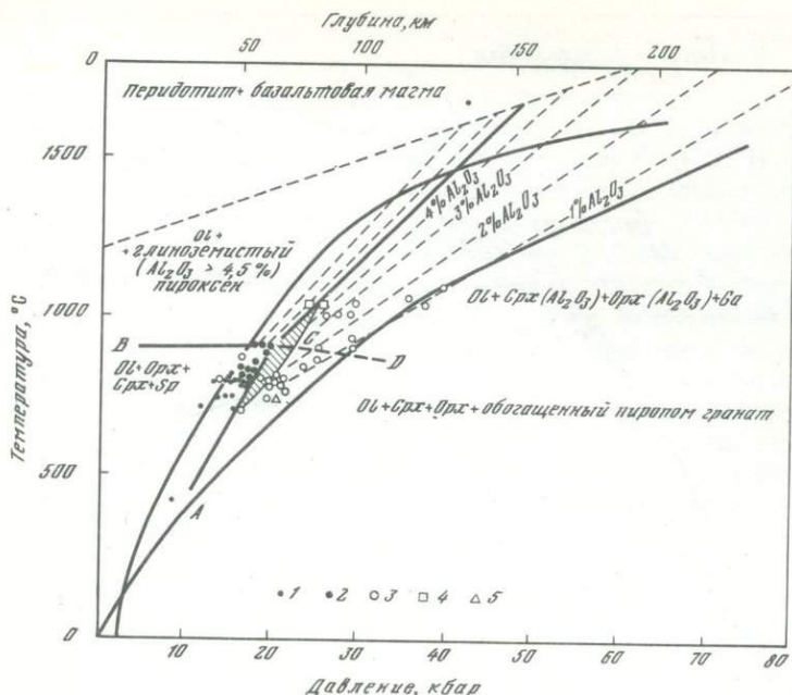
Рис. 53. P-T-диаграмма полей устойчивости минеральных ассоциаций в ультраосновных породах по природным парагенезисам
