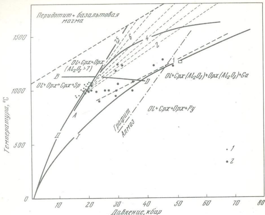
Рис. 54. P-T диаграмма полей устойчивости минеральных ассоциаций в ультраосновных породах по природным парагенезисам
