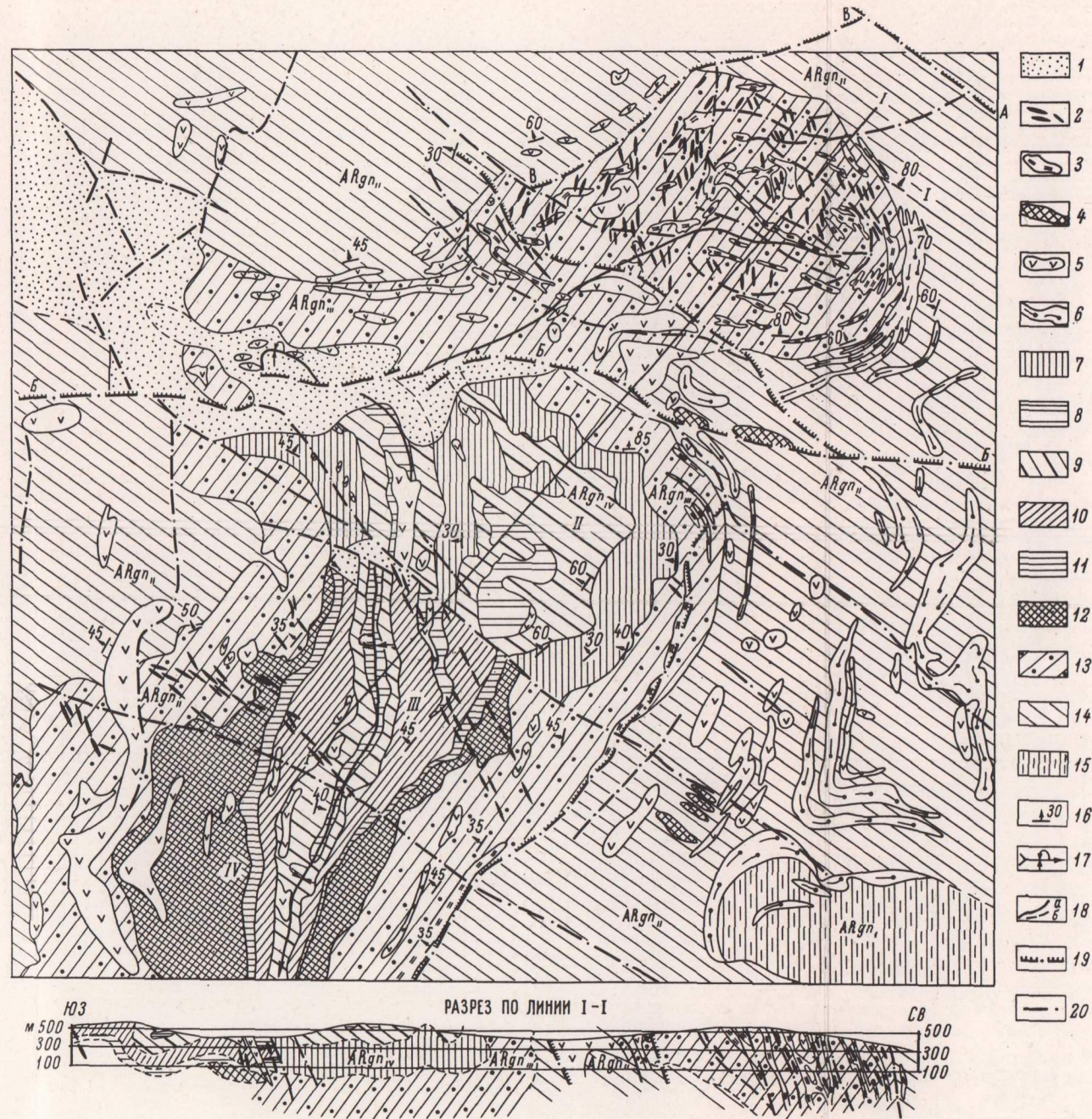
Рис. 1. Сводная геологическая карта района Риколатва—Высокое. Составила В. П. Проскурнина
