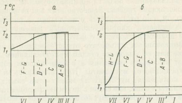
Рис. 4. Различия тепловой истории мусковитовых (а) и занорышевых (б) пегматитов в процессе их формирования.
