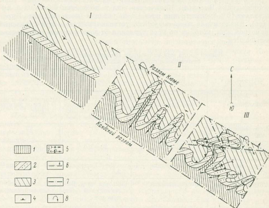
Рис. 2. Схема последовательности тектонического развития Высокогорского блока.
