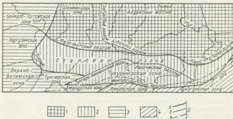
Рис. 1. Схема структурного районирования Олекминской и Джугджуро-Становой складчатых областей. Составил А. Н. Неелов, 1970 г.
