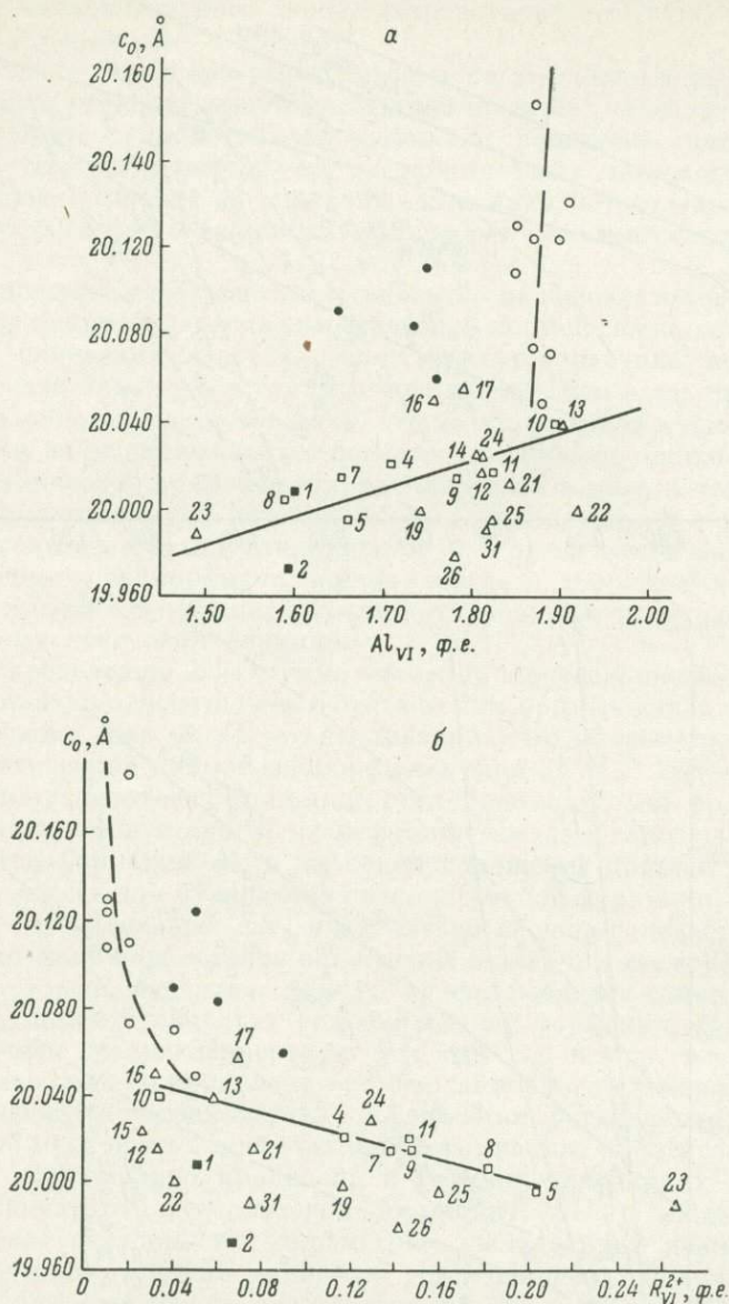
Рис. 5. Зависимость параметра c_0 от содержания Al_{VI} (а) и R_{VI}^{2+} (б) в мусковитах из пегматитов разных формаций.
