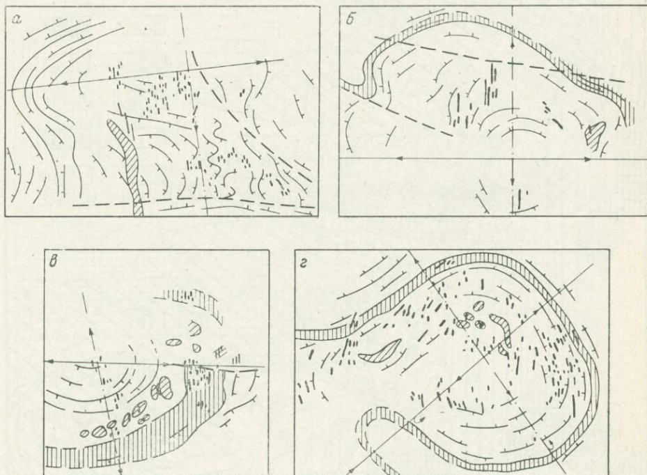
Рис. 2. Пегматитовые месторождения в сводовых структурах.
