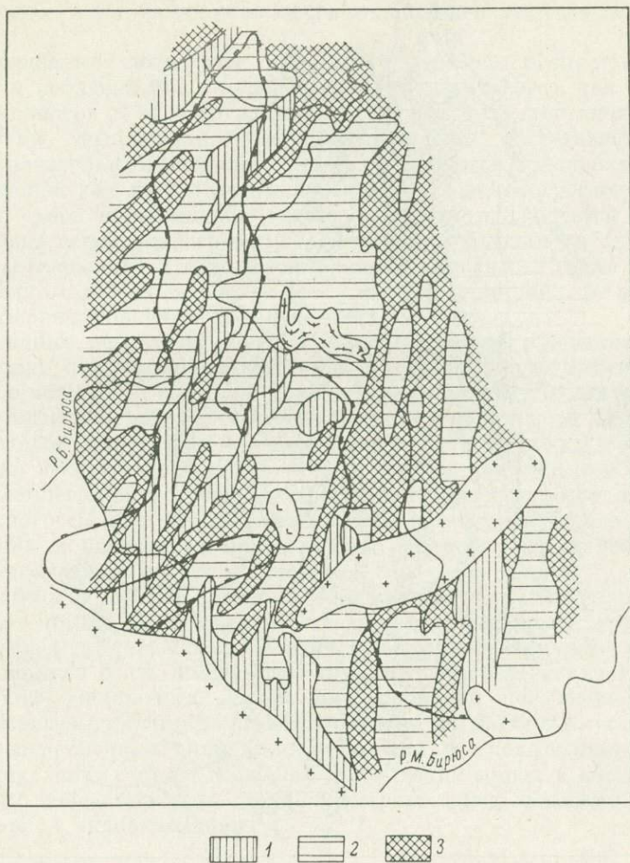
Рис. 3. Схема зональности пегматитовых полей по соотношениям след.
