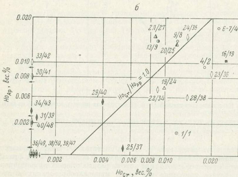
Рис. 6. Распределение Dy (а) и Ho (б) в сосуществующих апатитах и гранатах из пегматитов Карело-Кольского региона.
