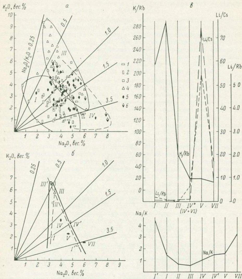
Рис. 2. Изменение состава щелочей и их отношений в главных типах пегматитов мусковитовой, мусковит-редкометальной и редкометальной формаций.
