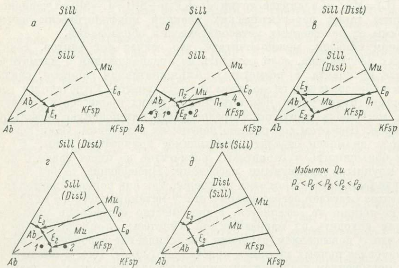
Рис. 2. Принципиальный вид диаграмм плавления для системы силлиманит—альбит—калиевый полевоы шпат (при избытке кварца) для разных давлений.
