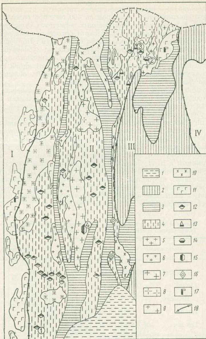
Рис. 1. Схема размещения пегматовых полей Мугоджар. (По: И. Е. Костик).
