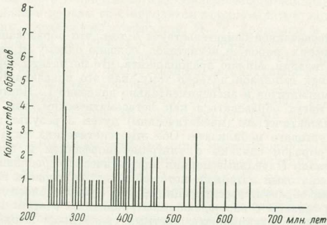
Рис. 2. Сопоставление значений возраста пегматитов Мугоджар.
