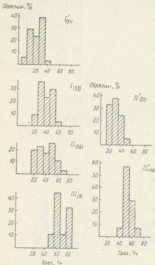
Рис. 7. Распределение Mn в гранатах из пегматитов восточной части Балтийского щита.
