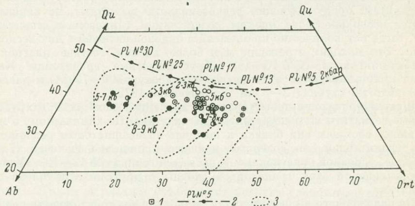
Рис. 2. Составы пегматитоносных гранитоидов на диаграмме Ab—Qu—Ort.
