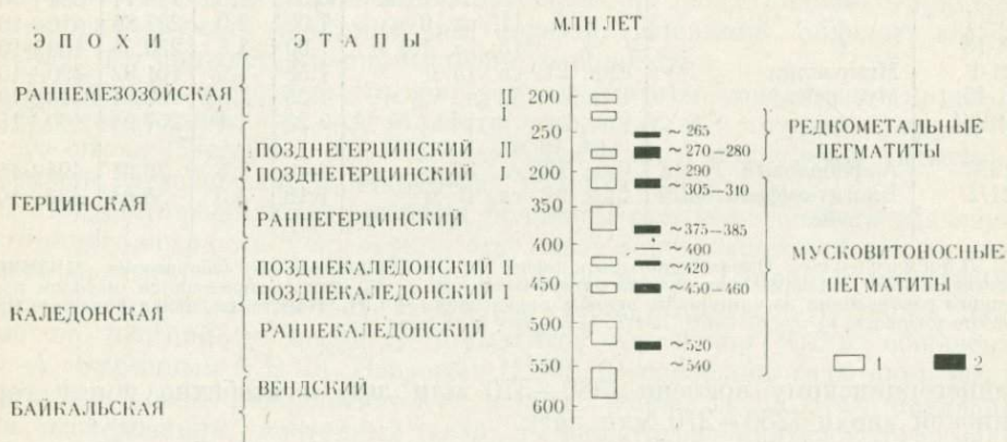
Рис. 3. Сопоставление главнейших этапов тектоно-магматической активности Мугоджар со временем образования пегматитов.
