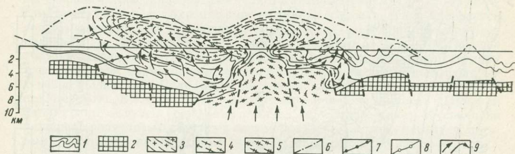
Рис. 2. Принципиальный разрез через Центральный мигматитовый купол.
