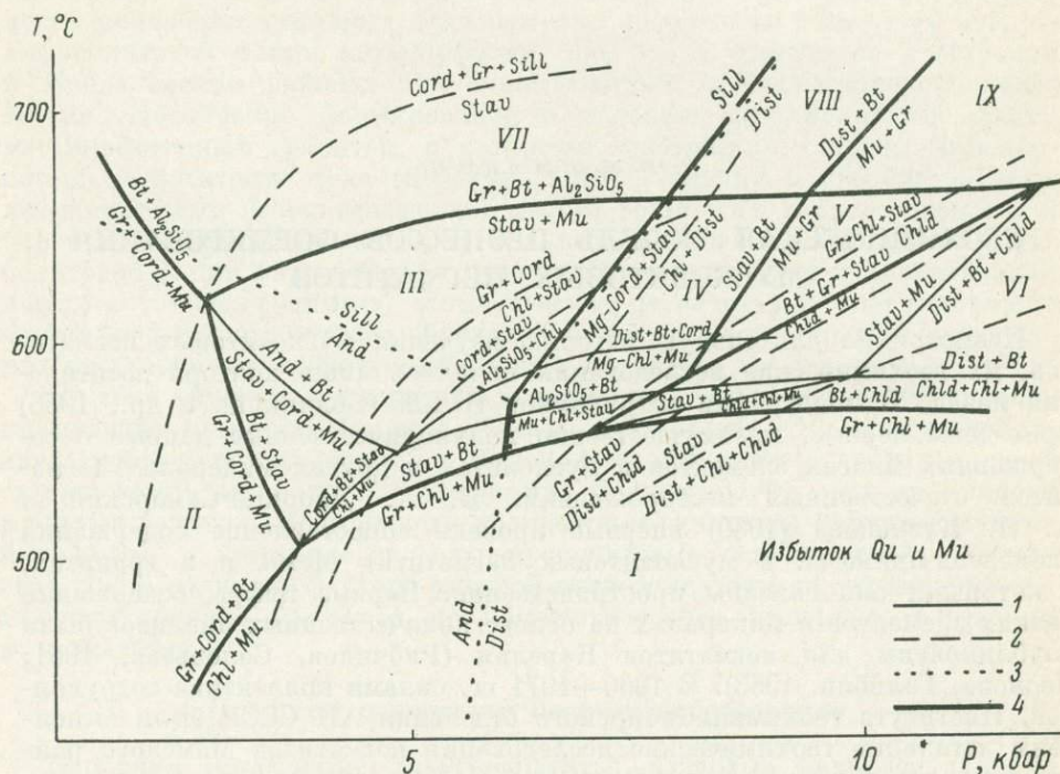
Рис. 3. P - T диаграмма для метапелитов с кварцем и мусковитом.
