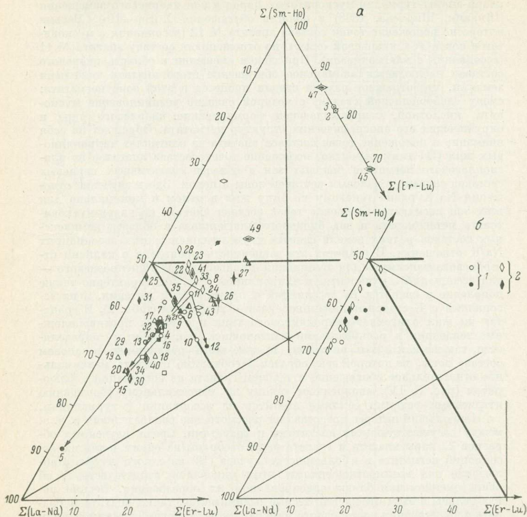
Рис. 2. Состав лантаноидов в апатитах из пегматитов Карело-Кольского региона и Восточной Сибири.
