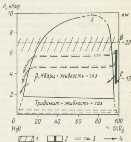
Рис. 1. Составы расплава и паровой фазы водных силикатных систем при P - T условиях солидуса. (Кадик и др., 1971).
