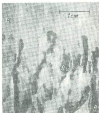
Рис. 1. Соотношение графических и блоковых пегматитов в зональной жиле (а) и в отдельных кристаллах полевого шпата (б, в).
