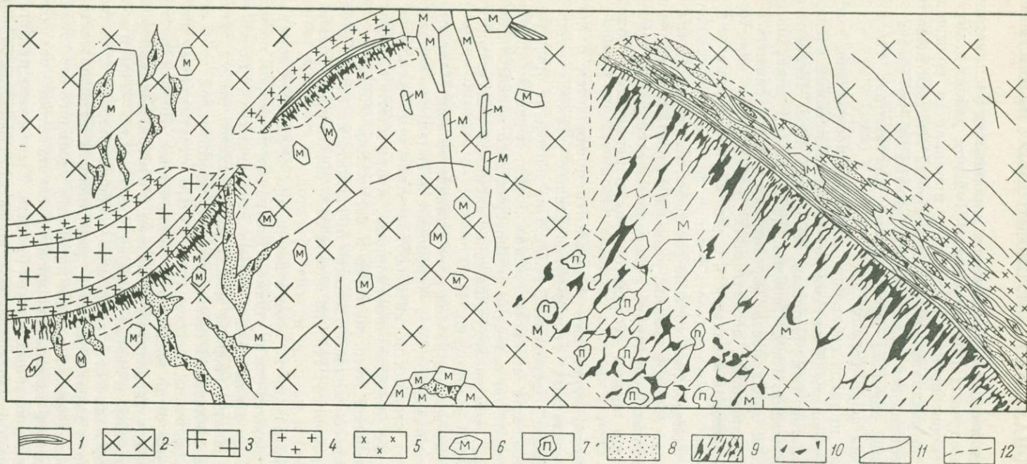
Рис. 1. Унаследование первичной [зональностью] пегматита элементов складчатой структуры метаморфических пород. Жила № 165 гольца Заозерного.
