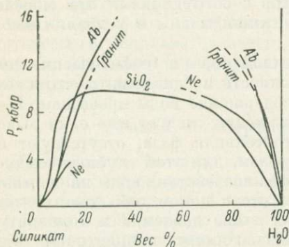
Рис. 1. Составы расплава и паровой фазы водных силикатных систем при P - T условиях солидуса. (Кадик и др., 1971).
