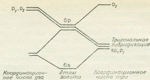
Рис. 1.2. Схема линейной ( sp_x ) и тригональной ( sp_x p_y ) гибридизации для золота (I).
