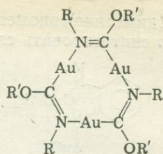
Рис. 7.3. Предполагаемая структура алкокси(алкилимино)метильных комплексов золота (I).
