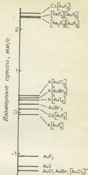
Рис. 10.1. Графическое представление изомерных сдвигов ^{197}\text{Au} для галогенидов и галогенидных комплексов золота (I), золота (III) и золота (V).
