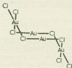
Рис. 2.4. Структура \text{Au}_4\text{Cl}_8 .
