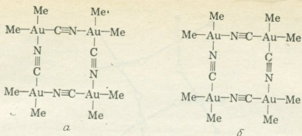
Рис. 7.6. Структура цианида диметилзолота.
