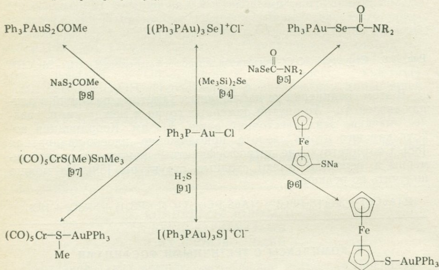
Рис. 3.8. Комплексы золота(I) с лигандами, координированными через серу и селен.
