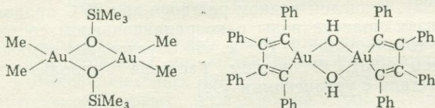
Рис. 7.8. Структуры (\text{Me}_2\text{AuOSiMe}_3)_2 и (\text{Ph}_4\text{C}_4\text{AuOH})_2 .
