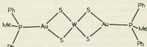
Рис. 3.9. Структура [WS 4 (AuPMePh 2 ) 2 ].
