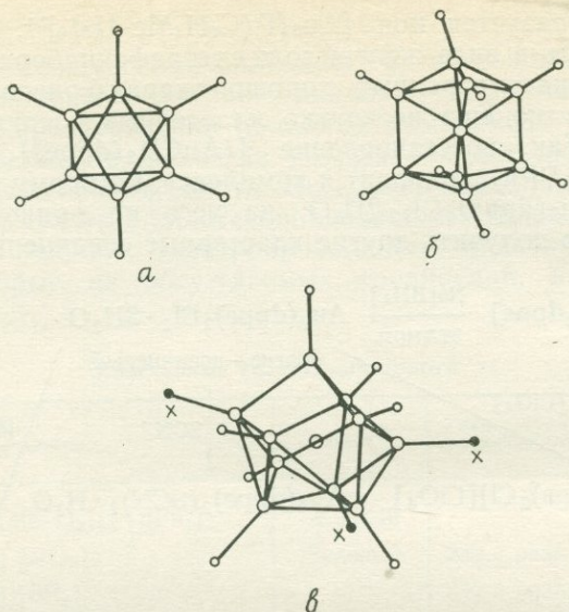
Рис. 8.3. Структура каркасов кластерных комплексов золота.
