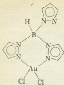
Рис. 5.2. Предполагаемая структура дихлоро(трипиразолилборато)золота (III).
