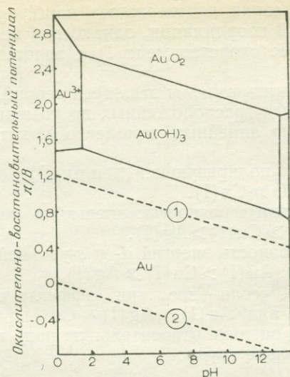
Рис. 1.4. Диаграмма Пурбэкса для системы Au—H 2 O при 25°C. Концентрация всех золотосодержащих частиц 10 -4 М.
