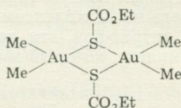
Рис. 7.10. Структуры некоторых диалкил(тиolato)комплексов золота.
