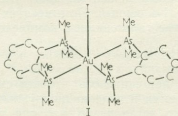
Рис. 5.3. Структура катиона дииодобис[1,2-бис(диметиларсино)бензол]золота (III).
