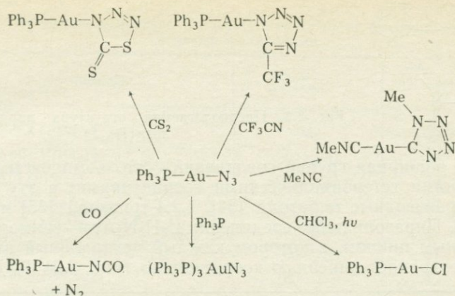
Рис. 3.1. Некоторые реакции азидо(трифенилфосфин)золота(I).
