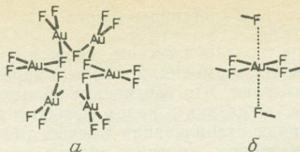
Рис. 2.1. Структура \text{AuF}_3 .
