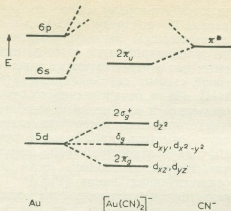
Рис. 10.4. Упрощенная схема уровней энергии молекулярных орбиталей для [\text{Au}(\text{CN})_2]^- .
