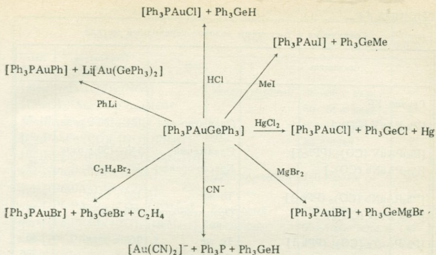
Рис. 8.5. Некоторые реакции трифенилгермил(трифенилфосфин)золота(I).
