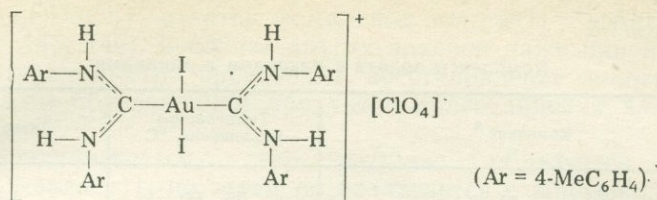
Рис. 7.11. Структура карбенового комплекса золота (III).
