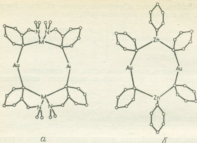
Рис. 7.5. Предполагаемые структуры Ag_4Au_2M_2 (где Ag - 2-Me_2NCH_2C_6H_4 , M - Cu или Li ) (а) и Ph_8Au_2Zn_2 (б).
