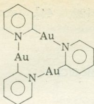
Рис. 7.2. Предполагаемая структура 2-пиридилзолота (I).
