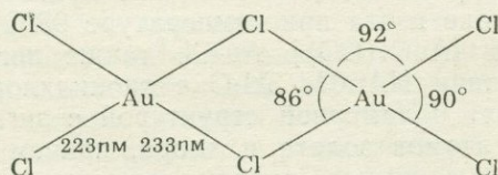
Рис. 2.3. Структура \text{Au}_2\text{Cl}_6 .
