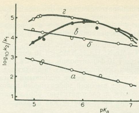
Рис. 9.1. Зависимость относительной реакционной способности от pK_a производных пиридина (am), замещаемых в [AuCl_3(am)] различными входящими группами: a — Cl^- ; b — Br^- ; v — N_3^- ; z — NO_2^- .
