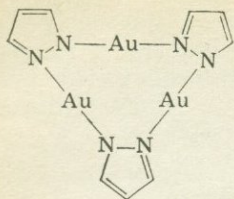
Рис. 3.2. Предполагаемая структура пиразолилзолота (I).
