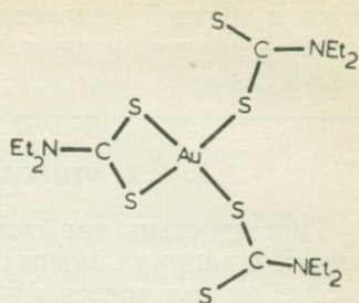
Рис. 5.4. Структура трис(N,N-диэтилдитиокарбамато)золота(III).
