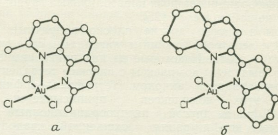
Рис. 5.1. Структура трихлоро(2,9-диметил-1,10-фенантролин)золота(III) (а) и трихлоро(2,2'-дихинолил)золота(III) (б). Кругжками обозначены атомы углерода; атомы водорода не показаны.
