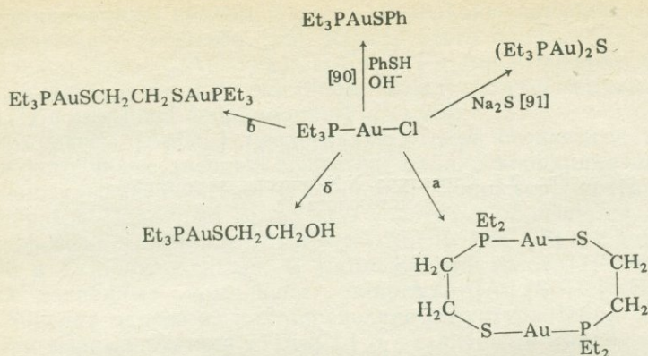
Рис. 3.7. Комплексы золота(I) с лигандами, координированными через тиольные группы [92].
