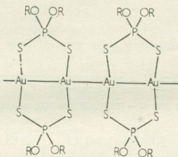
Рис. 3.6. Структура O,O' -дизопропилдитиофосфатозолота (I) ( R = \text{Me}_2\text{CH} ).
