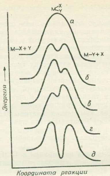
Рис. 9.3. Профили реакций замещения лигандов в плоско-квадратных комплексах.
