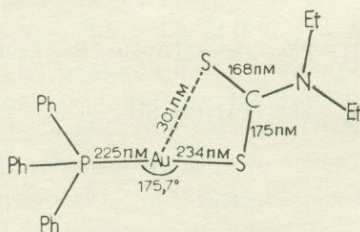
Рис. 3.3. Структура N,N-диэтилдитиокарбамато(трифенилфосфин)золота(I).
