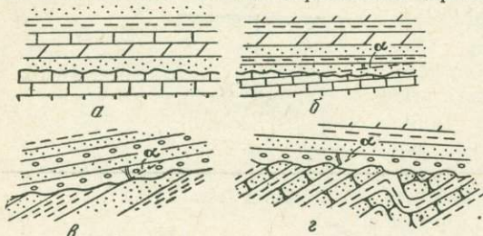
Рис. 8. Примеры различных значений угла несогласия \alpha . Типы несогласий: а — параллельное ( \alpha=0^\circ ), б — географическое ( \alpha < 1^\circ ), в — слабое угловое ( \alpha < 30^\circ ), г — резкое угловое ( \alpha > 30^\circ )
