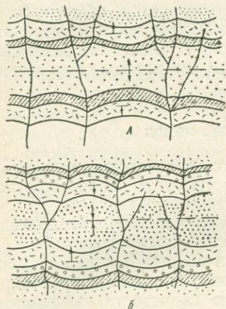
Рис. 28. Дешифрирование антиклинальной (А) и синклиальной (Б) складок по симметричному расположению пород и пластовым треугольникам
