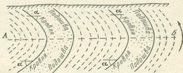
Рис. 5. Нормальное и опрокинутое залегание в вертикальном разрезе Ниже линии АБ слои залегают в нормальном положении (кровля располагается выше подошвы). Выше линии АБ слои опрокинуты (кровля располагается ниже подошвы); \alpha — угол падения слоя
