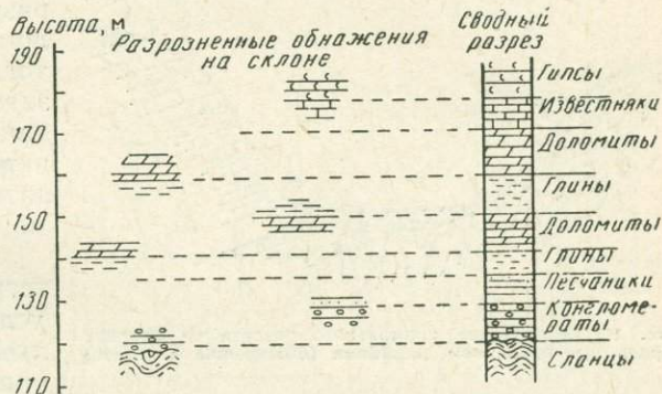
Рис. 10. Составление нормального разреза горизонтально залегающих пород по отдельным разрозненным обнажениям на склоне (объяснение в тексте)
