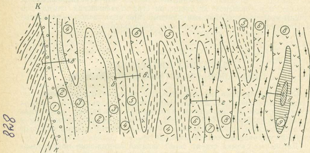
Рис. 12. Схема последовательного описания слоев при составлении стратиграфического разреза в складчатой структуре. План. Цифры — слои от древних к молодым; КК — поверхность несогласия; аб, бв, вг, гд — линии описываемых разрезов
