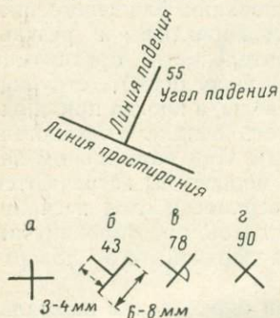
Рис. 4. Условные знаки для изображения элементов залегания: а — горизонтального, б — нормального наклонного, в — опрокинутого, г — вертикального
