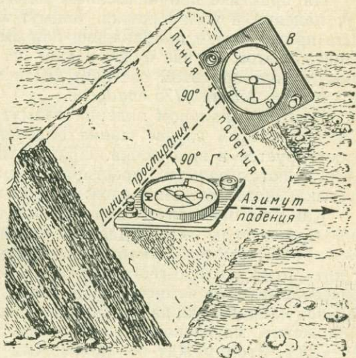
Рис. 3. Измерение горным компасом азимута направления падения ( Г ) и угла падения ( В ). Г — пластинка компаса в горизонтальном положении; В — пластинка компаса в вертикальном положении (угол падения показывает отвес)
