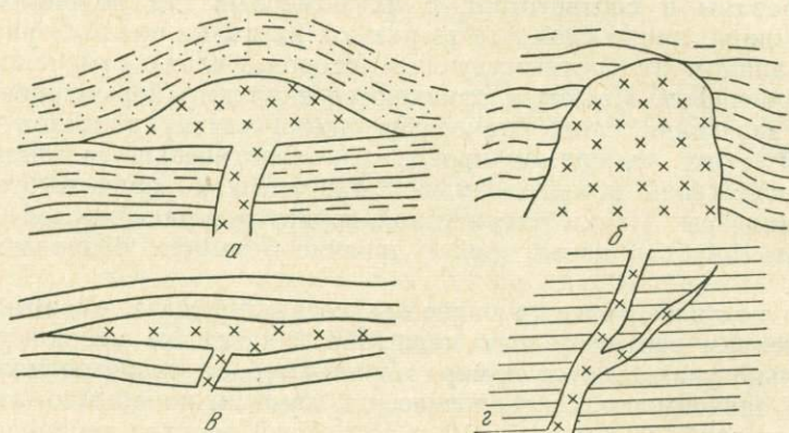
Рис. 17. Подразделение интрузивных тел по форме и характеру соотношений с вмещающими толщами а — лакколлит; б — штоки; в — силл; г — дайка
