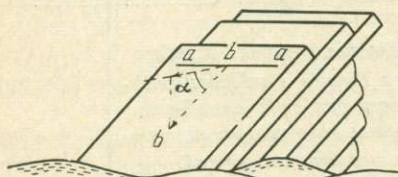
Рис. 2. Элементы залегания: aa — линия простирания; bb — линия падения; α — угол падения
