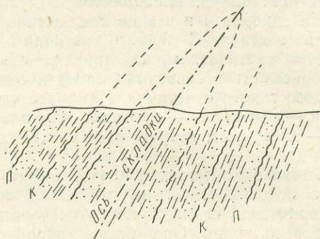
Рис. 14. Положение подошвы (П) и кровли (К) слоев в нормальном (справа) и перевернутом (слева) крыле синклинали
