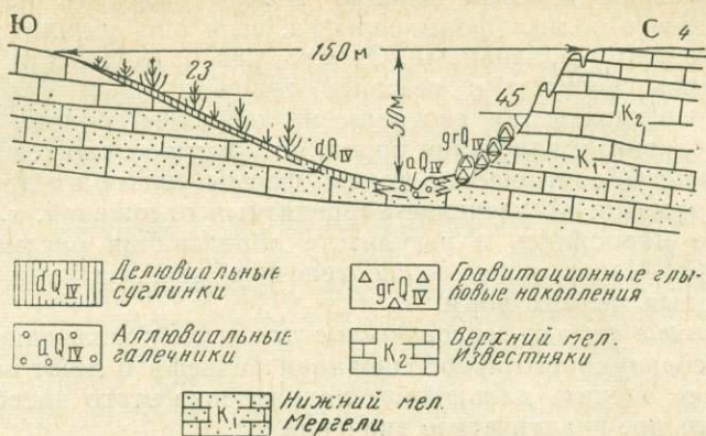
Рис. 22. Пример зарисовки асимметричного поперечного профиля долины продольного типа
