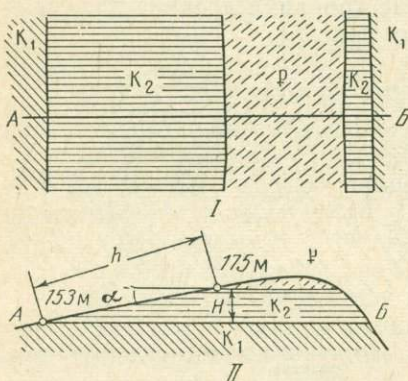
Рис. 6. Зависимость ширины выхода горизонтально залегающих слоев от рельефа и определение истинной мощности при горизонтальном залегании
