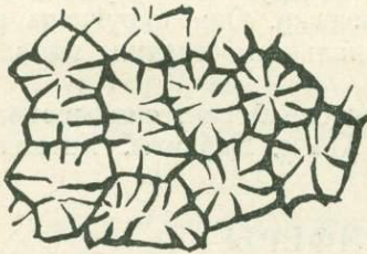
Рис. 34. Цериондная, или сотовидная, колония коралловых полипов
