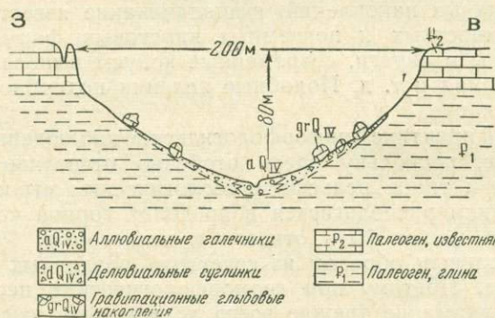
Рис. 23. Пример зарисовки симметричного поперечного профиля долины поперечного типа
