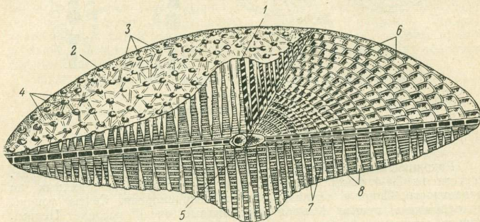
Рис. 33. Схема строения раковины Discocyclus
