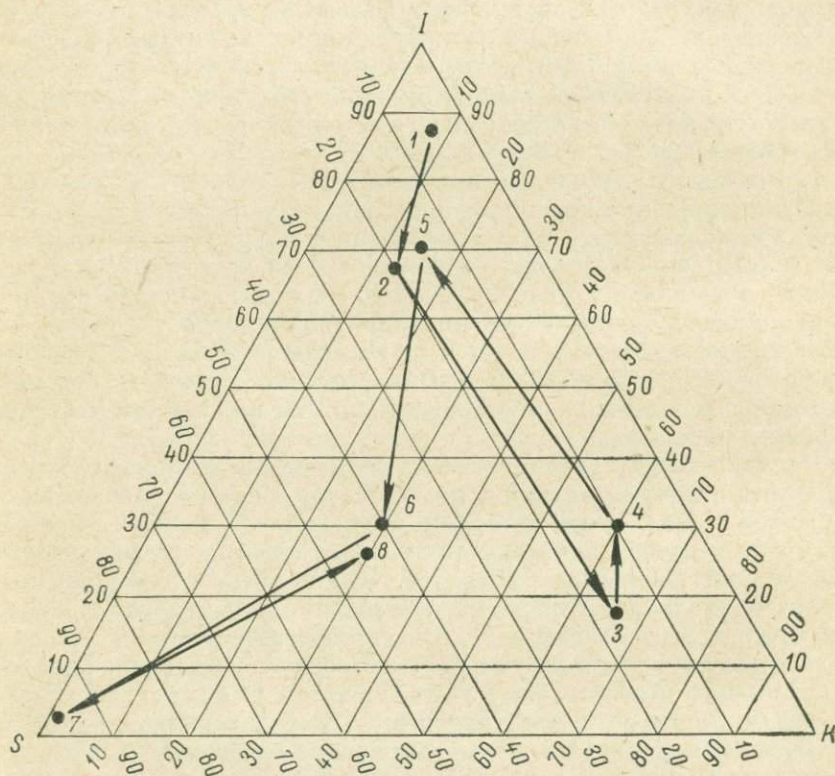
Рис. 1. Изменчивость среднего состава глинистого вещества осадочных отложений района Негева [364].
