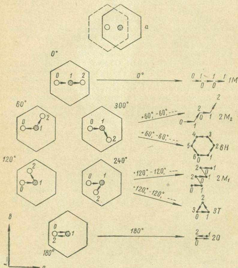
Рис. 3. Полиморфизм мусковита [500].
