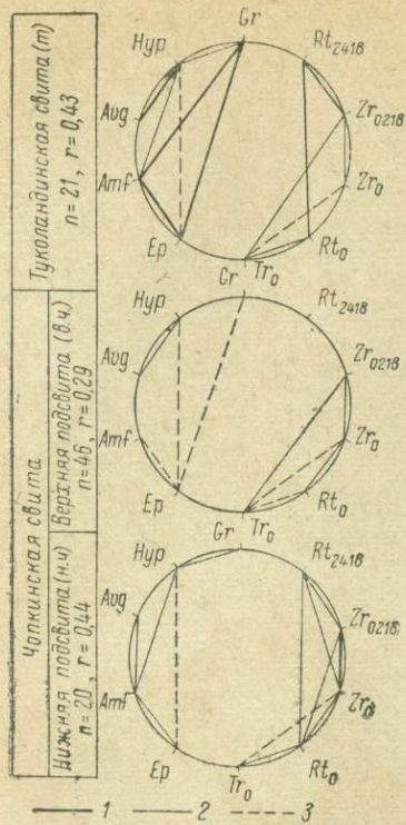
Рис. 5. Корреляционные связи минералов тяжелой фракции мергелей и глинистых известняков верхнекембрийских отложений, развитых на р. Чонко (бассейн р. Енисей).
