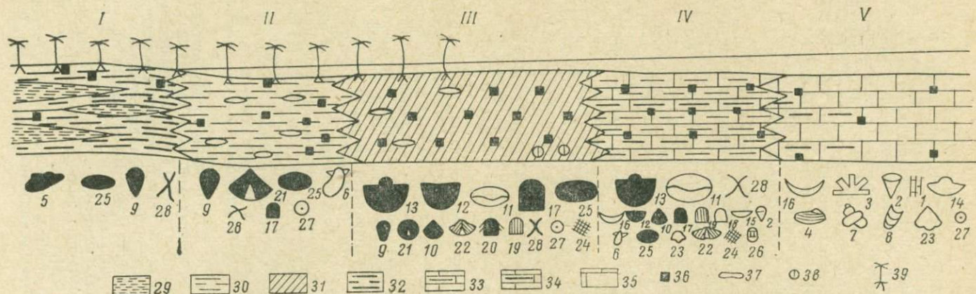
Рис. 28. Смена осадков и связанных с ними комплексов организмов в тульском бассейне Московской синеклизы. I—II — осадки эстуария и лагуны; III — осадки залива; IV — осадки близкой к берегу и тиховодной зоны моря; V — осадки более удаленной от берега зоны моря.
