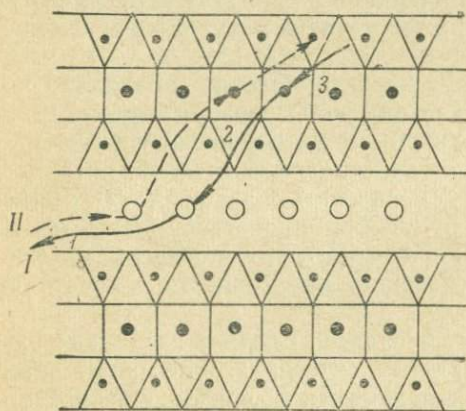
Рис. 4. Прогрессивная деградация (I) и миграция (II) трехслойного глинистого минерала [461].
