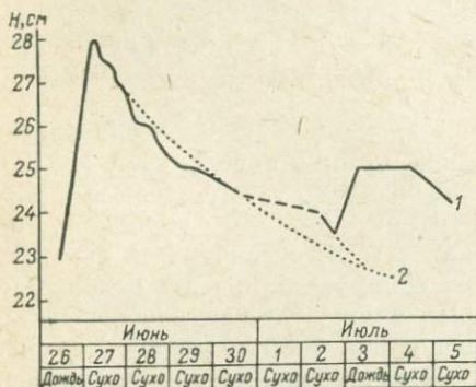
Рис. VI-1. Определение ожидаемой действительной скорости потока по кривой спада уровня подземных вод на хр. Мяо-Чан.
