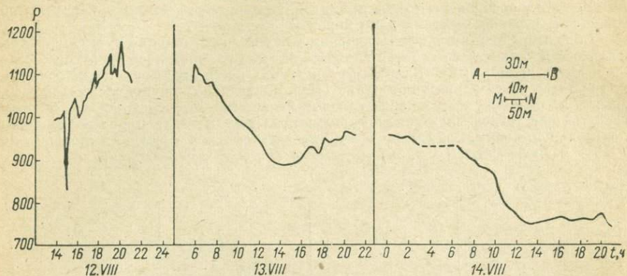
Рис. VI-3. Наблюдение за соевым ореолом с помощью ВЭЗ, хр. Мяо-Чан, 1965 г.
