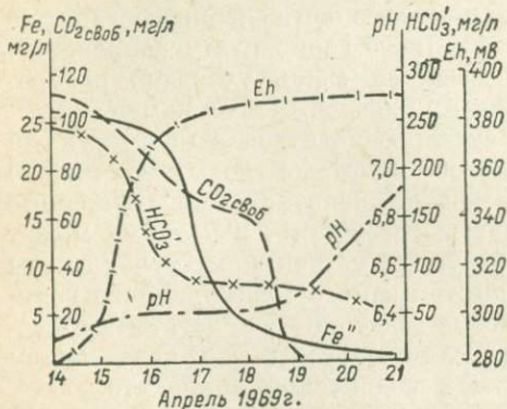
Рис. V-9. Изменение во времени рН, Eh и содержаний Fe ++ , HCO 3 ' , CO 2 свобод в воде скважины Полостровского завода минеральных вод при ее окислении кислородом воздуха.
