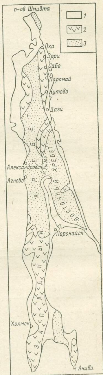
Рис. II-6. Схема зонального распределения хлоридных и гидрокарбонатных грунтовых вод о. Сахалина [Архангельский, 1959а].
