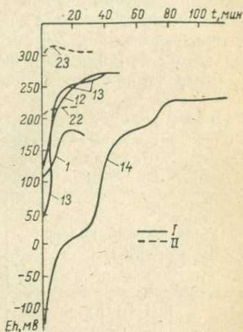
Рис. V-8. Изменение окислительно-восстановительного потенциала старорусских и хиловских минеральных вод и поверхностных вод района кислородом воздуха. I — подземные воды; II — поверхностные воды; цифры на графике — номера проб воды.
