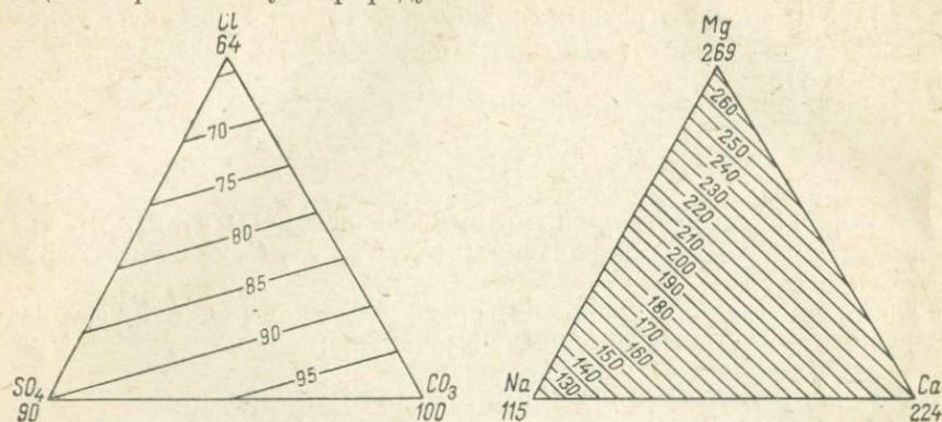
Рис. VII-1. Номограмма для расчетов среднего удельного EK анионов и катионов (ккал/г-эке).
