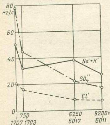
Рис. II-5. Изменение содержания Na + +K + , SO 4 2- , Cl - в пробах поверхностных вод на разном удалении от моря в районе Новороссийска [Колодяжная, 1965].
