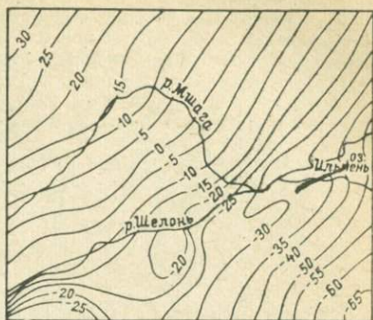
Рис. III-7. Структурная карта кровли старооскольско-швентойского комплекса в низовье р. Шелони (по А. И. Шмаенку).
