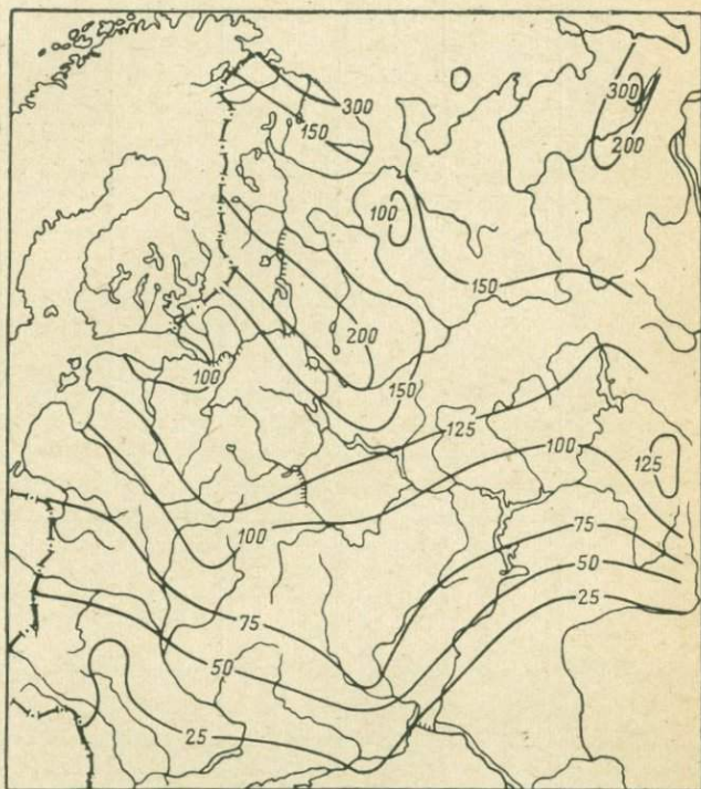
Рис. II-2. Схематическая карта слоя стока вод склонового происхождения (мм) для европейской части СССР [Скальский, 1966].
