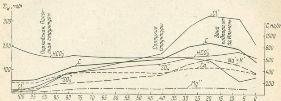
Рис. III-11. Гидрохимический профиль по р. Шелони на 7 августа 1964 г. Составил А. И. Коротков.
