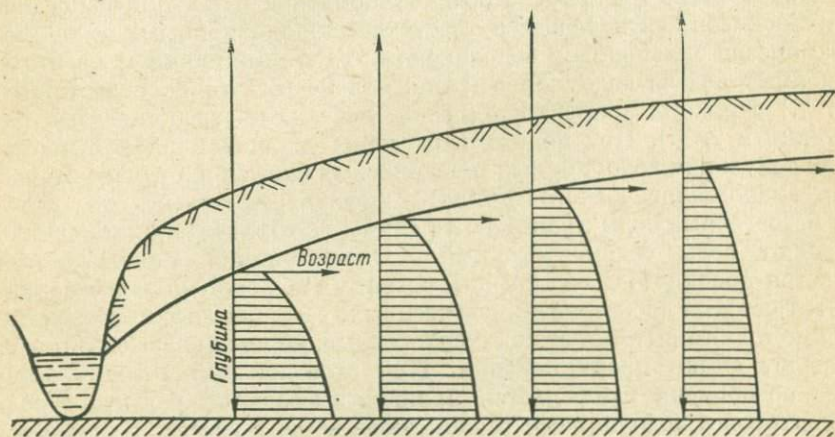
Рис. IV-1. Схема возрастной дифференциации в грунтовом потоке.
