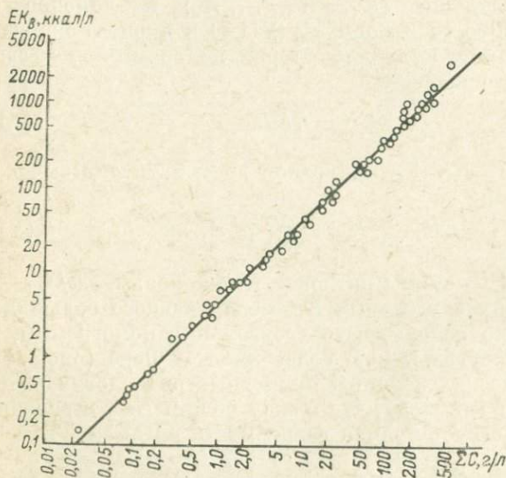
Рис. VII-2. Зависимость общего EK воды от минерализации.
