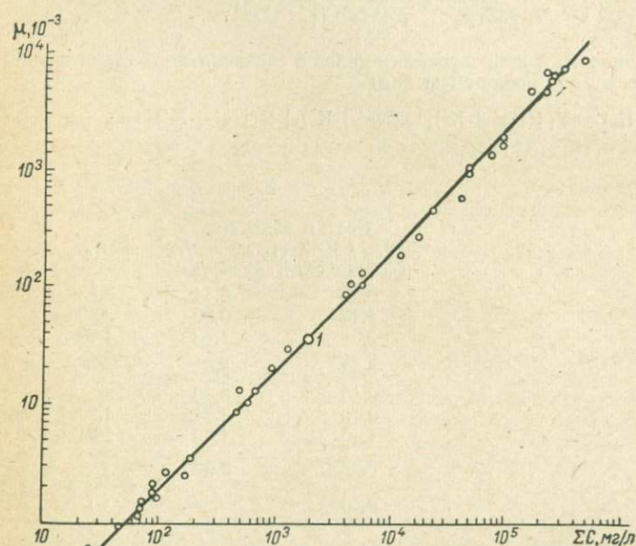
Рис. V-5. Региональная зависимость удельной минерализации природных вод \mu от общей минерализации \Sigma C .
