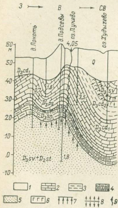
Рис. III-9. Характер засоления и разгрузки подземных вод в районе Локоть-Подсевского поднятия [Коротков, Селадына, 1968].
