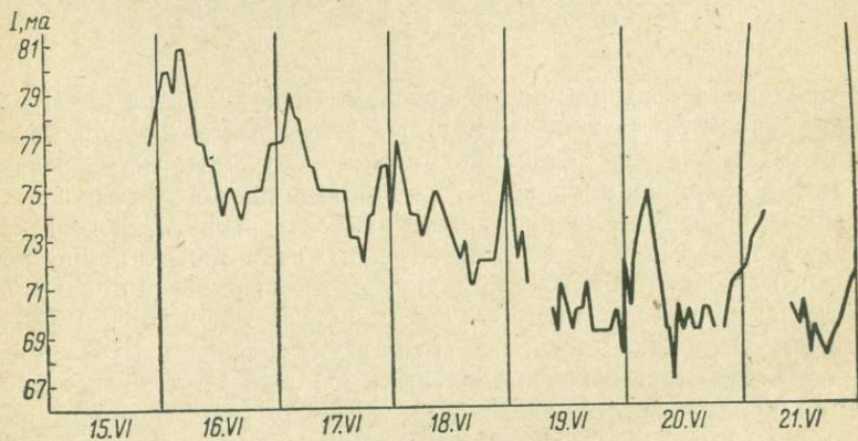
Рис. VI-4. Наблюдение за разубоживанием электролита по изменению силы тока в цепи обсадная труба — вода — электрод.
