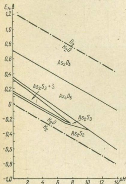
Рис. V-11. Диаграммы полей устойчивости реальгара и аурипигмента.
