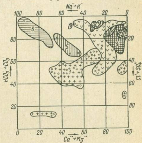
Рис. III-4. График-квадрат Н. И. Толстихина для подземных вод средней части Памбацкого хребта в Армении [Долуханова, 1956].
