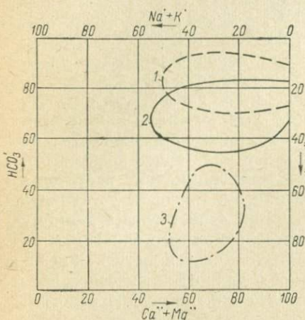
Рис. III-3. График-квадрат Н. И. Толстихина для подземных вод второй гряды Крымских гор (район Куйбышево — Голубинка).
