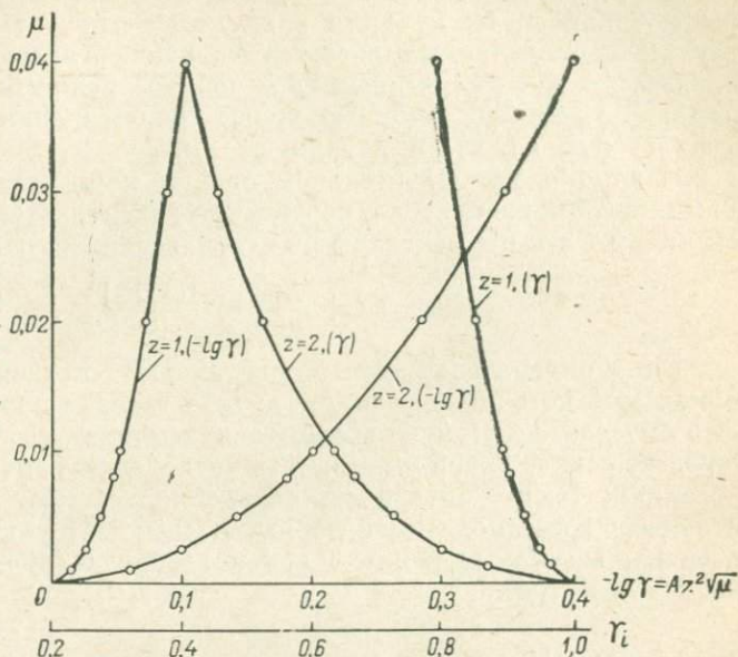
Рис. V-6. Зависимость коэффициента активности одно- и двухвалентных ионов от ионной силы раствора (для ориентировочных расчетов при t = 15^\circ \text{C} ).
