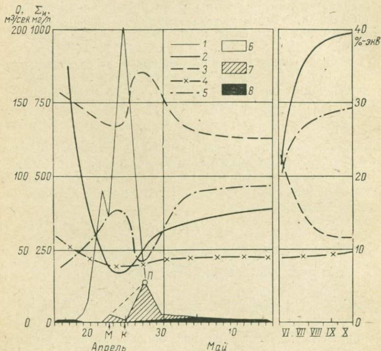
Рис. 11-1. Схема выделения генетических категорий вод местного стока путем расчленения гидрографа, 1955 г. [Воронков, 1963а].
