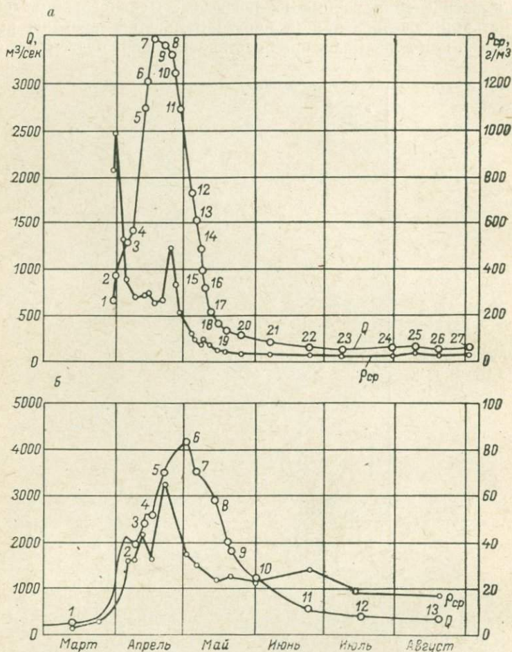
Рис. 11-3. Изменение мутности \rho и расходов воды Q рек Дона (а) и Волги (б) [Лопатин, 1952].
