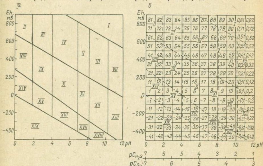
Рис. 1-1. Разделение диаграммы Eh — pH на геохимические группы (а) и классы (б) природных вод.
