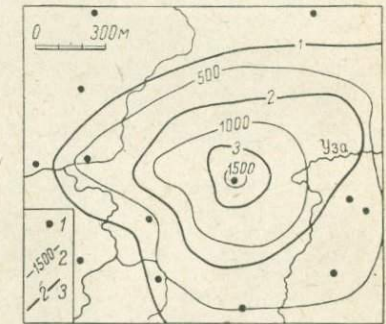
Рис. III-10. Характер распределения минерализации воды в псковско-чудовских известняках в районе Локоть-Подсевской структуры (по В. В. Селадыной, 1964 г.).
