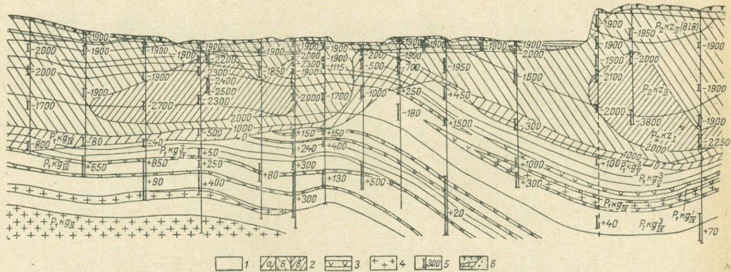
Рис. III-1. Профиль насыщенности сульфатом кальция подземных вод долины р. Камы в районе г. Соликамска [Зверев, 1967].
