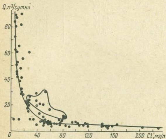
Рис. VI-8. Характер зависимости содержания хлор-иона от расхода воды в р. Шелони (по данным за 1946—1956 гг.). Обведены точки, характеризующие осенние паводки.
