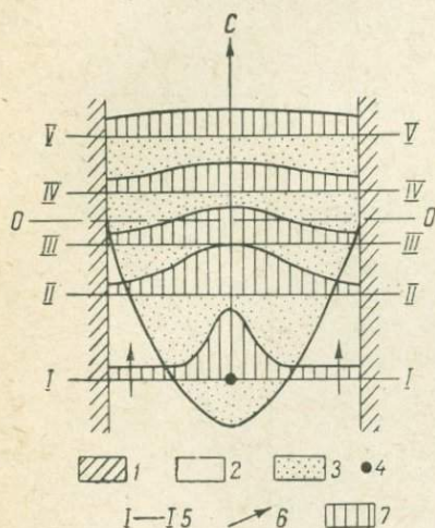
Рис. VI-6. Схема смешения при точечном внедрении вод одного состава ( C_2 ) в горизонт с водами другого состава ( C_1 ) (плановый поток).
