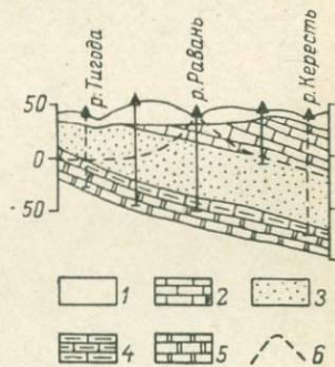
Рис. III-13. Характер залегания гидрохимической зоны солоноватых вод в нижнем течении р. Равани [Коротков, Саванин, 1965].
