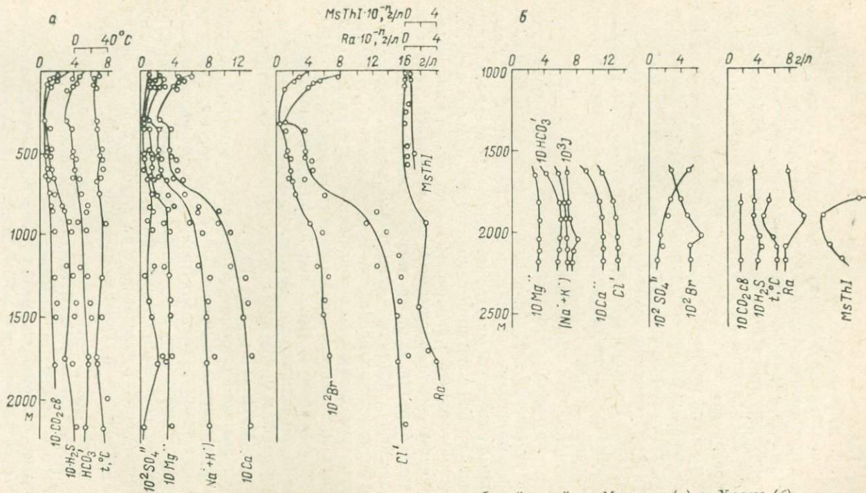
Рис. IV-2. Изменение химического состава вод с глубиной в районе Маесты (а) и Хосты (б).
