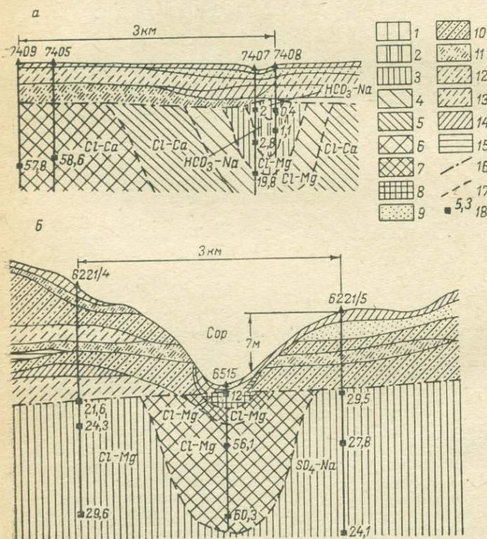
Рис. III-14. Гидрохимическая зональность грунтовых вод под дюнами (а) и сорами (б) [Самарина, 1963].
