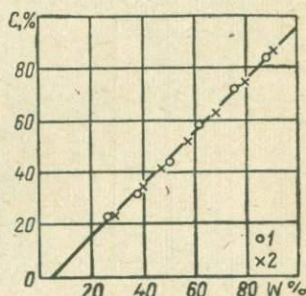
Рис. V-2. Связь гравитационного выноса солей с процессом дегидратации. 1, 2 — первый и второй эксперименты.
