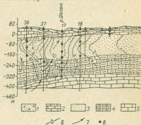
Рис. III-8. Распределение минерализации подземных вод старооскольско-швентойского водоносного комплекса в низовье р. Шелони (в разрезе).
