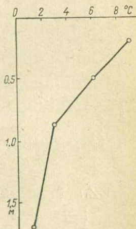
Рис. VI-5. Изменение максимальной суточной амплитуды температуры по глубине.
