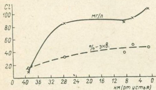
Рис. III-12. Изменение содержания хлоридов в воде р. Равани от верховьев к устью [Коротков, 1963а].
