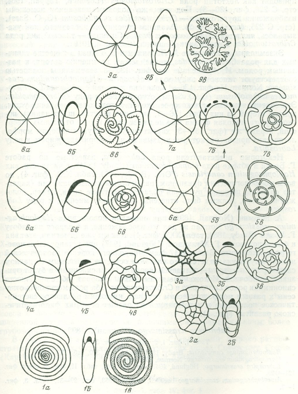
Рис. 1. Предполагаемые генетические связи некоторых представителей отряда Амфидисцида (на рисунке пропущена стрелка между фигурами 1в и 2а)
