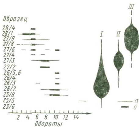
Р и с . 4. Схематическое изображение характера появления по две спиральные септулы второго порядка в раковинах лепидолин с булабовидными септулами (выборки распределяются снизу вверх по разрезу)
