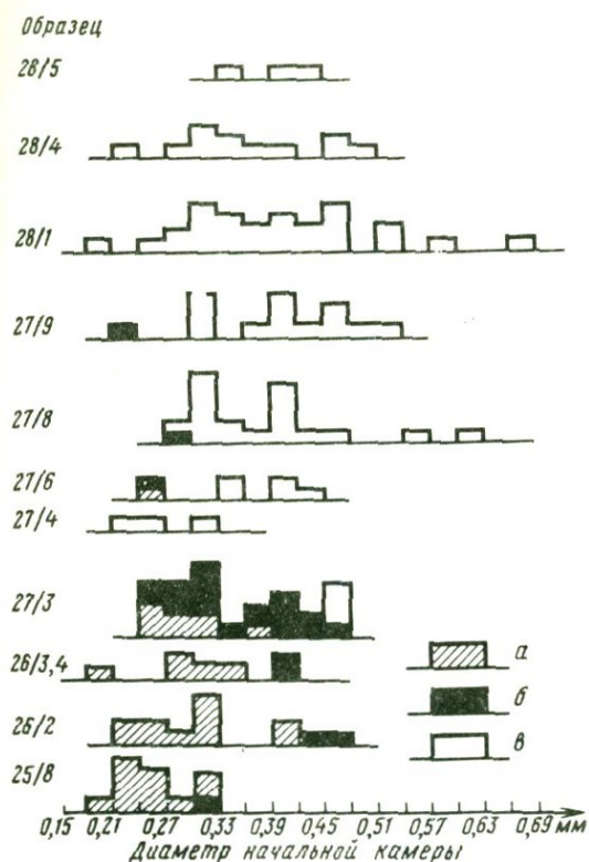
Р и с . 6. Гистограммы диаметров начальных камер Условные обозначения см. на рис. 5
