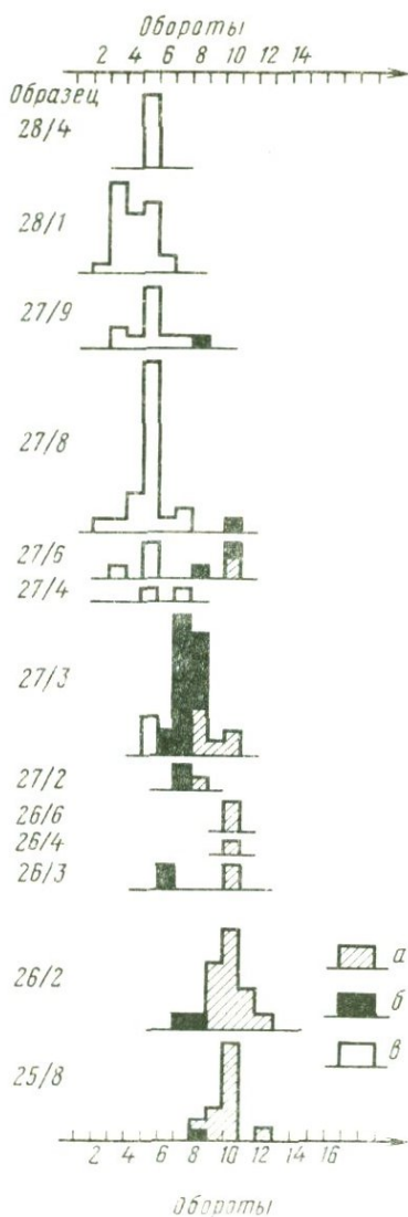
Р и с . 4. Схематическое изображение характера появления по две спиральные септулы второго порядка в раковинах лепидолин с булабовидными септулами (выборки распределяются снизу вверх по разрезу)
