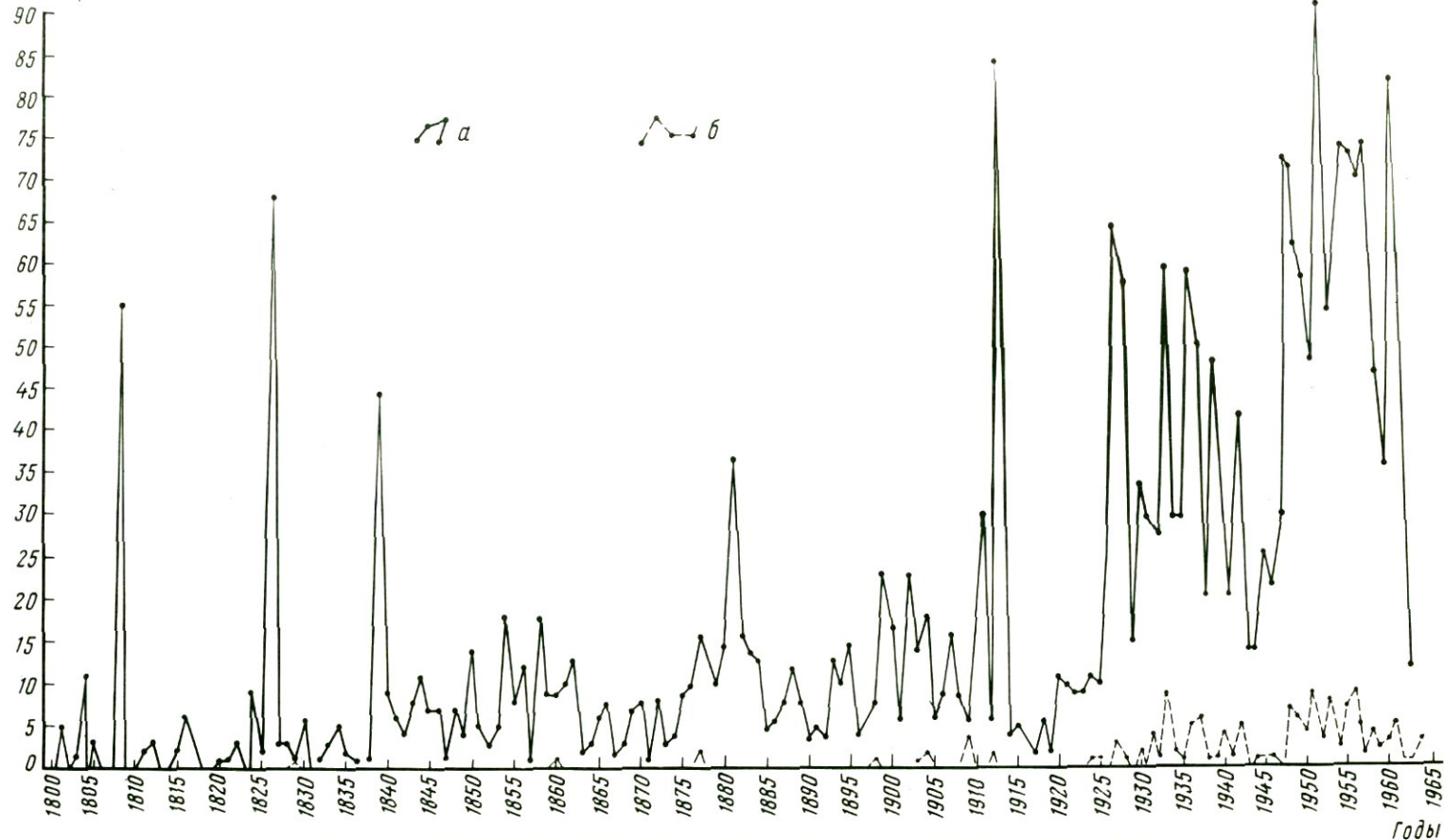
Р и с. 2. Распределение по годам вновь описанных таксонов фораминифер родового ранга а – численность всех фораминифер; б – то же, для Fusulinida
