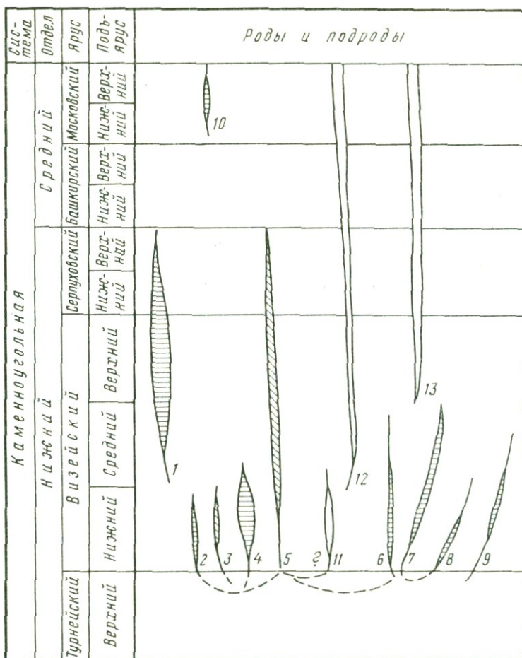
Рис. 2. Схема распространения генетически близких родов и подродов семейства Endothyranopsisidae и его предполагаемых потомков
