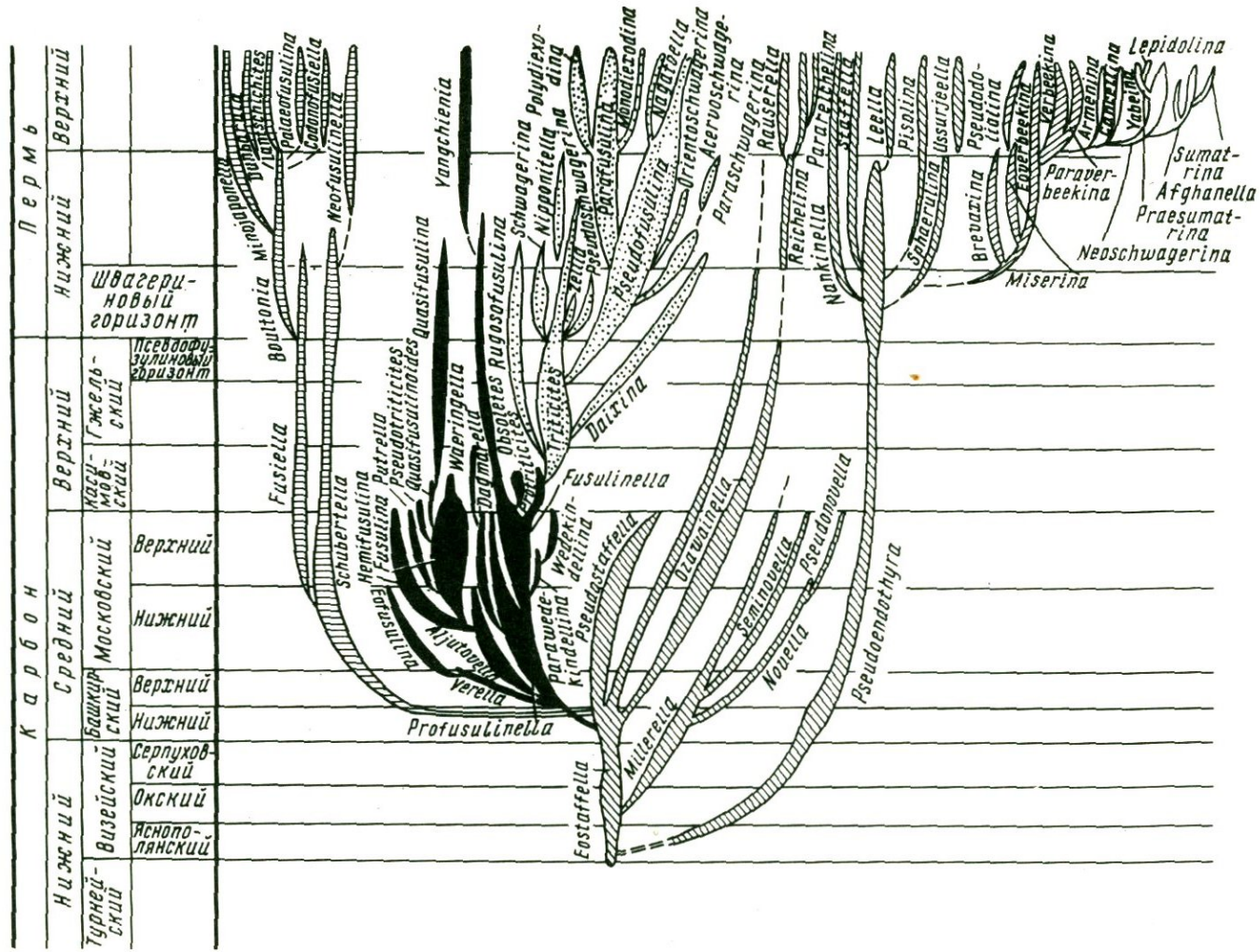
Р и с . 4. Схема филогенетического развития фузулинид по А.Д. Миклухо-Маклау, Д.М. Раузер-Черноусовой, С.Е. Розовской (1958)
