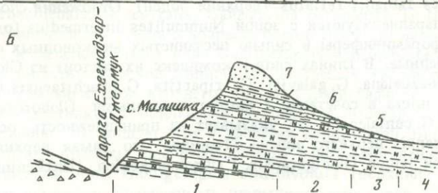
Рис. 16. Разрез Малишка
