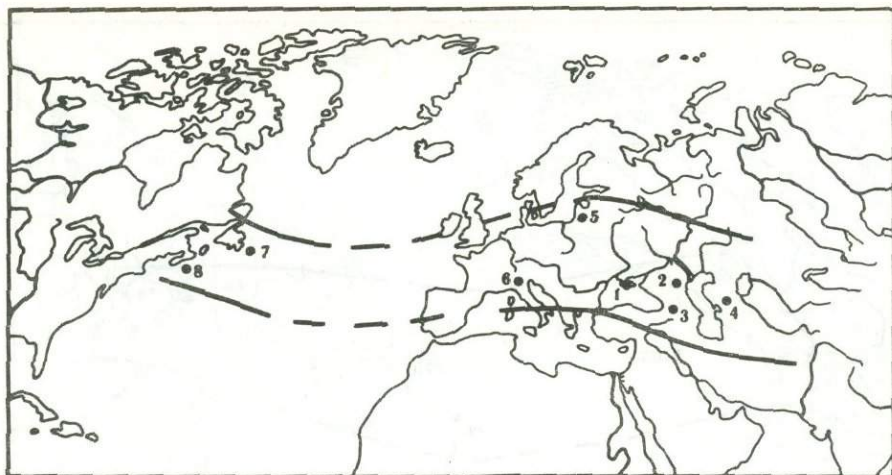
Рис. 1. Местонахождение Favosellidae и их состав в средней юре
