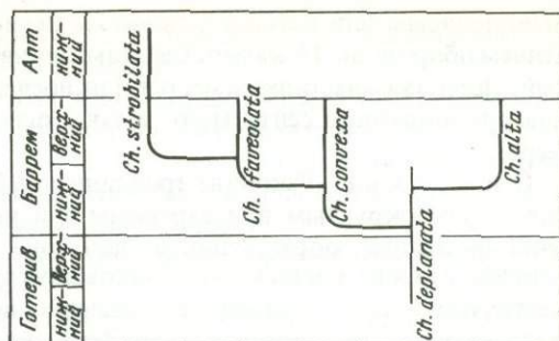
Рис. 2. Филогенетическая схема видов рода Chalilovella gen. nov. из нижнемеловых отложений Юго-Восточного Азербайджана
