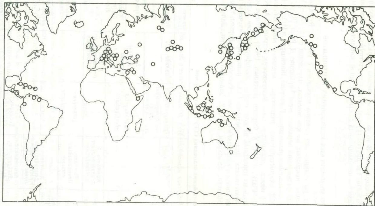
Р и с. 2. Местонахождения мезозойских радиолярий на континентах.
