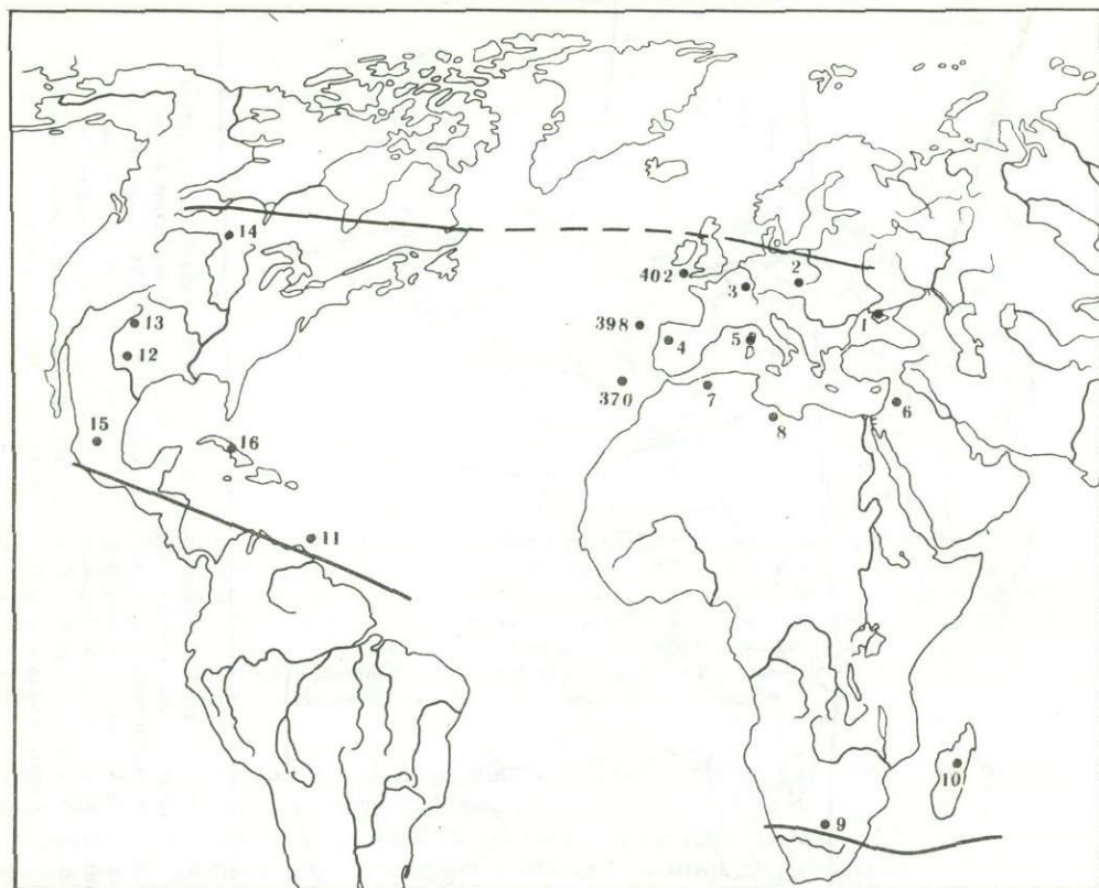
Р и с. 5. Местонахождения Favusellidae и их состав в раннем и позднем мелу (альб, сенюман)
