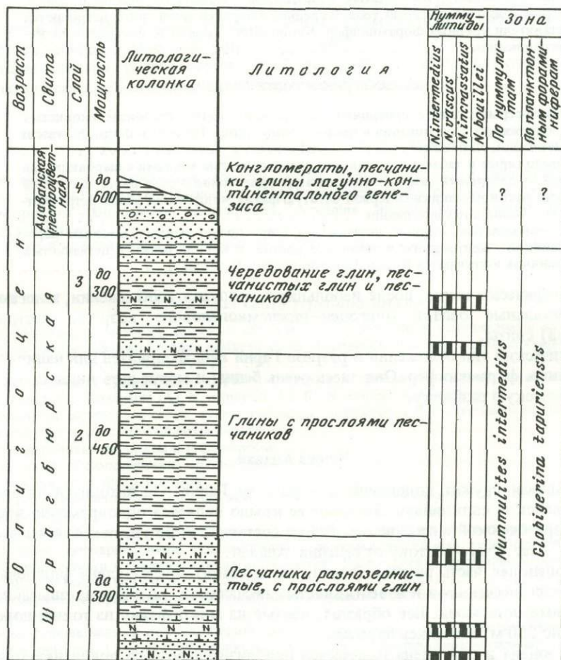
Р и с. 3. Разрез Шорагбюр: зональное деление по нуммулитидам, планктонным фораминиферам и стратиграфическое распределение нуммулитид Условные обозначения см. на рис. 2
