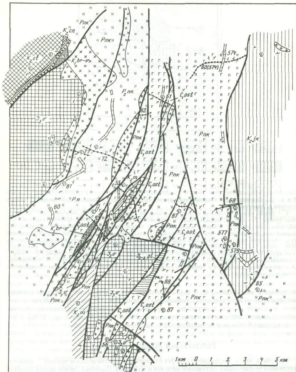
Р и с. 3. Схематическая геологическая карта междуречья Накпейляка и Хайидина Условные обозначения см. на рис. 2
