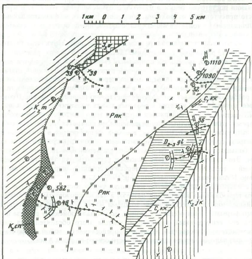
Рис. 4. Схематическая геологическая карта правобережья р. Ваамочки Условные обозначения см. на рис. 2.
