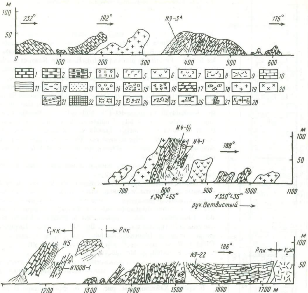
Р и с. 5. Схематическая зарисовка разреза какомейской и напейлякской толщ и их контакта с сенонскими отложениями на руч. Ветвистом
