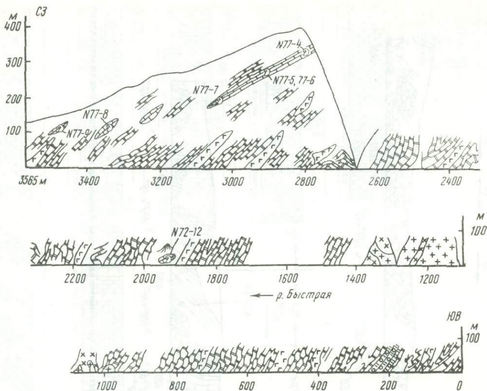
Р и с. 10. Схематическая зарисовка разреза накепейлякской толщи по р. Быстрой, левому притоку р. Накепейляк (обн. 72, 77)
