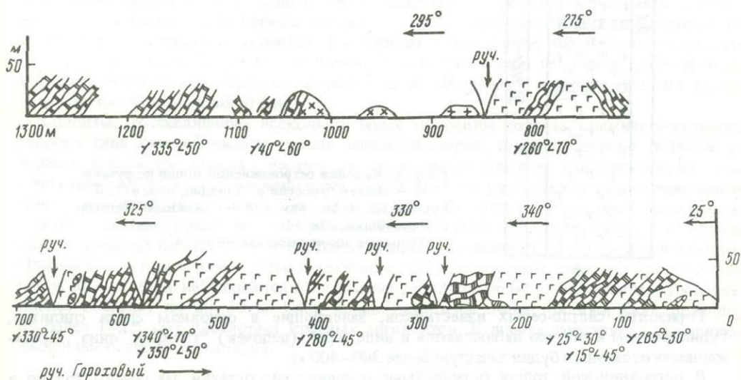
Р и с. 7. Схематическая зарисовка островнинской толщи по руч. Гороховому (левобережье р. Накепейляк, обн. 88)
