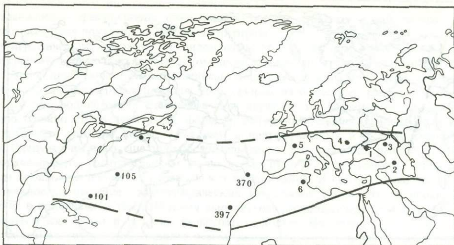
Р и с. 3. Местонахождения Favusellidae и их состав в раннем мелу (берриас, валанжин, готерив)
