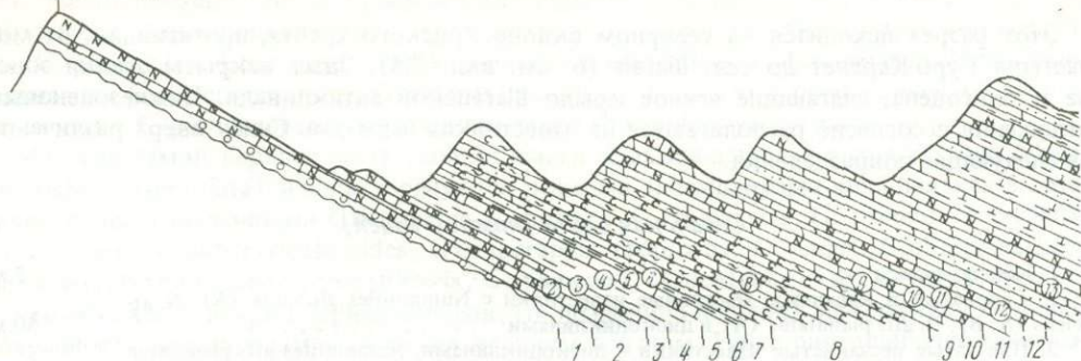
Р и с. 7. Разрез Шагап Схематический профиль
