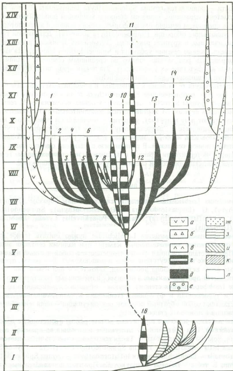
Схема филогенетического развития леблелиид и рода Spinoendothyra
