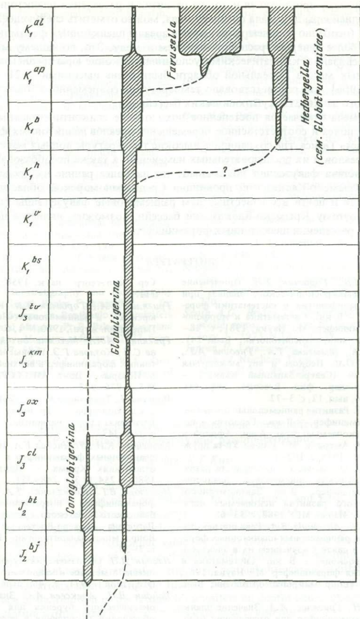
Р и с. 6. Филогенетическая схема фаузеллид
