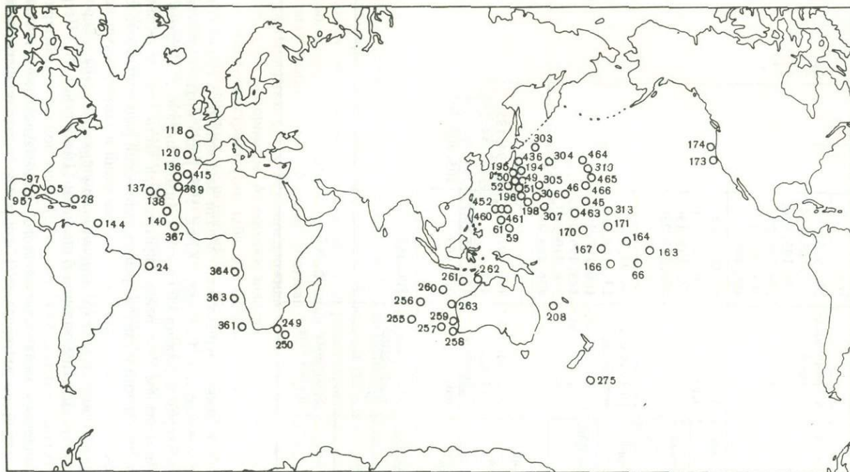
Рис. 1. Местоположение скважин DSDP (рейсы 1–62), вскрывших отложения с мезозойскими радиоляриями
