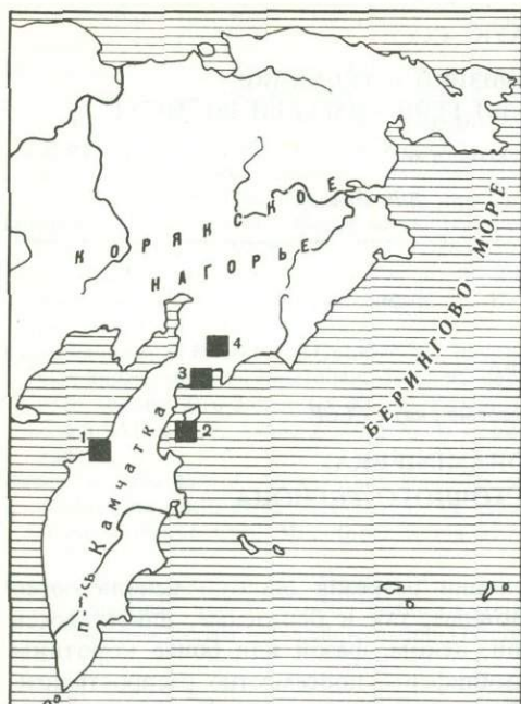
Рис. 1. Местоположение разрезов с кавказинами Разрезы: 1 - Тоцилинский, 2 - Карагинский, 3 - Ильпинский, 4 - Корфовский
