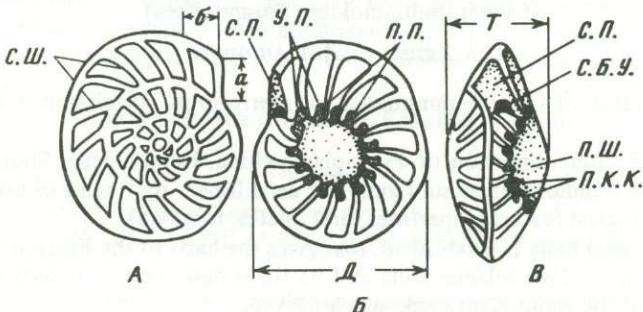
Р и с. 1. Схема строения раковины Chalilovella
