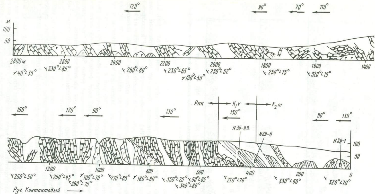
Р и с. 11. Схематическая зарисовка разреза накейляжской толщи и ее контакта с отложениями валанжина и последних с отложениями маастрихта на руч. Контактном, правом притоке р. Ваамочки (обн. 39) Условные обозначения см. на рис. 5.
