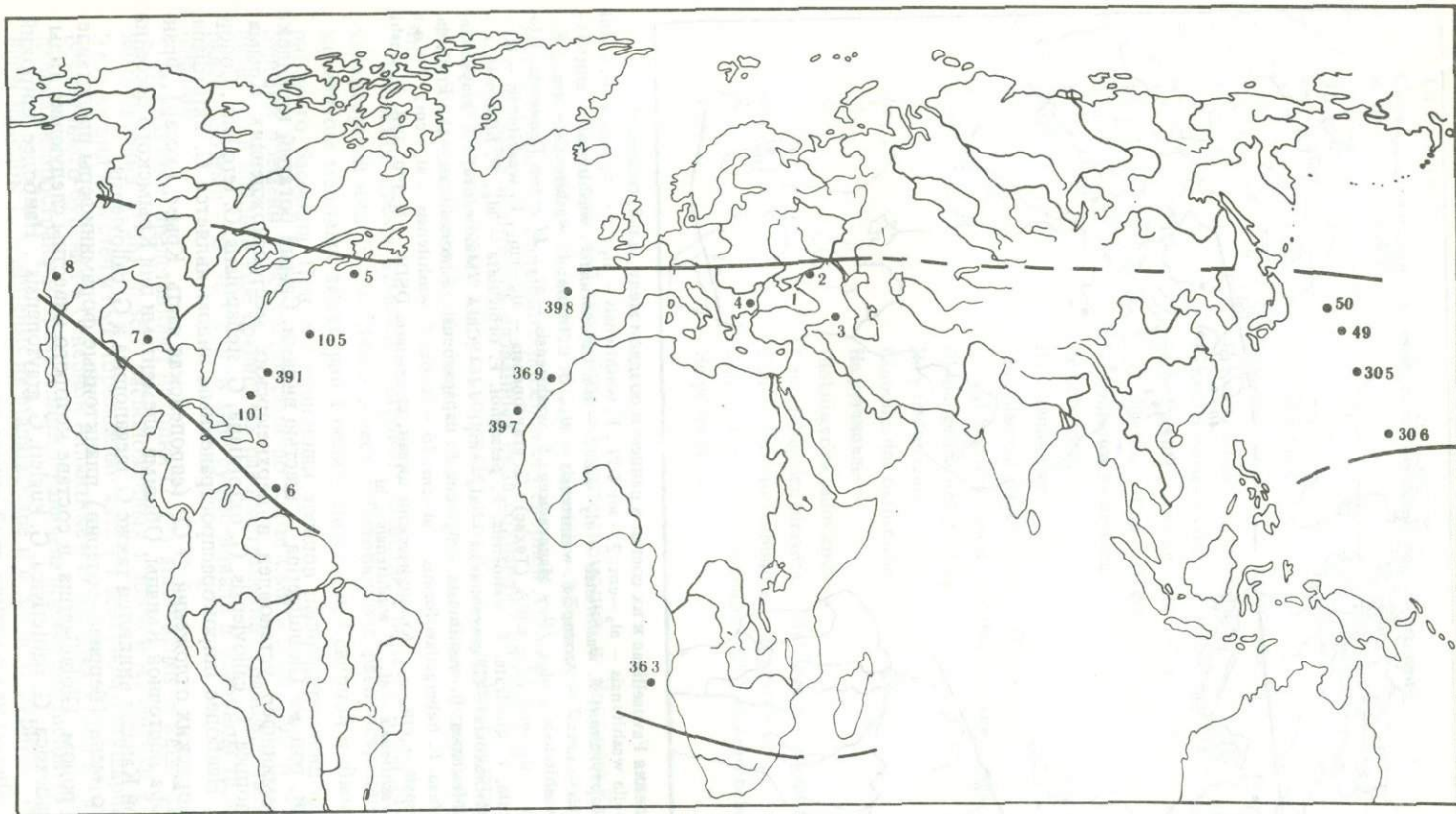
Рис. 4. Местонахождения Favusellidae и их состав в раннем мелу (баррем, апт)
