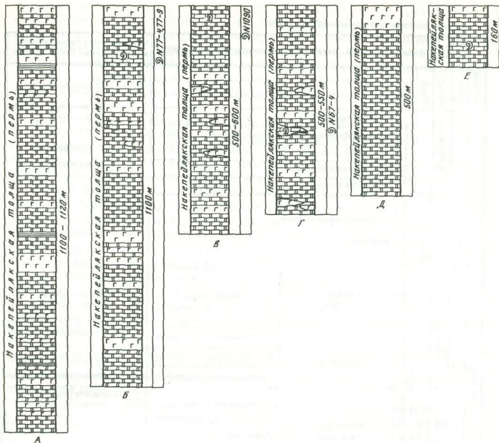
Р и с. 12. Колонки накепейлякской толщи
