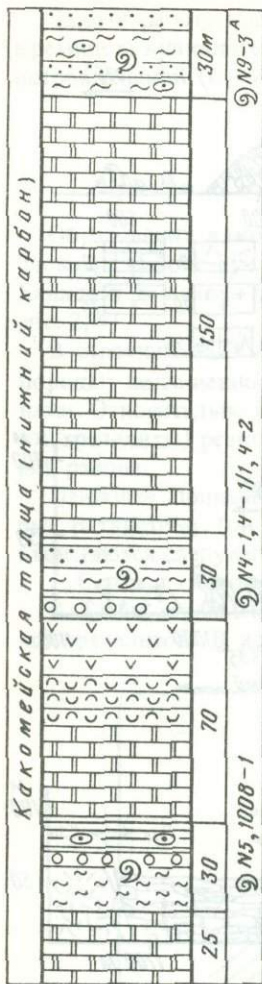
Рис. 6. Колонка какомэйской толщи по руч. Ветвистому Условные обозначения см. на рис. 5.
