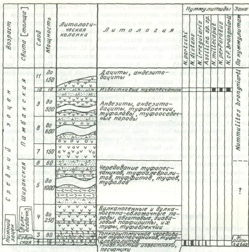
Рис. 20. Разрез южных отрогов Сомхетского хребта Зональное деление по нуммулитам и их стратиграфическое распределение Условные обозначения см. на рис. 2
