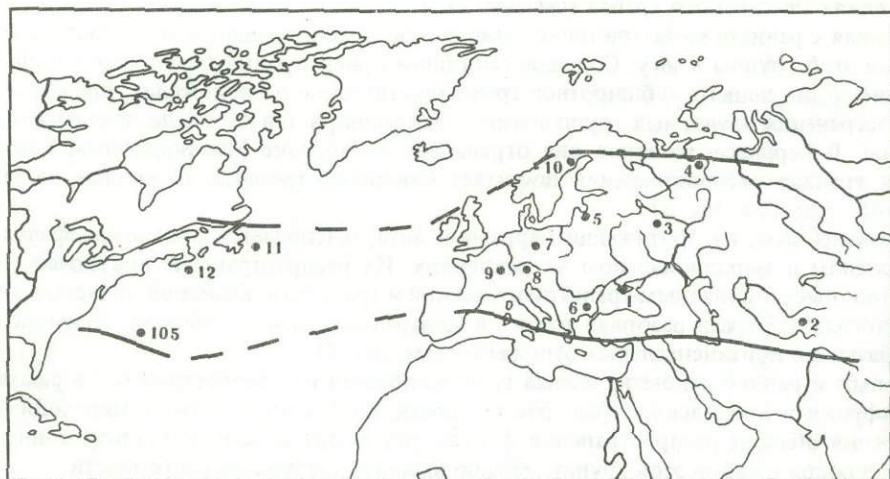
Рис. 2. Местонахождения Favosellidae и их состав в верхней юре
