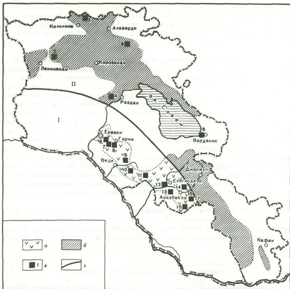
Р и с. 1. Структурно-фациальное районирование территории Армении
