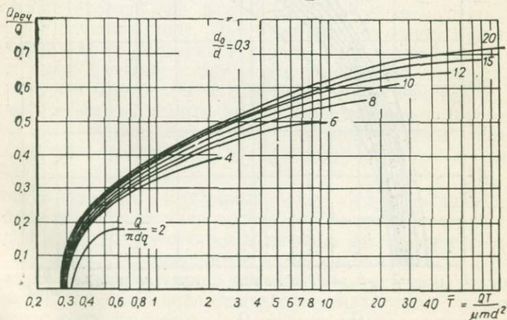
Рис. 18. График \frac{Q_{\text{реч}}}{Q} = f(\bar{T}, \frac{Q}{\pi d q}) для одиночного берегового водозабора при \beta = \frac{\pi}{2} и \frac{d_0}{d} = 0,3
