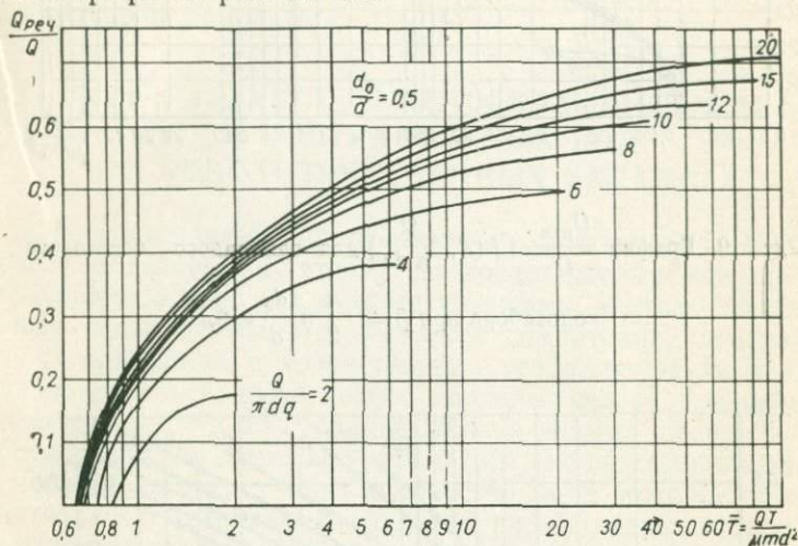
Рис. 17. График \frac{Q_{\text{реч}}}{Q} = f(\bar{T}, \frac{Q}{\pi d q}) для одиночного берегового водозабора при \beta = \frac{\pi}{2} и \frac{d_0}{d} = 0,5
