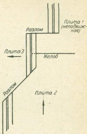
Рис. 55. Положение трех плит литосферы, ограниченных поднятием, желобом и разломом, в три последовательных отрезка времени [166].
