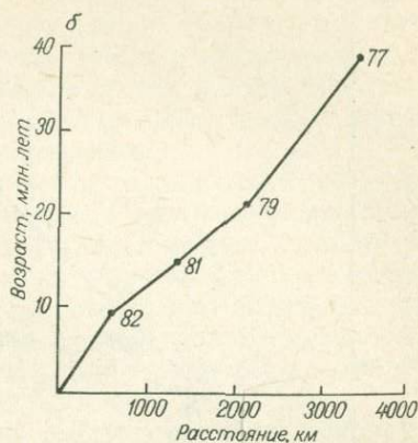
Рис. 3. Возраст древнейших осадков, вскрытых глубоководным бурением, как функция расстояния от оси Срединно-Атлантического хребта (а) и от оси Восточно-Тихоокеанского поднятия (б). Цифры вдоль линии графика — номера скважин.
