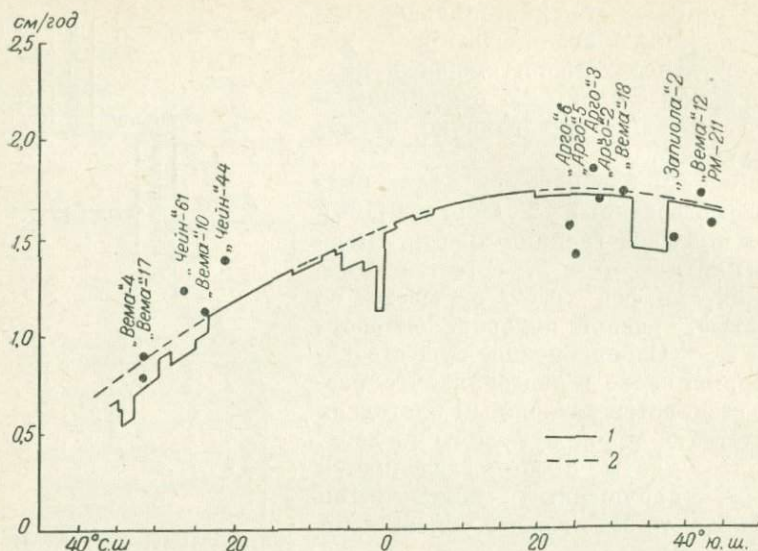
Рис. 56. Сравнение между разрастанием, основанном на магнитных аномалиях, и раздвижением двух плит для Срединно-Атлантического хребта (между Азорскими островами и о. Буве). Координаты полюса вращения 62^\circ с. ш. и 36^\circ з. д.
