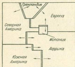
Рис. 116. Открытие Атлантического океана, по Ж. Франшто [64].
