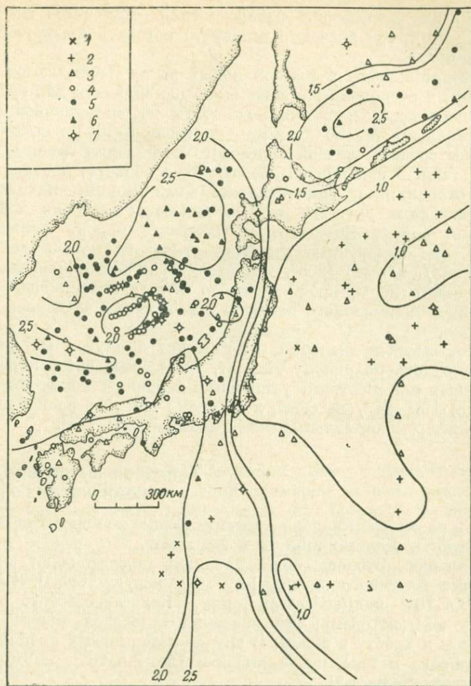
Рис. 76. Тепловой поток в районах, прилегающих к Японии (по С. Уеда и В. Ваке. Японский национальный доклад по Проекту верхней мантии).
