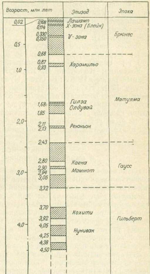
Рис. 33. Изменение полярности геомагнитного поля за последние 4,5 млн лет. Из Ф. Стейса, 1972. Заштрихованные участки — прямая полярность; незаштрихованные — обратная.
