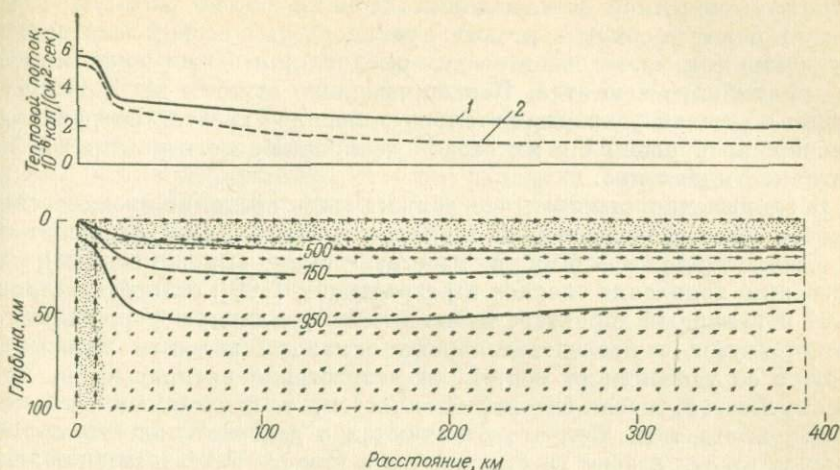
Рис. 86. Изотермы (внизу) и тепловой поток (вверху) для модели восходящего потока. По М. Лагсету и К. Ле Пиншону, 1968. 1 — кривая теплового потока для Восточно-Тихоокеанского поднятия; 2 — то же, для Атлантико-Индийского хребта.
