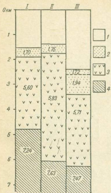
Рис. 66. Сейсмические разрезы в районе хр. Рейкьянес. По М. Юингу и Дж. Юингу, 1959.
