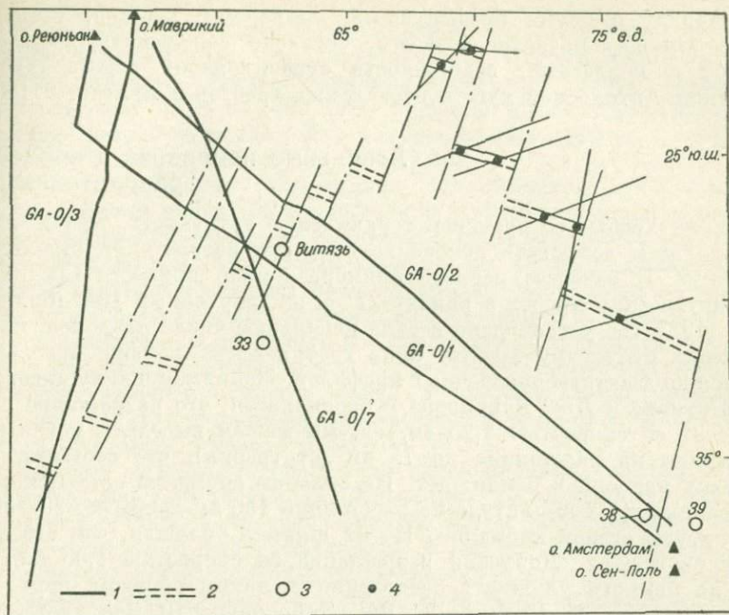
Рис. 46. Юго-западная и юго-восточная ветви Срединно-Индийского хребта [197]. 1 — профили; 2 — предполагаемая ось хребта; 3 — сейсмическое профилирование МПВ; 4 — осевая магнитная аномалия.
