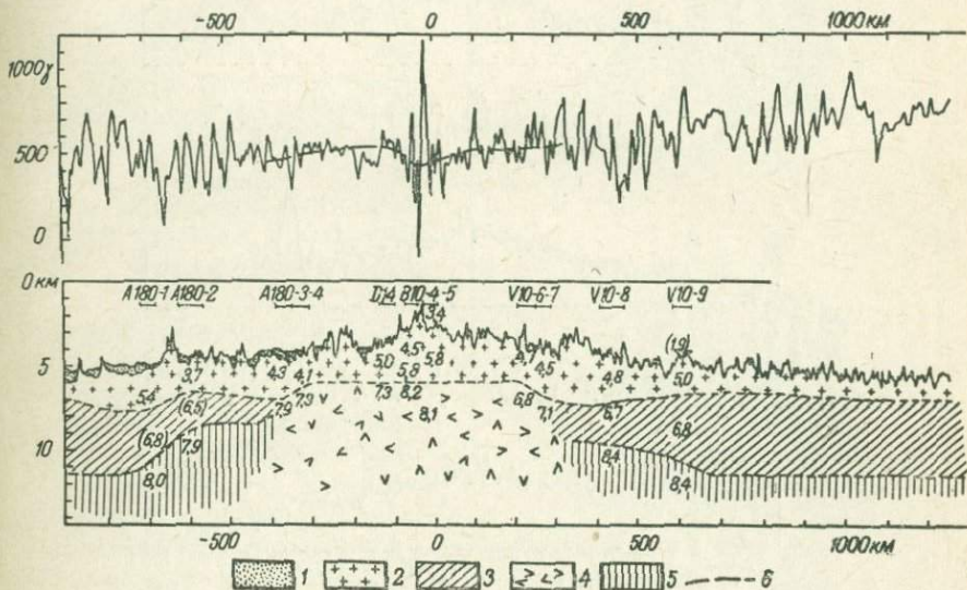
Рис. 15. Магнитный профиль через Средне-Атлантический хребт на 32^\circ с. ш., приведенный к постоянной глубине 3 км [88].
