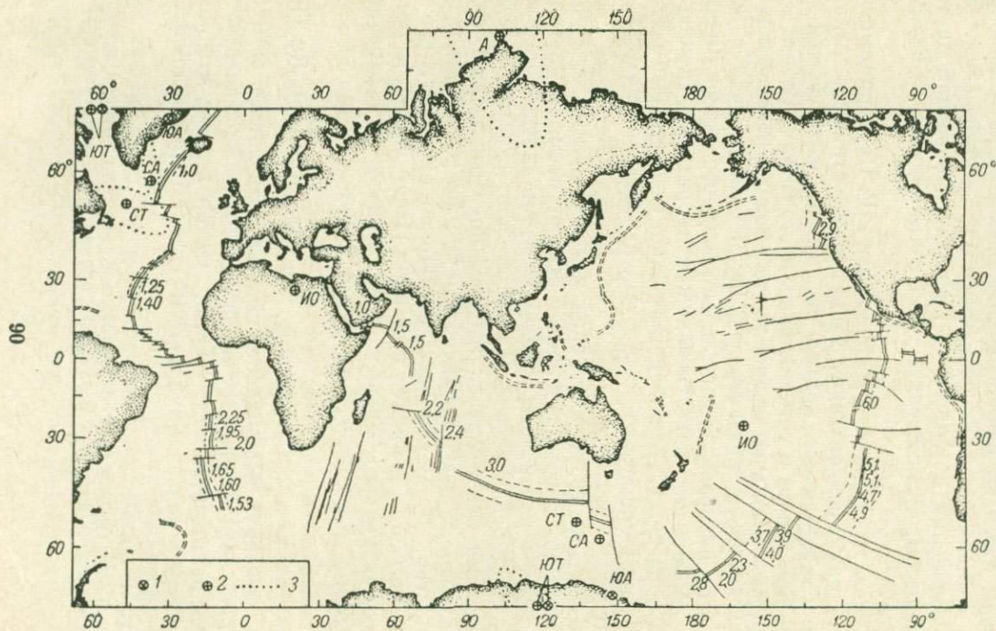
Рис. 57. Магнитные аномалии и полюса вращения Атлантического, Тихого и Индийского океанов [121].
