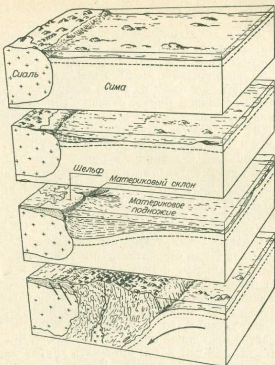
Рис. 98. Геосинклинальный цикл и рост материков [36].
