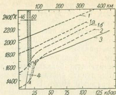
Рис. 93. Возможность плавления верхней мантии по пиролитовой гипотезе [139]. 1 — ликвидус ( \alpha — 50% расплава, \beta — 25% расплава); 2 — солидус; 3 — градиент 1,3 град/км; 4 — градиент 27 град/км.
