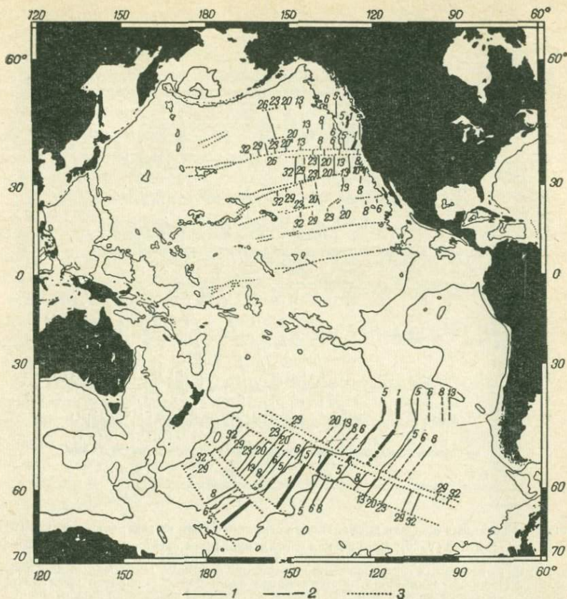
Рис. 48. Магнитные аномалии Тихого океана [184].
