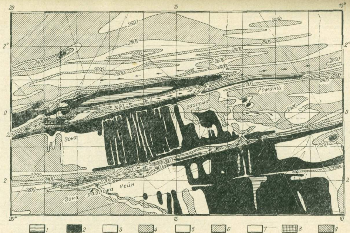
Рис. 27. Батиметрическая схема части зоны разломов Чейн и Романиш. По Б. Хизену, Э. Бане, Дж. Херри и М. Тарп, 1964. Линии зондирования показаны точечными линиями. Изобаты, где возможно, проведены через 200 морских саженей. Глубина, морск. сажень: 1 — менее 1400; 2 — 1400—2000; 3 — 2000—2200; 4 — 2200—2400; 5 — 2400—2600; 6 — 2600—2800; 7 — 2800—3000; 8 — 3000—4000; 9 — более 4000.
