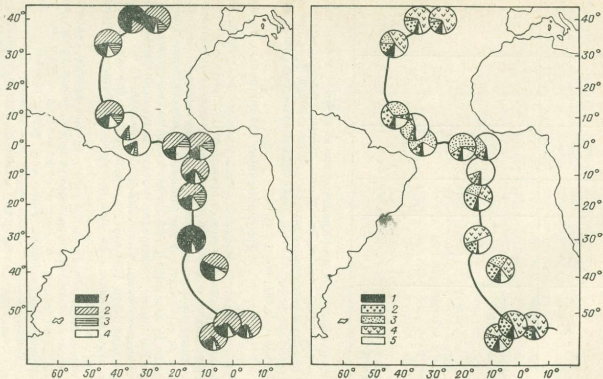
Рис. 67. Минеральный состав драгированных песков тяжелой (а) и легкой (б) фракций [63].
