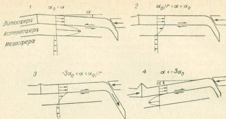
Рис. 109. Горизонтальное движение плит литосферы по моделям Л. Ллибуэри [130].
