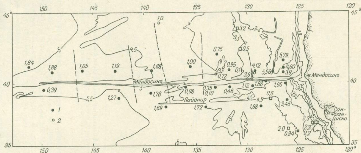
Рис. 80. Тепловой поток вблизи зон разломов Мендосино и Пайонир. По Р. П. фон Герцену, 1964.
