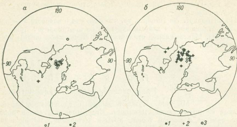
Рис. 52. Положение полюса, определенного по палеомагнитным данным для Северной Америки (а) и Европы (б) [192].
