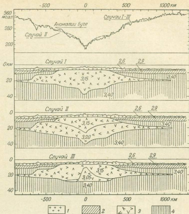
Рис. 71. Модель строения коры Срединно-Атлантического хребта, на которой (в отличие от модели на рис. 70) показано существование нормальной мантии в зоне склонов хребта [211].
