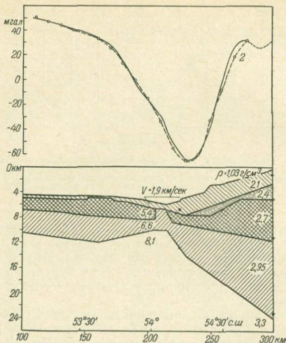
Рис. 75. Строение земной коры Алеутского желоба по гравиметрическим, сейсмическим и магнитным данным [180]. Аномалии Фая: 1 — наблюдаемые; 2 — рассчитанные.
