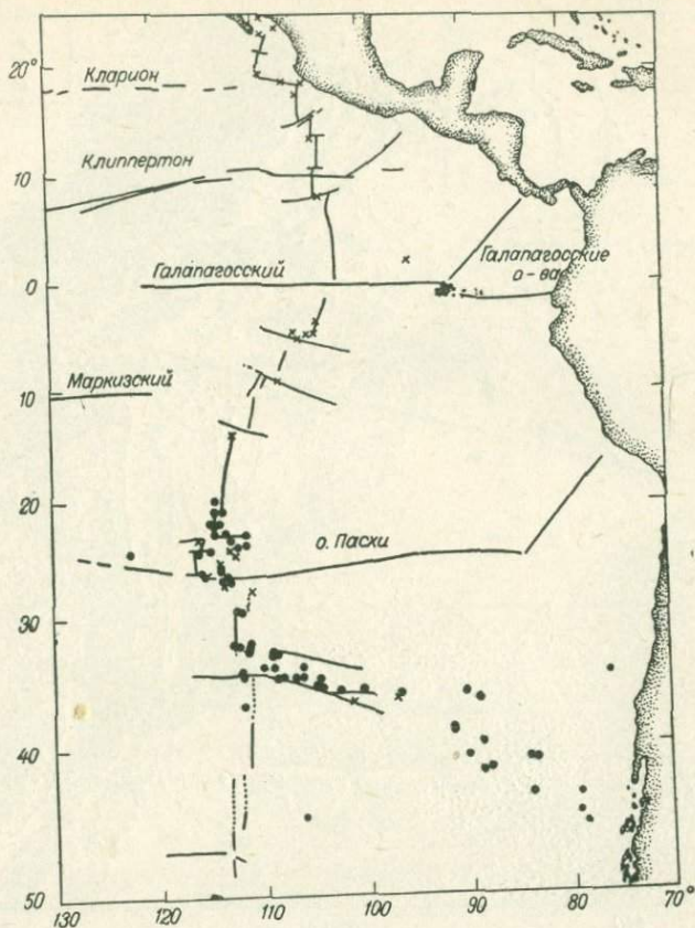
Рис. 30. Гребень Восточно-Тихоокеанского поднятия, смещенный активными разломами. Точками показаны эпицентры землетрясений, по Л. Сайксу (1963); крестиками — то же, по данным Международной сейсмологической службы [153].
