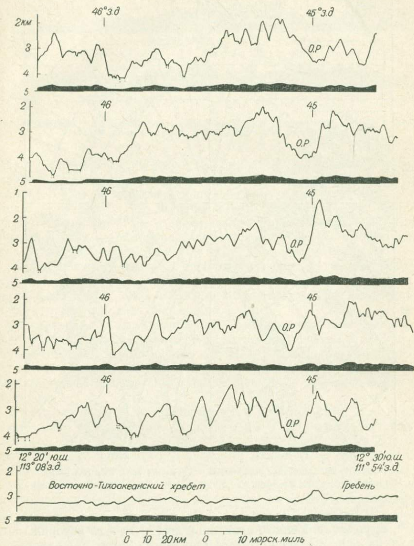
Рис. 6. Профили через Срединно-Атлантический хребет между 22 и 23° с. ш. и Восточно-Тихоокеанское поднятие в районе 12° ю. ш. [222].
