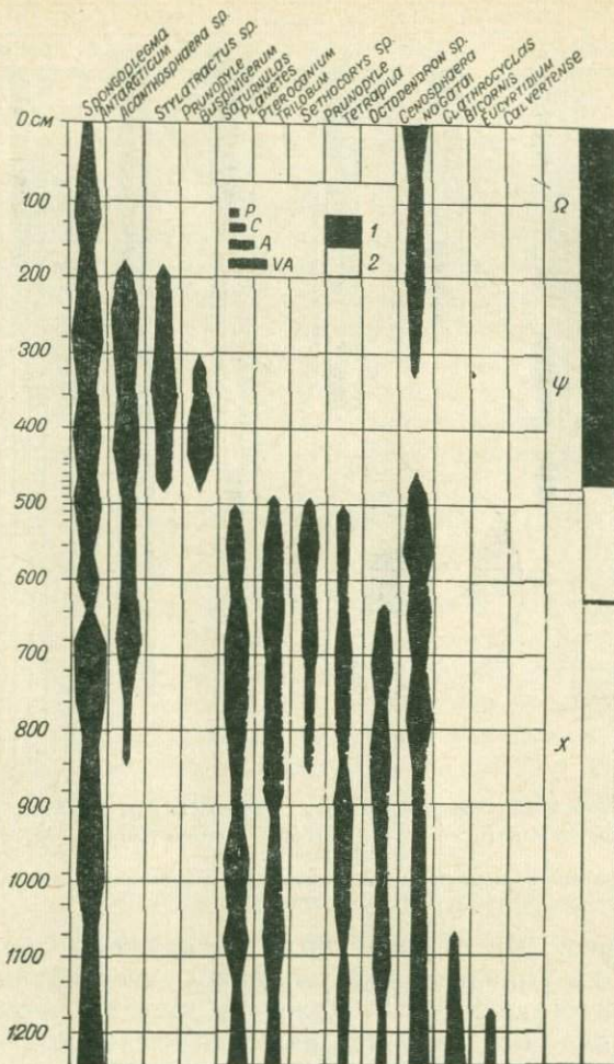
Рис. 35. Частота встречаемости руководящих видов в антарктической колонке [174].
