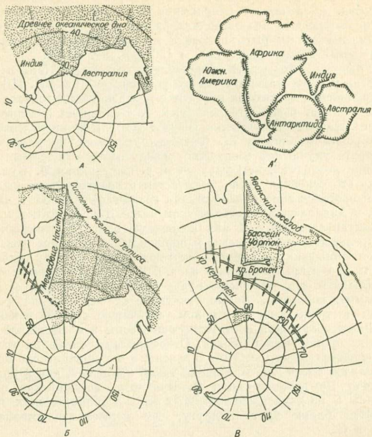
Рис. 119. Диаграммы временной последовательности событий, показывающие отделение Индии и Австралии от Антарктиды, их последующий дрейф и сохранение древней коры в бассейне Уортон [223].
