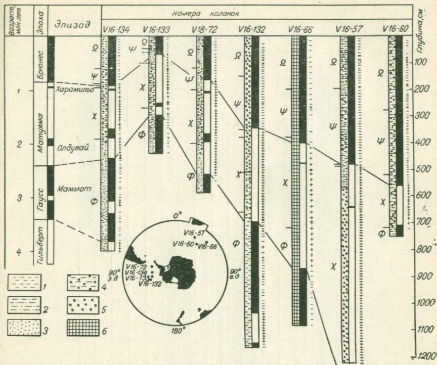
рис. 34. Корреляция магнитных событий между семью антарктическими колонками [174]. 1 — лютит; 2 — лютит и ил; 3 — ил; 4 — лютит с диатомитами; 5 — диатомитовые осадки; 6 — карбонатные осадки. Знаком минус показана нормальная намагниченность; знаком плюс — обратная; греческими буквами обозначены фаунистические зоны.
