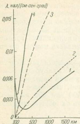
Рис. 91. Распределение теплопроводности в верхней мантии [131].
