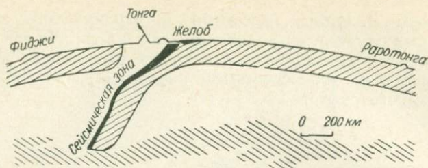
Рис. 41. Схематический разрез литосферы по профилю Фиджи — Тонга — Раротонга [171].
