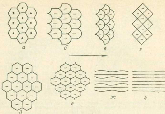
Рис. 96. Эволюция конвекционных ячеек в потоке с умеренной, но постоянной скоростью (по А. Грэмму; рис. Ж. Кулона и Ж. Луазеля, 1940).
