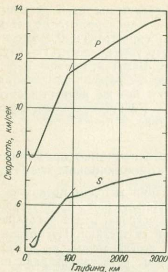
Рис. 64. Скорости волн P и S в мантии, по Б. Гутенбергу, экстраполированные к поверхности [24].
