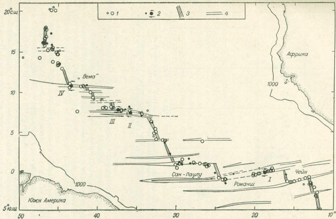
Рис. 39. Эпицентры Экваториальной Атлантики за 1955—1965 гг. и механизм четырех землетрясений на Срединно-Атлантическом хребте [209].
