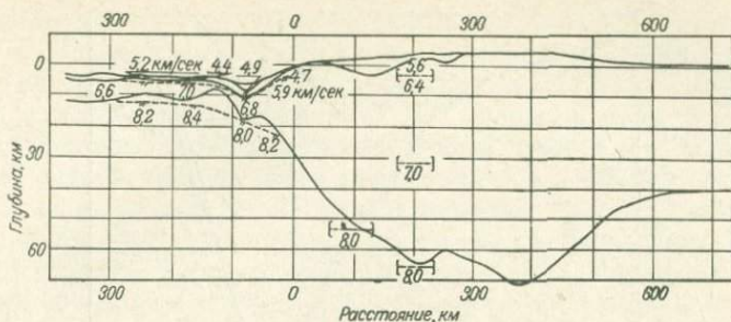
Рис. 74. Разрез земной коры через материковую окраину и глубоководный желоб вблизи г. Антофагаста (Чили), построенный по гравиметрическим данным (П. Уиншед, неопубликованная диссертация) в сравнении с недавними результатами сейсмических исследований Р. Фишера и Р. Райта [239].
