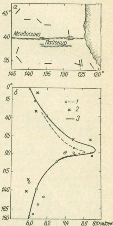
Рис. 69. Положение сейсмических профилей, выполненных по методу преломленных волн, по Р. Райту (а) и зависимость скорости волны P от азимута (б). 1 — район Мендосино; 2 — район Мауи; 3 — две области вместе.
