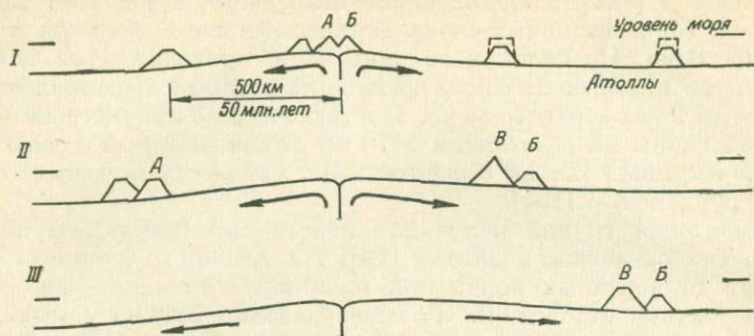
Рис. 99. Образование гайотов и атоллов [96].
