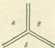
Рис. 106. Схема соединения трех плит литосферы, имеющих общую точку (triple point) [146].
