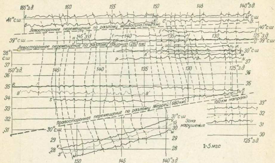
Рис. 25. Профили магнитных аномалий к западу от Калифорнии [221].
