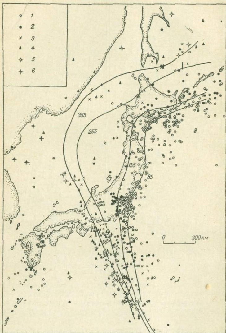
Рис. 4. Эпизентры глубоких землетрясений за 1926—1956 гг. (материалы Метеорологической службы Японии). Контуры, по данным А. Суги ура и С. Уеда (Японский национальный доклад по Проекту верхней мантии, 1967).
