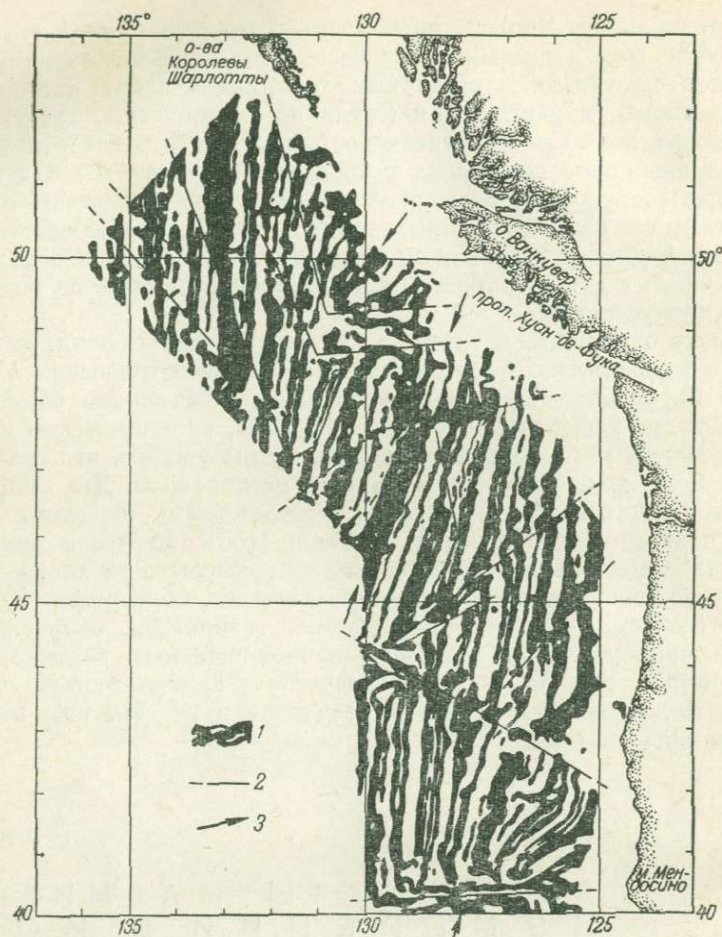
Рис. 13. Магнитные аномалии, открытые А. Раффом и Р. Мейсоном в 1961 г. [226].
