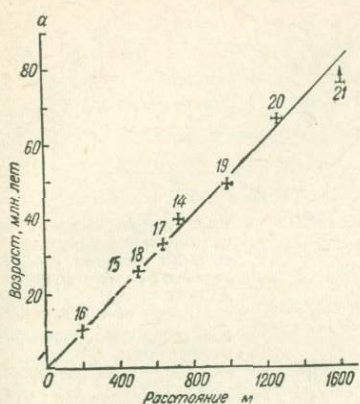
Рис. 3. Возраст древнейших осадков, вскрытых глубоководным бурением, как функция расстояния от оси Срединно-Атлантического хребта (а) и от оси Восточно-Тихоокеанского поднятия (б). Цифры вдоль линии графика — номера скважин.
