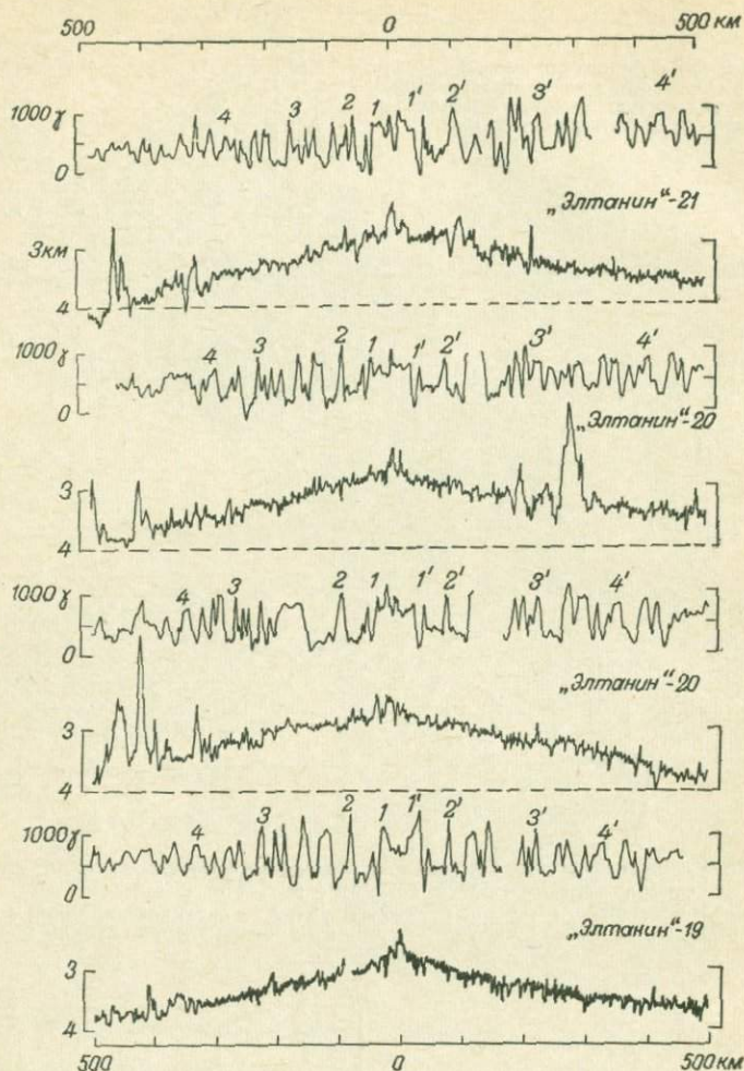
Рис. 17. Магнитные и топографические профили по маршрутам, перпендикулярным к оси хребта [183].
