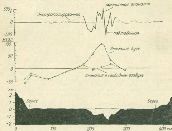
Рис. 20. Разрез через Красное море в районе 16° с. ш. с магнитным и гравиметрическим профилями. По Ч. Дрейку и Р. Гирдлеру, 1964.
