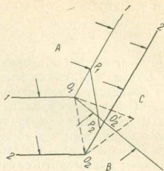
Рис. 107. Эволюция тройного соединения.
