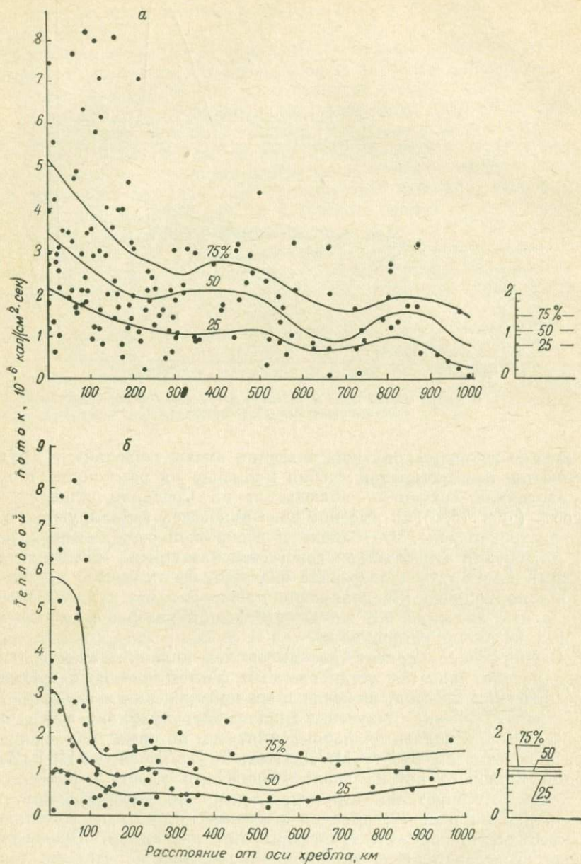
Рис. 78. Зависимость величины теплового потока от расстояния до гребней Восточно-Тихоокеанского (от 50° ю. ш. до 20° с. ш.) поднятия (а) и Срединно-Атлантического хребта (б) [118].
