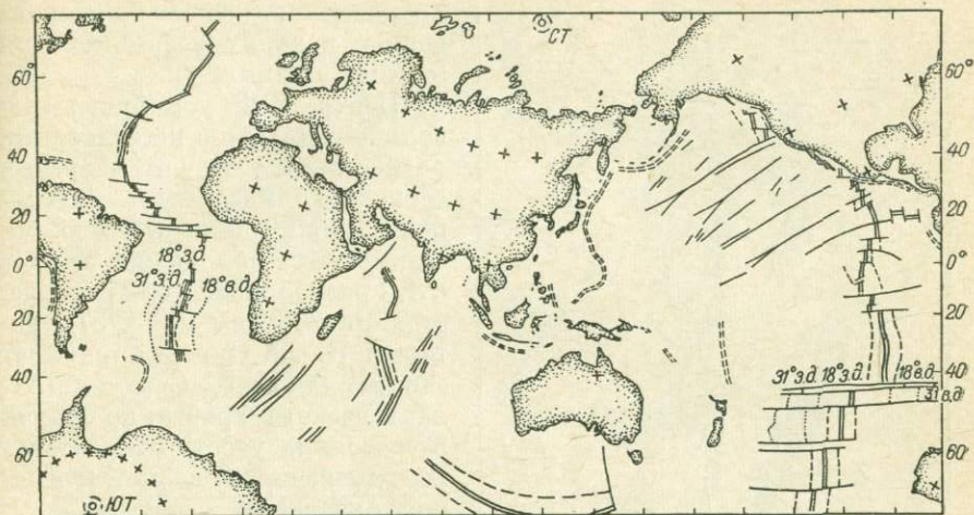
Рис. 58. Полюс проекции в южной части Тихого океана ( 69^\circ ю. ш., 123^\circ в. д.) [121]. Показаны аномалии 5, 10 и 31. Крестиком отмечено пересечение современных параллелей и меридианов с интервалом 20^\circ .
