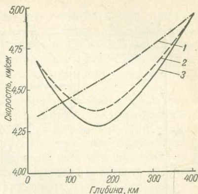
Рис. 88. Скорости поперечных сейсмических волн в верхней мантии [225].
