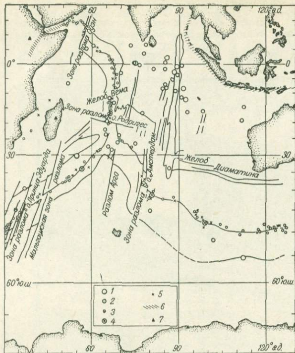
Рис. 28. Эпицентры землетрясений Индийского океана за 1942—1964 гг. По Ч. Стоверу, 1966.
