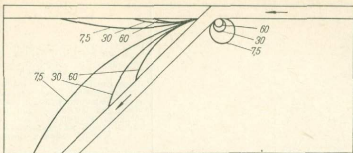
Рис. 110. Тепловое поле напряжений, обусловленное вязкой диссипацией, в единицах 10^{-7} эрг·см -3 ·сек -1 [142]. Разогрев мантии происходит более интенсивно в тылу дуги, чем перед ней.
