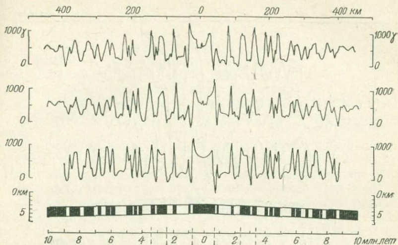
Рис. 42. Профиль аномального магнитного поля, полученный судном «Элтанн-19» (в середине) [183]. Вверху тот же профиль в обратном направлении (с запада на восток). Внизу модель для Тихоокеанско-Антарктического хребта.
