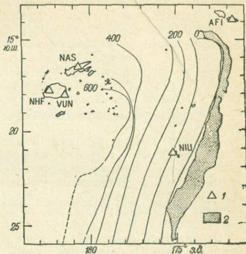
Рис. 5. Распределение глубокофокусных очагов в районе желоба Тонга [171].
