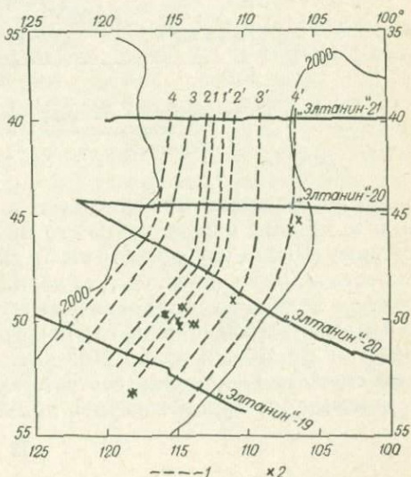
Рис. 16. Маршрут судна «Этанин» [183]. 1 — аномалии, выявленные на четырех профилях; 2 — примерное положение эпицентров землетрясений. Глубины даны в морских саженях.
