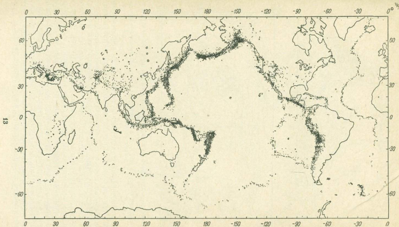
Рис. 1. Распределение эпицентров землетрясений с глубиной очагов 0—100 км (а) и 100—700 км (б) за 1961—1967 гг. [40].
