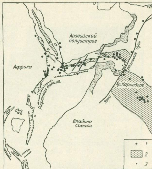
Рис. 29. Смещение хр. Карлсберг по разлому Оуэн. По А. Ляутону, 1967.
