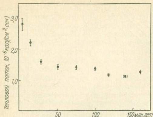
Рис. 111. График зависимости средних значений теплового потока от возраста провинции в северной части Тихого океана [202].
