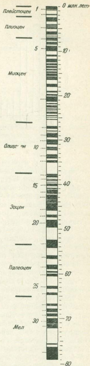
Рис. 50. Ламонтская шкала инверсий магнитного поля [90]. Слева направо: фанерозойская шкала геологического времени, номер аномалии, магнитная полярность (нормальная полярность показана черными отрезками рядом с колонкой).
