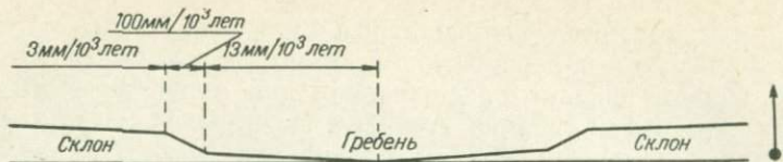
Рис. 47. Общая схема распределения мощностей осадков в зоне гребня и на склонах срединно-океанического хребта, составленная на основе данных по экваториальной части Тихого океана [52].
