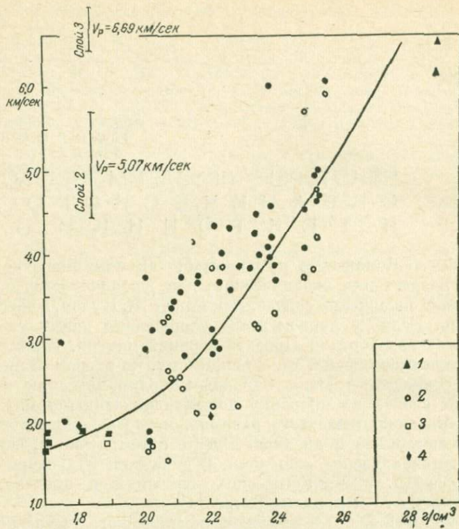
Рис. 1. Зависимость скорости продольных волн от плотности для литифицированных осадков и базальтов [84*].
