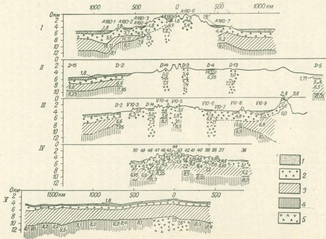
Рис. 65. Разрезы строения коры Средне-Атлантического хребта (профили I—IV) и Восточно-Тихоокеанского поднятия (профиль V) [127]. 1 — неконсолидированные отложения; 2 — фундамент; 3 — океанический слой; 4 — нормальная мантия; 5 — аномальная мантия ( V_p = 7,3 км/сек).
