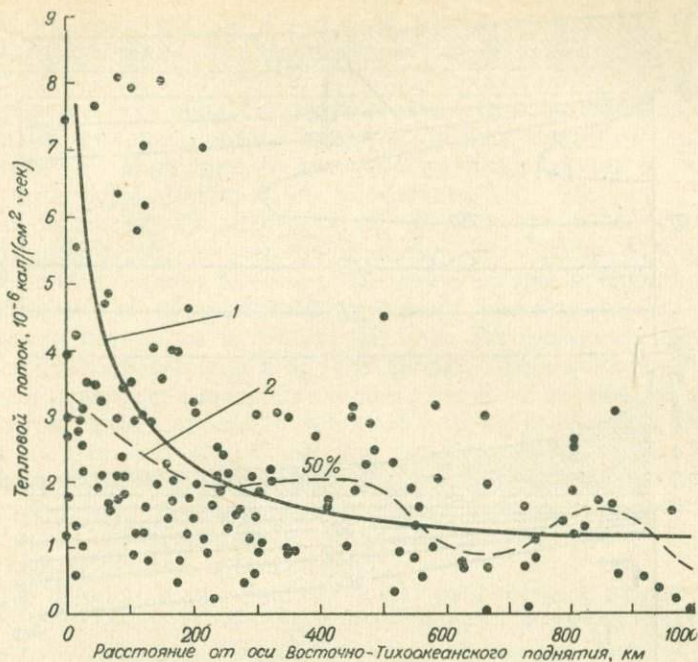
Рис. 83. Тепловой поток в Тихом океане [141].
