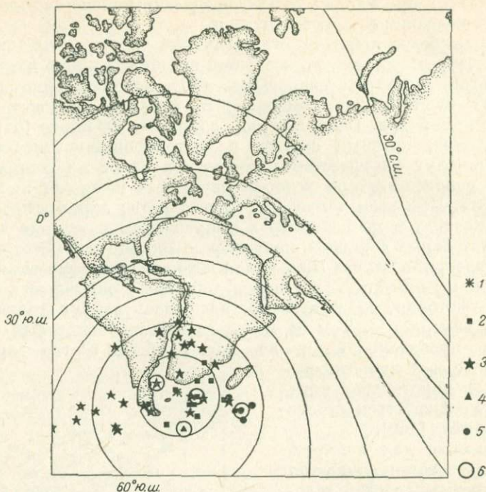
Рис. 118. Палеогеография материков, прилегающих к Атлантическому океану в позднекаменноугольное время (совмещение по Э. Булларду с соавторами в меркаторской проекции) [64]. 1 — среднее положение южного магнитного полюса; 2 — южные полюса для Северной Америки; 3 — то же, для Европы; 4 — то же, для Африки; 5 — то же, для Южной Америки; 6 — среднее положение полюса для каждого материка. Северная Америка считалась неподвижной. Палеошироты, найденные по палеомагнитным данным, проведены через 15^\circ .
