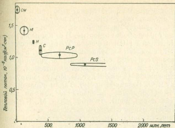
Рис. 112. График зависимости средних значений теплового потока от возраста складчатости материков, по Б. Г. Поляку и Я. Б. Смирнову (1968) [202].
