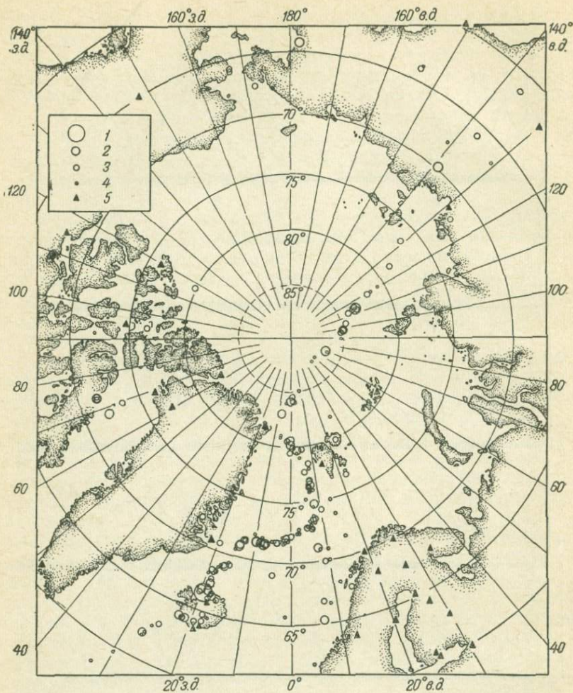
Рис. 7. Распределение эпицентров в Арктике (1955—1965 гг.) [208]. Магнитуда: 1 — 7,0; 2 — 6,0; 3 — 5,0; 4 — 4,0; 5 — сейсмические станции.
