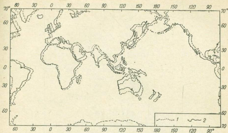
Рис. 61. Положение материков относительно Антарктиды [121].
