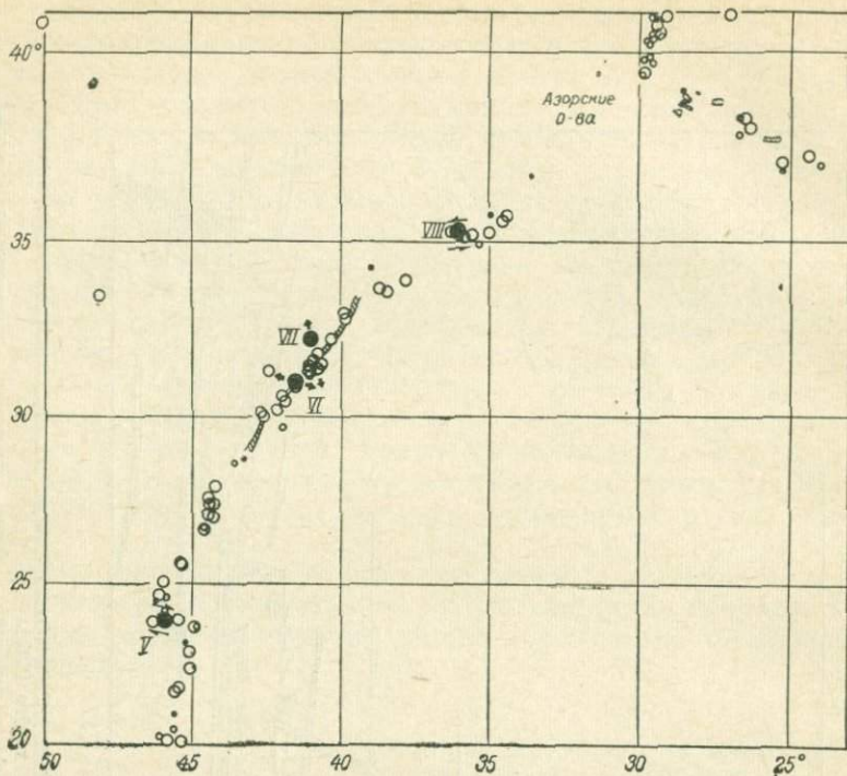
Рис. 40. Эпицентры землетрясений за 1955—1965 гг. на одном из сегментов Средне-Атлантического хребта [209].
