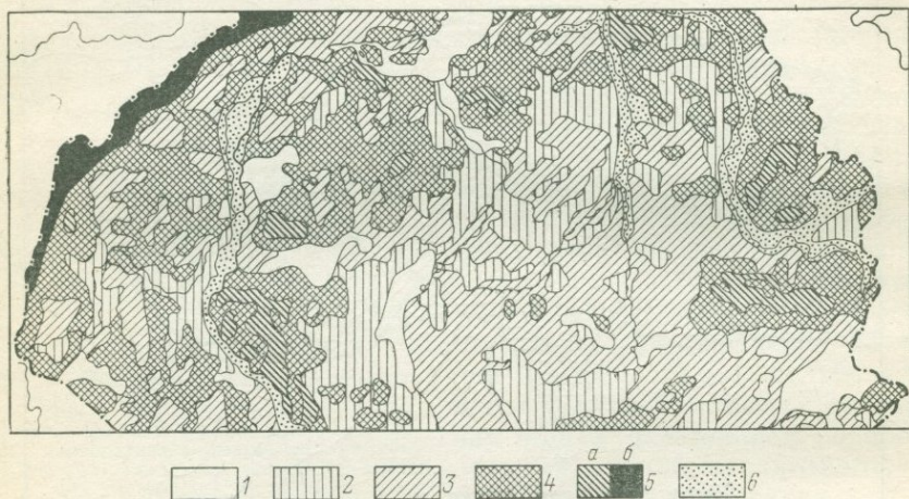
Рис. 10. Карты густоты расчленения рельефа (по Е. М. Николаевской).
