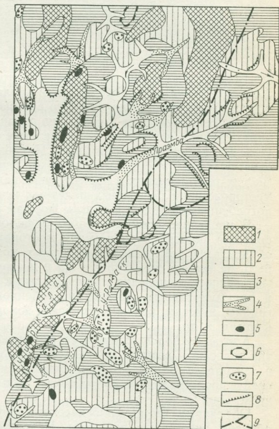
Рис. 21. Палеогеоморфологическая карта юго-восточной части Прикаспийской впадины (по Ф. М. Мешалкину и М. В. Проницовой).
