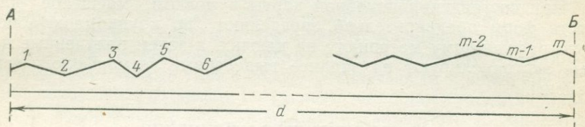
Рис. 11. Профиль рельефа (по В. Н. Ченцову)
