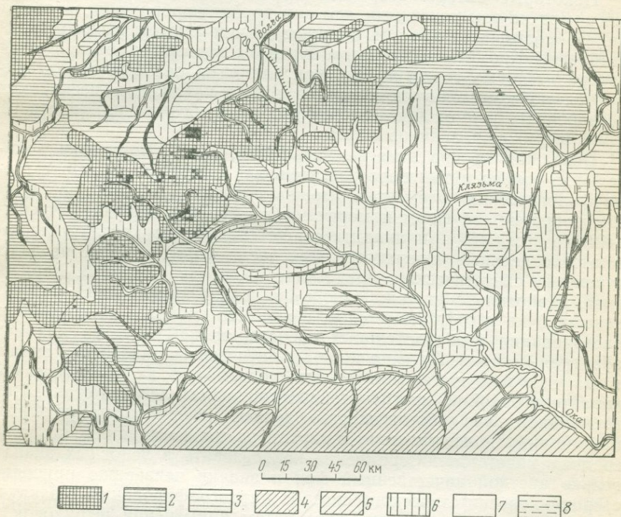
Рис. 2. Синтетическая геоморфологическая карта (центр Европейской части СССР) Аккумулятивные ледниковые и водноледниковые равнины, значительно переработанные флювиальными и склоновыми процессами. 1 — краевые образования среднечетвертичных оледенений — моренно-камовые холмисто-грядовые с моренными западинами, котловинами спущенных и заросших озер, ложбинами стока талых вод, расчлененные эрозией долинно-балочной сетью; 2 — возвышенные холмистые и плоские моренные равнины, сильно расчлененные долинно-балочной сетью; 3 — низкие преимущественно плоские и плоскохолмистые моренные равнины относительно слабо расчлененные долинно-балочной сетью. Эрозийные равнины на близком залегании коренного пластово-моноклиального основания; 4 — высокие равнины, интенсивно расчлененные долинно-балочной и овражной сетью; 5 — средневисотные и низкие равнины слабо расчлененные долинно-балочной и овражной сетью с реликтами плоских поверхностей на междуречьях; 6 — террасированные задрово-аллювиальные плоские и плосковолнистые низкие равнины и нерасчлененные средне- и позднечетвертичные террасы; 7 — поймы; 8 — днища крупных озерных котловин
