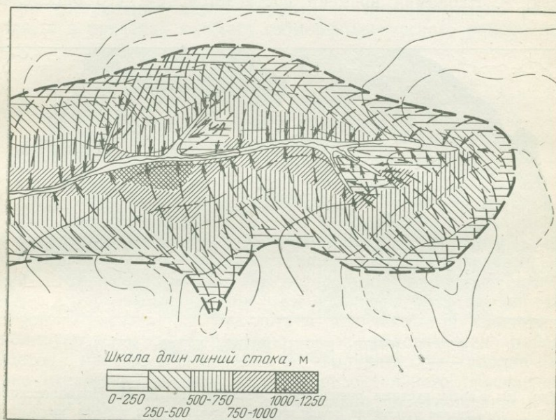
Рис. 9. Карта длин линий стока (по Е. А. Мировой)
