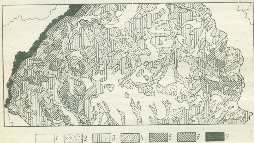
Рис. 13. Карты глубины расчленения рельефа (по Е. М. Николаевской). Относительные высоты местных базисов эрозии, м: 1 — менее 5; 2 — 5—10; 3 — 10—25; 4 — 25—50; 5 — 50—100; 6 — 100—200; 7 — более 200
