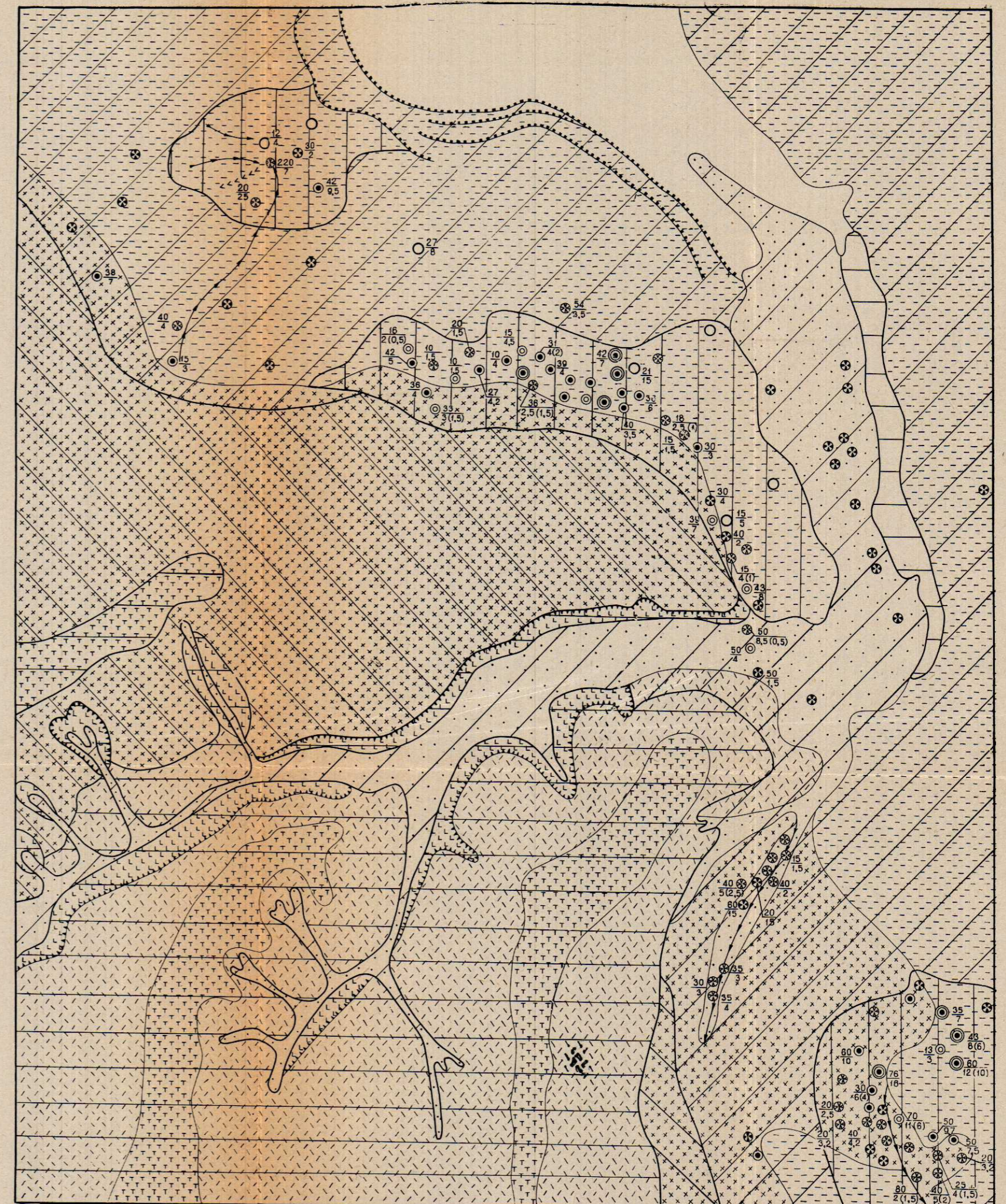
Рис. 23. Фрагмент инженерно-геоморфологической карты района водохранилища (по А. Л. Ревзону и др.)
