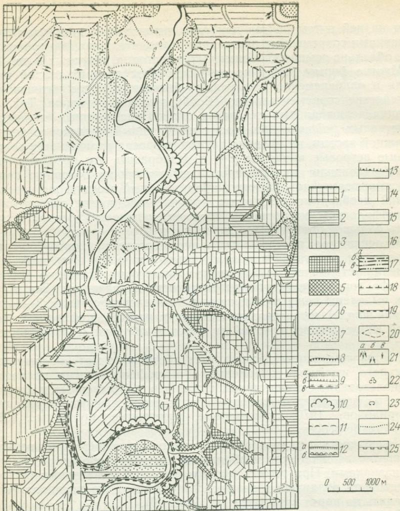
Рис. 20. Карта современных геоморфологических процессов
