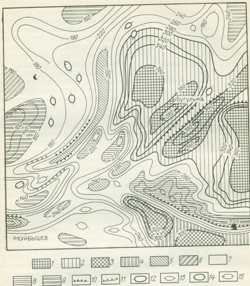
Рис. 3. Фрагмент карты морфоструктур Волго-Уральской нефтеносной области (по С. К. Горелову)
