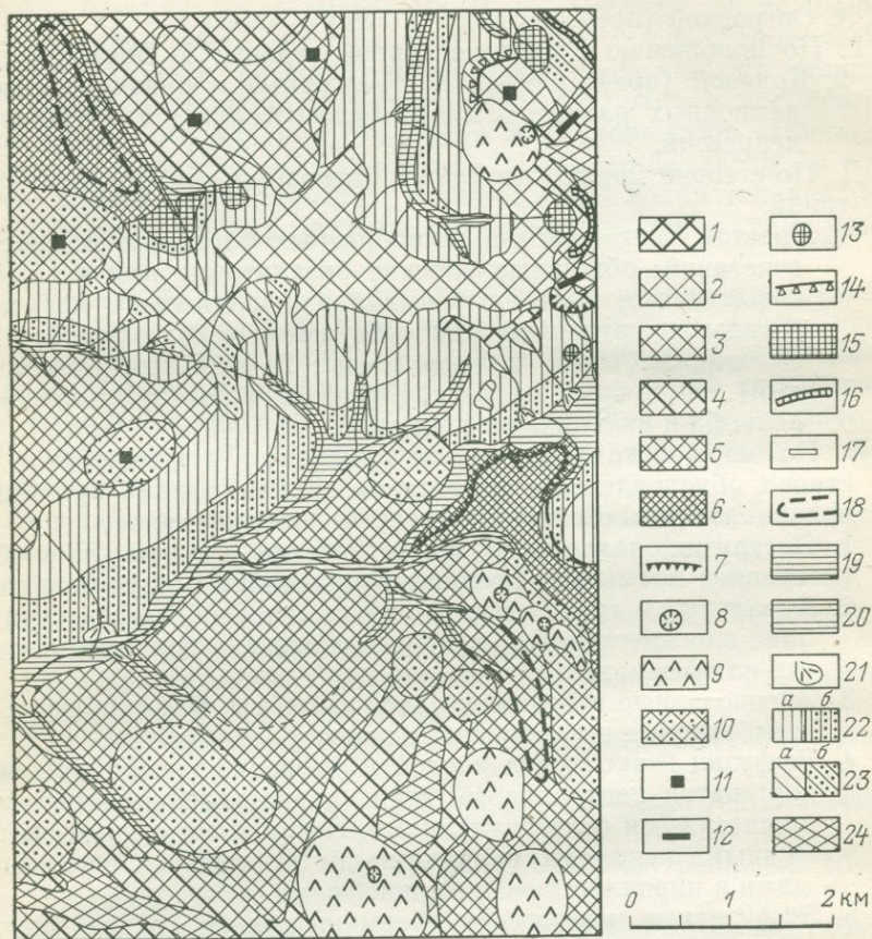
Рис. 5. Геоморфологическая карта горно-вулканического района
