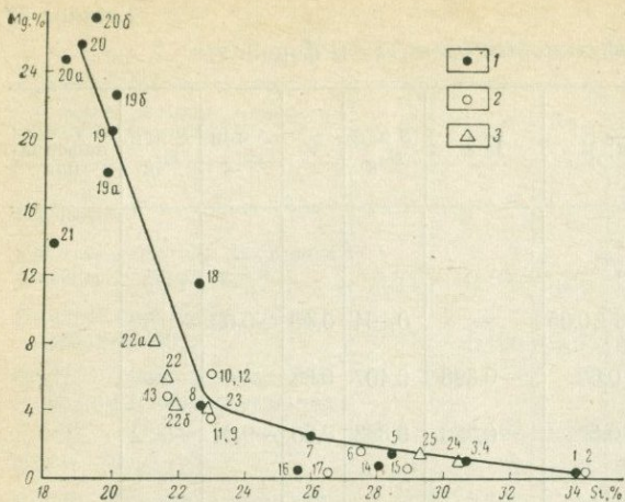
Рис. 13. Вариационная диаграмма магний — кремний в горных породах литосферы
