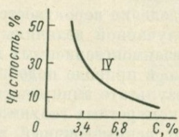
Рис. 1. Типы вариационных кривых
