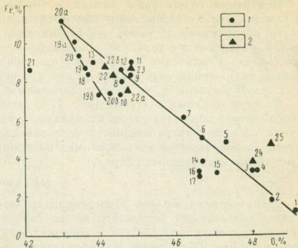
Рис. 8. Вариационная диаграмма железо — кислород в горных породах литосферы
