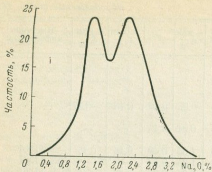
Рис. 17. Двугорбность кривой распределения натрия в кристаллических сланцах литосферы
