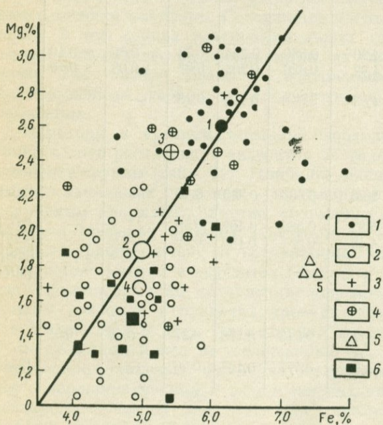
Рис. 12. Вариационная диаграмма железо — магний в средних породах
