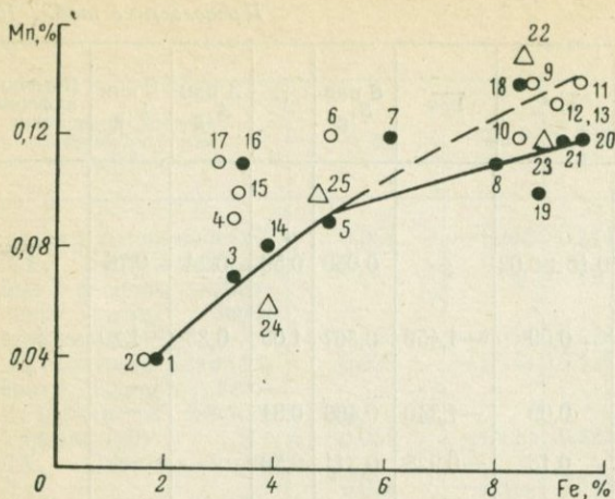
Рис. 23. Вариационная диаграмма марганец — железо в горных породах. Усл. обозначения см. на рис. 22.
