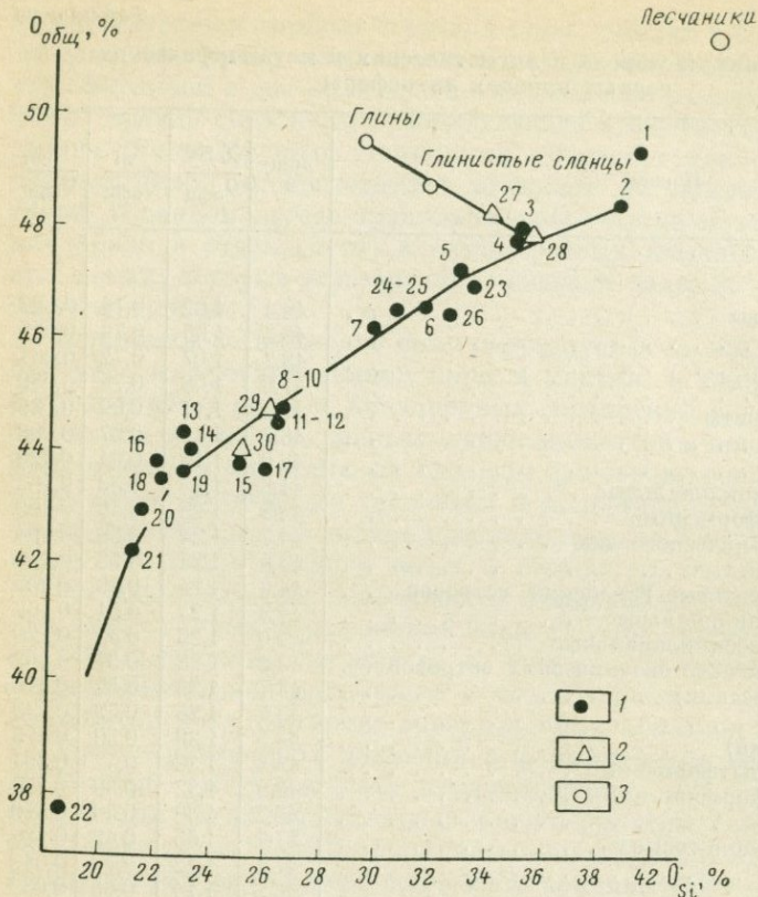
Рис. 3. Зависимость между общим содержанием кислорода ( O_{общ} ) и частью кислорода, связанного с кремнием ( O_{Si} ) в горных породах литосферы (номера пород см. в табл. 14)
