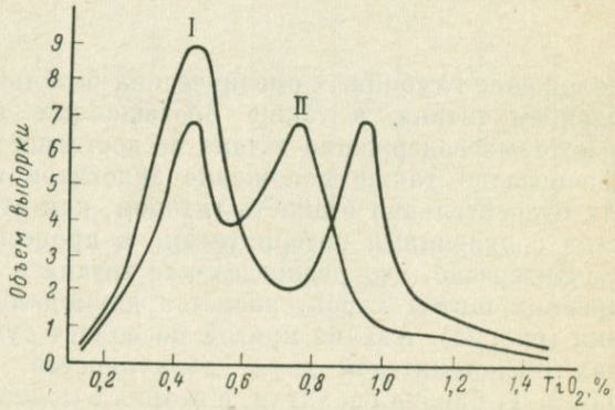
Рис. 21. Двумодальная кривая распределения титана в гранодиоритах шцитов:
