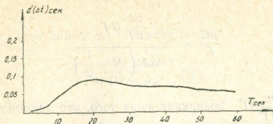
Рис. 3. Абсолютная ошибка фазовой характеристики типowego прибора СК.
