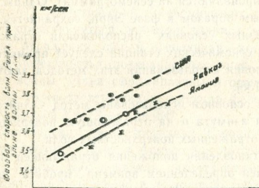
Рис. 38. Сравнительная зависимость между фазовой скоростью волн Релея при длине волны 110 км и осредненной аномалией Буге для территории США, Японии, Кавказа.
