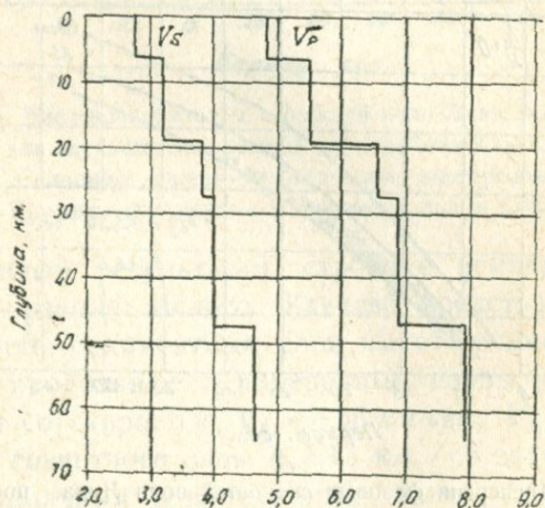
Рис. 30. Изменение скоростей продольных и поперечных сейсмических волн в зависимости от глубины земной коры.
