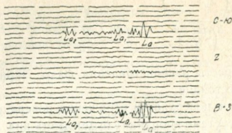
Рис. 39. Фотокопия сейсмограммы зангезурского землетрясения 9/VI 68 г.
