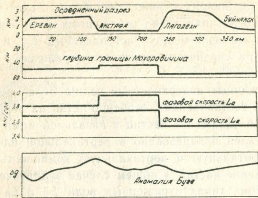
Рис. 37. Корреляция между фазовой скоростью волн Релея, рельефом земной поверхности и гравитационной аномалией Буге по трассам Ереван—Актафа—Лагодехи—Буйнакск—Кизляр.
