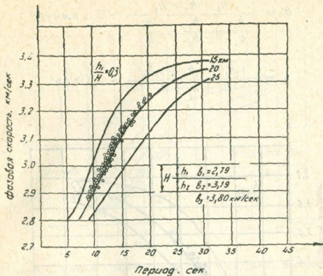
Рис. 26. Дисперсия фазовых скоростей волн Релея, построенная для верхнего слоя земной коры района Кавказа.
