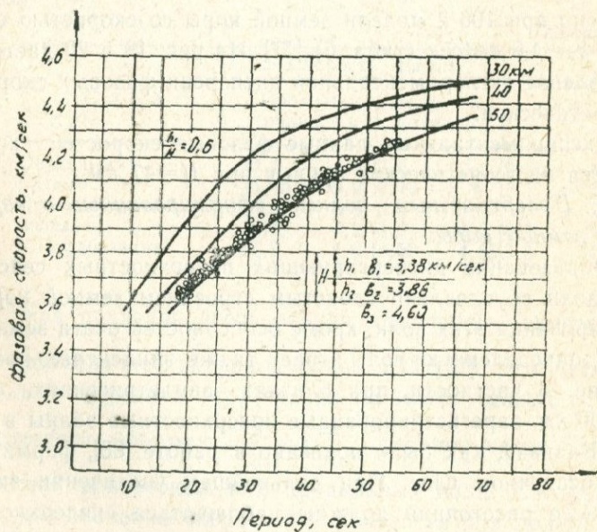
Рис. 20. Дисперсия фазовых скоростей волн Лява, построенная для земной коры в районе Кавказа. Сплошные линии—теоретические дисперсионные кривые. Кружки—полученные экспериментальные точки.
