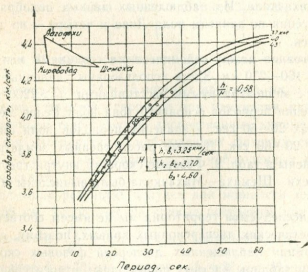
Рис. 34. Дисперсия фазовых скоростей волн Лява внутри треугольника сейсмических станций Лагодехи—Кировабад—Шемаха.
