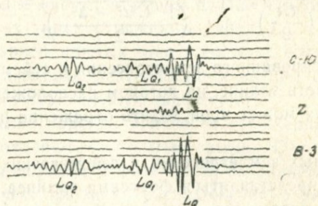
Рис. 40. Фотокопия сейсмограммы зангезурского землетрясения 15/VI 68 г.
