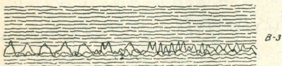
Рис. 15. Запись поверхностной волны Релея с наложением обертона.
