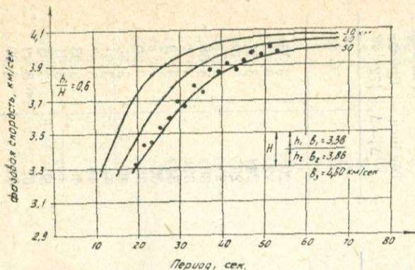
Рис. 7. Дисперсия фазовых скоростей волн Релея для землетрясения 4 сентября 1965 г. (о. Кадьяк) по трассе Нахичеван — Тбилиси, рассчитанная на ЭВЦМ. Сплошные линии — теоретические кривые. Черные кружки — полученные экспериментальные точки.
