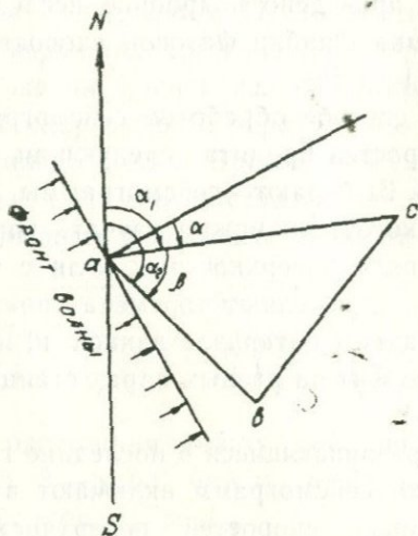
Рис. 2. Распространение плоского волнового фронта через треугольник станции.
