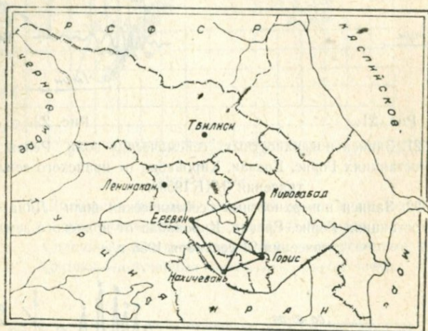
Рис. 25. Расположение исследуемых треугольников сейсмических станций в районе Малого Кавказа.
