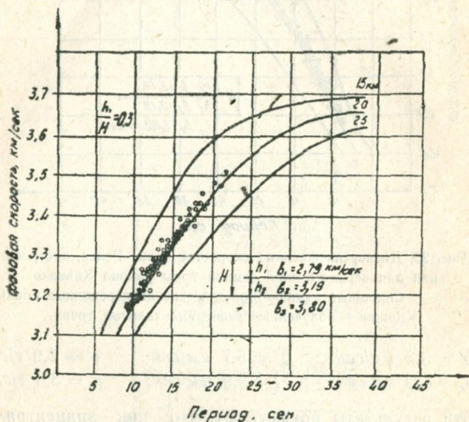
Рис. 27. Дисперсия фазовых скоростей волн Лява, построенная для верхнего слоя земной коры района Кавказа. Сплошные линии—теоретические дисперсионные кривые. Кружки—полученные экспериментальные точки.
