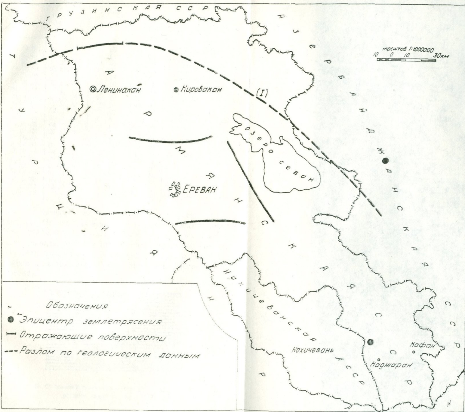
Рис. 42. Схема эпицентра и отражающих поверхностей.
