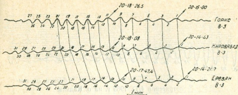
Рис. 13. Записи поверхностных сейсмических волн на станциях Горис, Кировабад, Ереван от перуанского землетрясения 15 января 1958 г.
