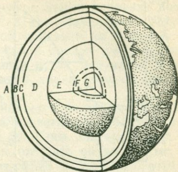
8.2. Строение «твердой» Земли. Границы между геосферами А и В, D и E, F и G резкие, между В и С, E и F условные, так как переход постепенный (Белоусов В. В. и др., 1972 г.).
