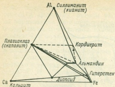
19.2. Минеральные парагенезисы гранулитовой фации (по П. Эсколе).
