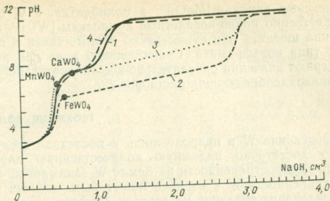
17.2. Порядок выделения вольфраматов при нейтрализации растворов кремневольфрамовых гетерополиоксидов раствором NaOH [Gundlach H., 1967 г.].
