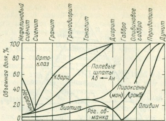
11.4. Последовательность образования пород как результат проявления кристаллизационной дифференциации по принципу Боуэна.
