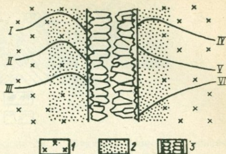
16.1. Изменение содержания минералов и значений пористости в зонах околожильной грейзенизации на вольфрамитовых месторождениях Забайкалья.
