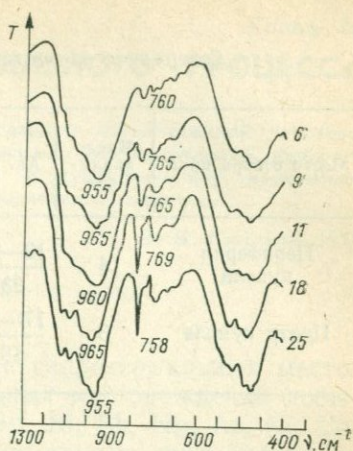
15.5. ИК-спектры поглощения амфиболов из скарнов Приладожья.
