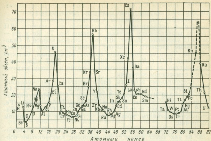
10.8. Геохимическая таблица элементов, расположенных на кривой атомных объемов [Эляшевич М. А., Штейнман Р. Я., 1970 г.].
