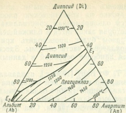
11.1. Диаграмма плавкости системы альбит—анортит—диопсид в массовых долях, %.
