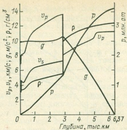
8.1. Физические характеристики вещества Земли на разной глубине.
