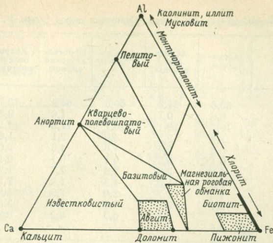
19.5. Диаграмма Al_2O_3-CaO-FeO+MgO , отражающая поля состава пяти химических классов метаморфических пород. Показан также состав главнейших минералов изверженных и осадочных пород (кроме кварца, щелочных полевых шпатов и фельдшпатовидов). Границы между классами проведены условно [Fyfe W. S., Turner F. J., Verhoogen J., 1958 г.].
