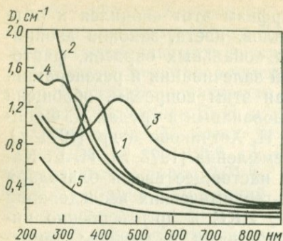
13.8. Спектры оптического поглощения цитринов в ультрафиолетовой и видимой областях (по Балицкому В. С., Лисицкой Е. Е. [1981 г.]).
