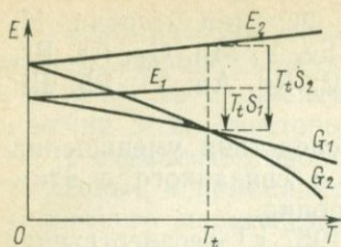
9.3. Соотношение энергии и температур полиморфных модификаций [Burger M., 1948 г.].
