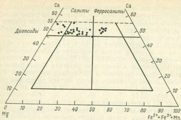
15.2. Химический состав пироксенов в числе атомов Ca, Mg, Fe 2+ +Fe 3+ +Mn на формульную единицу, %, по данным табл. 15.3.
