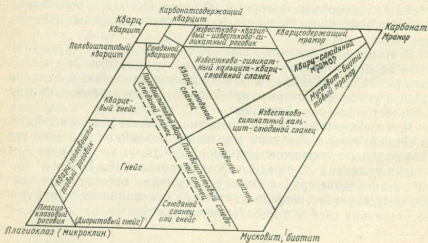
19.4. Метаморфические породы амфиболитовой фации [Винклер Г., 1969 г.].
