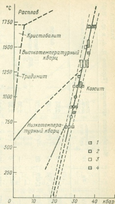
13.6. Области устойчивости различных модификаций кремнезема [Торопов Н. А. и др., 1965 г.].
