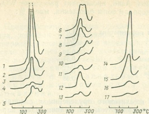
17.3. Кривые термолюминесценции шеелита.
