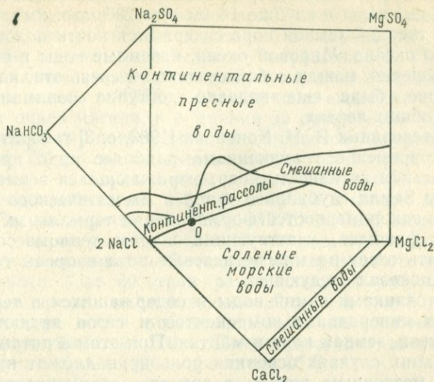
20.1. Связь различных по составу типов континентальных и морских вод. O — океаническая вода при солёности 35 г/кг [Валяшко М. Г., 1962 г.].
