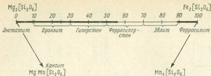
12.6. Смесимость фаз в системе Mg_2[Si_2O_6]-Fe_2[Si_2O_6]-Mn_2[Si_2O_6] в молярных долях, %.
