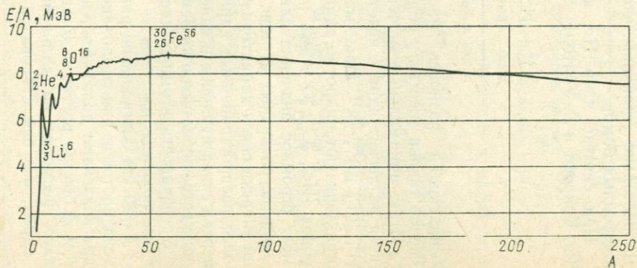
4.3. Зависимость удельной энергии связи нуклонов в ядре от массового числа.
