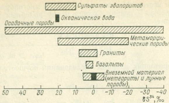
5.2. Отношение S 34 /S 32 в некоторых геологически важных объектах (δS 34 относительно троилита) [Хёфс И., 1983].
