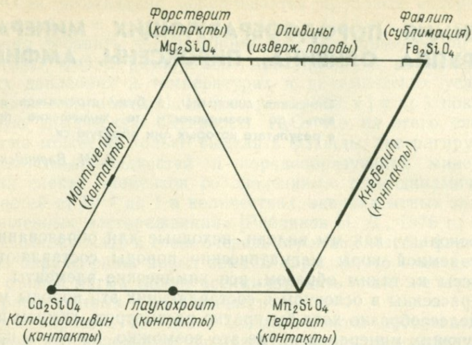
12.1. Смесимость фаз в природных системах Mg_2SiO_4 — Fe_2SiO_4 — Mn_2SiO_4 — Ca_2SiO_4 — Mg_2SiO_4 .
