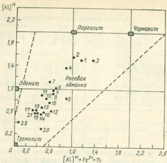
15.4. Колебания химических составов кальциевых амфиболов, выраженных в числе атомов [Al]^{VI} + Fe^{3+} + Ti и Al^{IV} на формульную единицу.
