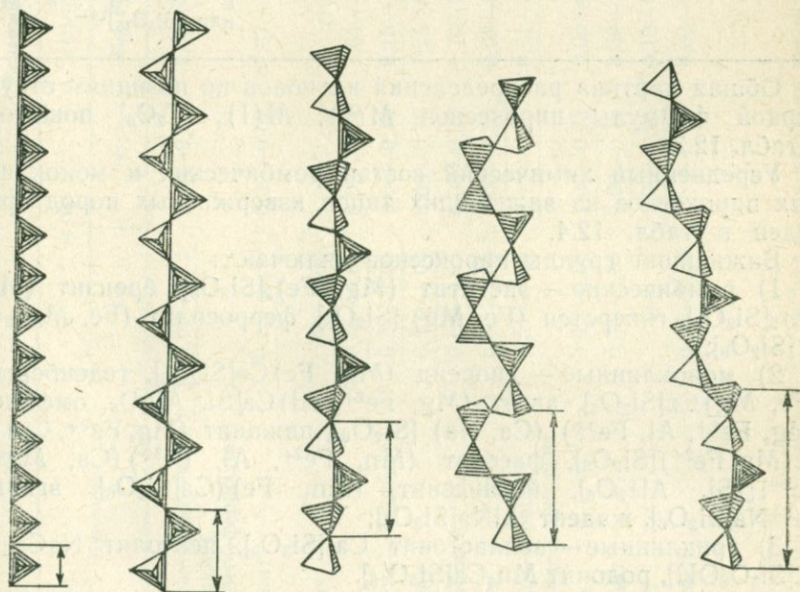
12.5. Главнейшие типы цепочек \text{SiO}_4 -тетраэдров.
