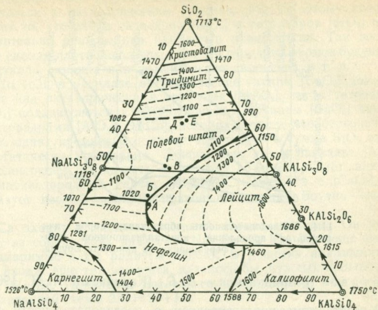
11.3. Диаграмма нефелин—калиофилит—кварц.
