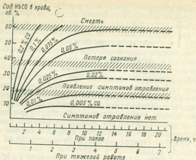
21.2. Токсичность окиси углерода по Франке [1973 г.].
