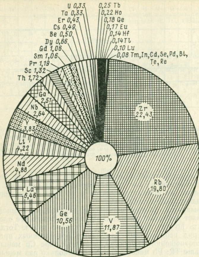
10.2. Соотношение редких элементов в земной коре [Власов К. А., 1964 г.]. Общее содержание 0,125 масс. % принято за 100 %.
