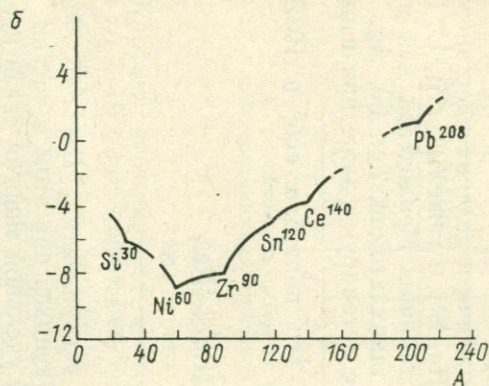
4.2. Зависимость упаковочного коэффициента от массового числа. Элементы: а — легкие, б — тяжелые.
