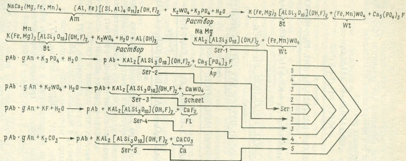
13.4 Схема образования зональных жильбертитов.
