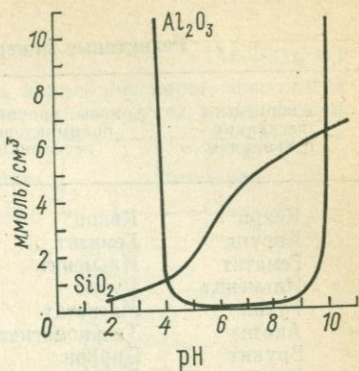
18.5. Влияние pH среды на растворимость кремнезема и глинозема [Correns С. W., 1949 г.].
