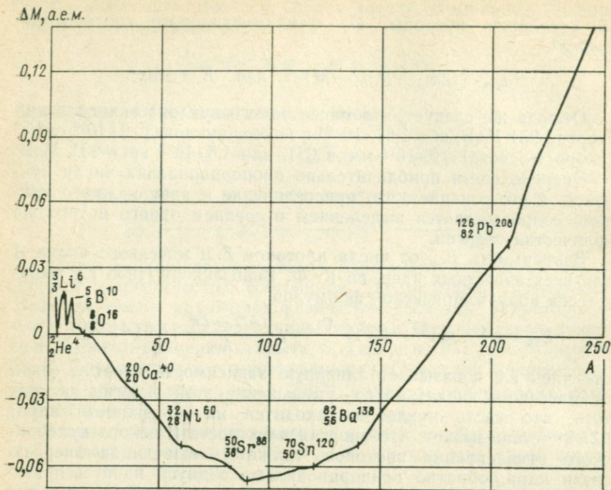
4.1. Дефект масс.
