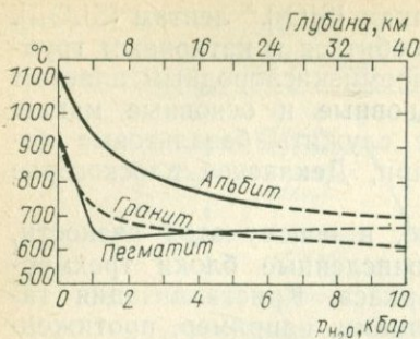
11.6. Влияние паров воды на температуры плавления альбита, гранита, пегматита [Tuttle O. F., Bowen N. L., 1958].
