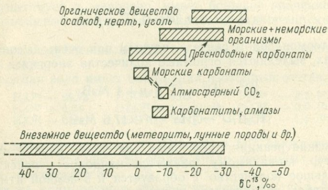
5.3. Отношение C 13 /C 12 в наиболее распространенных соединениях углерода (δC 13 относительно PDB) [Хёфс И., 1983].
