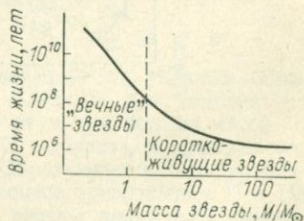
6.4. Продолжительность эволюции звезды в зависимости от ее массы.
