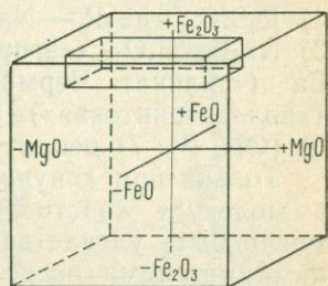
12.3. Объемная диаграмма факторных нагрузок на Fe 2 O 3 , FeO и MgO, в которой выделена область факторного пространства, заселенная фигуративными точками никеленосных интрузий.
